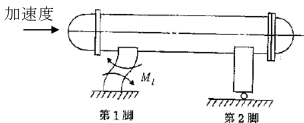
軸方向加速度により 脚が受ける局部モーメント
