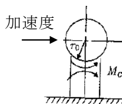
軸直角方向加速度により 脚が受ける局部モーメント
