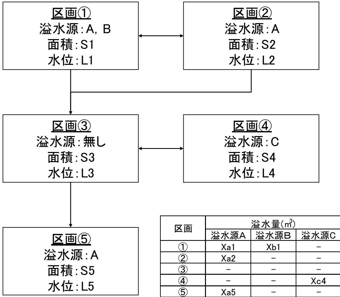
第7.6.2-1図 地震時溢水伝播評価のモデルケースの設定
