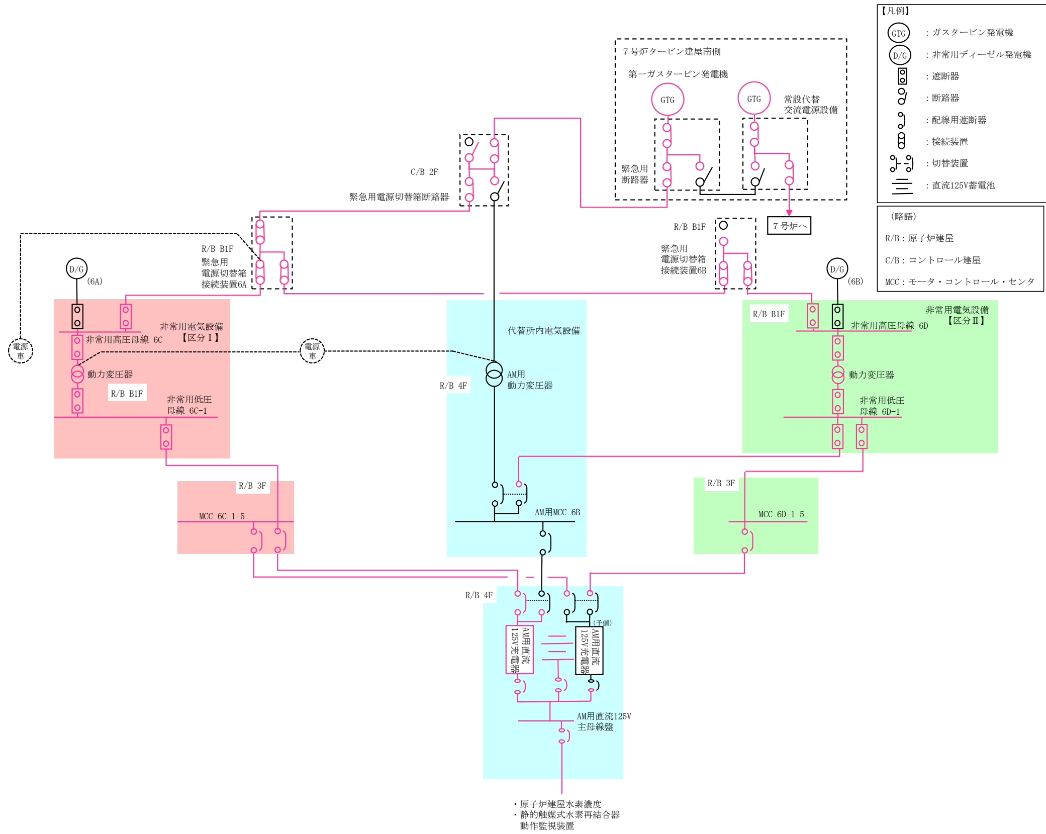
図 2-56 単線結線図 (6号炉)
