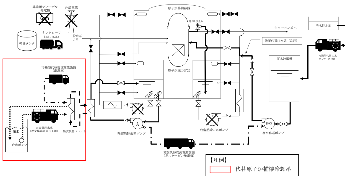
第 1-2 図 代替原子炉補機冷却系 系統概要図
