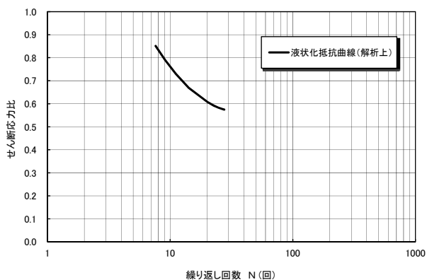
洪積砂質土層Ⅱ
