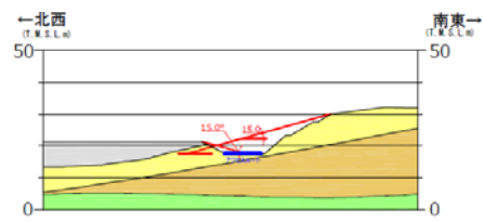
③断面
