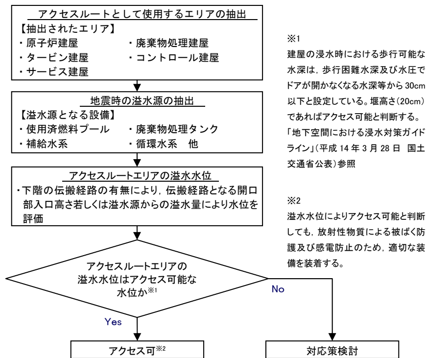
第1図 地震随伴の内部溢水評価フロー図
