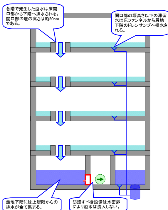
第2図 水位評価概要図
