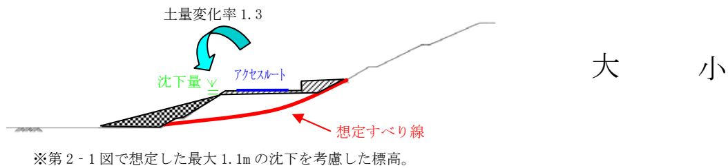
第 5 図 斜面のすべり範囲に応じた沈下量のイメージ
