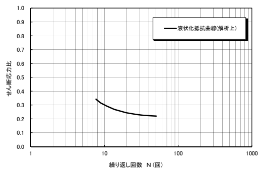
洪積砂質土層Ⅰ
