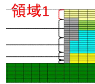
1F床以深(T.M.S.L.12.3m~)
