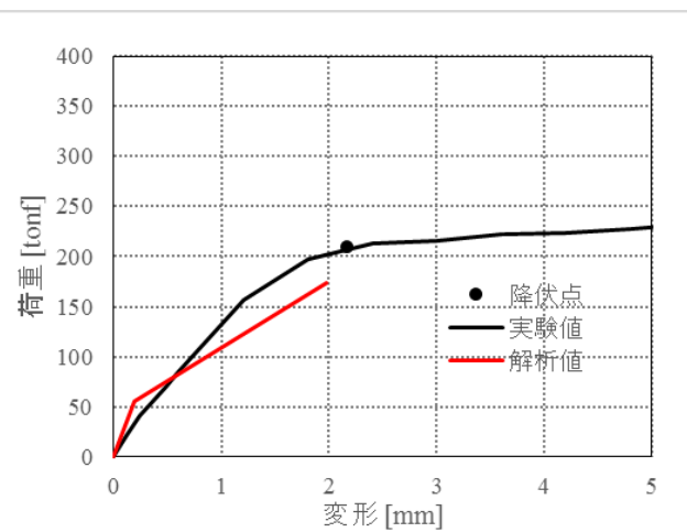
第 4-8 図 実験 2 SC150-3
