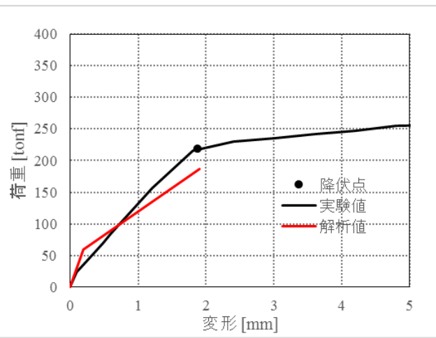
第 4-6 図 実験 2 SC150-0
