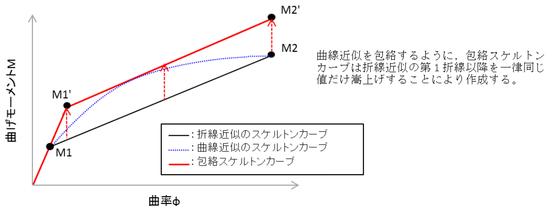
第 4-1 図 包絡スケルトンカーブの概念図
