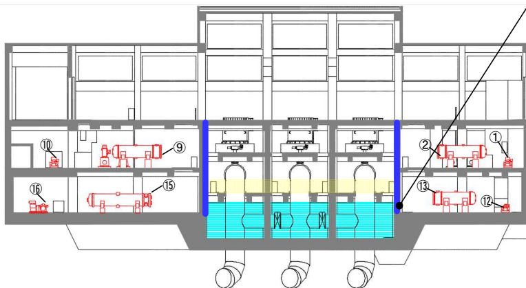
B-B断面
