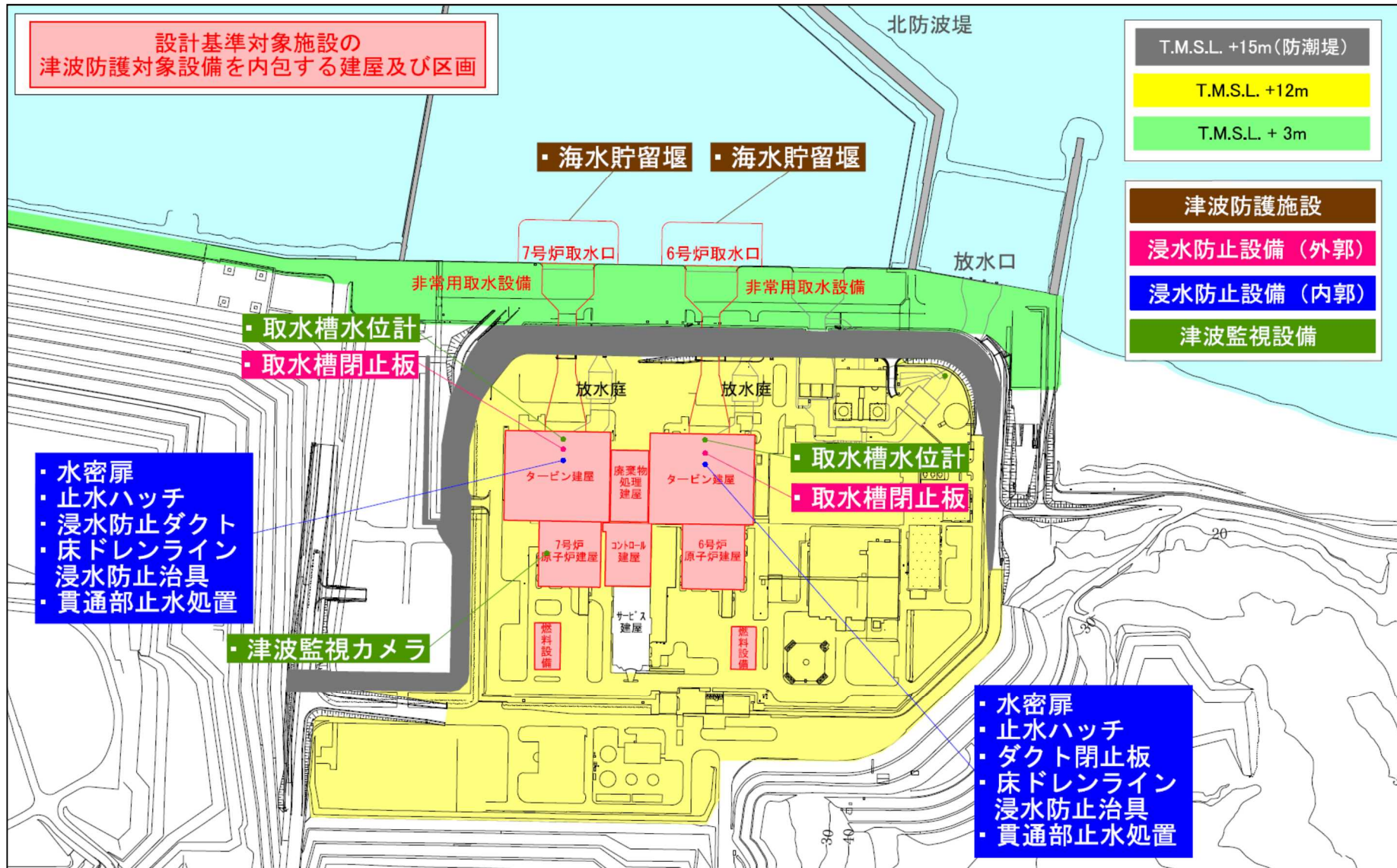
第 2.1-1-3 図 敷地の特性に応じた津波防護の概要 (大湊側詳細)
