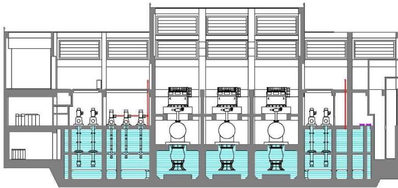
A-A 断面
