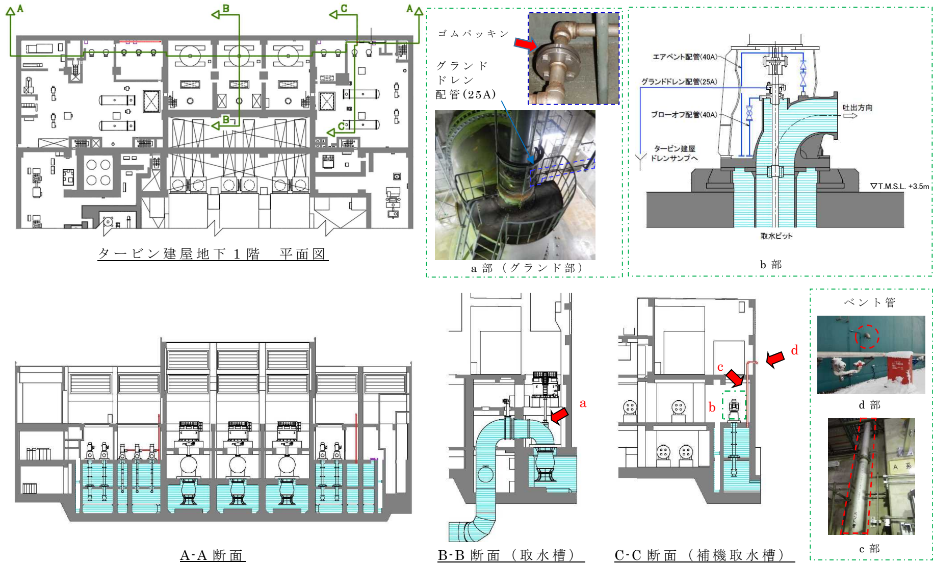
第 2.3-4-1 図 取水槽及び補機取水槽上部床面を介した漏水の可能性の検討 (6 号炉の例)
