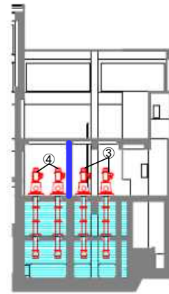
C-C断面
