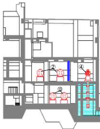
B-B断面
