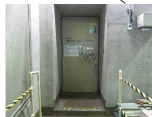
水密扉 設置例
