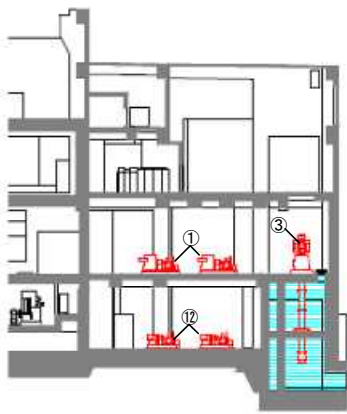
A-A断面
