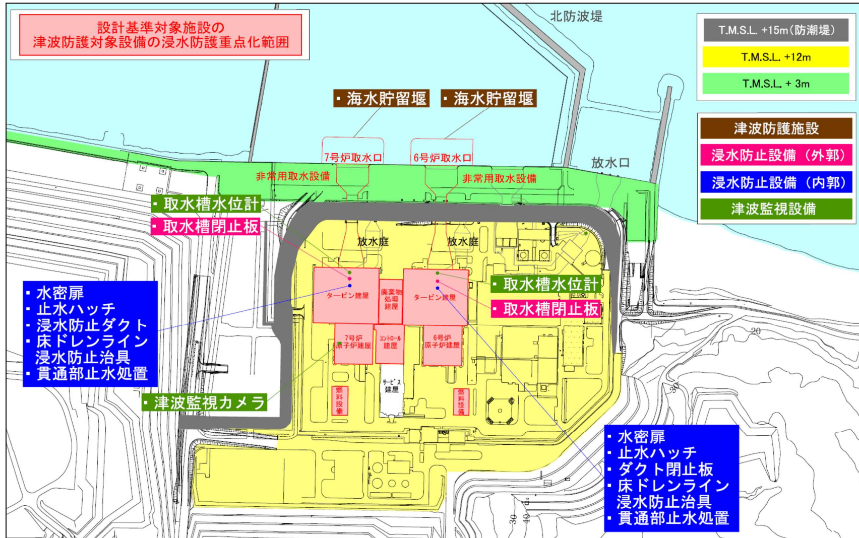
第 2.4-1 図 浸水防護重点化範囲概略図
