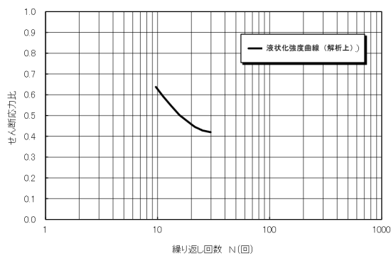
第 11-9-20 図 液状化強度曲線
