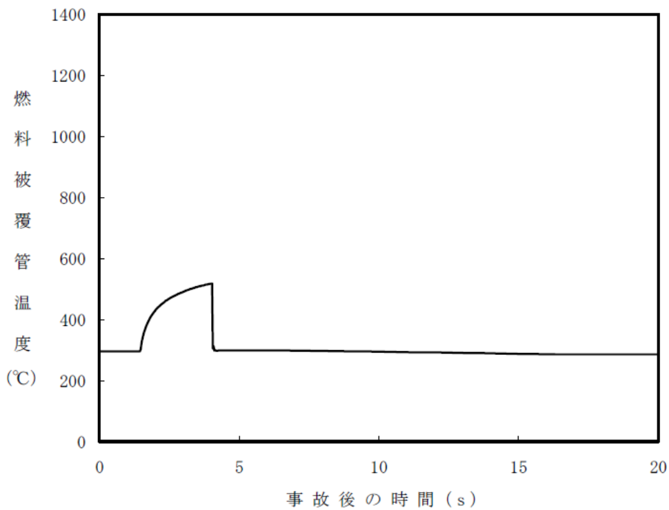
補足第 3. 6. 4. 1-3 図 原子炉冷却材流量の喪失 + 給水制御系の故障解析結果 (原子炉建屋起因) (2/2)
