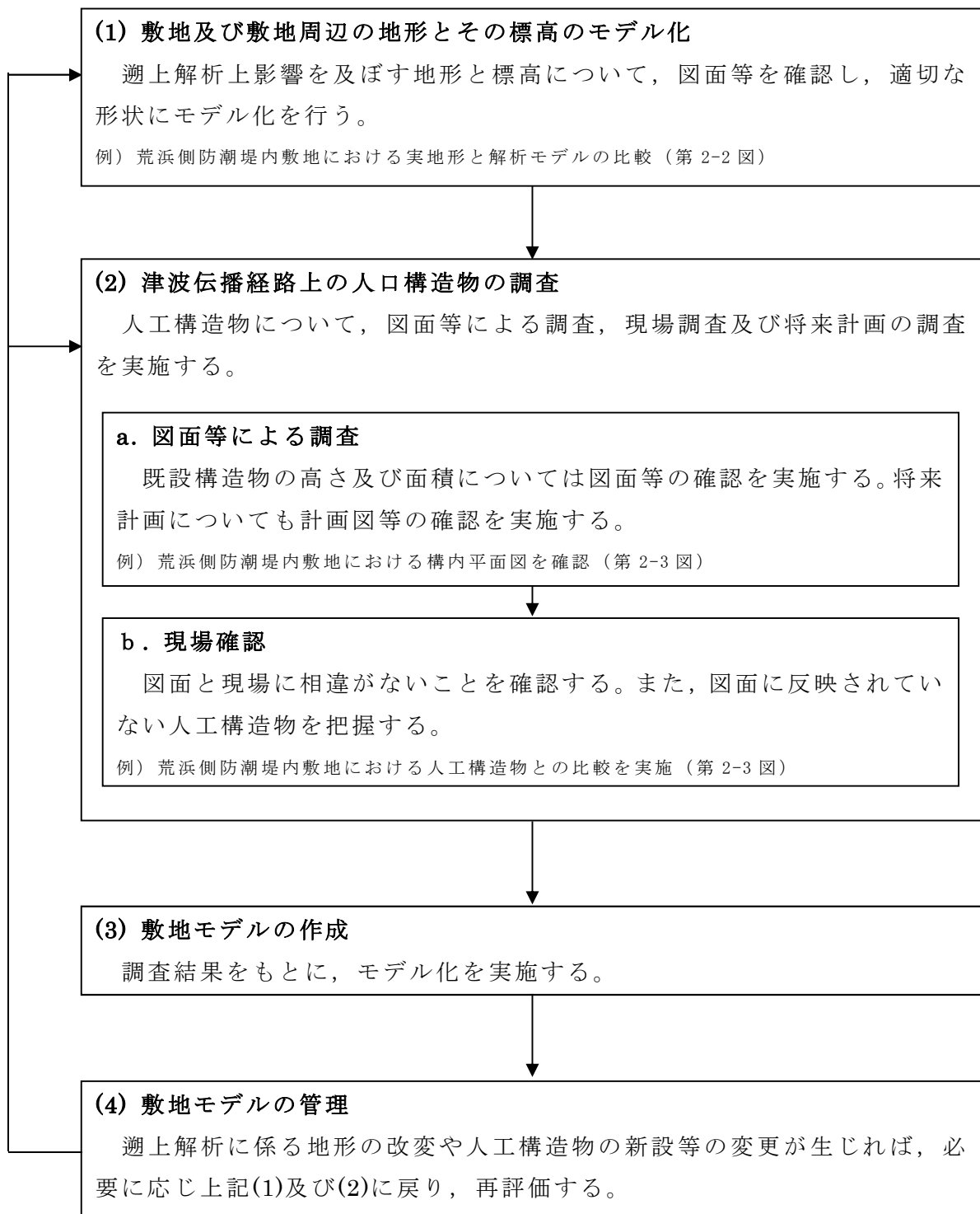
第 2-1 図 敷地モデルの作成プロセスフロー図
