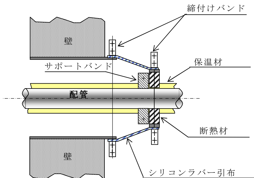
添付第 14-8 図 ブーツ構造施工例 (2/2)
