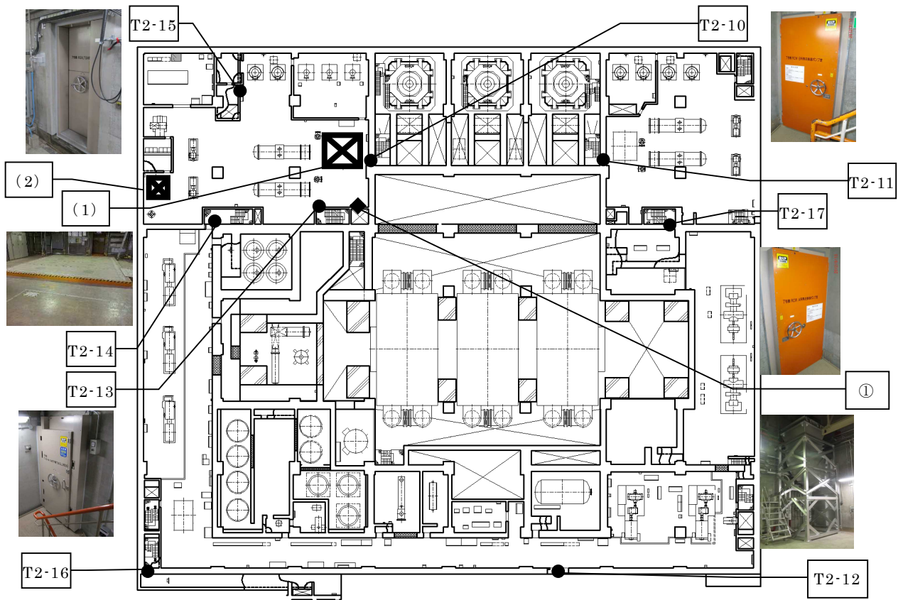
添付第 14-2-3 図 水密扉, 浸水防止ダクト及び止水ハッチの設置位置並びに施工例 (7号炉 タービン建屋地下1階)
