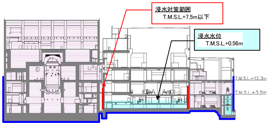
B-B 断面
