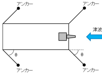
添付第 23-3 図 走錨状態
