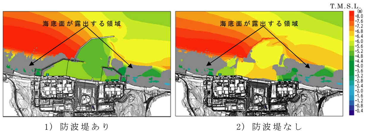
添付第 28-3 図 最低水位分布（基準津波 2）
