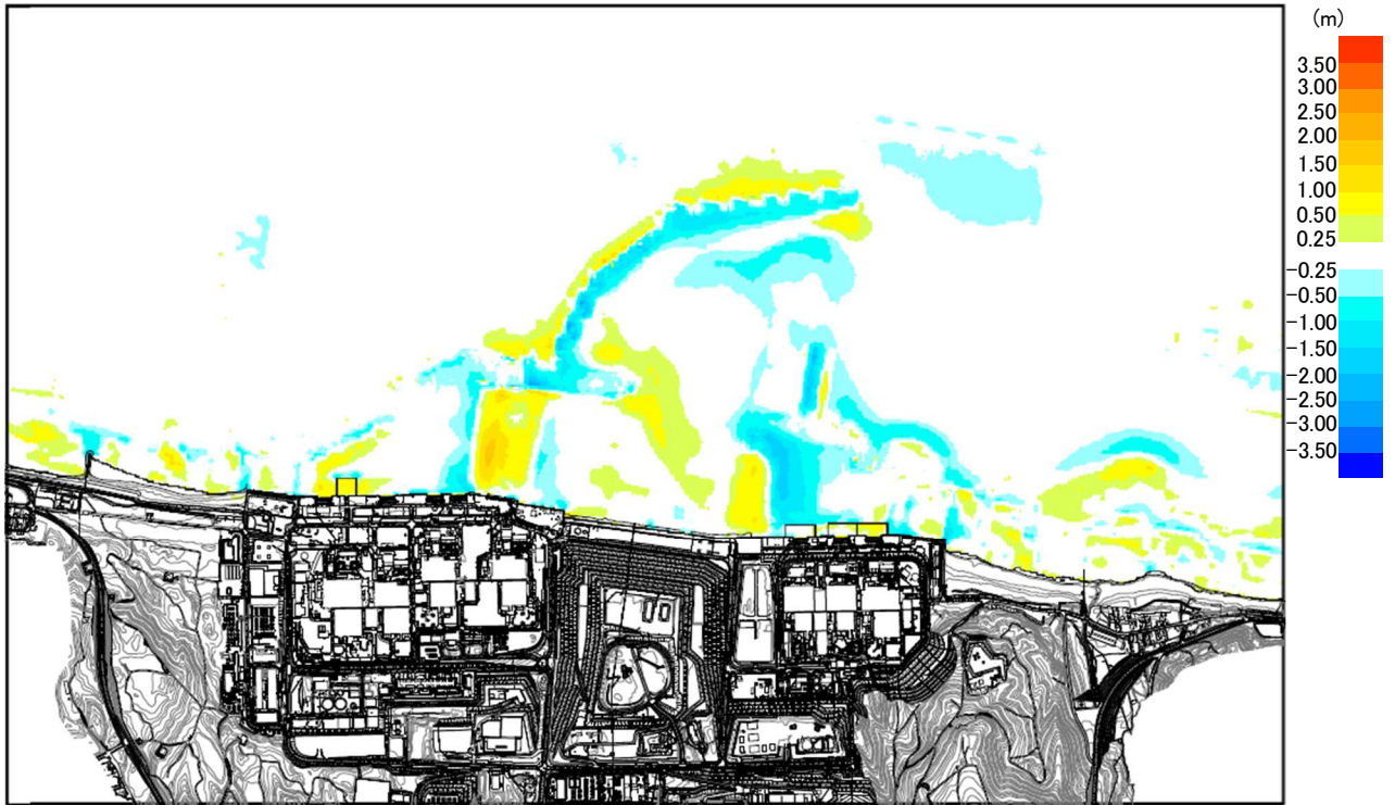
添付第 17-3 図 (4) 防波堤なし
