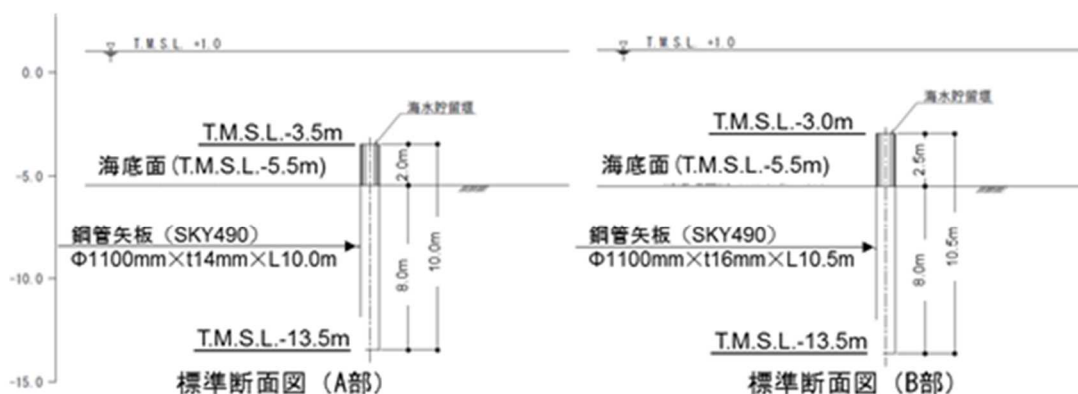
添付第 28-2 図 海水貯留堰の断面図
