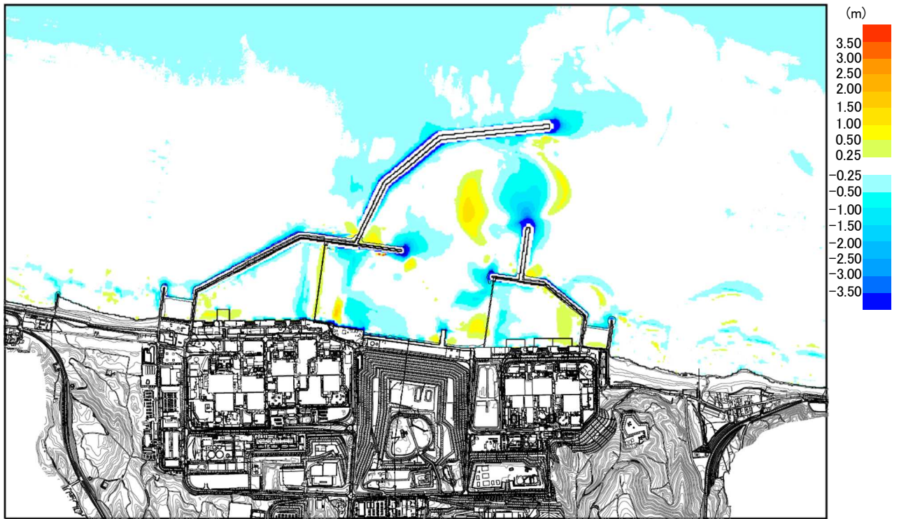
添付第 17-2 図 (6) 堆積侵食分布図 D10 相当 (0.1mm)
