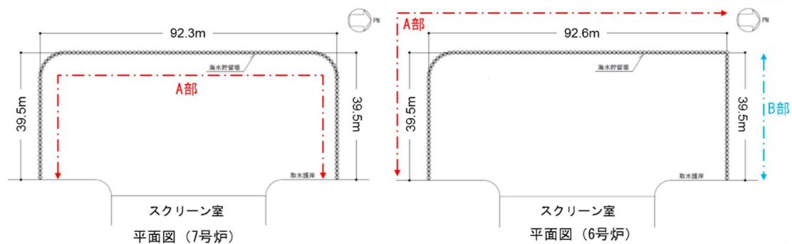
添付第 28-1 図 海水貯留堰の平面図
