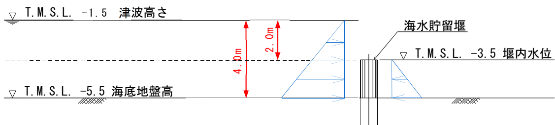
添付第 28-6 図 津波波力の作用イメージ (海水貯留堰天端高さ T.M.S.L. -3.5m の場合)
