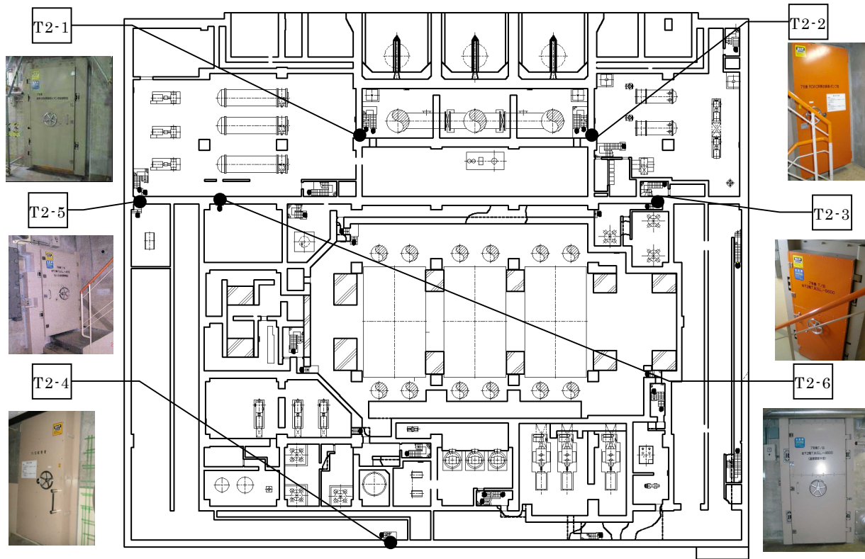
添付第 14-2-1 図 水密扉，浸水防止ダクト及び止水ハッチの設置位置並びに施工例（7号炉 タービン建屋地下2階）
