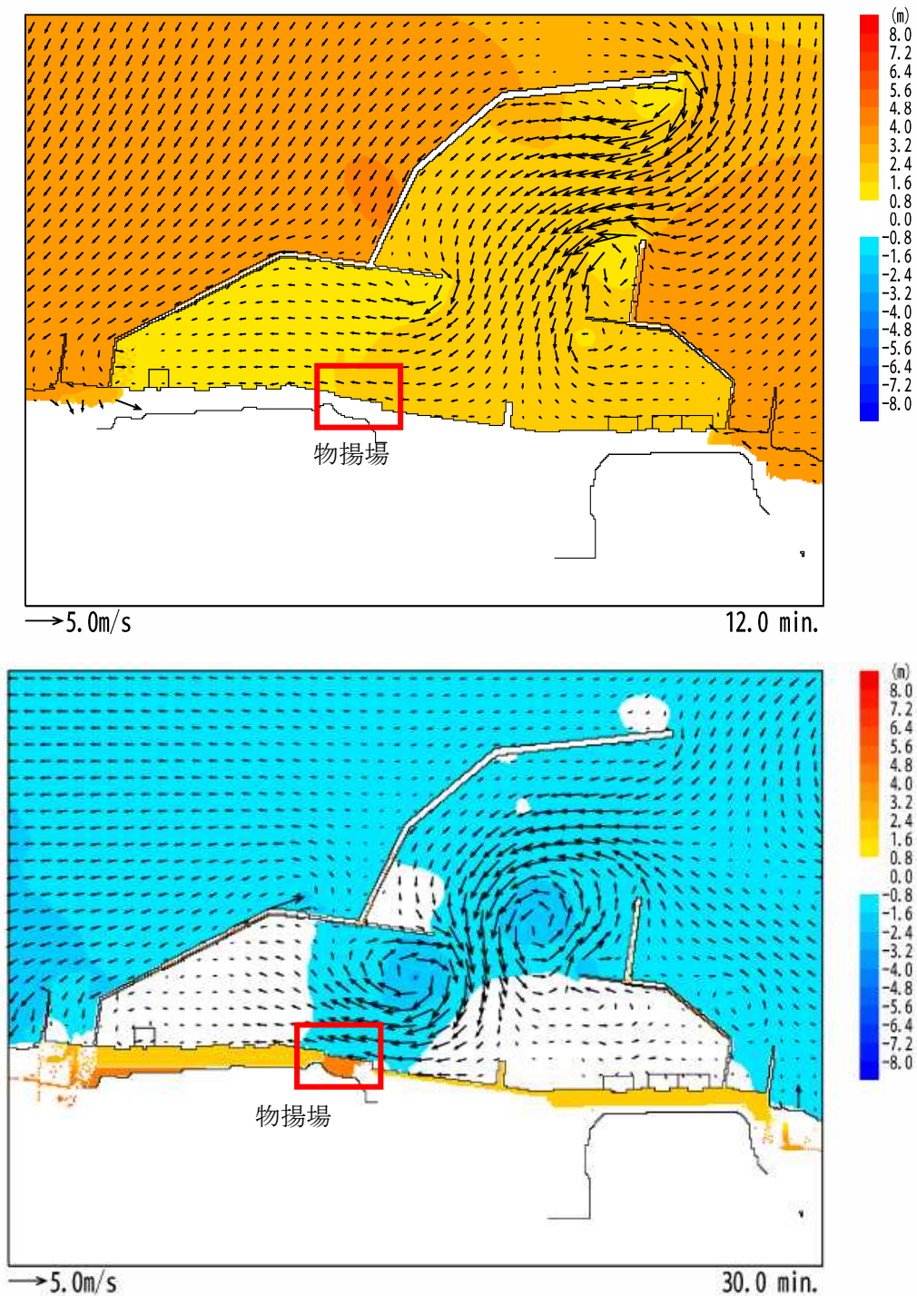
添付第 21-2 図 基準津波 3 の流向
