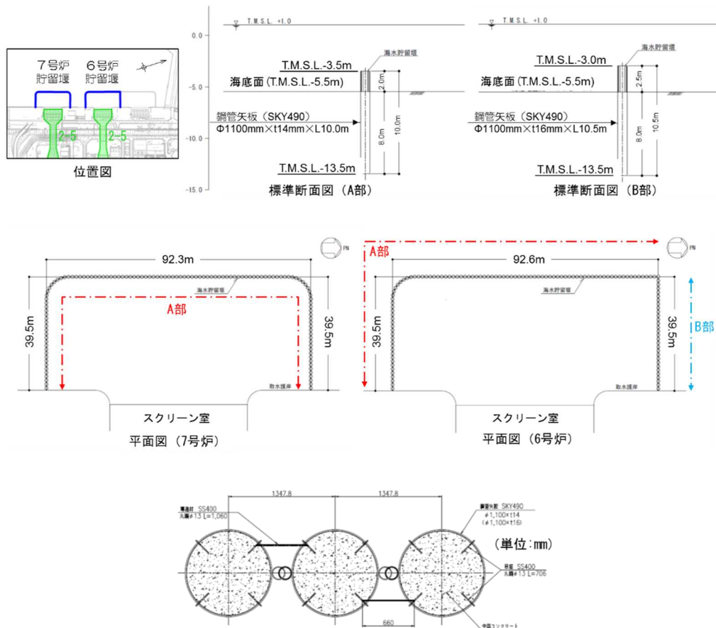
添付第 32-2 図 6 号及び 7 号炉海水貯留堰の構造概要
