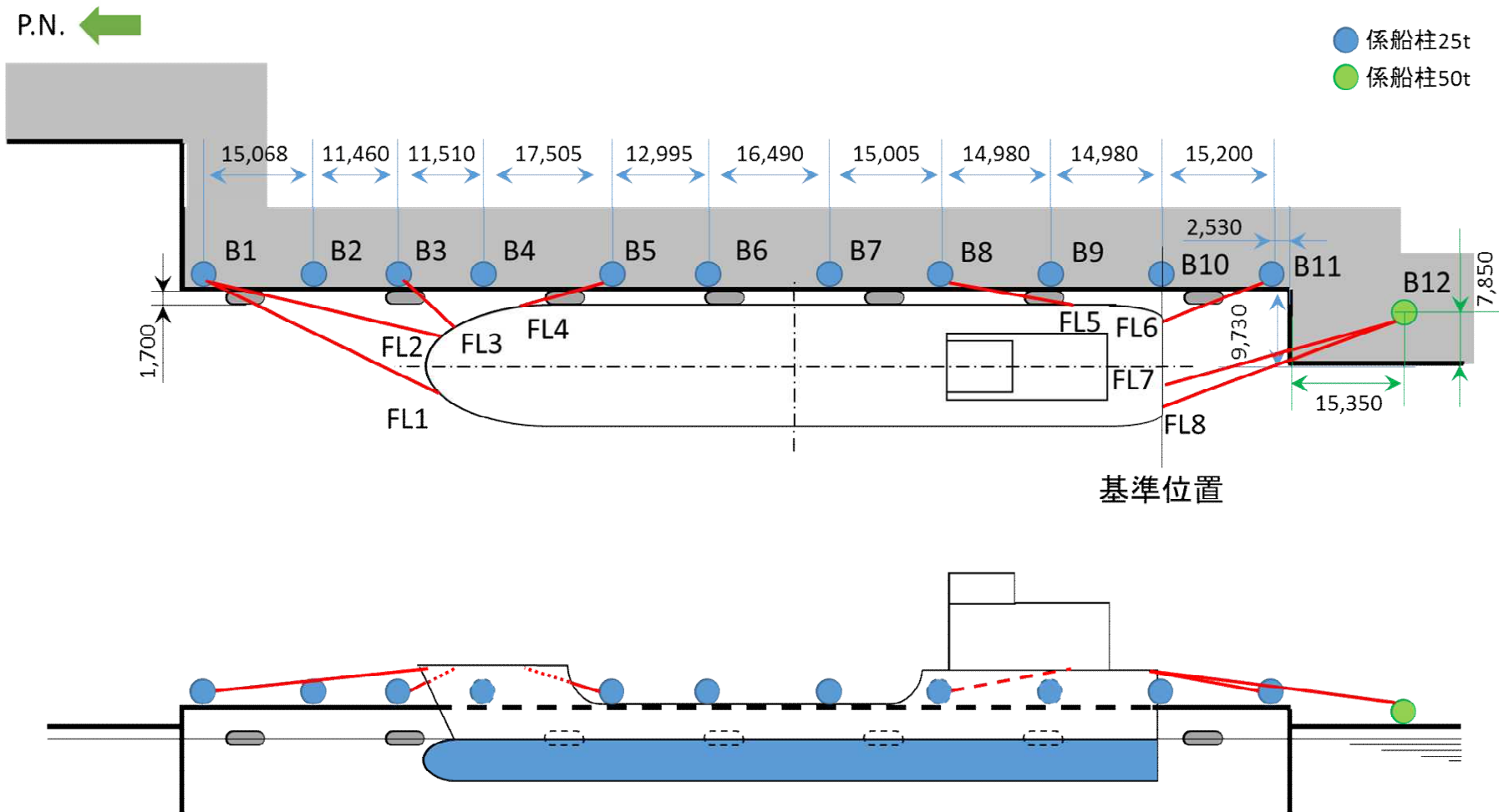
添付第 21-1 図 輸送船，係留索，係船柱の配置
