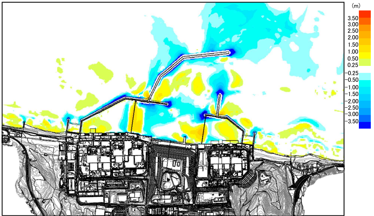
添付第 17-3 図 (1) 防波堤あり
