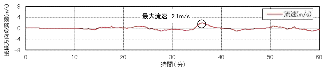
添付第21-3-2図 防波堤損傷時における基準津波3の流速（物揚場前面）
