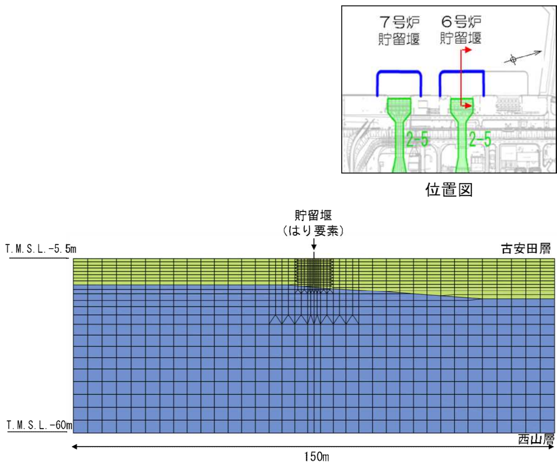
添付第 31-8 図 地震応答解析モデル
