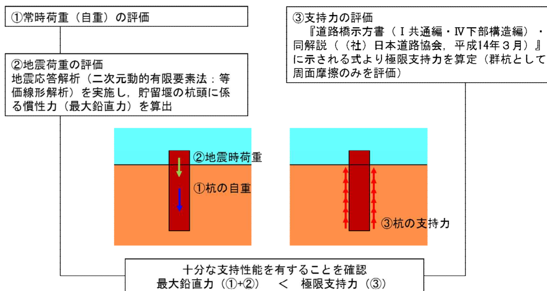
添付第 31-4 図 海水貯留堰の評価フロー
