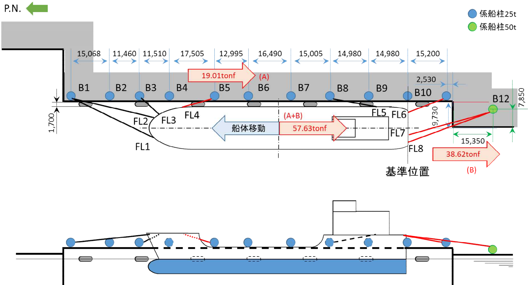
添付第 21-5 図 船首方向への移動に対する船尾方向係留力
