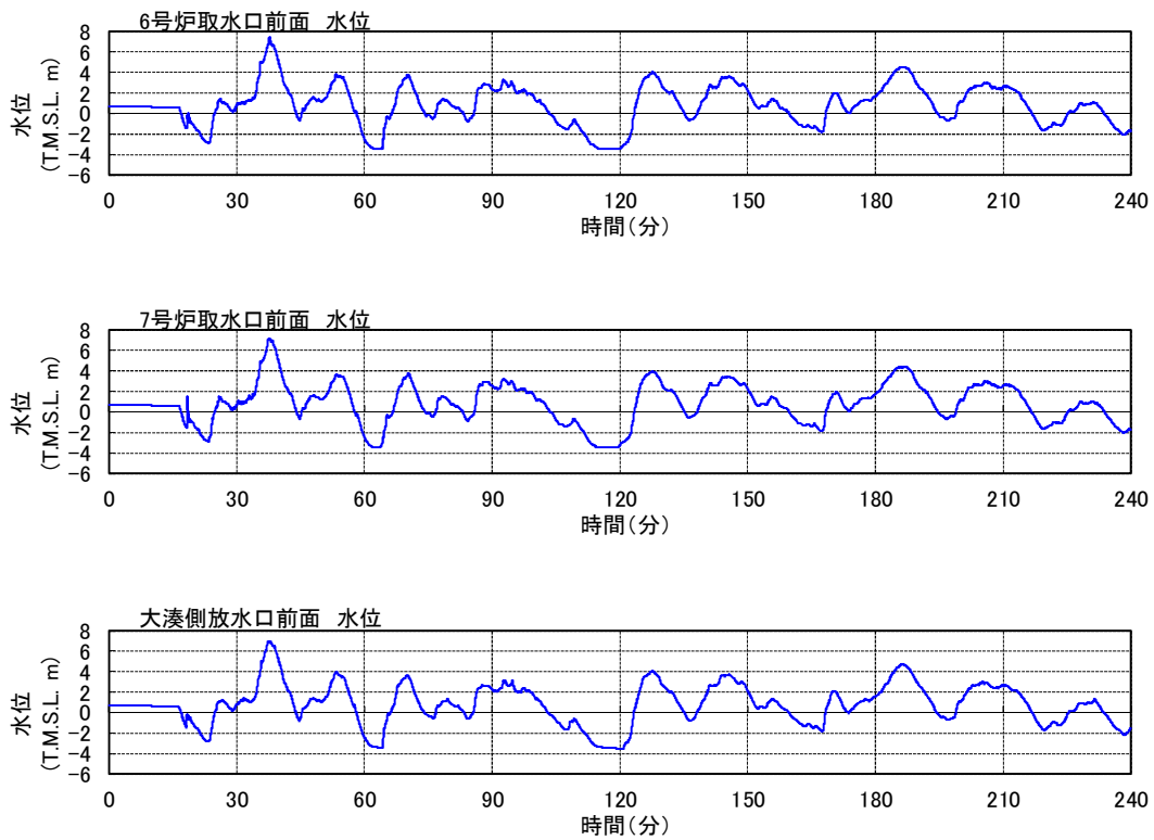
添付第13-3-1図 基準津波1の入力津波波形 (6号及び7号炉取水口前面, 大湊側放水口前面)
