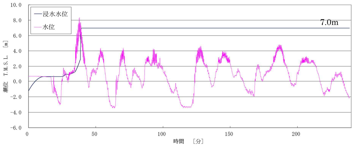
添付第13-2-4図 補機取水槽の水位及びタービン補機冷却水系熱交換器を設置するエリアの浸水水位の時刻歴波形（6号炉）
