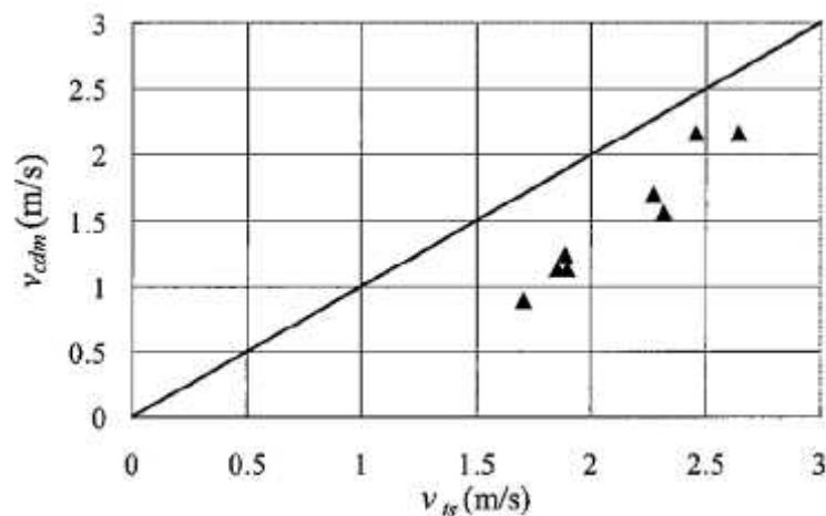
添付第 25-1 図 津波流速 v_{ts} と最大漂流速度 v_{cdm} の関係
