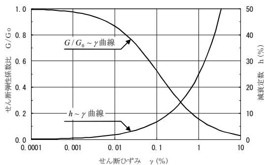
添付第 31-5 図 古安田層のひずみ依存性
