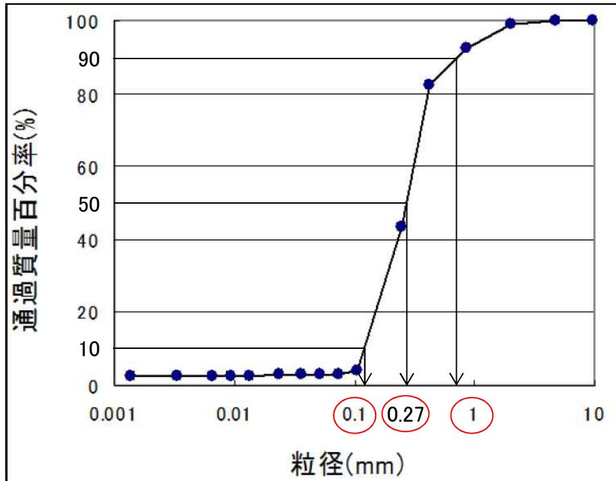
添付第 17-1 図 粒径加積曲線
