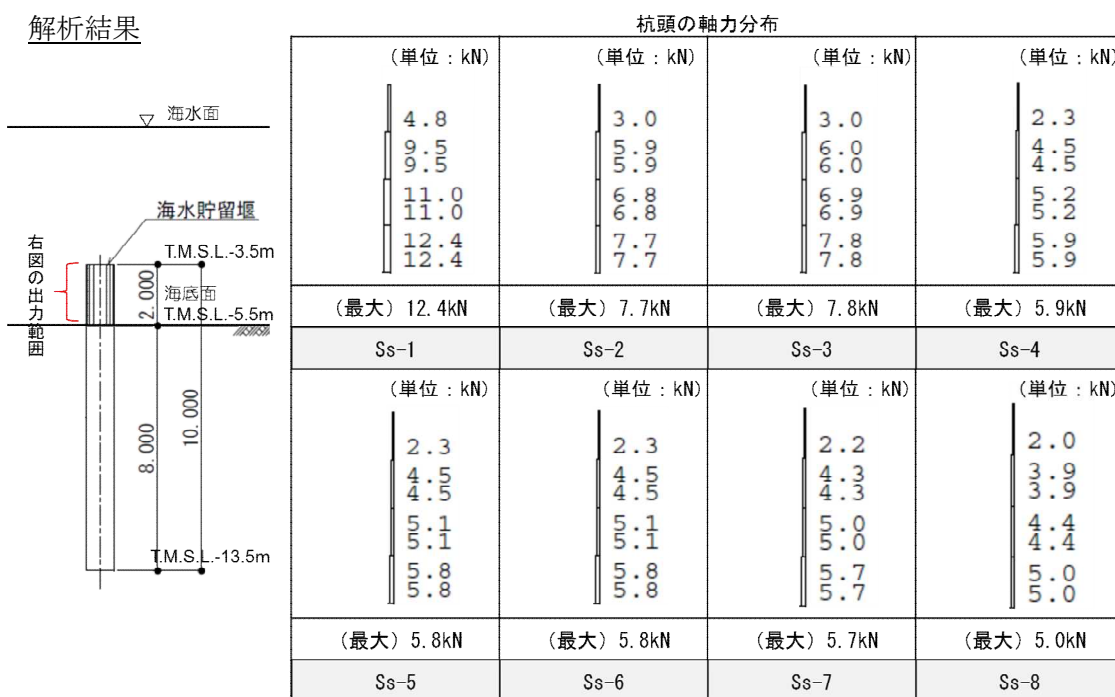
添付第 31-9 図 発生軸力分布
