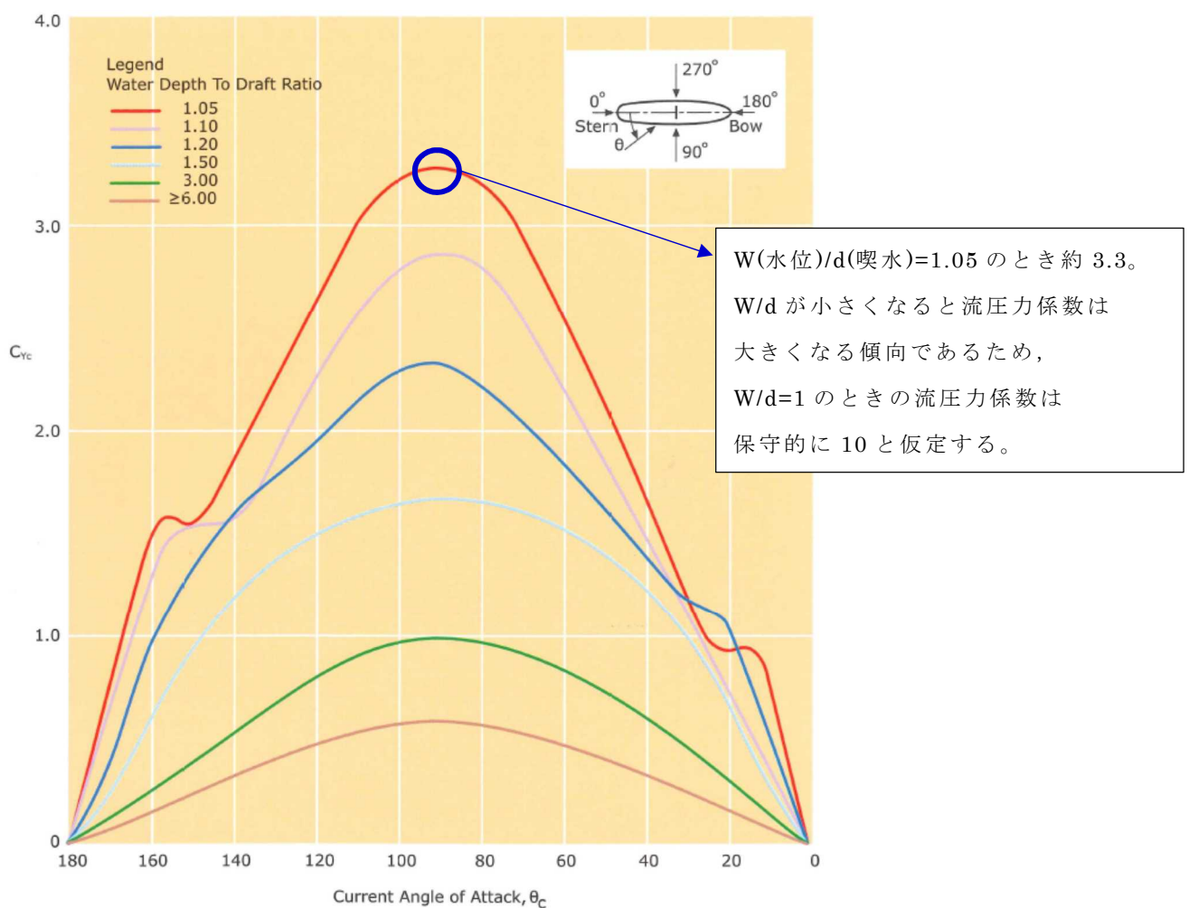
図 7 横方向の流圧力係数 1)
