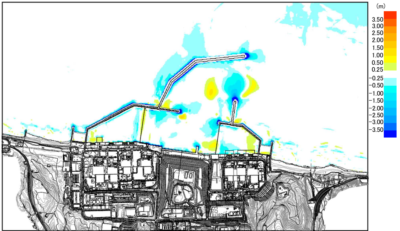
添付第 17-2 図 (3) 堆積侵食分布図 D10 相当 (0.1mm)
