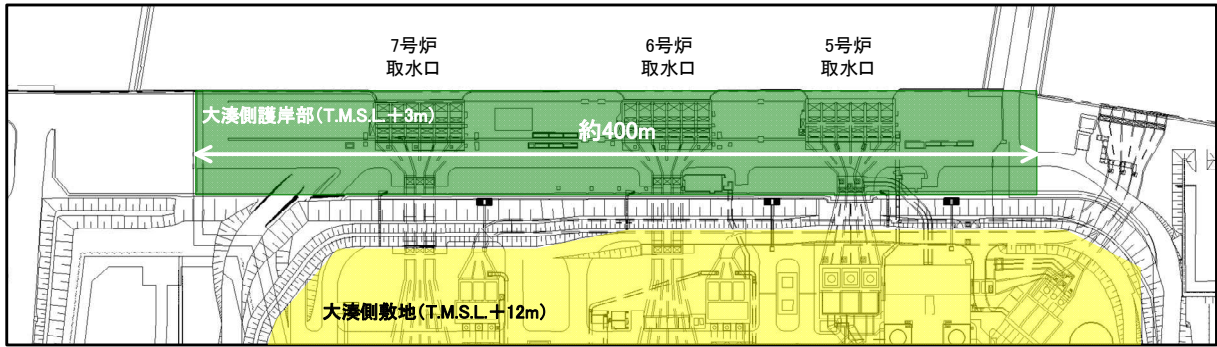
添付第 24-1 図 大湊側護岸部の概略
