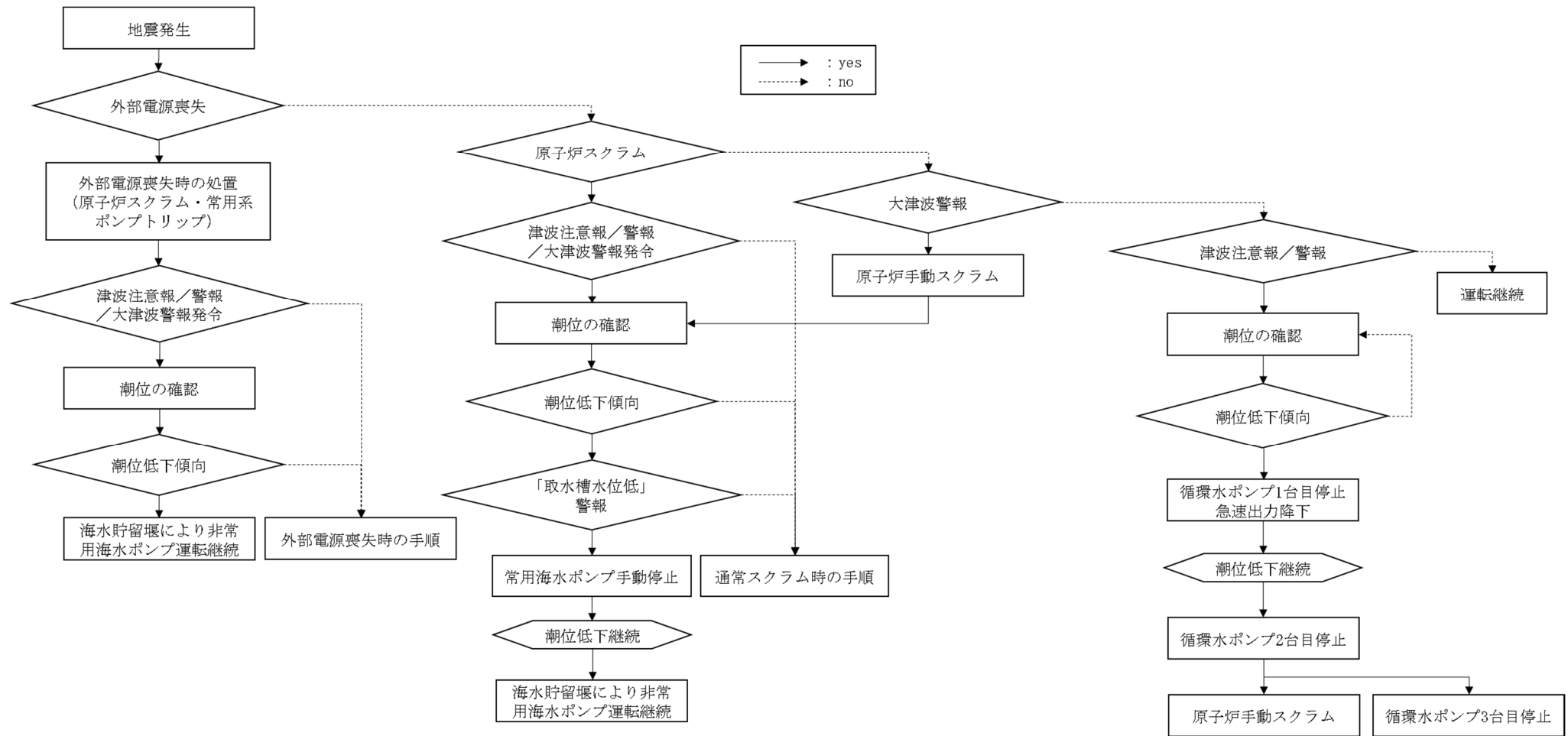
添付第 26-1 図 地震・津波時の対応フロー
