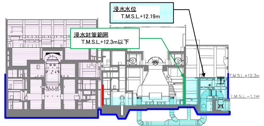
D-D 断面
