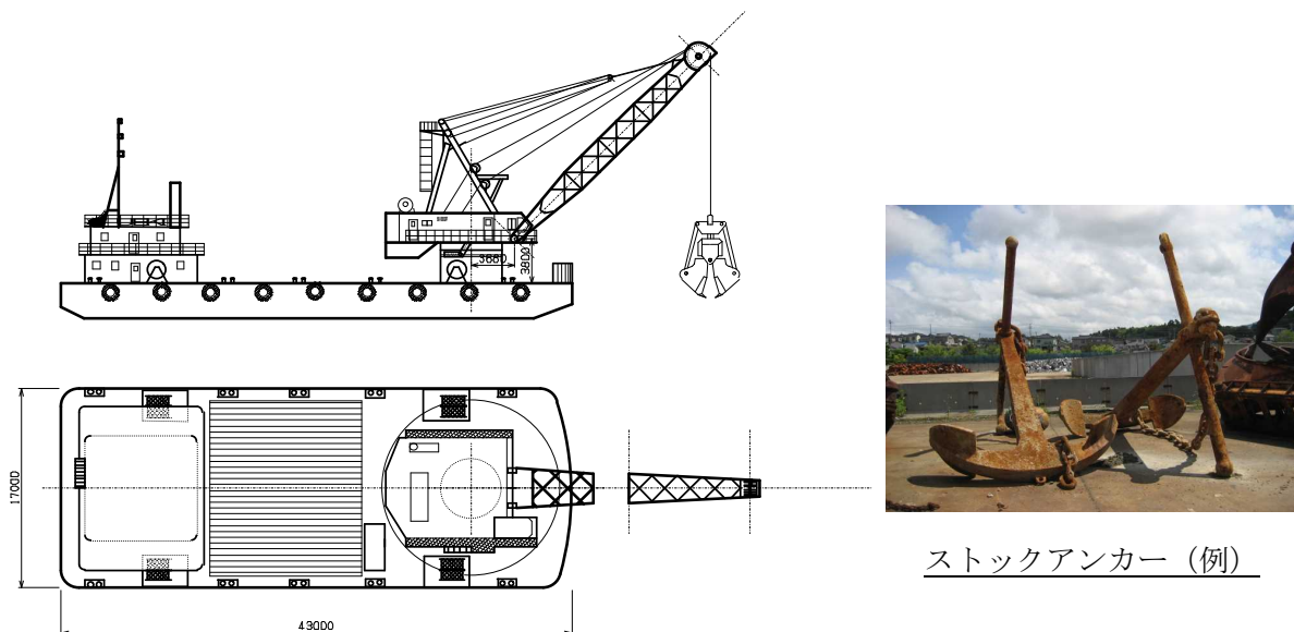
添付第 23-1 図 浚渫船の外形図
