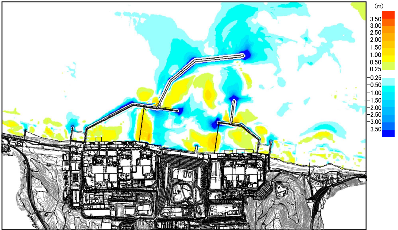
添付第 17-3 図 (3) 防波堤あり
