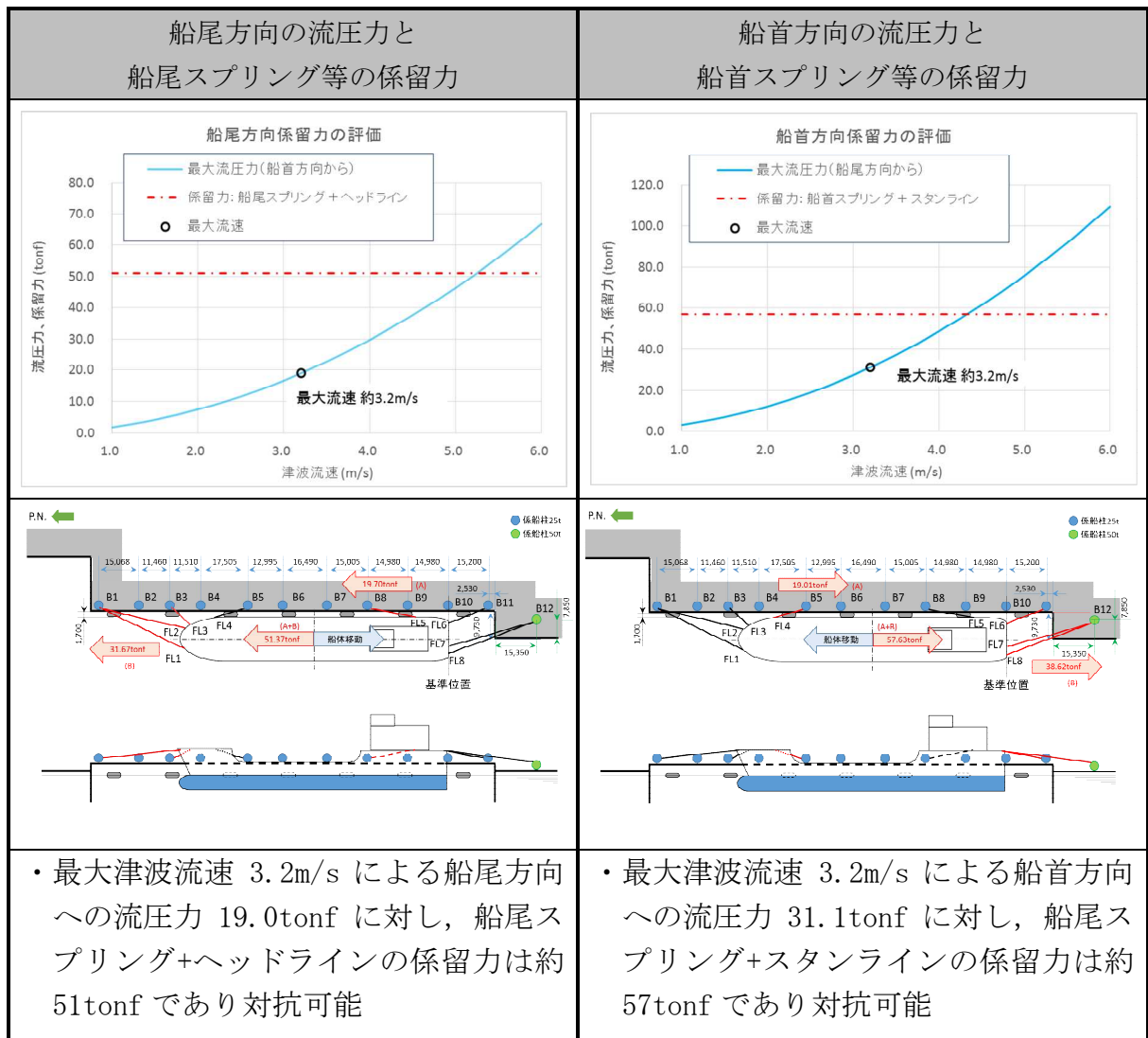
添付第 21-6 図 流圧力と係留力の比較
