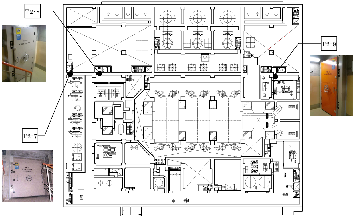
添付第 14-2-2 図 水密扉，浸水防止ダクト及び止水ハッチの設置位置並びに施工例（7号炉 タービン建屋地下中2階）
