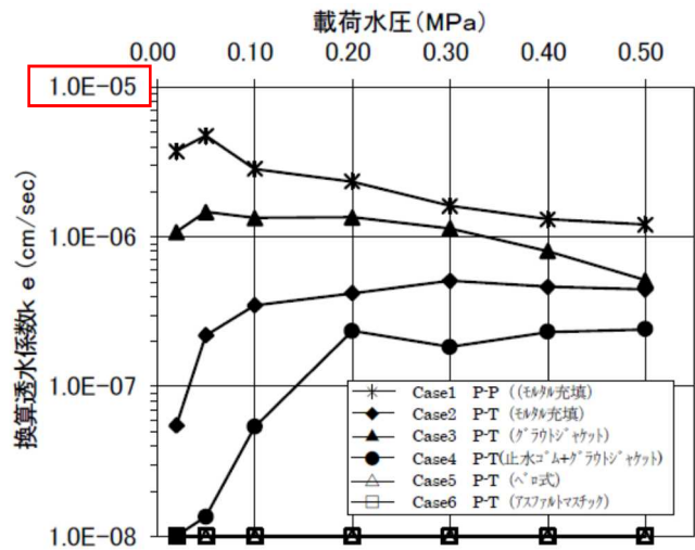
図- 11 継手遮水性能試験結果
