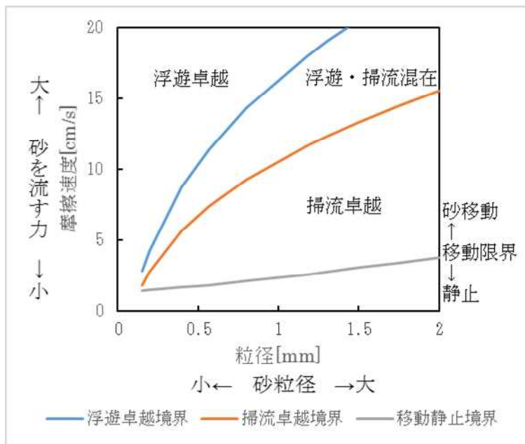
図 1 砂移動の形態
