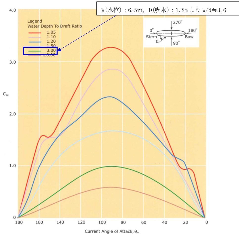
添付第 23-4 図 横方向流圧力係数 [C_{Yc}] 1)
