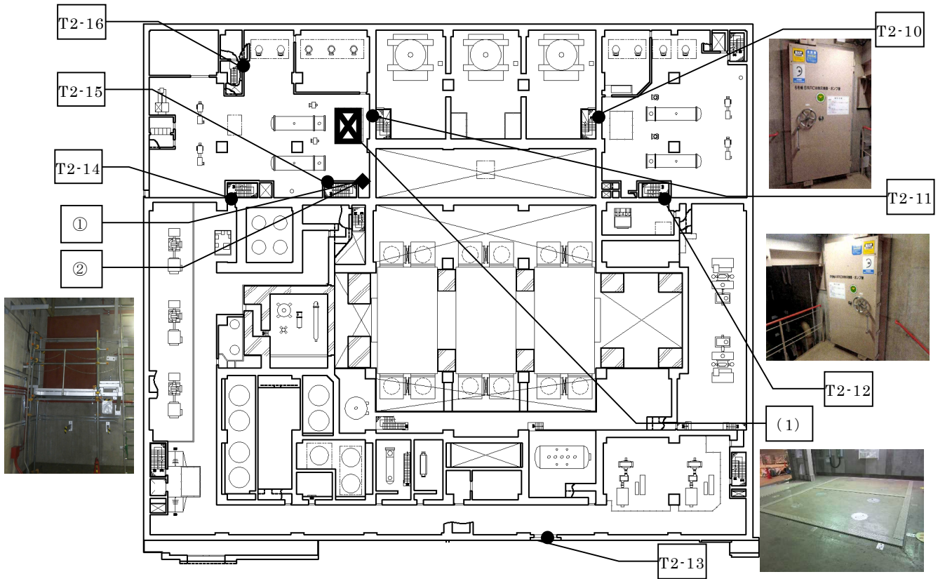
添付第 14-1-3 図 水密扉，ダクト閉止板及び止水ハッチの設置位置並びに施工例（6号炉 タービン建屋地下1階）
