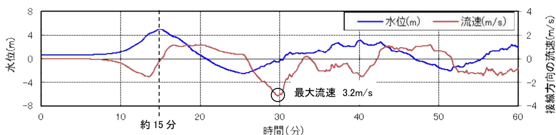
添付第21-3-1図 基準津波3の水位・流速（物揚場前面）
