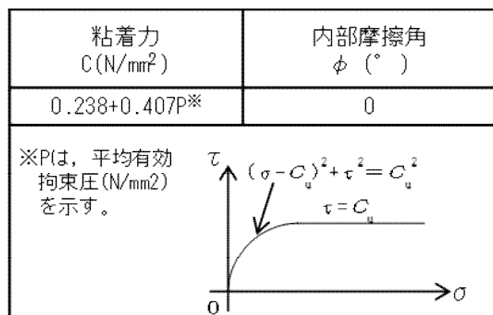
添付第 31-7 図 古安田層の強度特性
