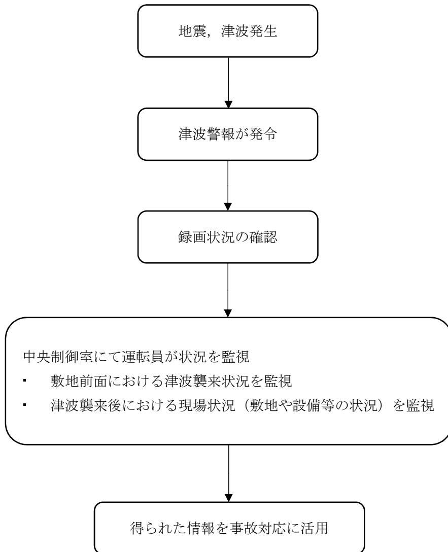
添付第 26-2 図 津波監視カメラ運用フロー
