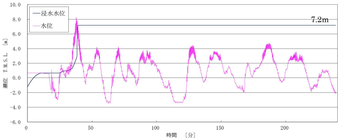
添付第13-2-5図 補機取水槽の水位及びタービン補機冷却水系熱交換器を設置するエリアの浸水水位の時刻歴波形（7号炉）
