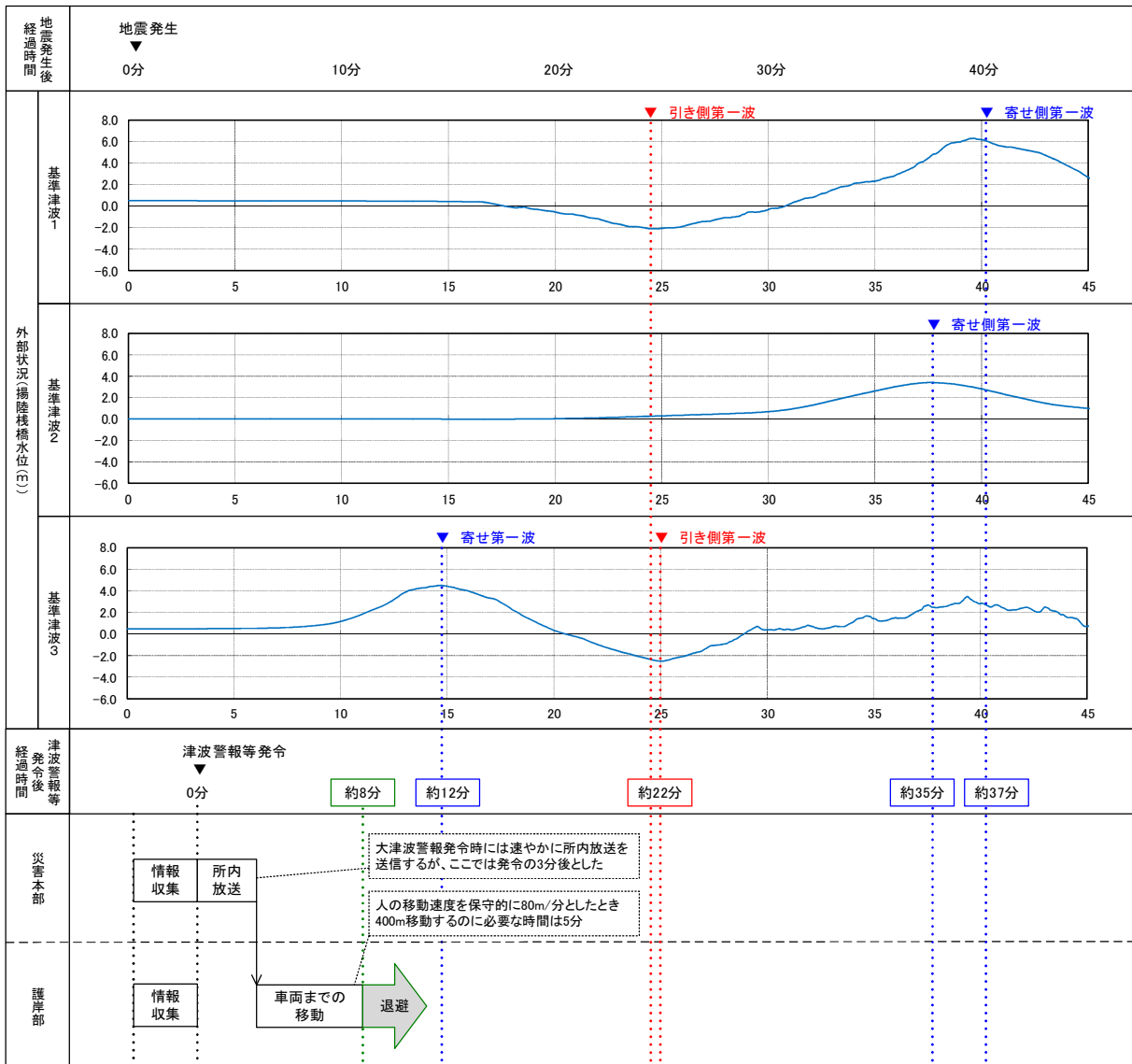
添付第 24-2 図 津波の到達と車両の退避に要する時間
