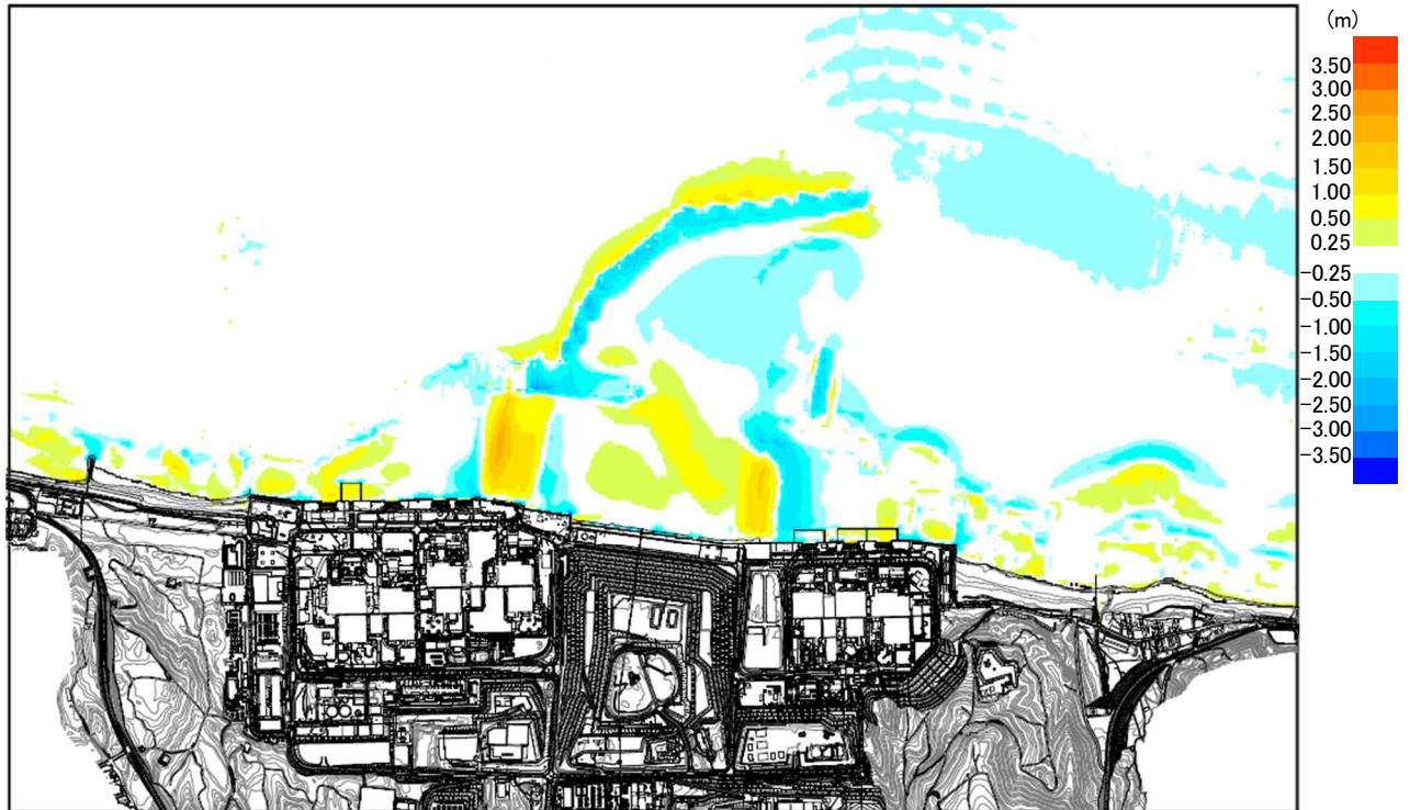
添付第 17-3 図 (2) 防波堤なし
