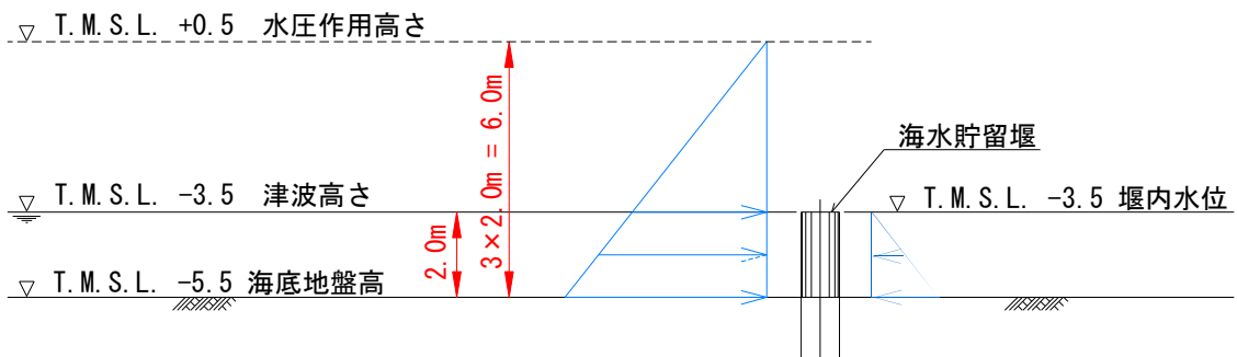
添付第 28-4 図 津波波力の作用イメージ （海水貯留堰天端高さ T.M.S.L. -3.5m の場合）
