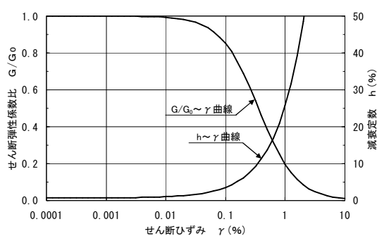
添付第 31-6 図 西山層のひずみ依存性
