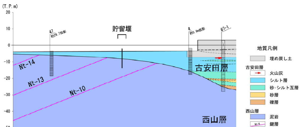
地質断面図（7号炉断面）
