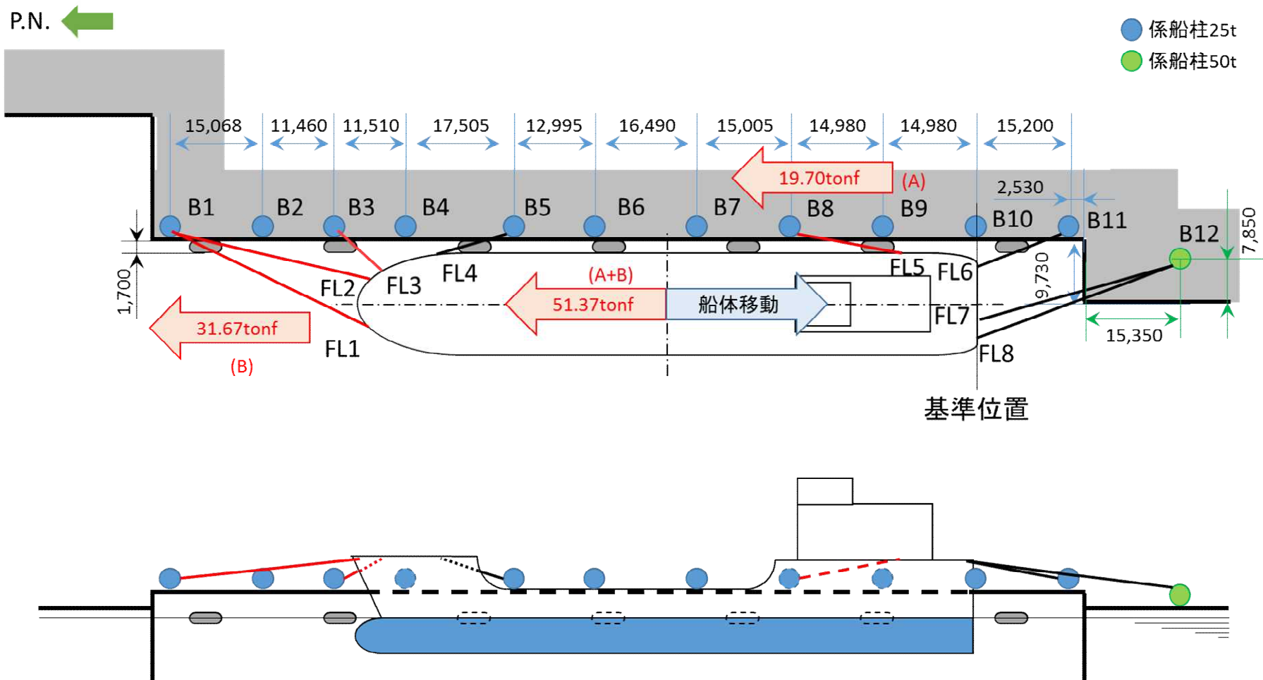
添付第 21-4 図 船尾方向への移動に対する船首方向係留力
