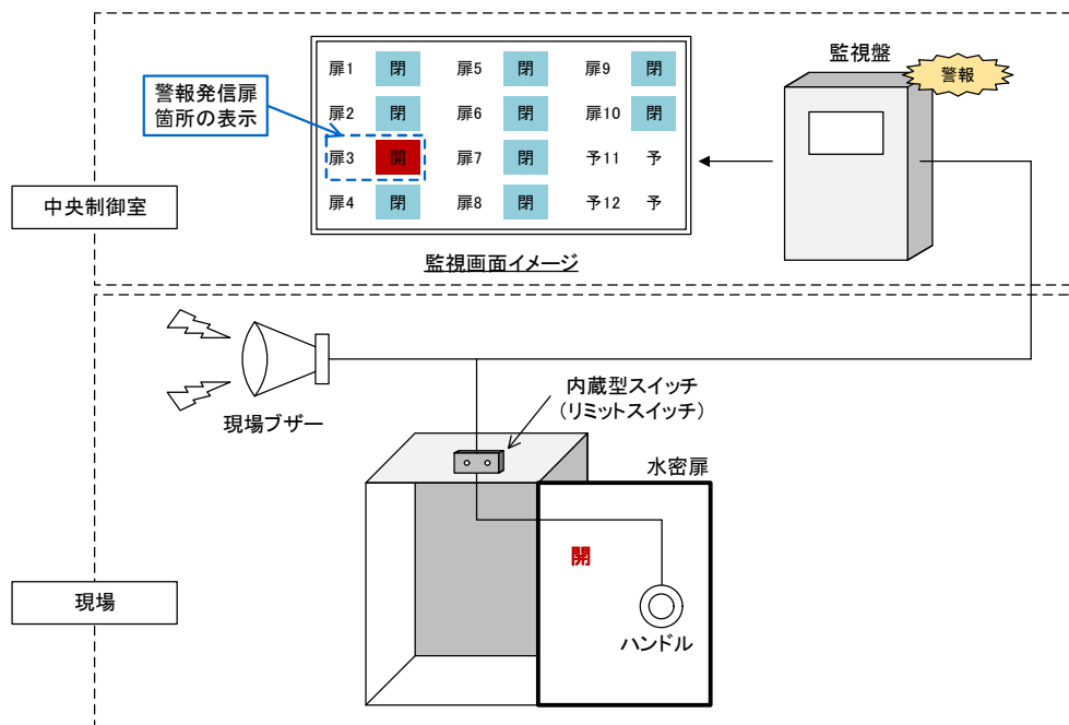
添付第 33-1 図 水密扉監視設備の概略図
