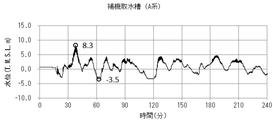
添付第 13-2-2 図 補機取水槽における入力津波波形 (7号炉) (補機取水槽 (A系))
