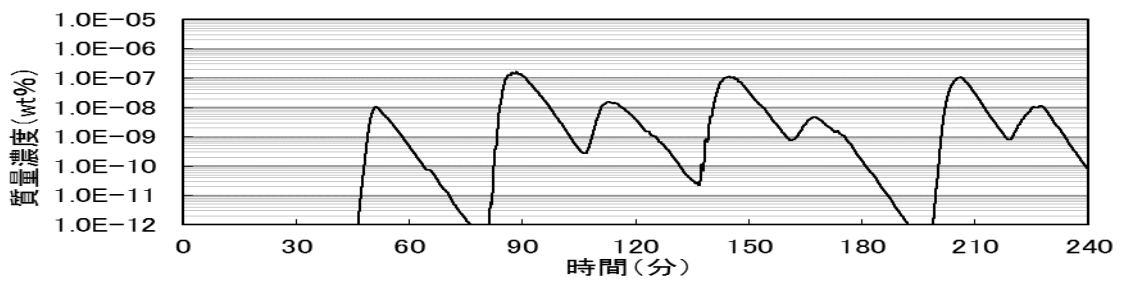
添付第 19-2 図 6号炉 基準津波 1 浮遊砂濃度時刻歴 (防波堤なし)
