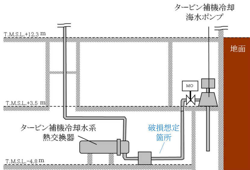
添付第 13-2-3 図 タービン補機冷却海水配管レイアウトイメージ (6号及び7号炉)
