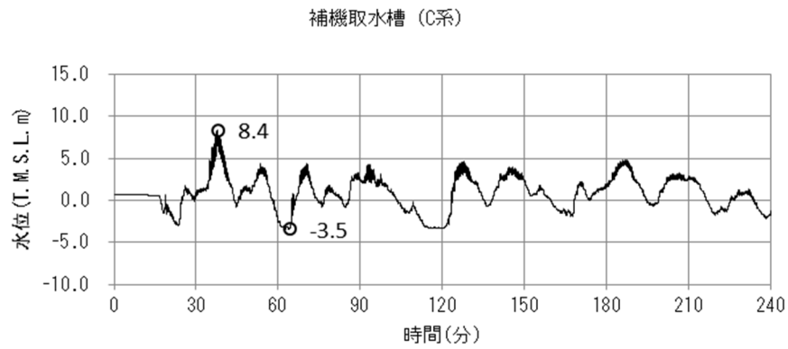
添付第 13-2-1 図 補機取水槽における入力津波波形 (6号炉) (補機取水槽 (C系))
