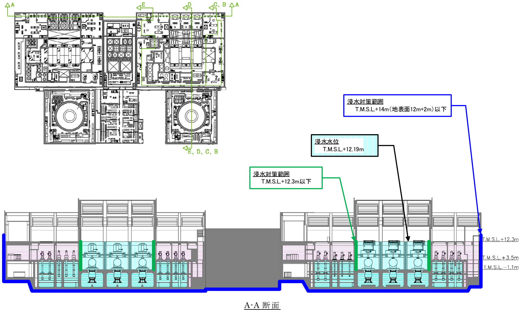
添付第 14-4 図 貫通部止水処置及び床ドレンライン浸水防止治具の実施範囲 (6号炉縦断面) (1/2)
