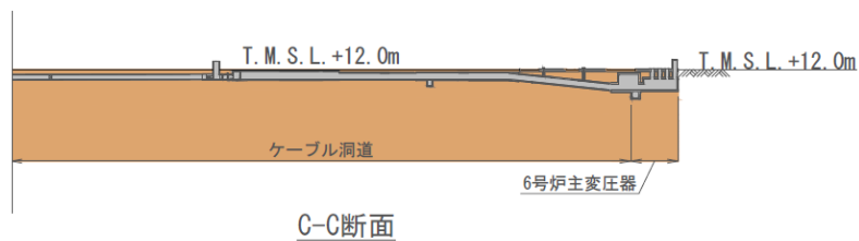
添付第 2-8 図 外部電源に係るケーブルを敷設する範囲のケーブル洞道断面図
