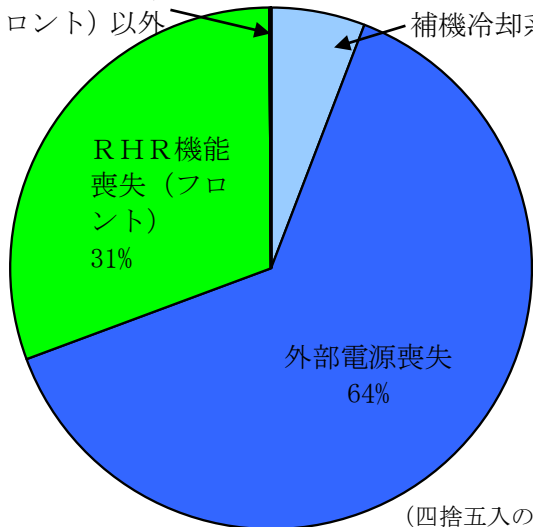
第 1. 1. 2. h-8 図 起因事象別の燃料損傷頻度の割合 (感度解析)
