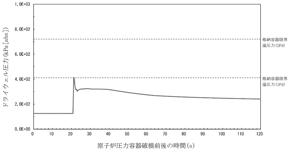
第1図 ドライウエル圧力
