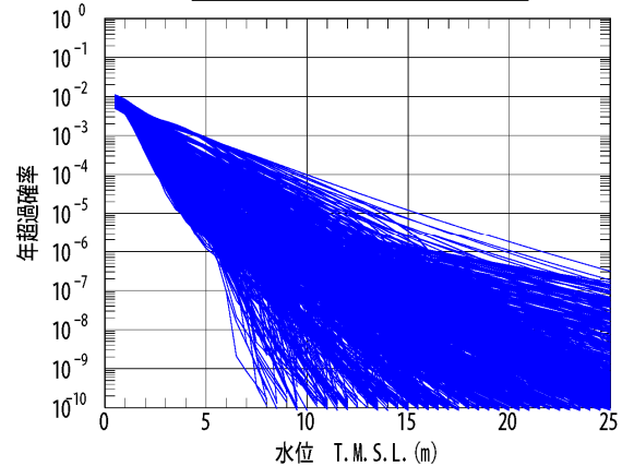
2000本のハザード曲線 (大湊側遡上域)
