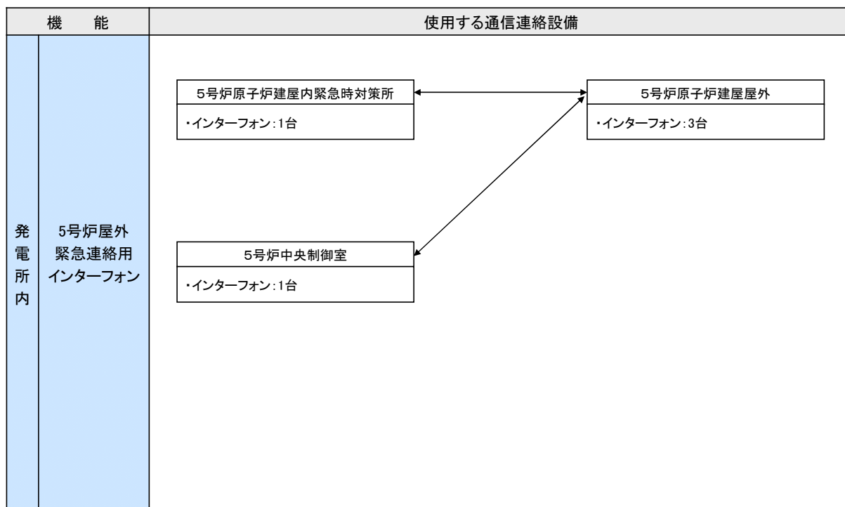
図62-6-4 機能ごとに必要な通信連絡設備（発電所内）（4 / 4）
