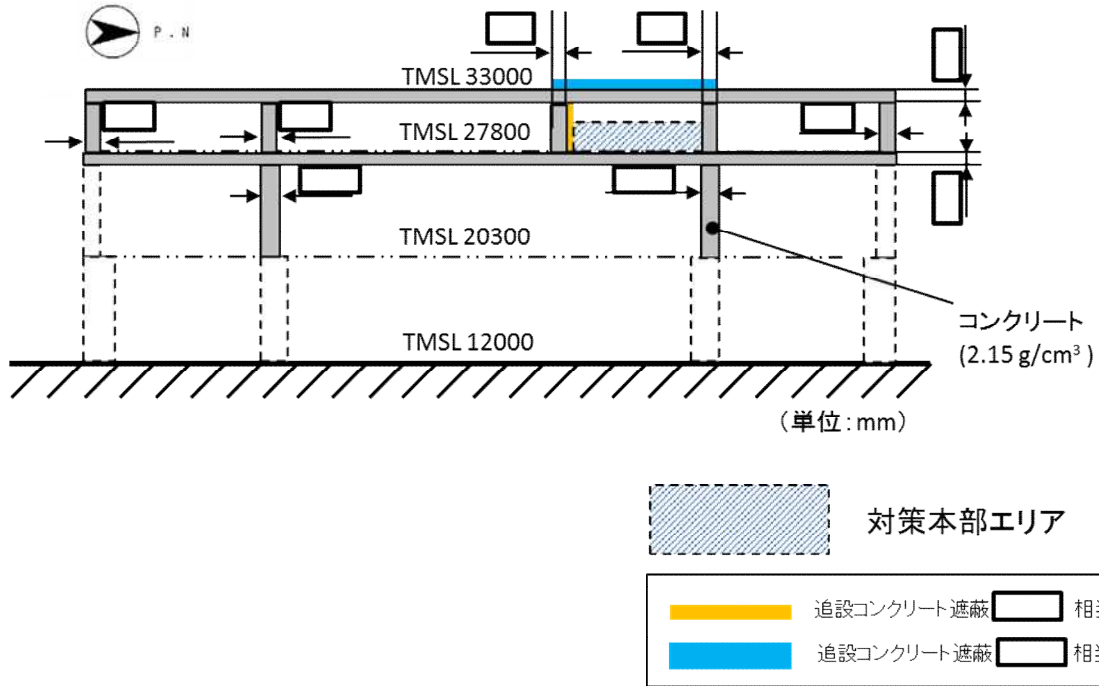
図 61-3-9 5号炉原子炉建屋内緊急時対策所（対策本部）遮蔽 断面図（NS 方向）
