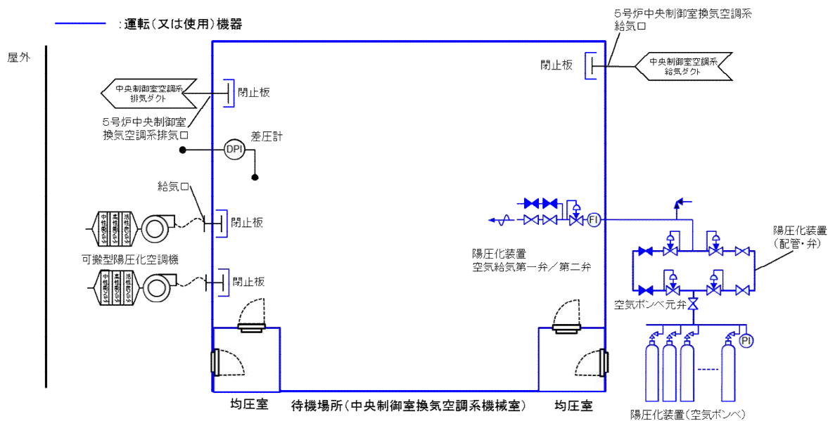
図 61-5-9 5号炉原子炉建屋内緊急時対策所（待機場所）換気設備 陽圧化装置（空気ボンベ）による陽圧化時の気密性，陽圧化機能に関する 試験・検査性 概略図
