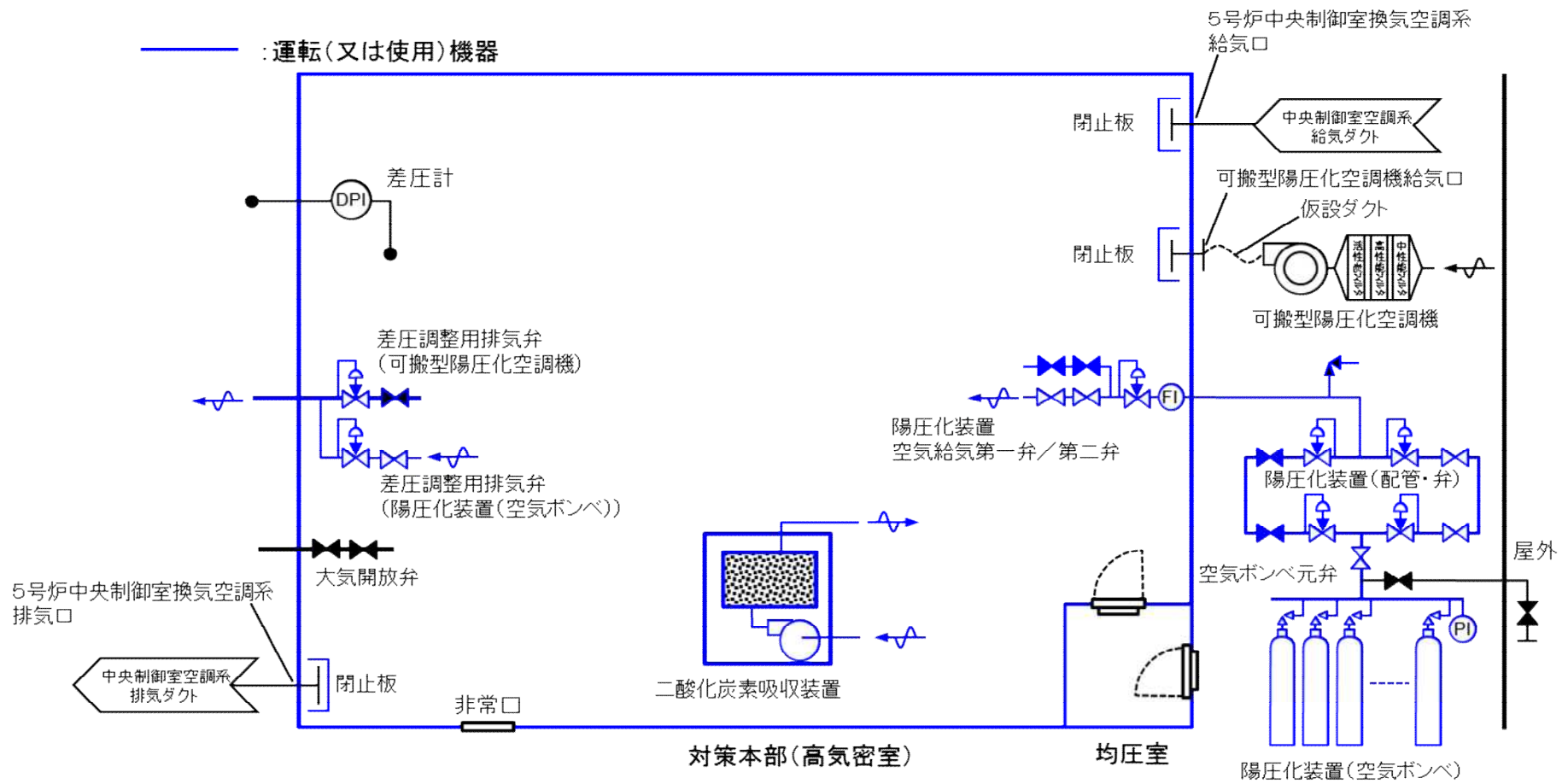
図 61-4-2 5号炉原子炉建屋内緊急時対策所(対策本部)換気設備 系統概略図 (プルーム通過中:陽圧化装置(空気ポンプ)による陽圧化)
