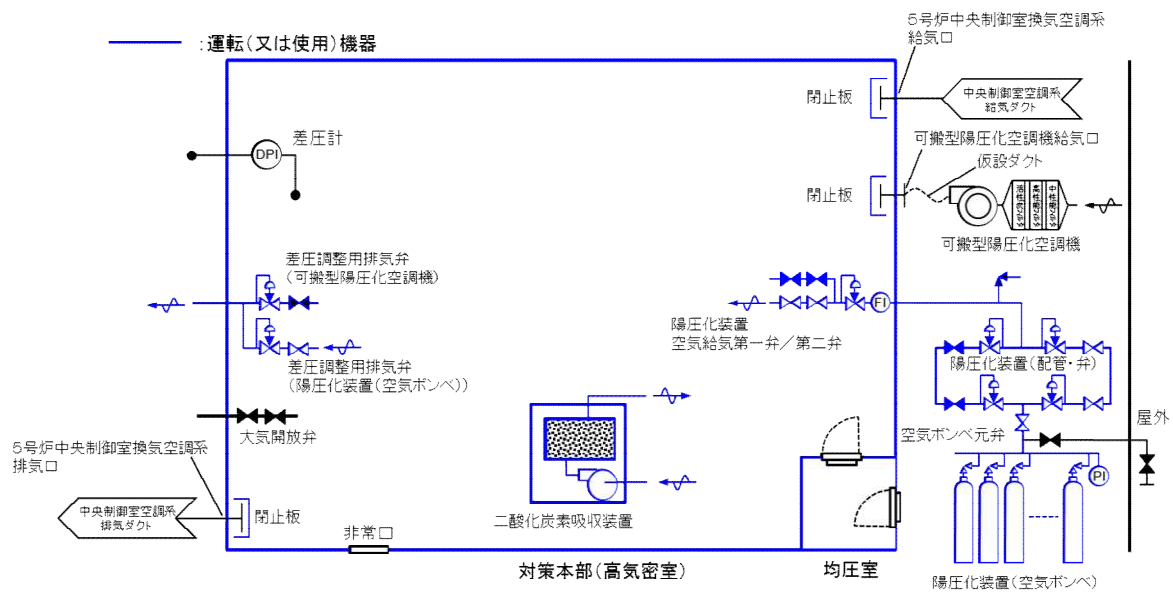
図 61-5-7 5号炉原子炉建屋内緊急時対策所(対策本部)換気設備 陽圧化装置(空気ポンペ)による陽圧化時の気密性, 陽圧化機能に関する 試験・検査性 概略図
