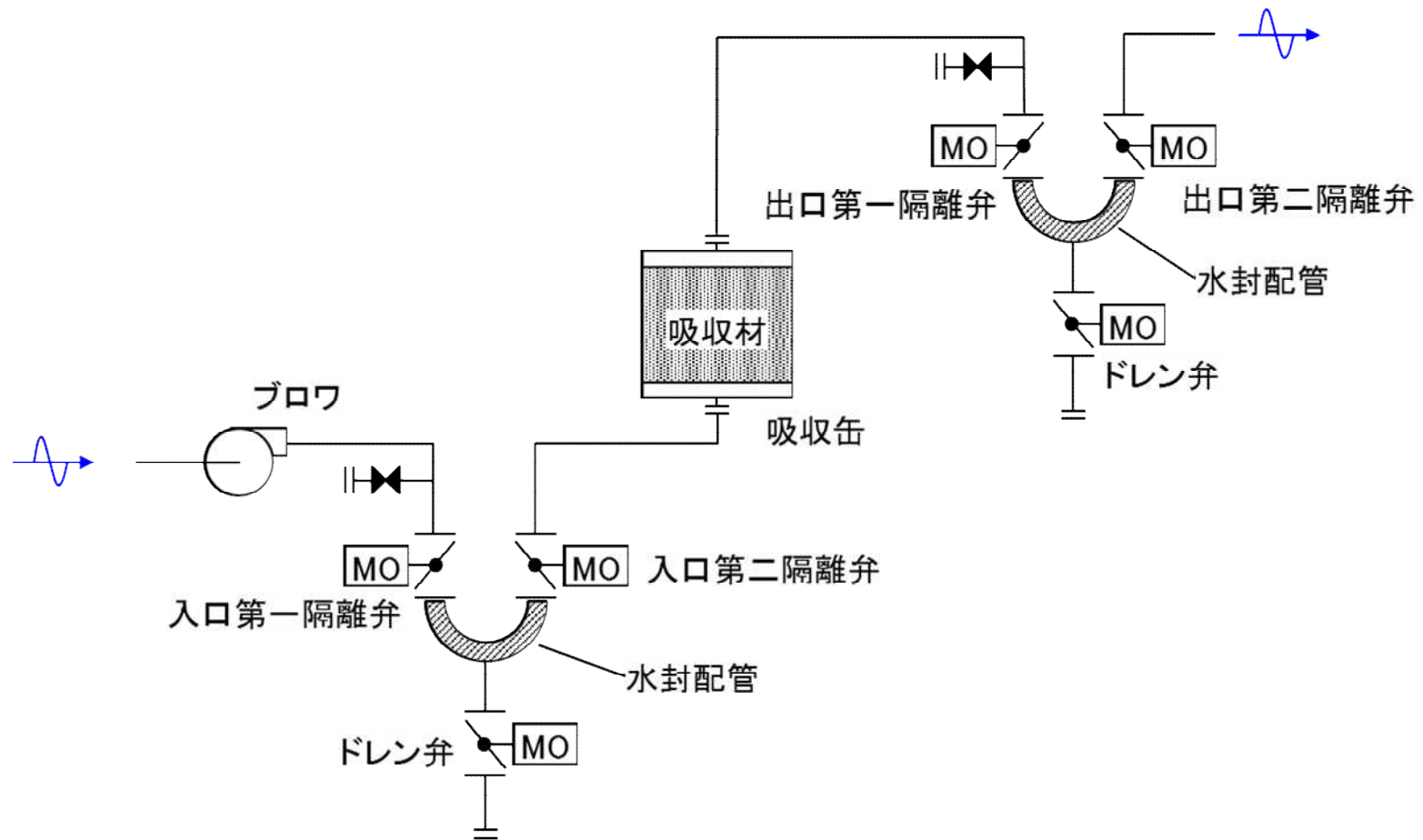
図 61-4-5 5号炉原子炉建屋内緊急時対策所（対策本部）二酸化炭素吸収装置 系統概略図
