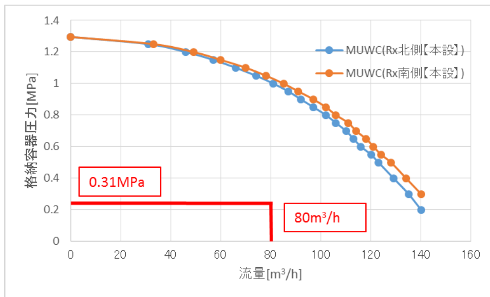
図2 代替格納容器スプレィ注水特性（低圧代替注水 40m 3 /h 同時注水時）
