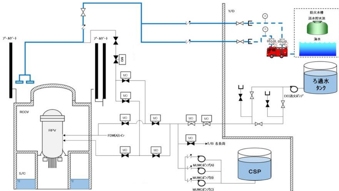
図1 格納容器頂部注水系 概要図
