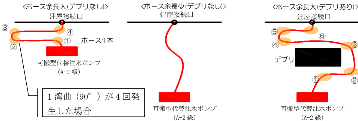
図 15 想定される消防ホースの引き回しパターン (イメージ)
