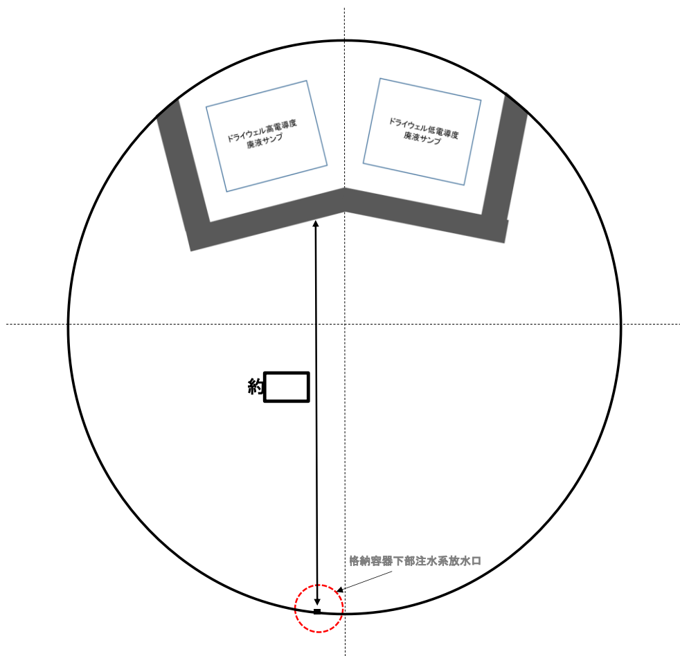
図2 コリウムシールドと原子炉格納容器下部注水設備放水口との設置位置概要図
