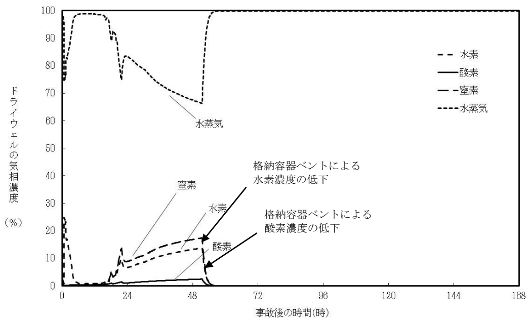
図 52-6-3 原子炉格納容器（ドライウエル）気相濃度 （大 LOCA+SB0+全 ECCS 機能喪失，代替循環冷却系使用）
