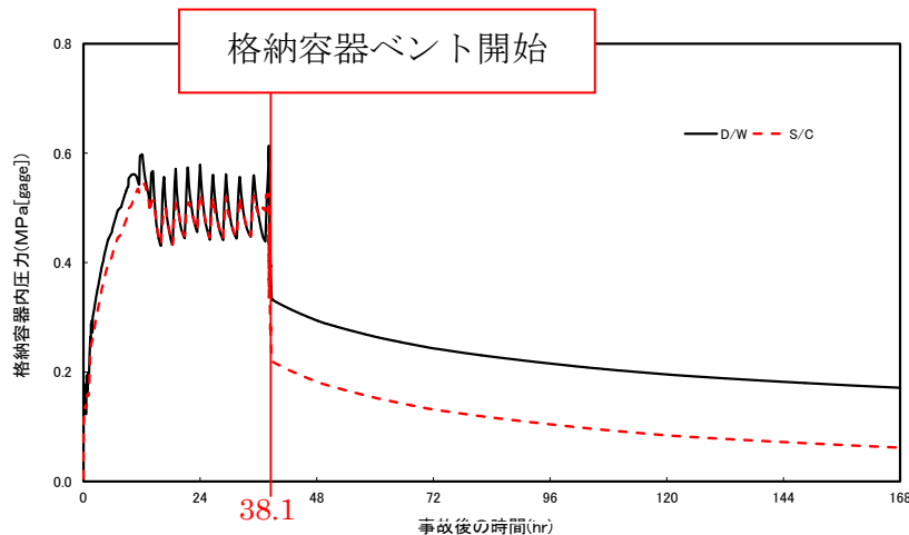
図 50-7-5 原子炉格納容器圧力推移 (大 LOCA+SB0+全 ECCS 機能喪失)
