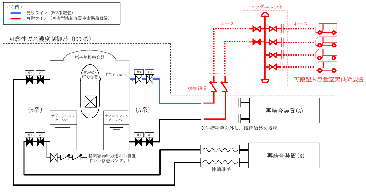
図 52-12-1 可搬型格納容器窒素供給設備 系統概要図
