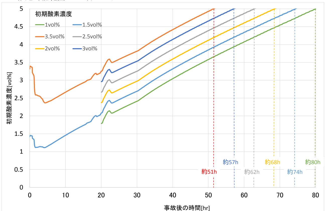
図 52-8-5 格納容器過圧・過温破損 (代替循環冷却系を使用する場合) の格納容器内酸素濃度変化
