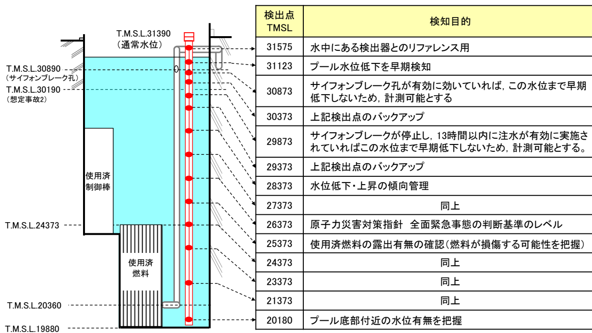
図4 使用済燃料貯蔵プール水位 (SA 広域) の水位設定点 (7号炉)
