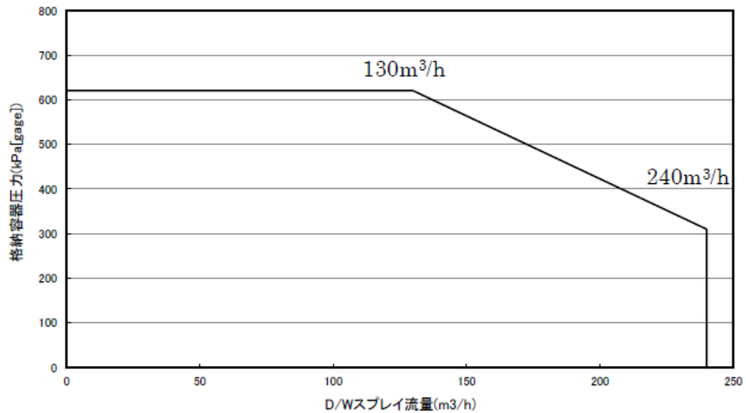
図4 ドライウェルスプレイ注水特性 (ペDESTAL 50m³/h 同時注水時)
