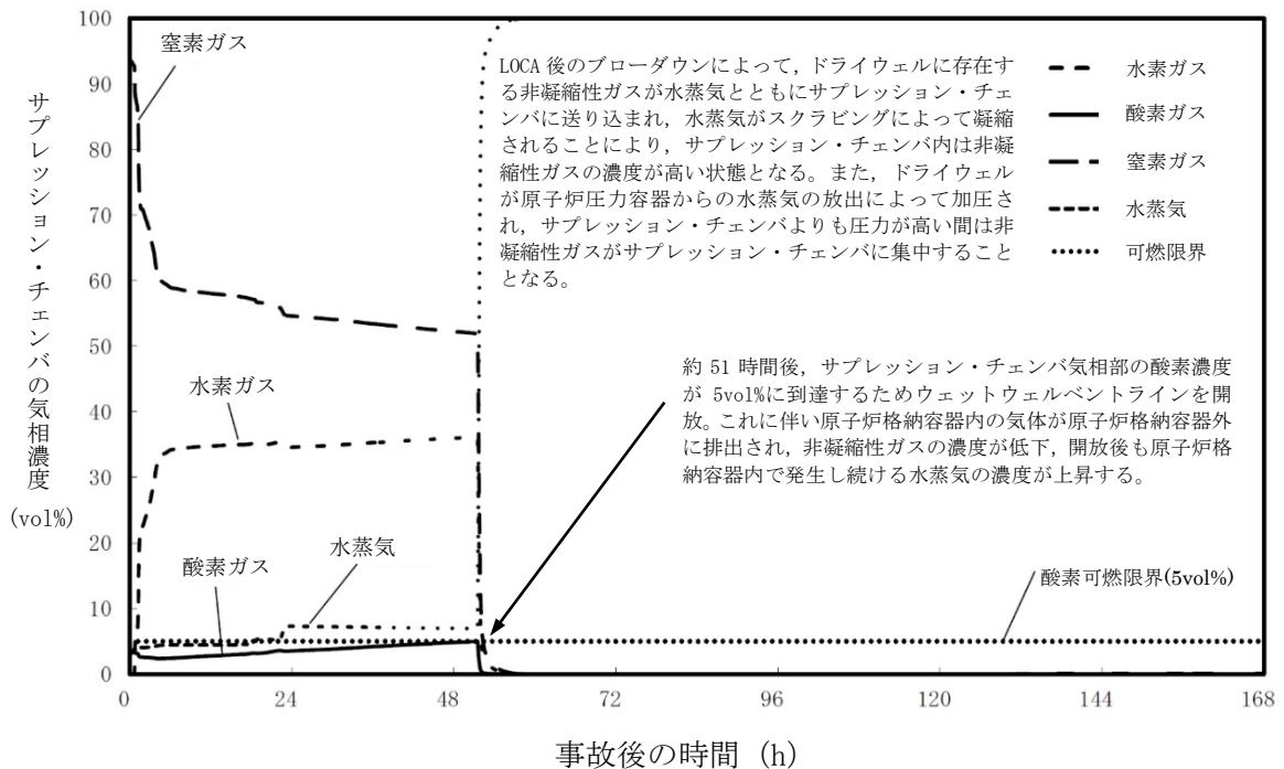
図 52-8-4 G 値を設計基準事故ベースとした場合のサブプレッション・チェンバの気相濃度の推移 (ウェット条件)
