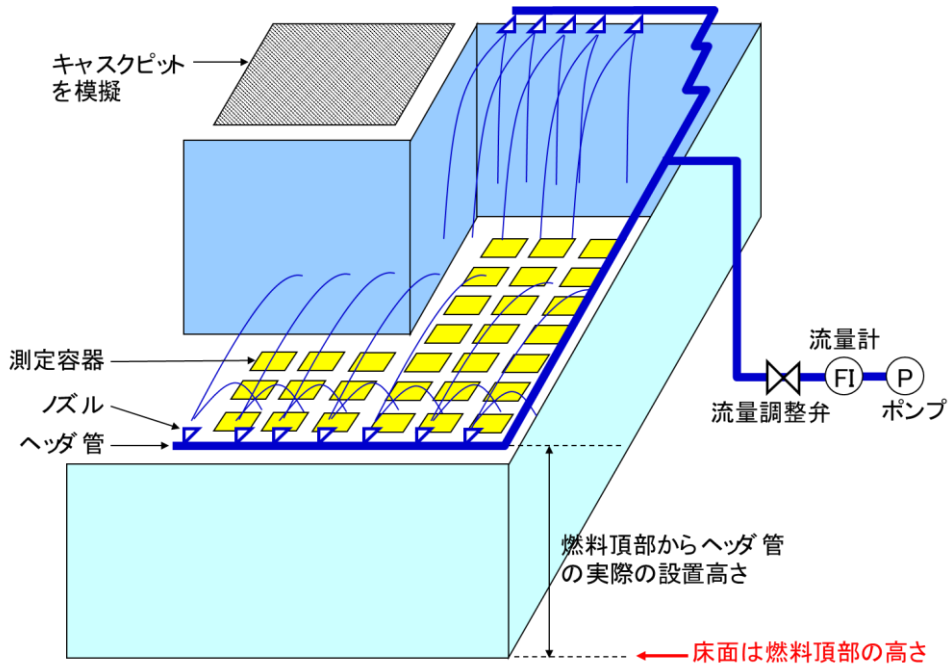
図 11 試験設備概要図
