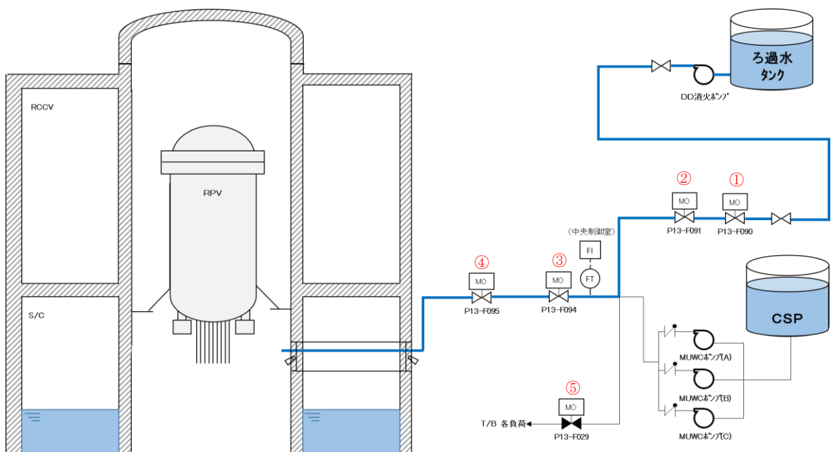
図1 消火系による原子炉格納容器下部への注水手順の概要図 (7号炉の例)
