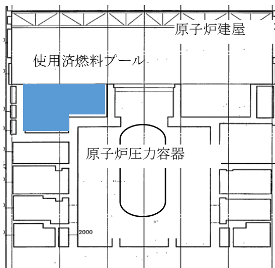
図1. 原子炉建屋内の使用済燃料プールの位置
