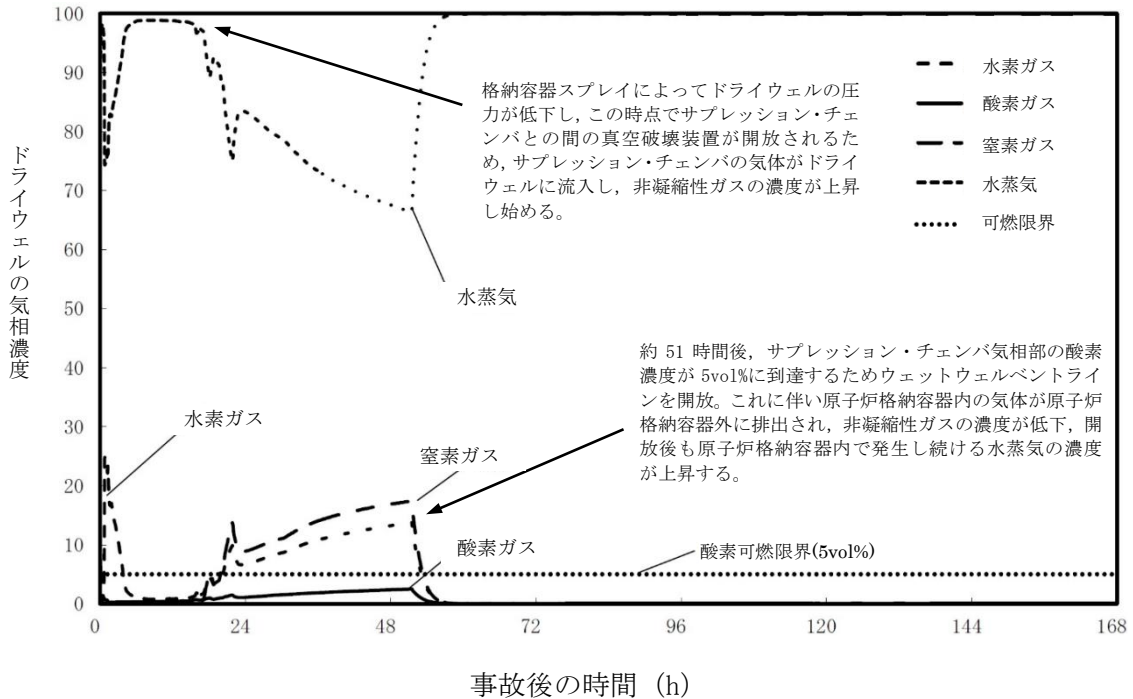
図 52-8-3 G 値を設計基準事故ベースとした場合のドライウエルの気相濃度の推移 (ウェット条件)
