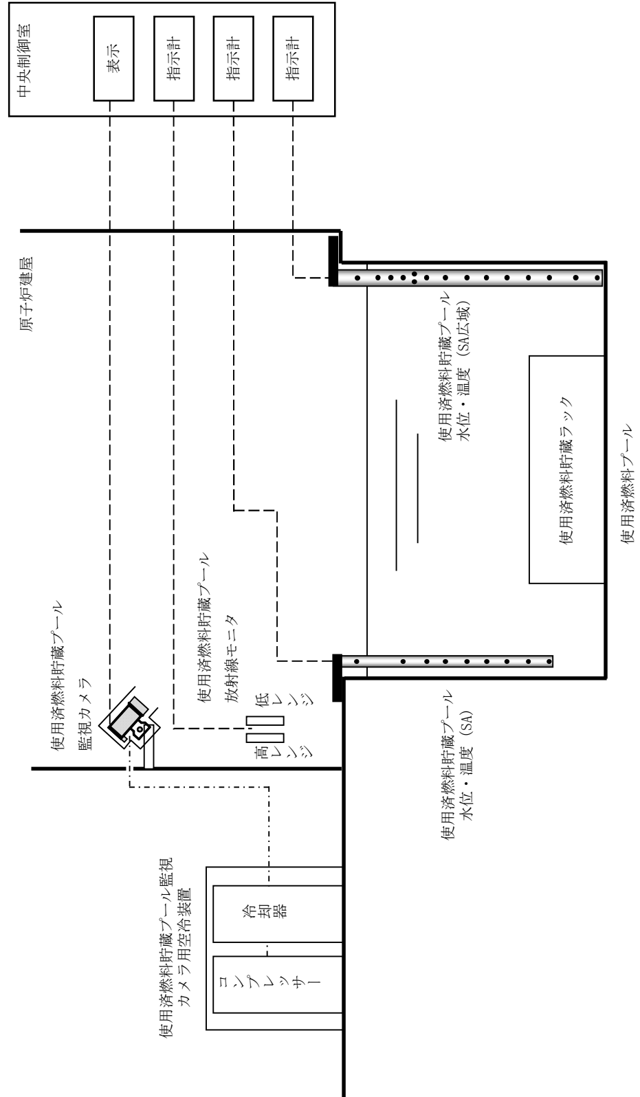
図 7 6号炉 使用済燃料プール監視設備の系統概要図
