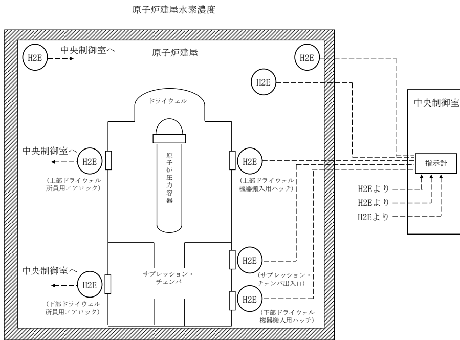
図 2 原子炉建屋水素濃度の系統概要図
