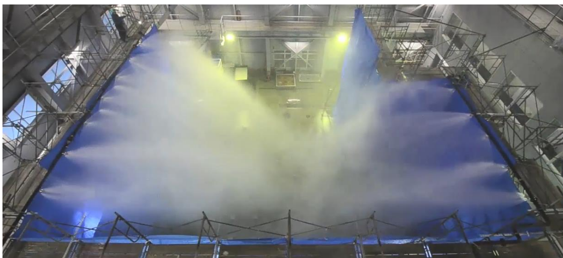
図 13 スプレイ状態の試験状況（スプレイ量：132m 3 /h）
