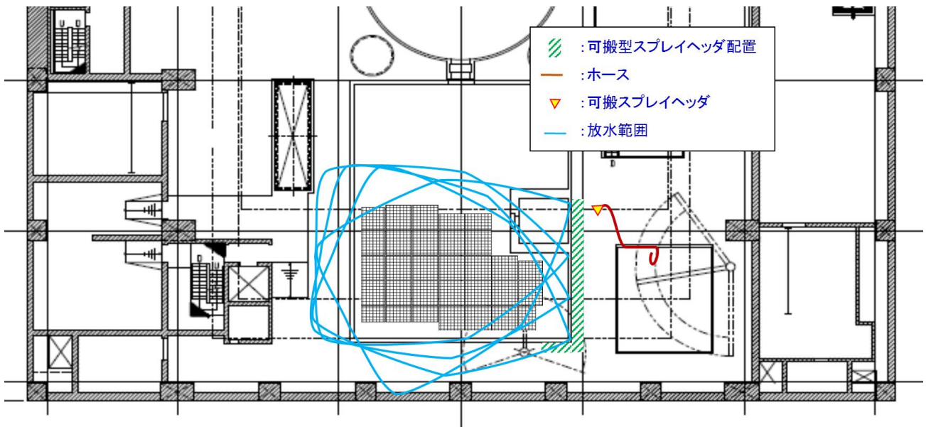
図10 可搬型スプレィヘッドのスプレィ範囲（北面からスプレィする場合）
