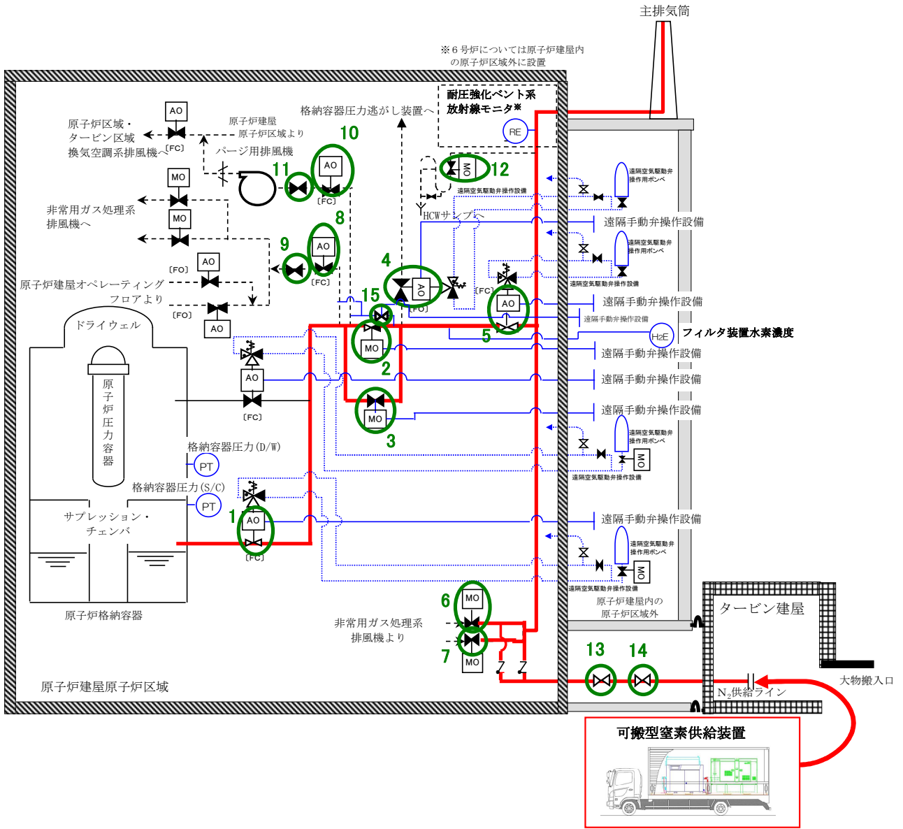
図 52-4-1 耐圧強化ベント系 系統概略図
