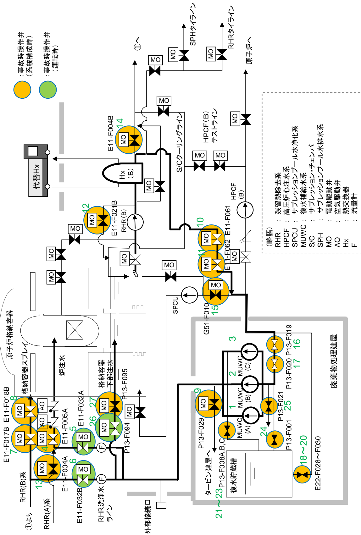
図 50-5-3 代替循環冷却系 系統概要図 (7号炉)
