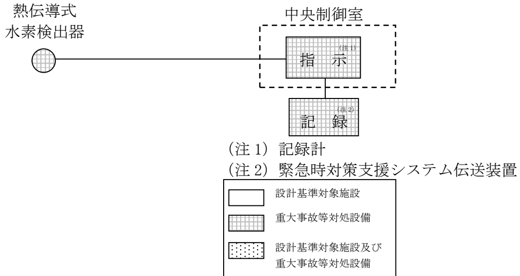
図 3 原子炉建屋水素濃度の概略構成図
