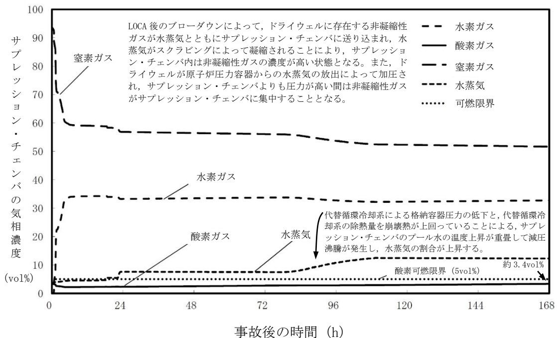
図 52-8-2 サブプレッション・チェンバの気相濃度の推移(ウェット条件) 格納容器過圧・過温破損（代替循環冷却系を使用する場合）
