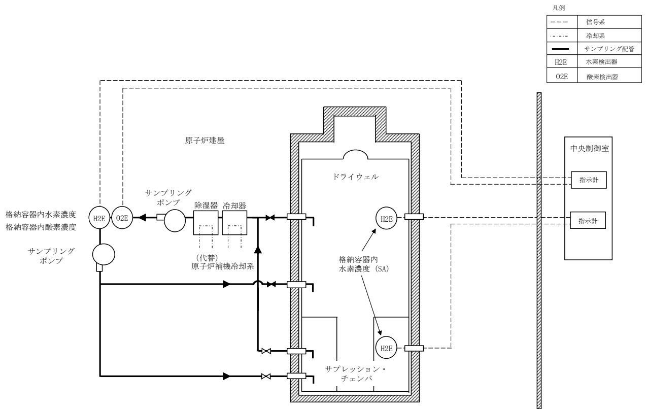
図 52-4-2 水素濃度監視設備及び酸素濃度監視設備に関する系統概要図
