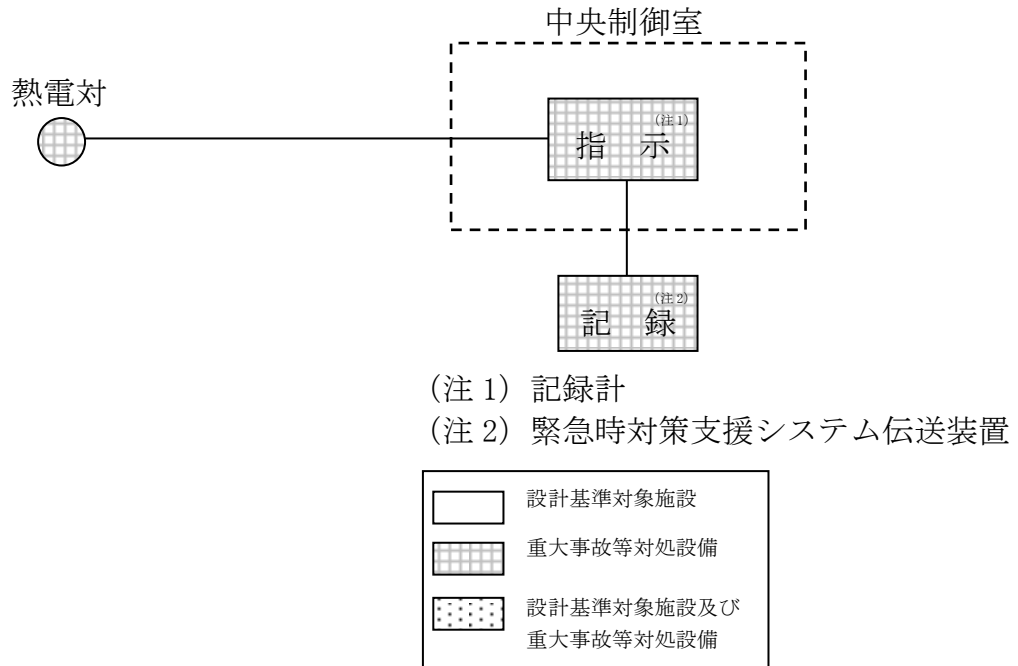
図6 使用済燃料貯蔵プール温度 (SA) の概略構成図
