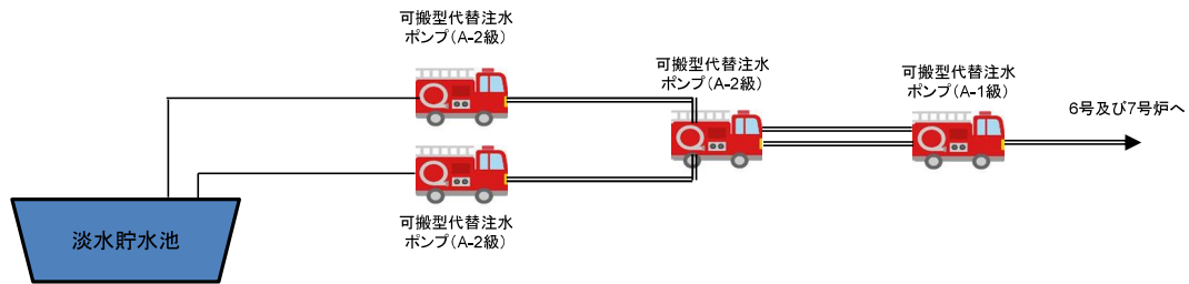
図2 燃料プール代替注水系（常設スプレイヘッド）によるスプレイ 系統概要図
