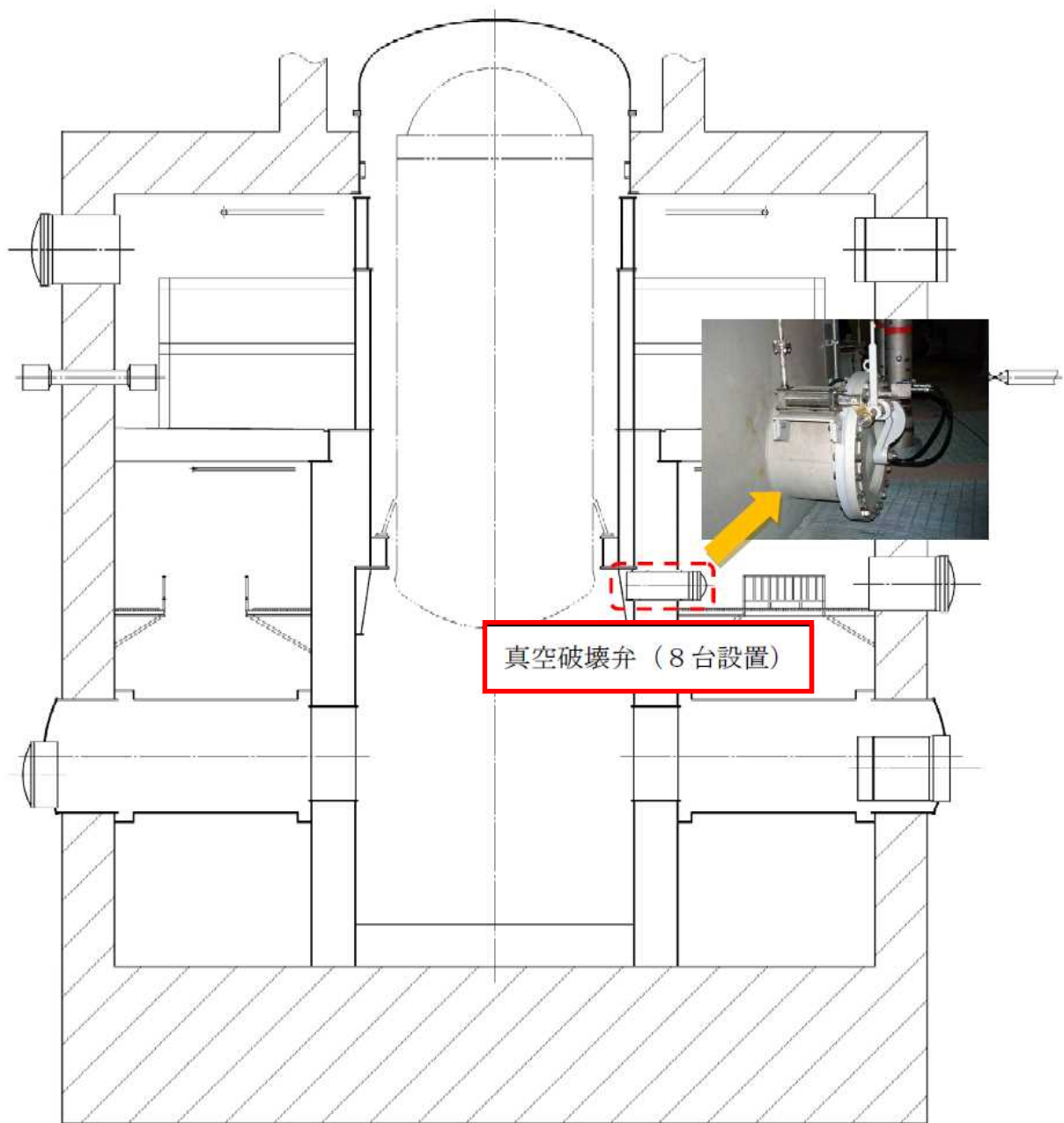
图 52-3-13 6/7 号炉 真空破壞弁 設置位置图
