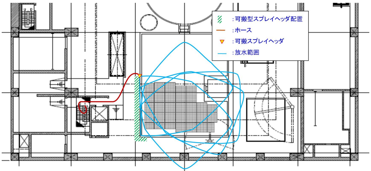
図9 可搬型スプレィヘッドのスプレィ範囲（南面からスプレィする場合）
