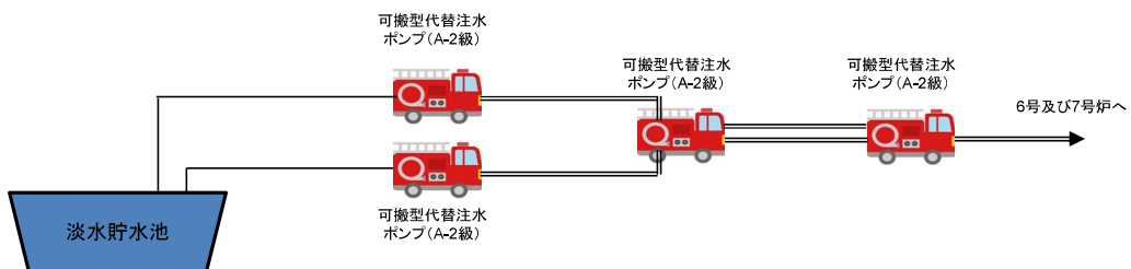
図1 燃料プール代替注水系 (可搬型スプレイヘッダ/常設スプレイヘッダ) による注水, 燃料プール代替注水系 (可搬型スプレイヘッダ) によるスプレイ 系統概要図
