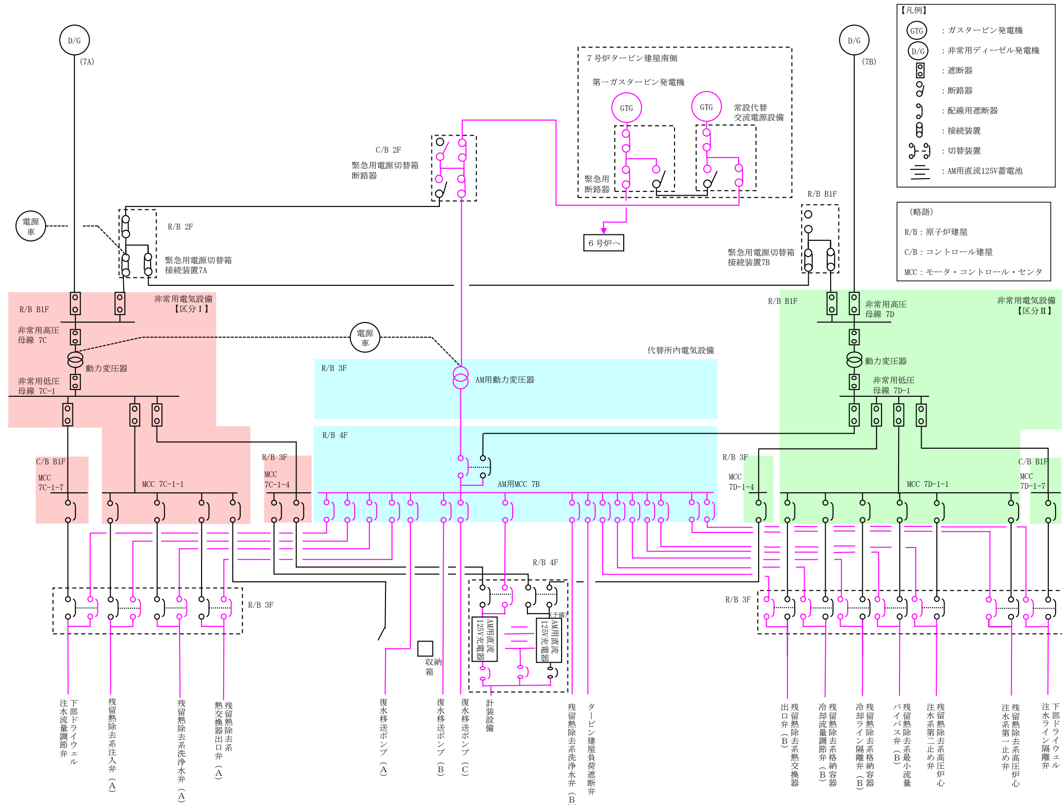
図 50-2-4 代替循環冷却系の単線結線図 (代替所内電気設備経由で電源供給時)
