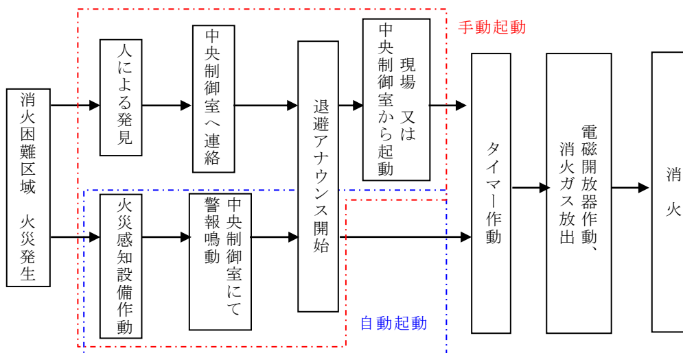
第5図：火災発生時の信号の流れ
