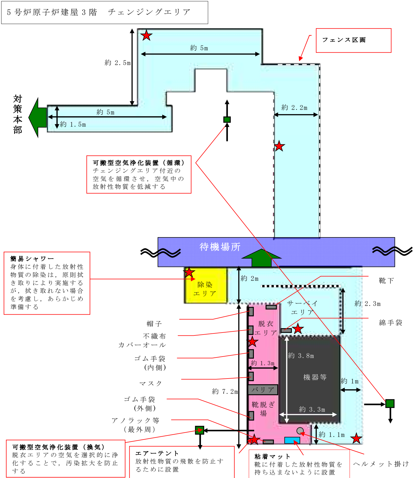
第 5 図 5号炉原子炉建屋内緊急時対策所チェンジングエリア (5号炉原子炉建屋北東側アクセスルート)
