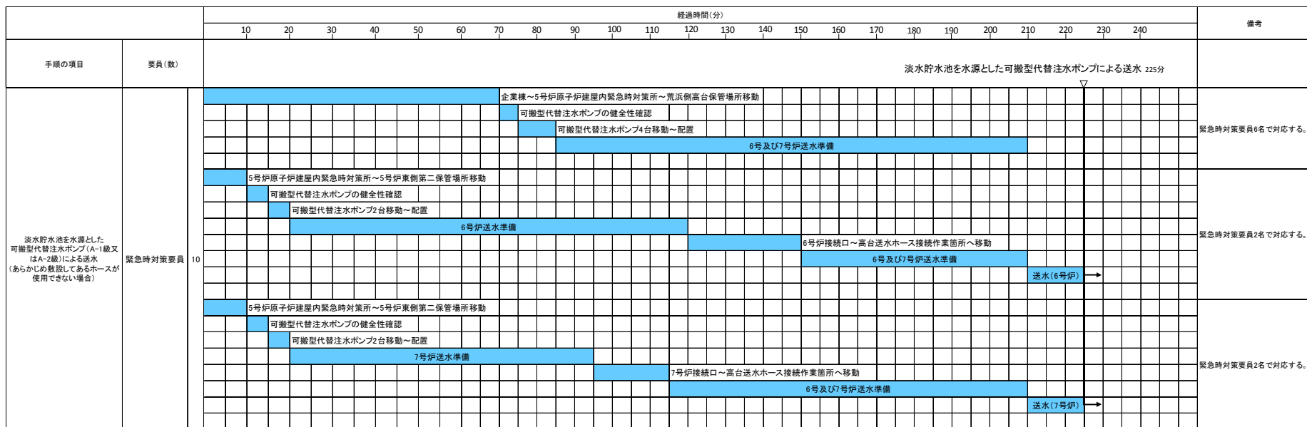
第 1.13.7 図 淡水貯水池を水源とした可搬型代替注水ポンプ(A-1級又はA-2級)による送水 タイムチャート(2/2) (あらかじめ敷設してあるホースが使用できない場合)
