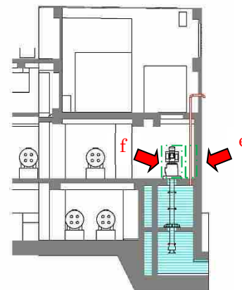
C-C 断面 (補機取水層)
