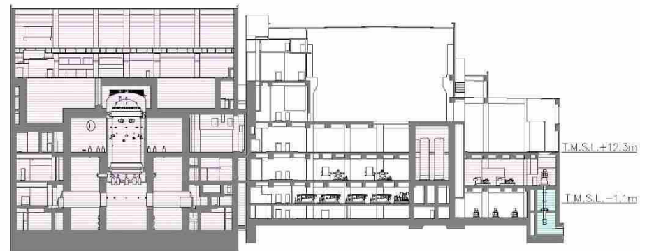
D-D 断面
