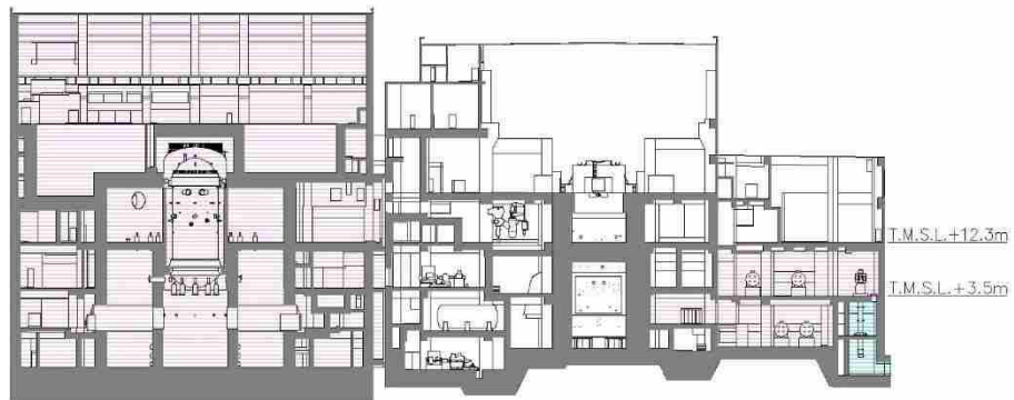
B-B 断面
