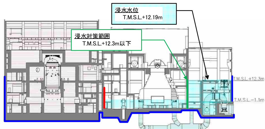
D-D 断面
