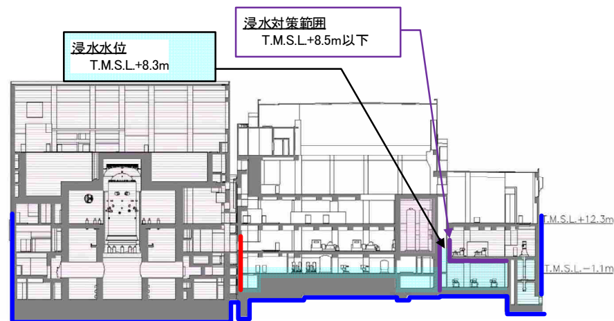
D-D 断面
