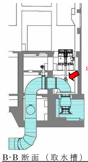
第 2.3-4-1 図 取水槽及び補機取水槽上部床面を介した漏水の可能性の検討 (6号炉の例)
