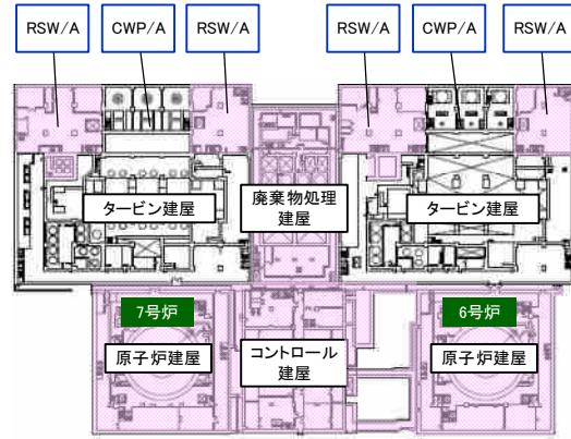
地下1階(タービン建屋地下1階) * タービン建屋床面高さT.M.S.L.+4.9m
