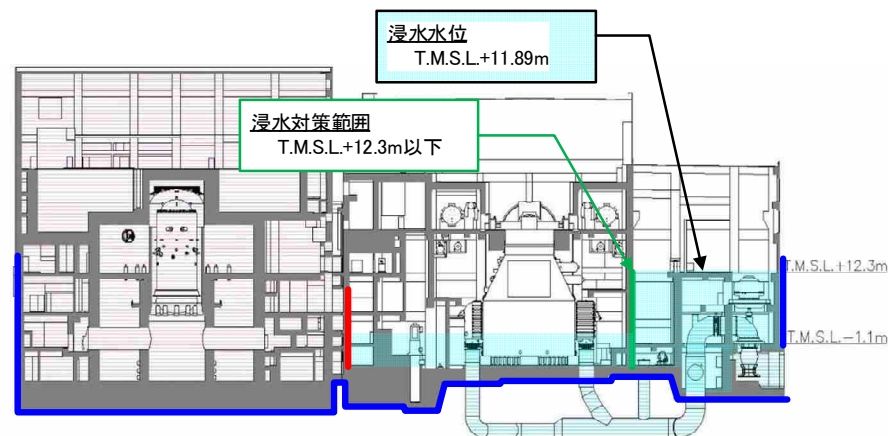
D-D 断面
