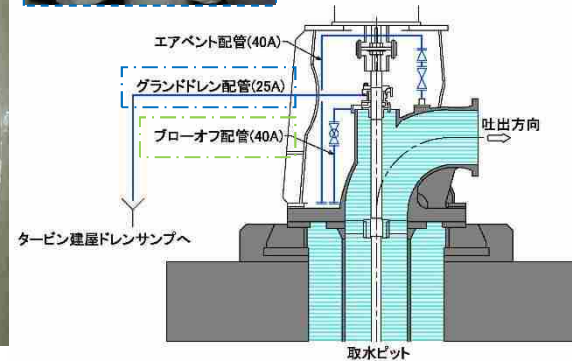
f 部 原子炉補機冷却海水ポンプ グランドドレン配管
