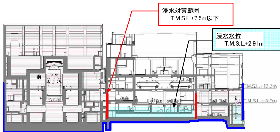
B-B 断面
