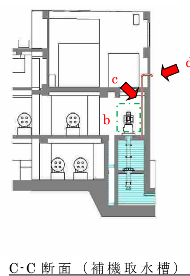
第 2.3-4-1 図 取水槽及び補機取水槽上部床面を介した漏水の可能性の検討 (6号炉の例)
