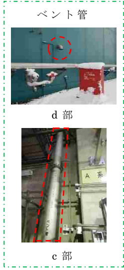
第 2.3-4-1 図 取水槽及び補機取水槽上部床面を介した漏水の可能性の検討 (6号炉の例)
