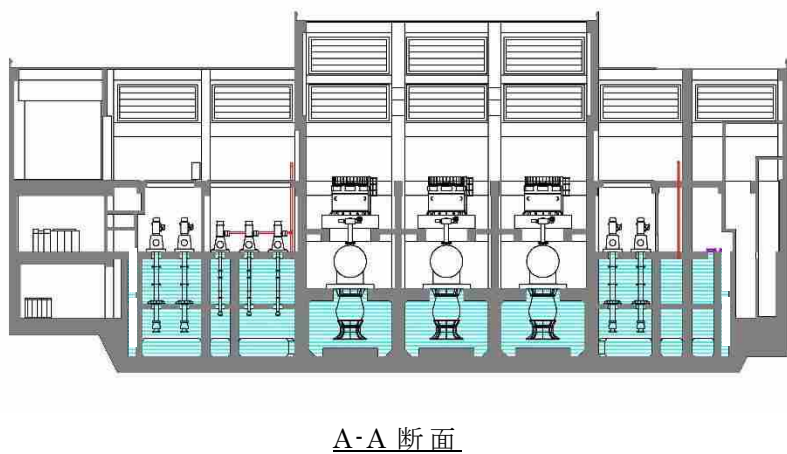
第 2.3-4-1 図 取水槽及び補機取水槽上部床面を介した漏水の可能性の検討 (6号炉の例)
