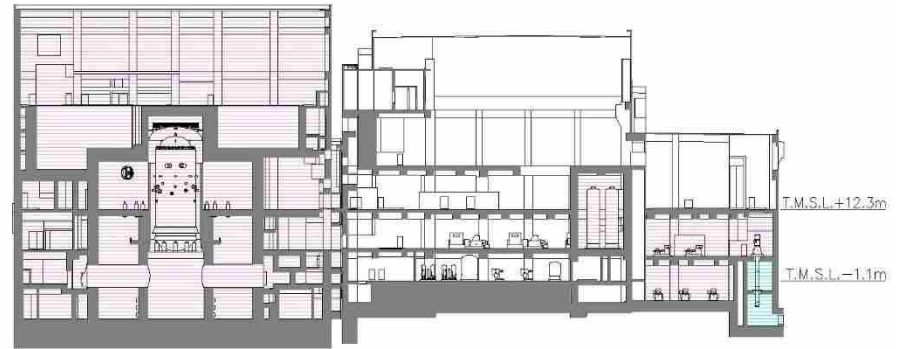
E-E 断面
