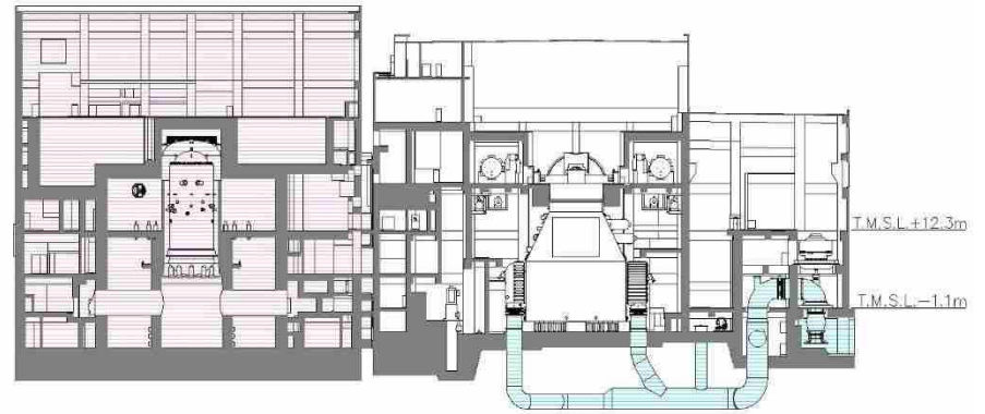
D-D 断面
