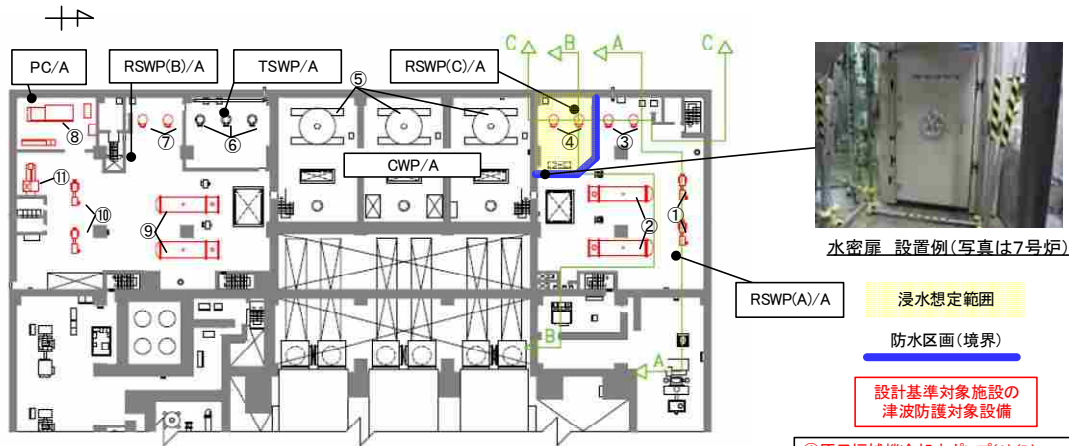
タービン建屋地下1階 平面図
