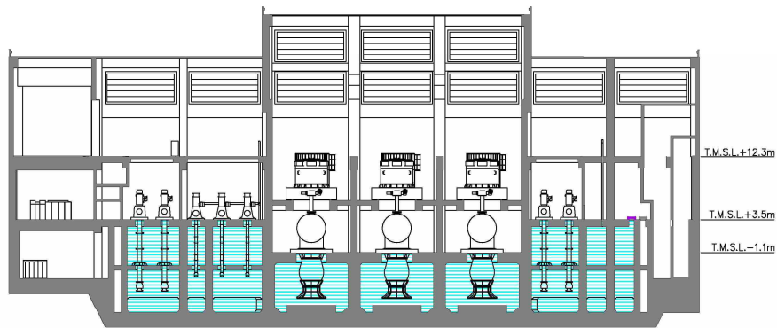
I-I 断面
