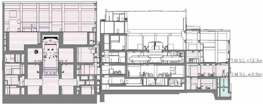
B-B 断面
