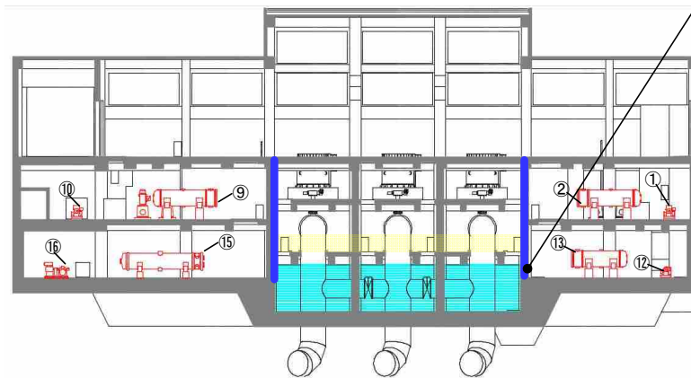
B-B断面
