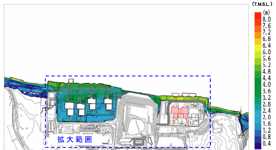
最大浸水深分布 (敷地全体)
