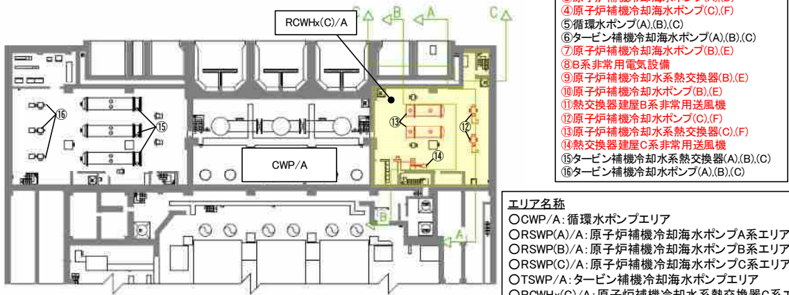
タービン建屋地下2階 平面図
