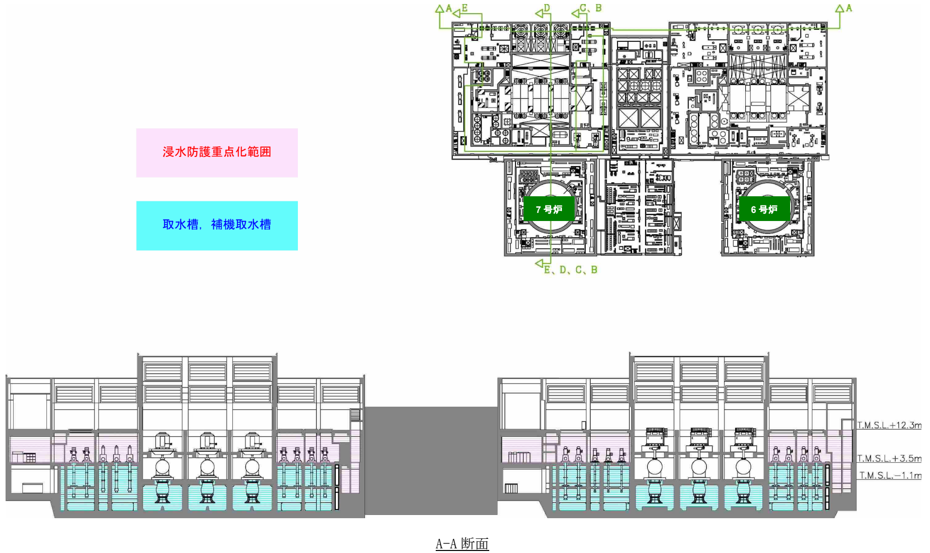
第 2.4-2-3 图 浸水防護重点化範圍詳細图 (7号炉縦断面) (1/2)
