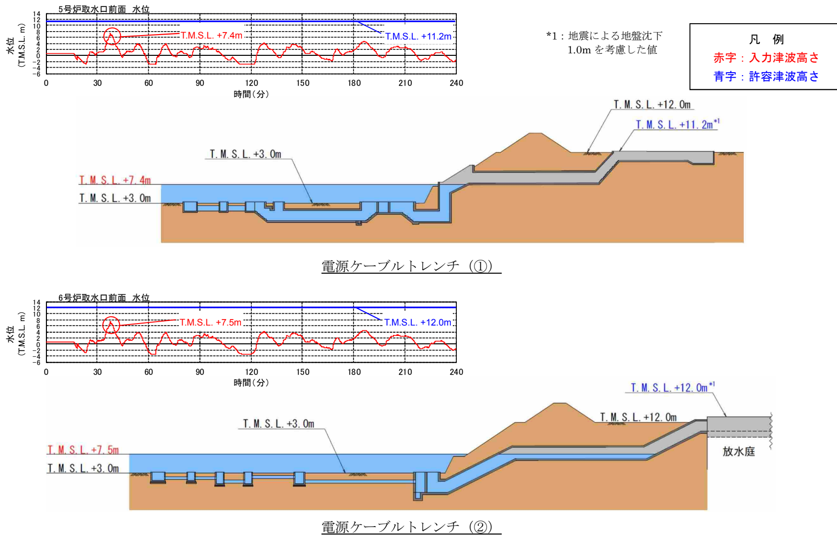
第 2.2-6-2 図 電源ケーブルトレンチ断面図
