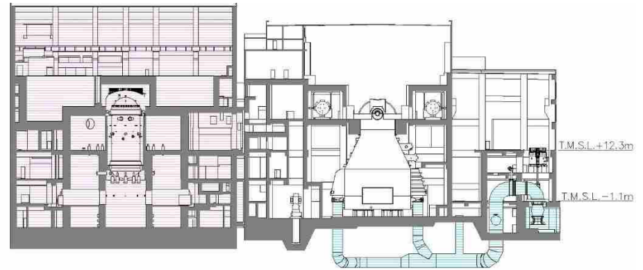
D-D 断面
