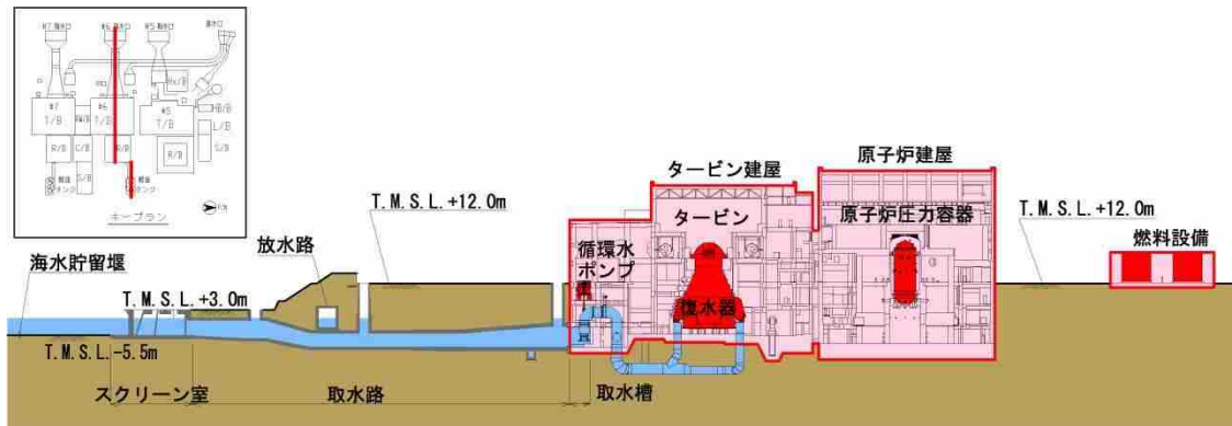
取水路断面
