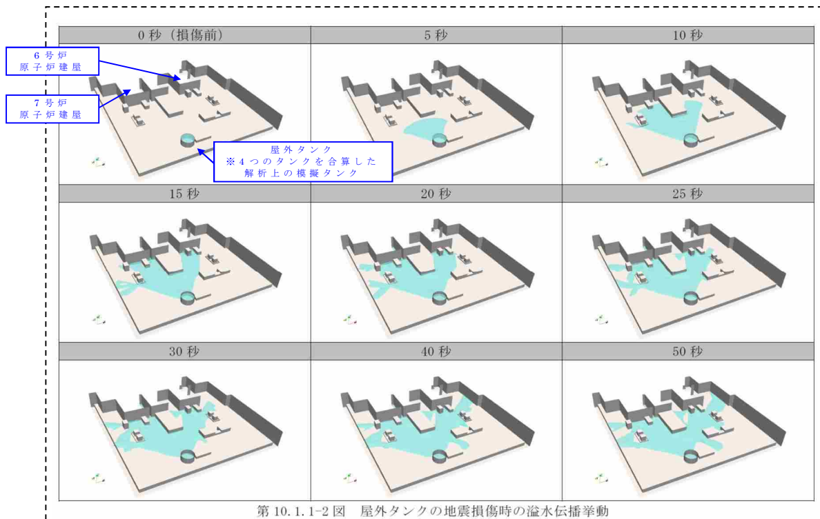
第 2.4-7 図 溢水伝播挙動のイメージ
