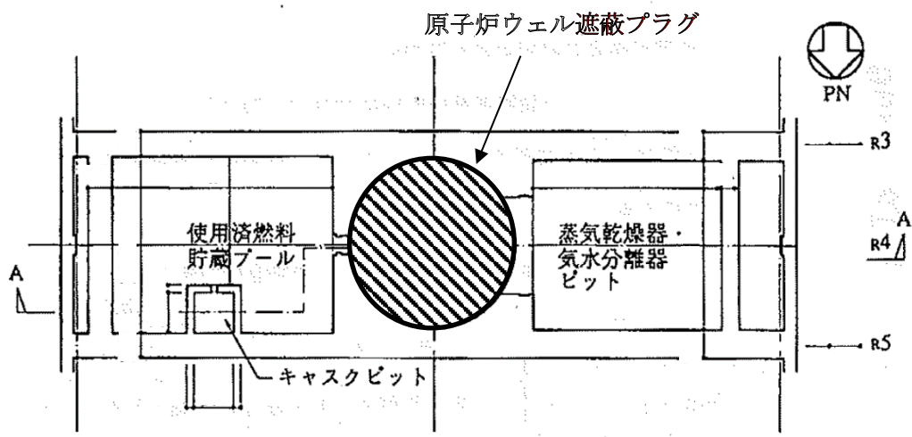
平面図
