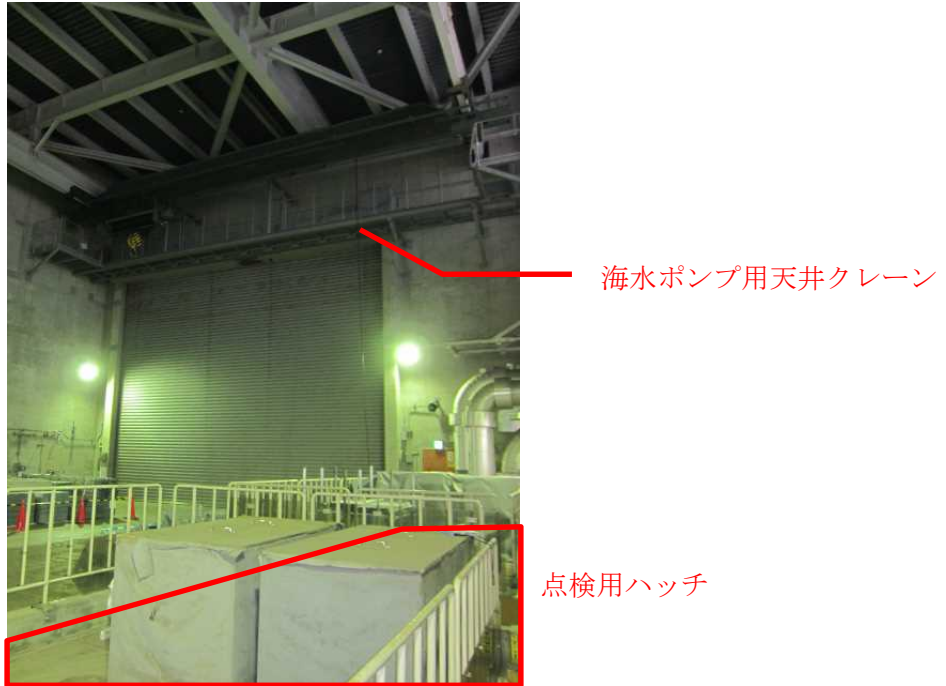
第5図 海水ポンプ用天井クレーン設置状況（7号炉北側）
