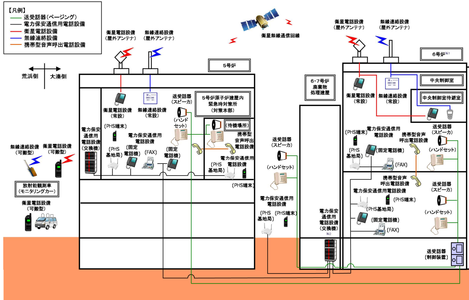
図 2.2-1 通信連絡設備（発電所内）の概要
