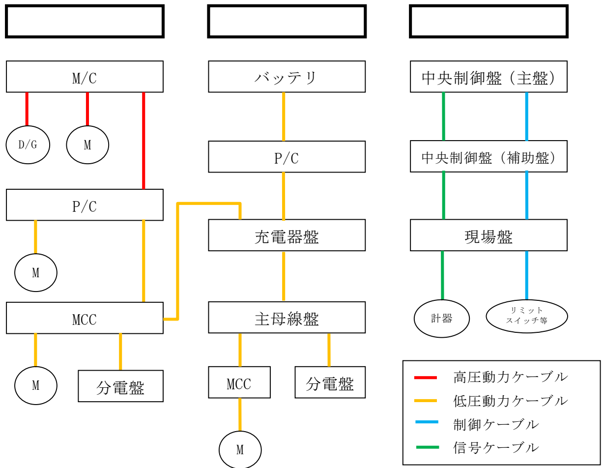
第 2-5 図：火災防護対策対象ケーブル調査範囲
