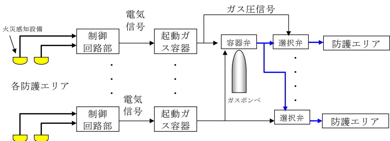
第3図 二酸化炭素消火設備の系統構成
