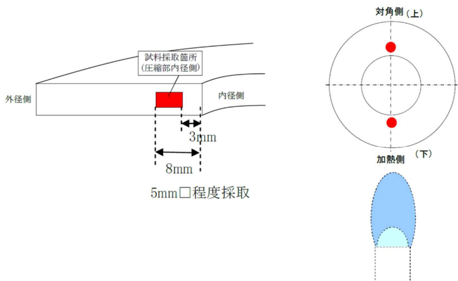
第3図 熱重量測定の実験箇所
