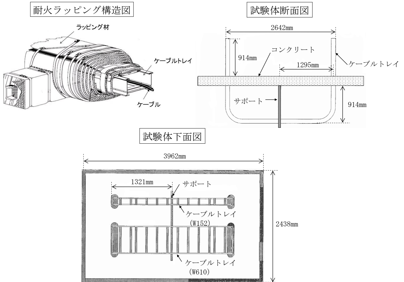
第 12 図 耐火ラッピング試験体構造の例
