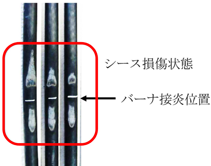
第2図 No.14同軸ケーブルのUL垂直燃焼試験後の状態
