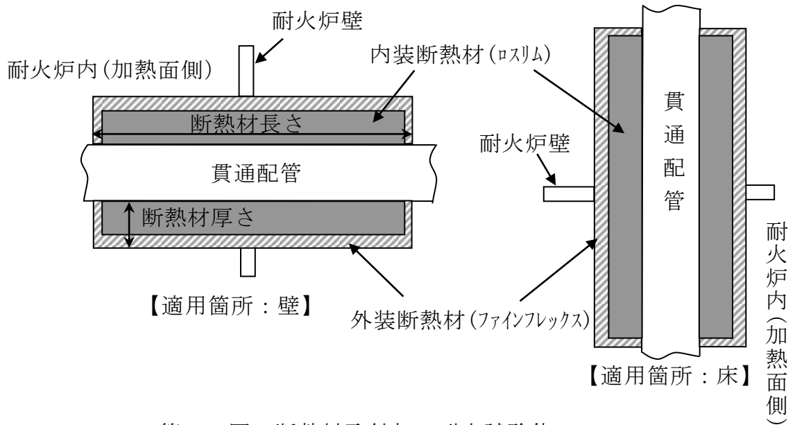
第4-1図 断熱材取付部の耐火試験体
