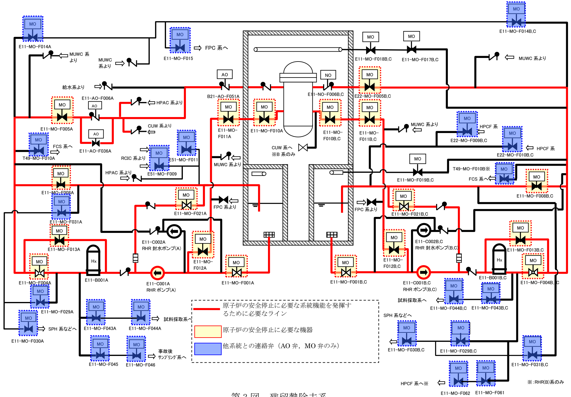
第 3 図 残留熱除去系
