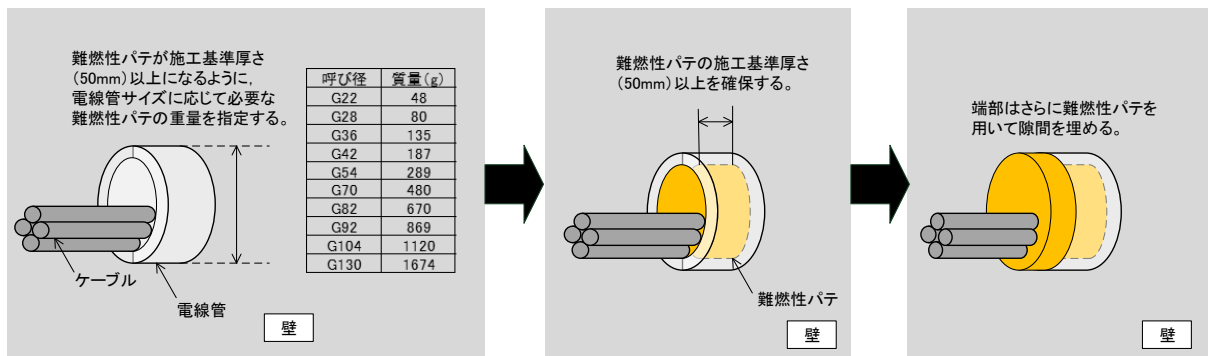
第8図 電線管貫通部処理時の管理方法（7号炉の例）
