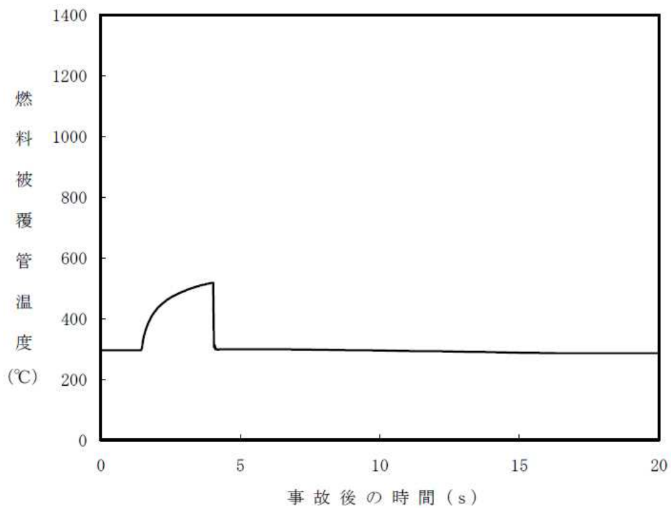
図 6-3 原子炉冷却材流量の喪失+給水制御系の故障解析結果 (R/B 起因) (2/2)
