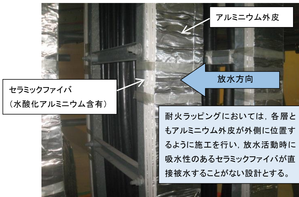
第 23 図 耐火ラッピング施工途中のケーブルトレイの外観写真
