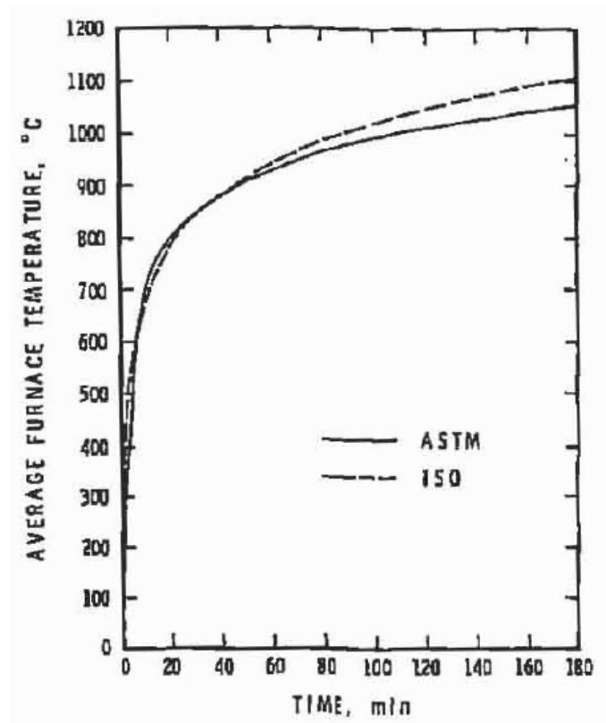
第 11 図 加熱曲線の比較(出典:Comparison of Severity of Exposure in ASTM E119 and IS0834 Fire Resistance Tests)
