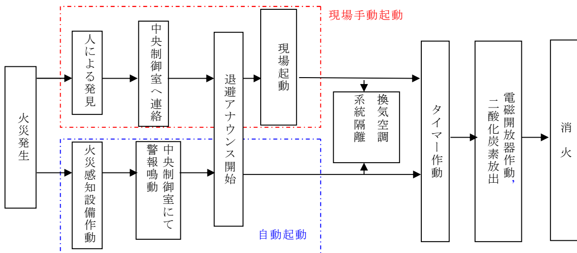
第2図 火災発生時の信号の流れ
