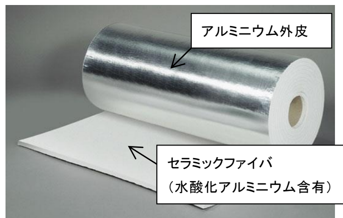
第 22 図 耐火ラッピング材料の外観写真
