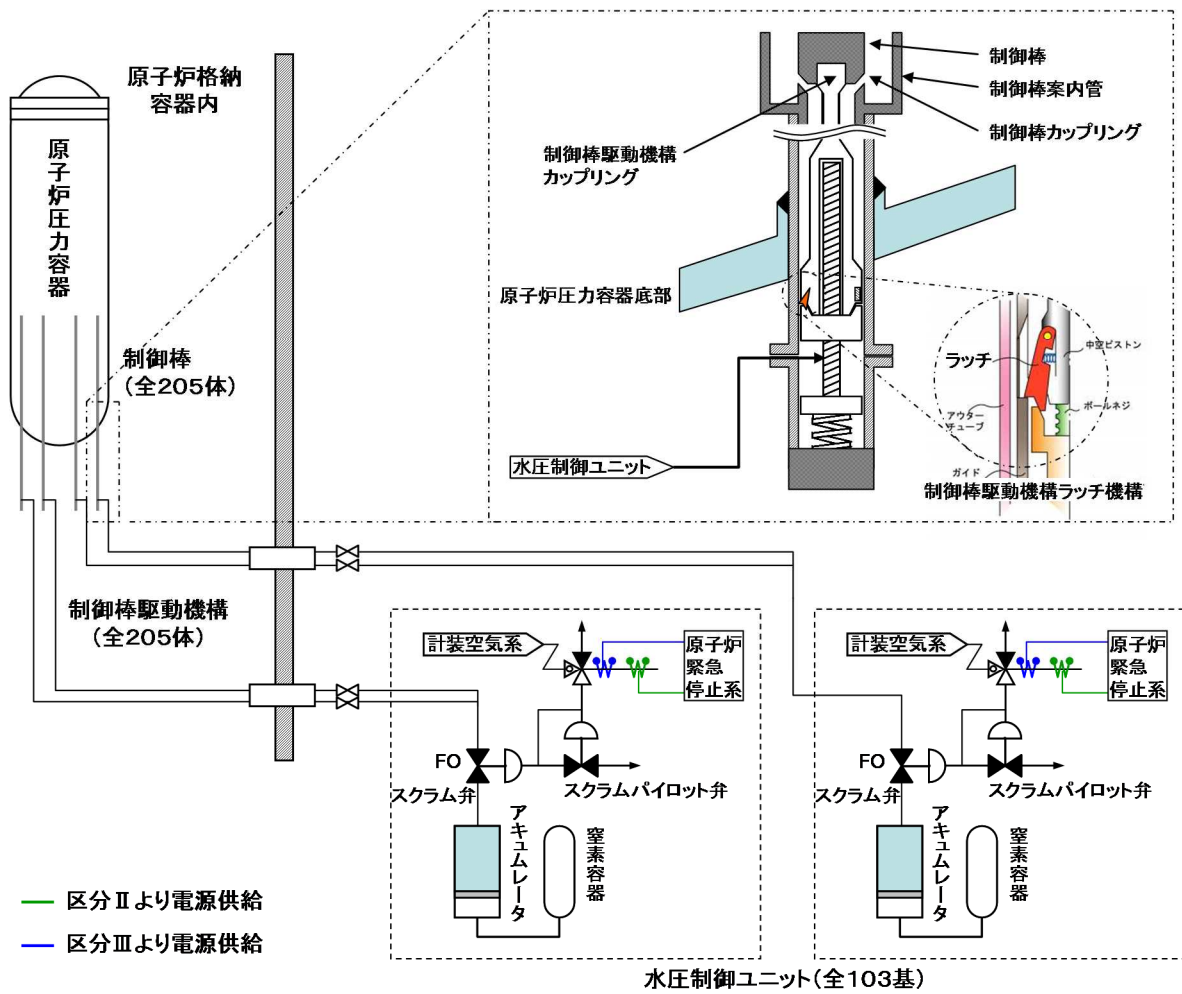
第1図：原子炉の緊急停止機能の概要
