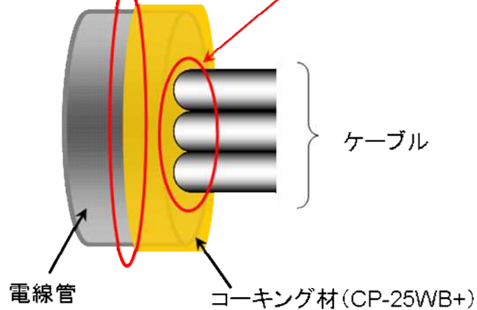
第2図：コーキング材（CP-25WB+）の施工方法
