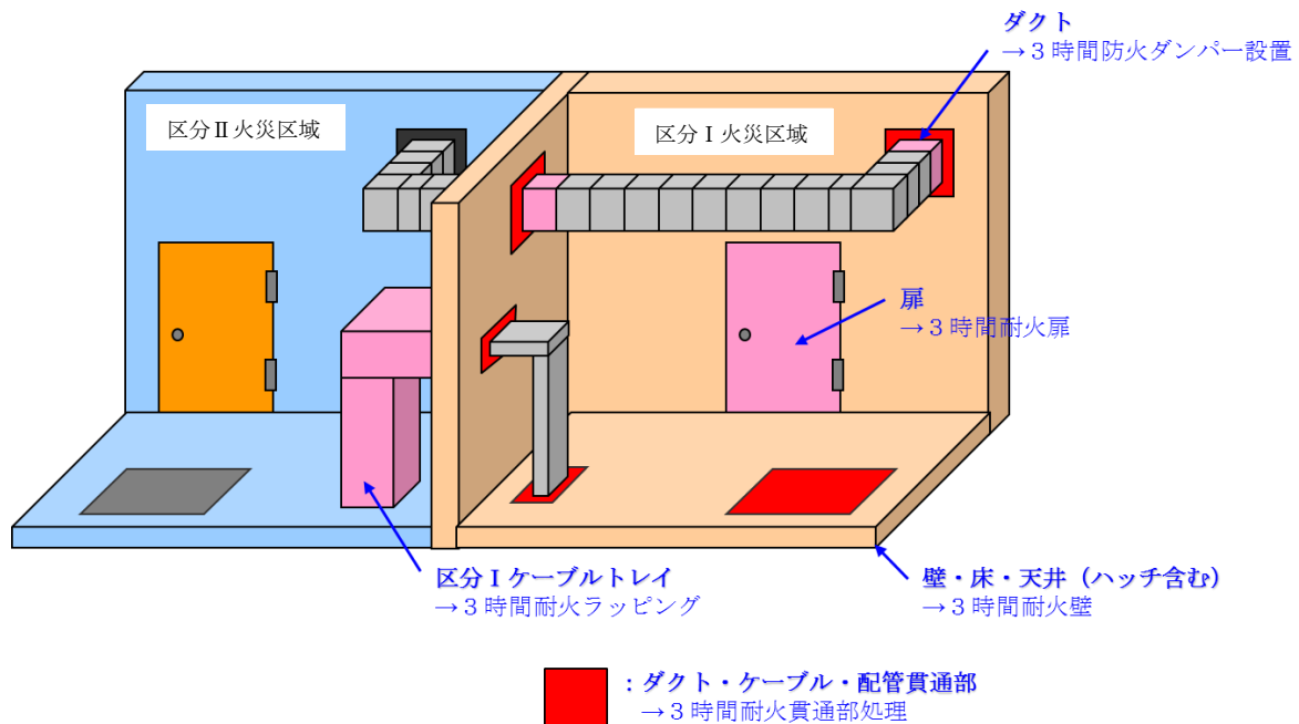
第2図：火災の影響軽減対策とケーブルラッピング
