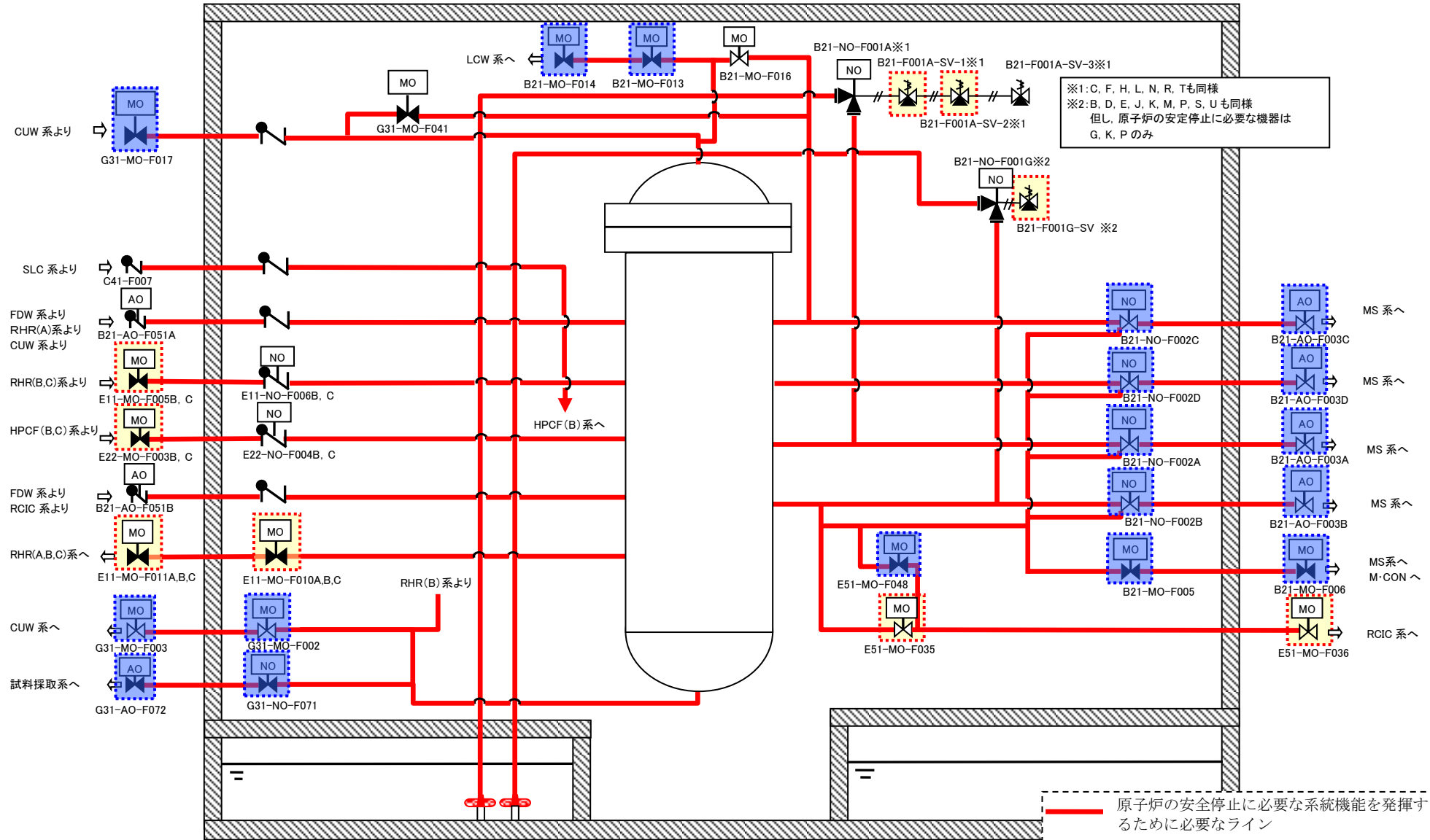
第1図 原子炉冷却材圧力バウンダリ/自動減圧系/逃がし安全弁
