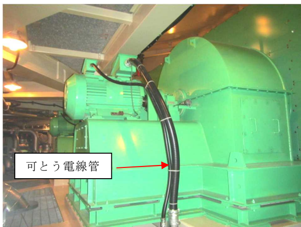
機器へのケーブル取合い状況 (D/W 冷却機との取合い)
