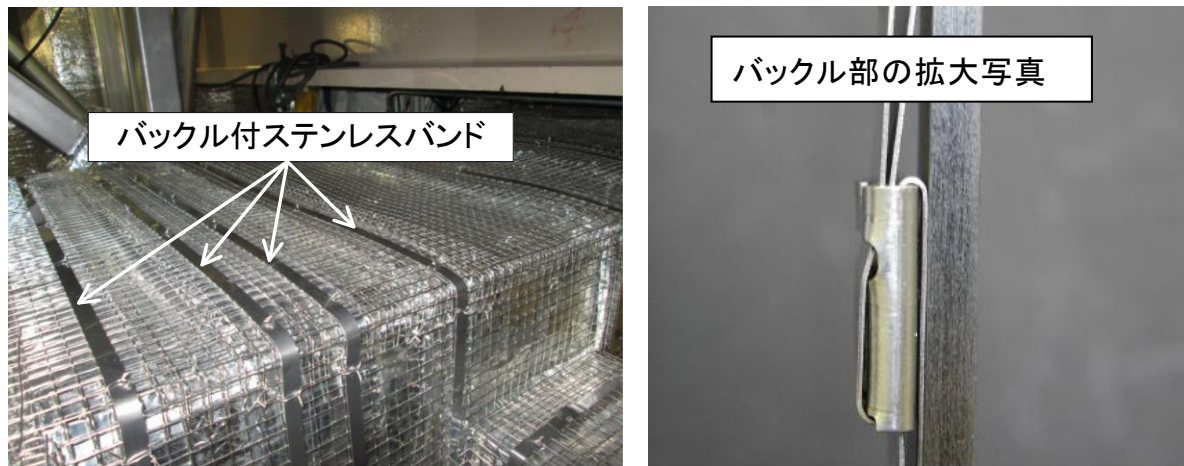
第 20 図 耐火ラッピングの固定状況
