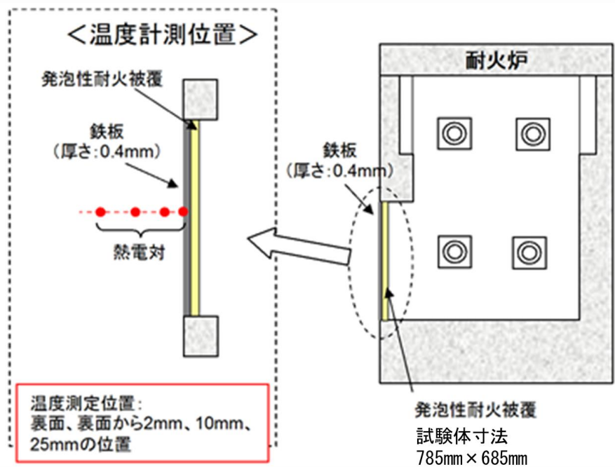
第 3-1 図 鉄板+発泡性耐火被覆 試験体
