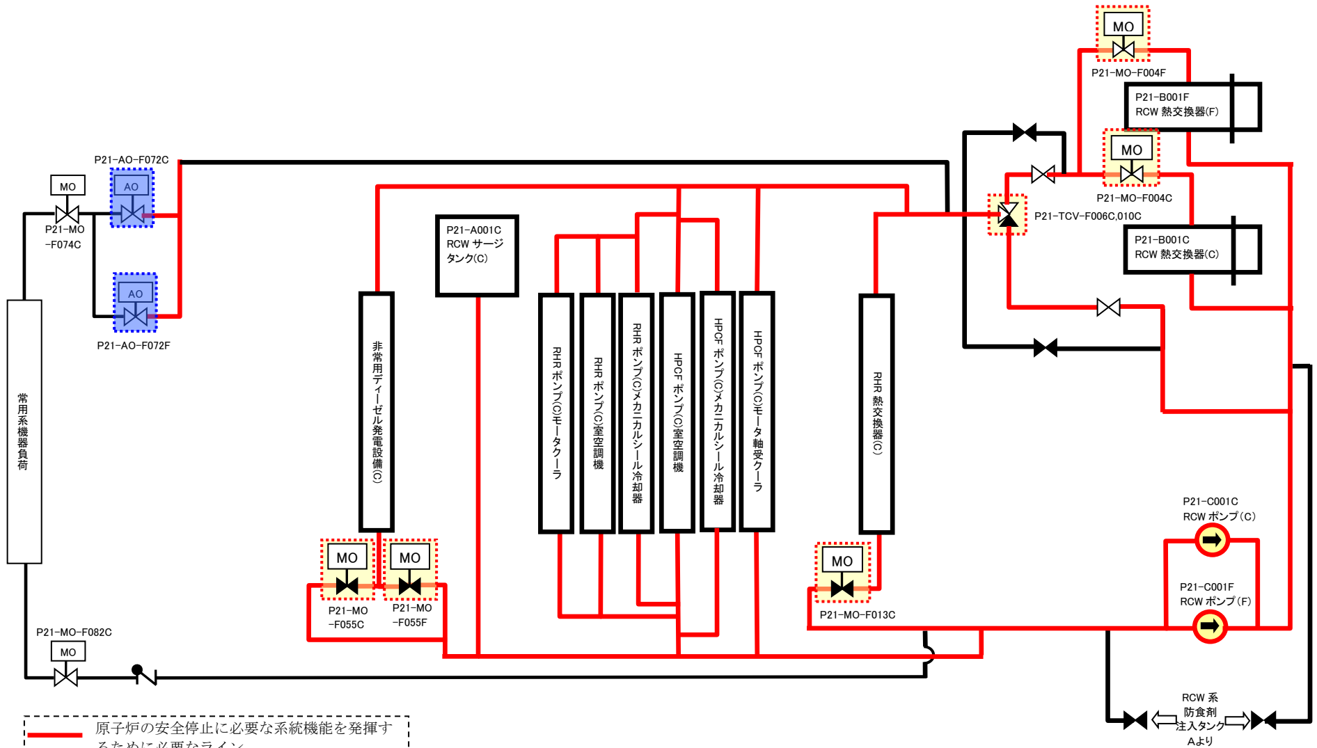
第 7 図 原子炉補機冷却系 (その 2)
