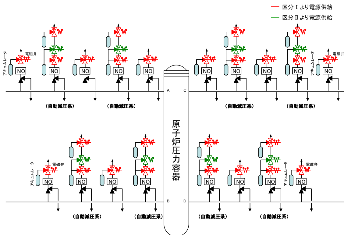
第 4 図：原子炉冷却材圧力バウンダリの過圧防止機能の概要
