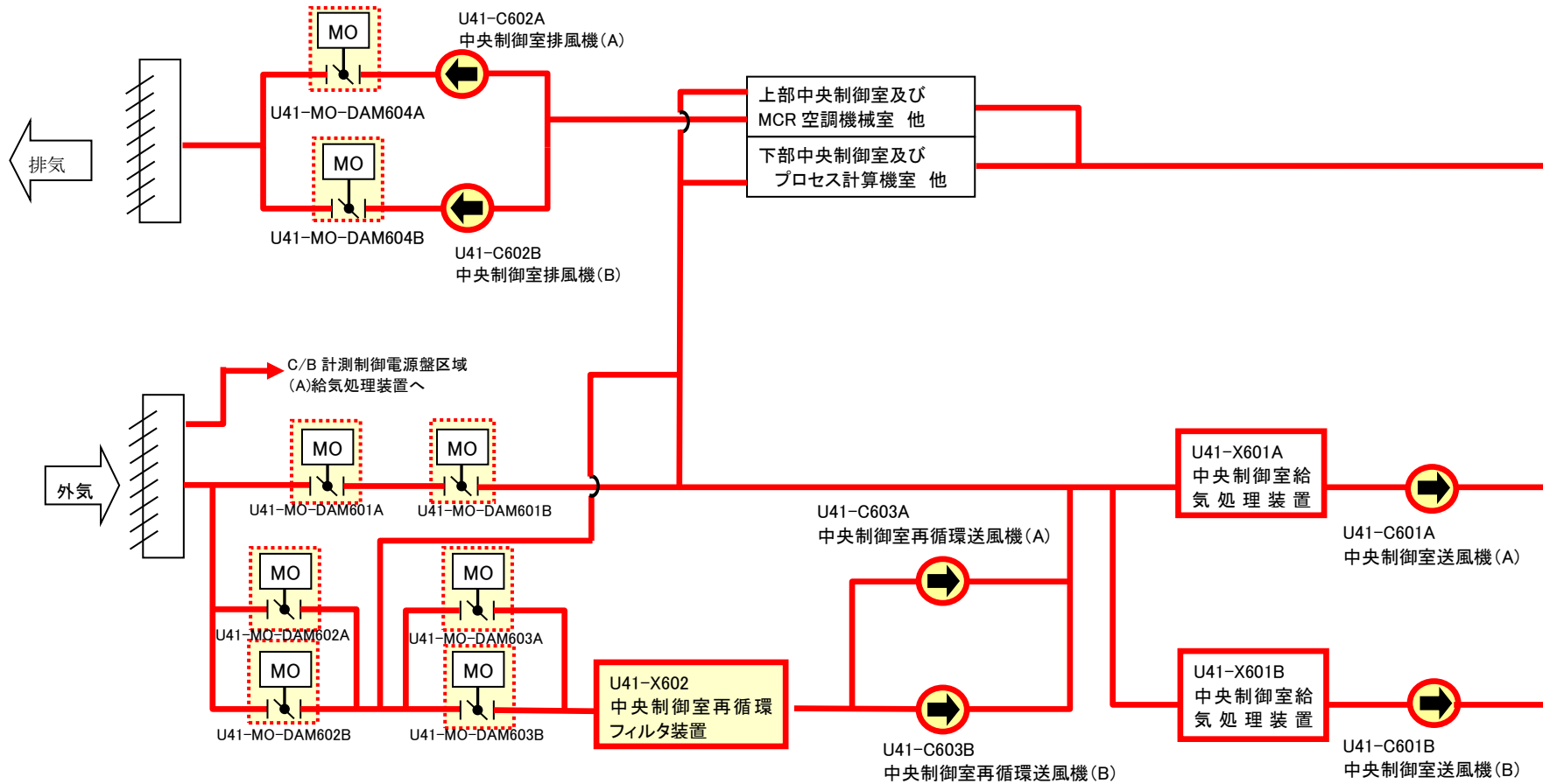
第 14 図 中央制御室非常用換気空調系
