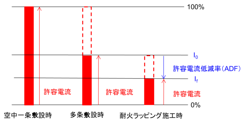
第 13 図 ケーブル許容電流と許容電流低減率（ADF）
