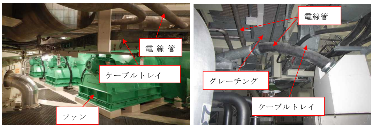
第 8-7 図 原子炉格納容器内の機器等の設置状況
