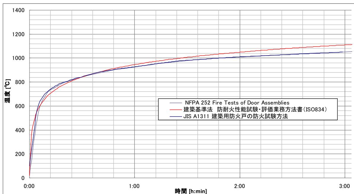
第 2 図 加熱曲線の比較
