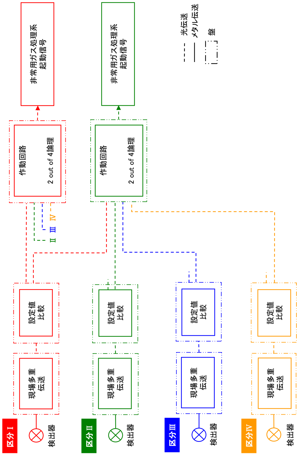
第20図：非常用ガス処理系の安全保護回路の概要図
