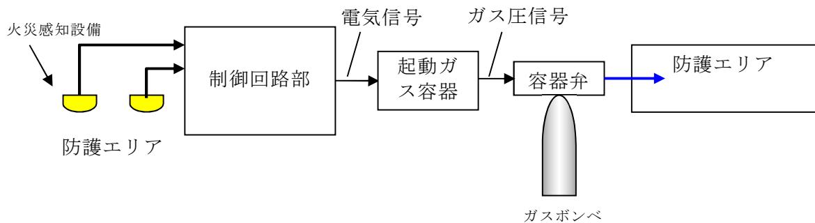
第7図：全域ガス消火設備（専用型）の系統構成
