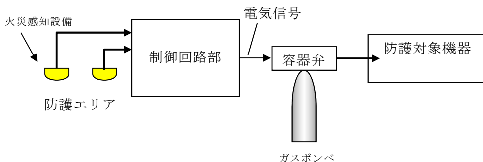
第9図：局所ガス消火設備（油内包機器，盤）の系統構成
