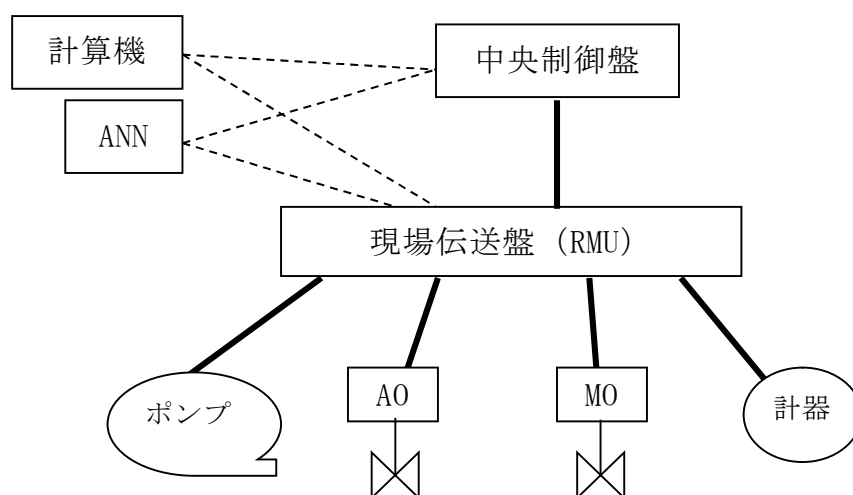
第2-6図：制御系ケーブル抽出対象範囲
