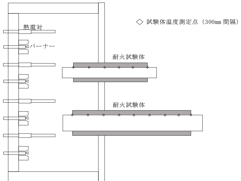
第4-2図 耐火試験炉
