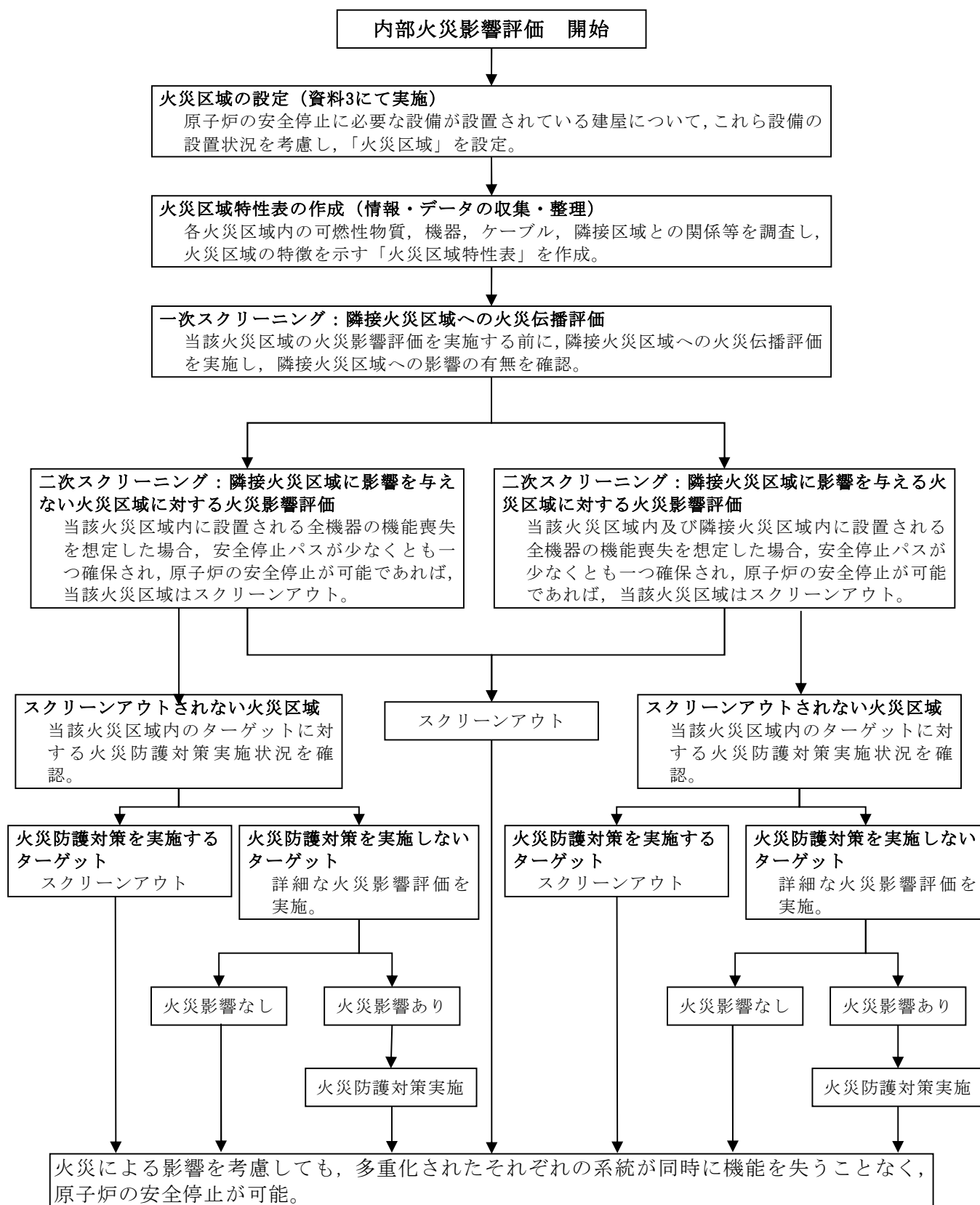
第10-1図 火災影響評価の手順の概要フロー
