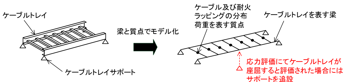
第 19 図 耐火ラッピング後のケーブルトレイ耐震性評価の概要
