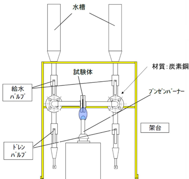
第1図 加熱試験の概要
