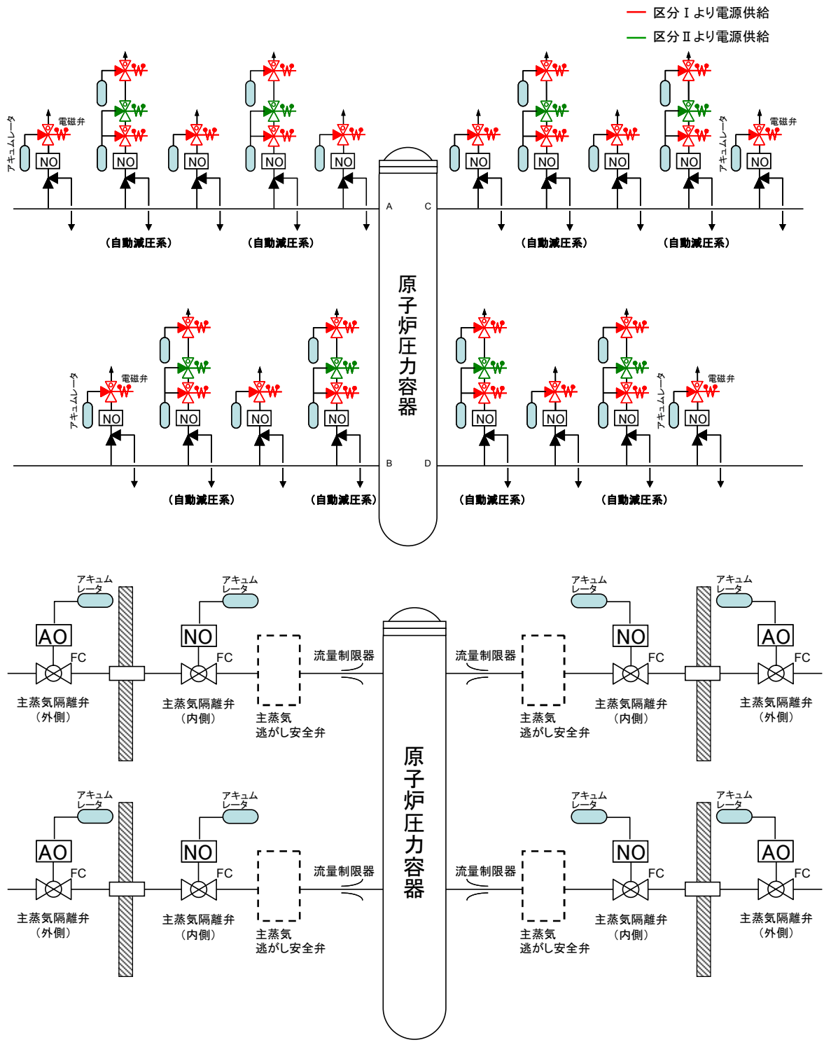
第 13 図：圧縮空気供給機能の概要
