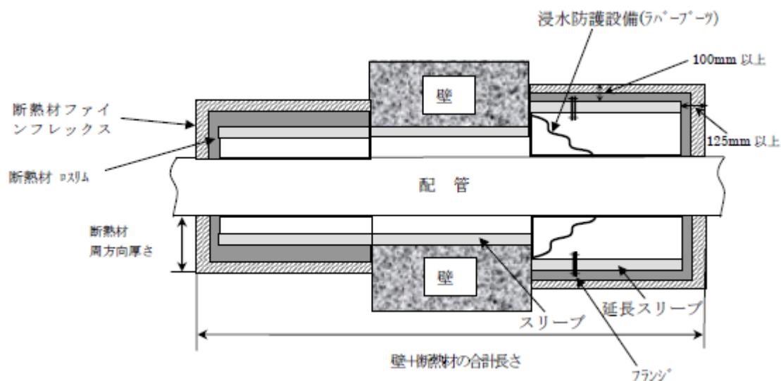
第 4-3 図 干渉物が有る場合の断熱材施工例
