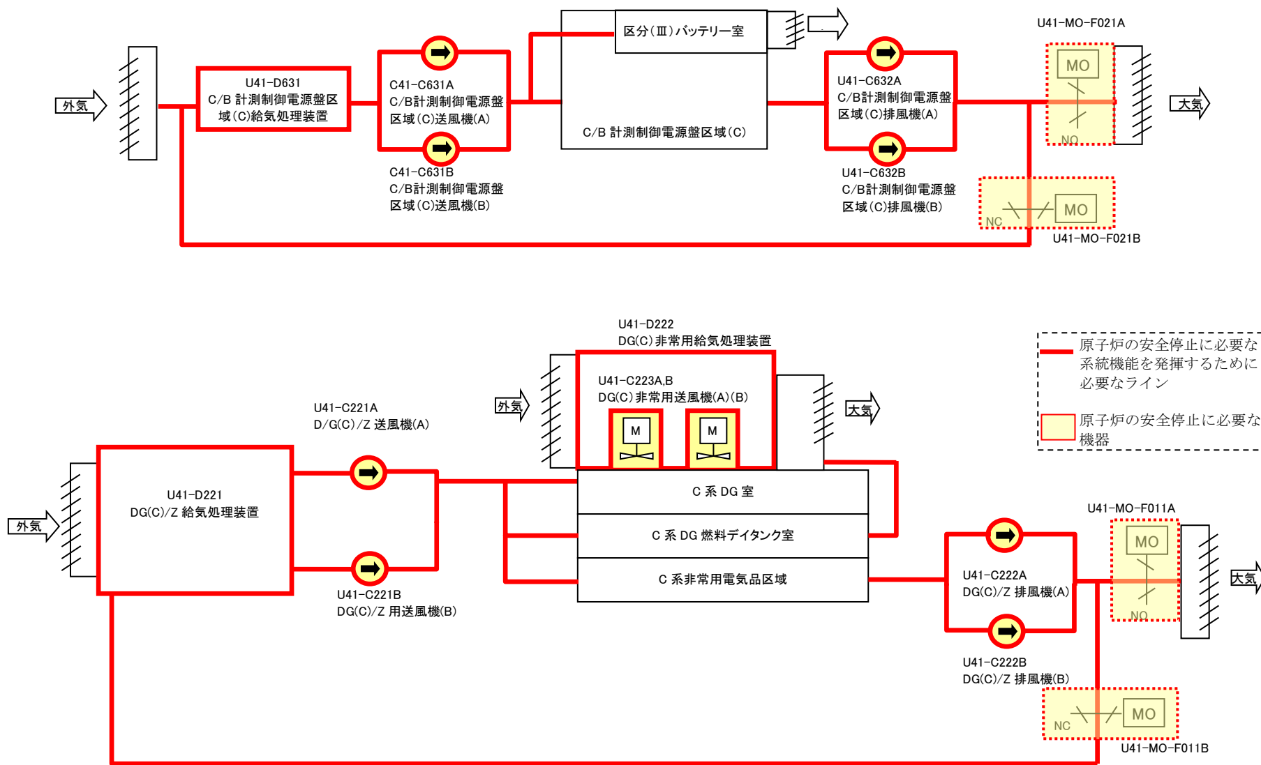
第 13 図 非常用換気空調系 (その 2)
