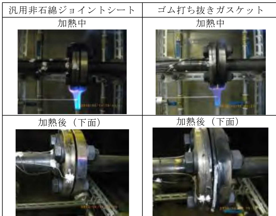
第2図 試験体の加熱状況
