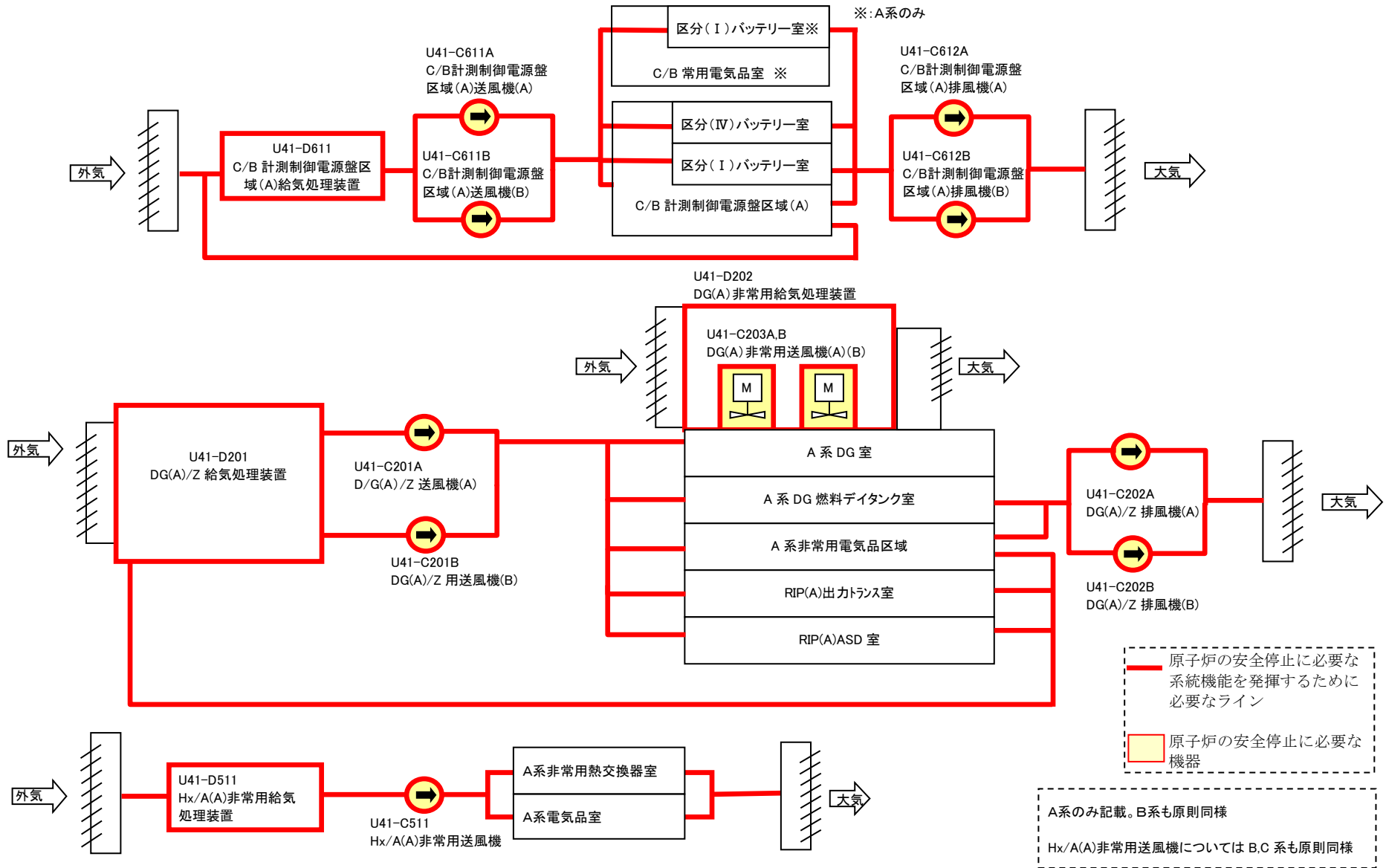
第 12 図 非常用換気空調系 (その 1)
