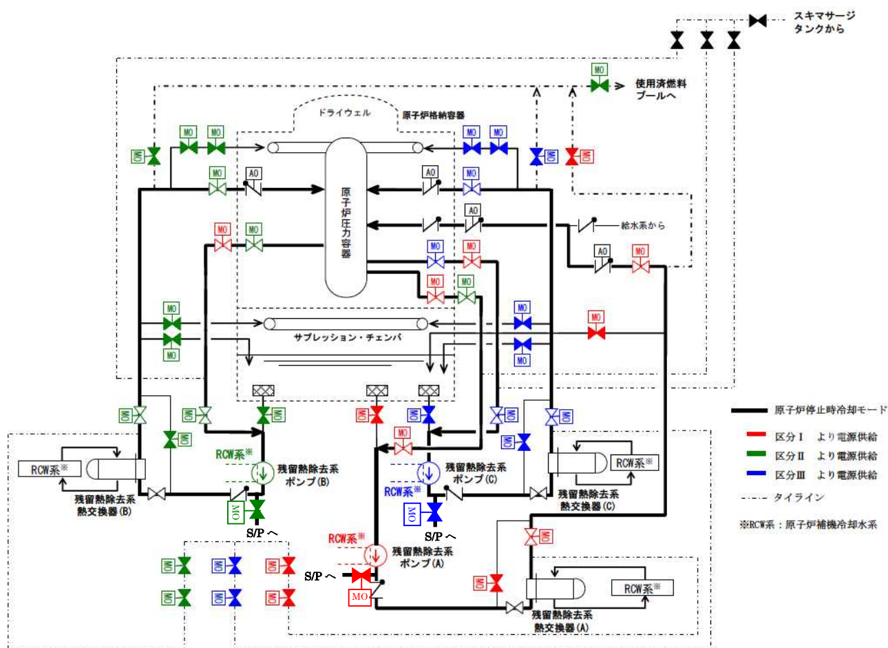
第1図 残留熱除去系（原子炉停止時冷却モード）
