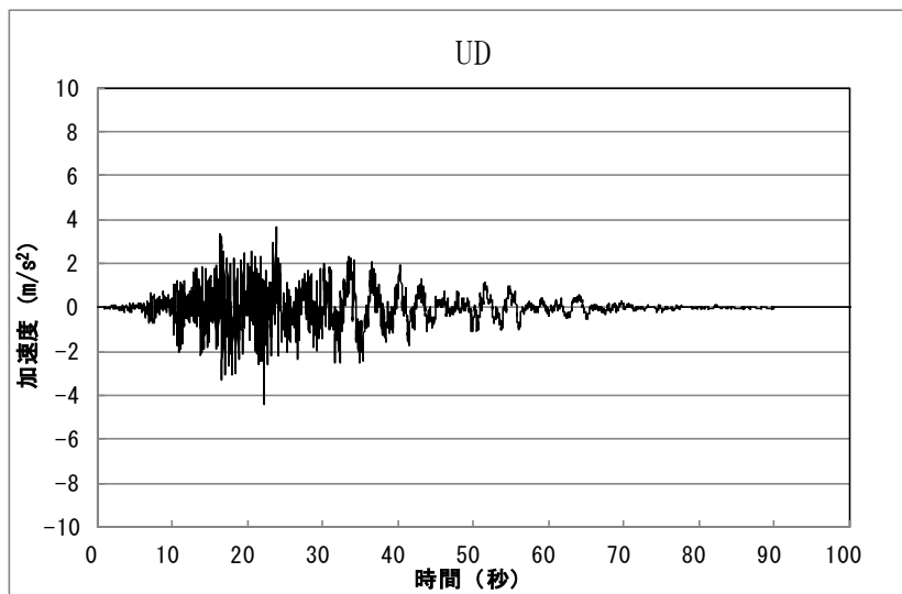
第 8.1-5 図 基準地震動 Ss-7 時刻歴加速度 (7号炉)
