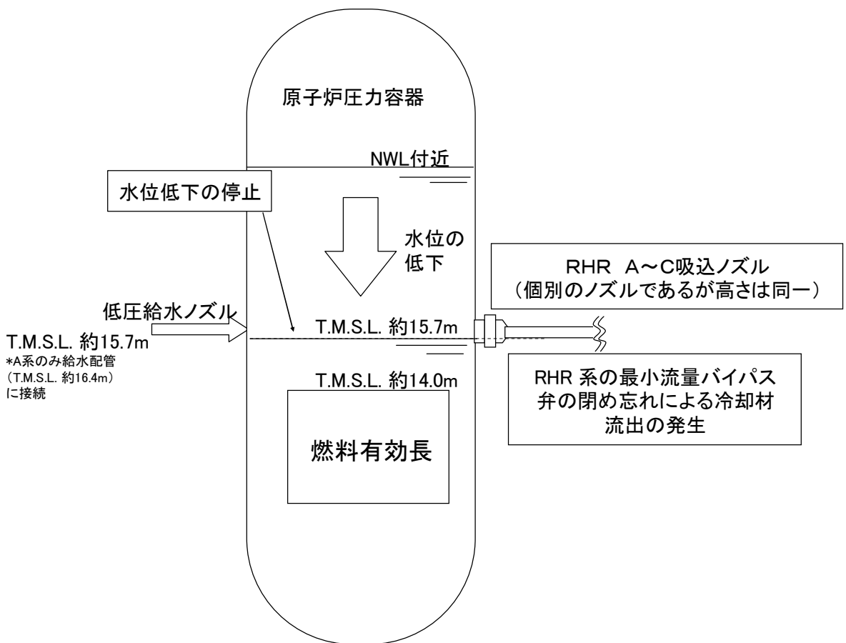
図 RHR 吸込配管のノズルの高さ と燃料有効長頂部の高さ
