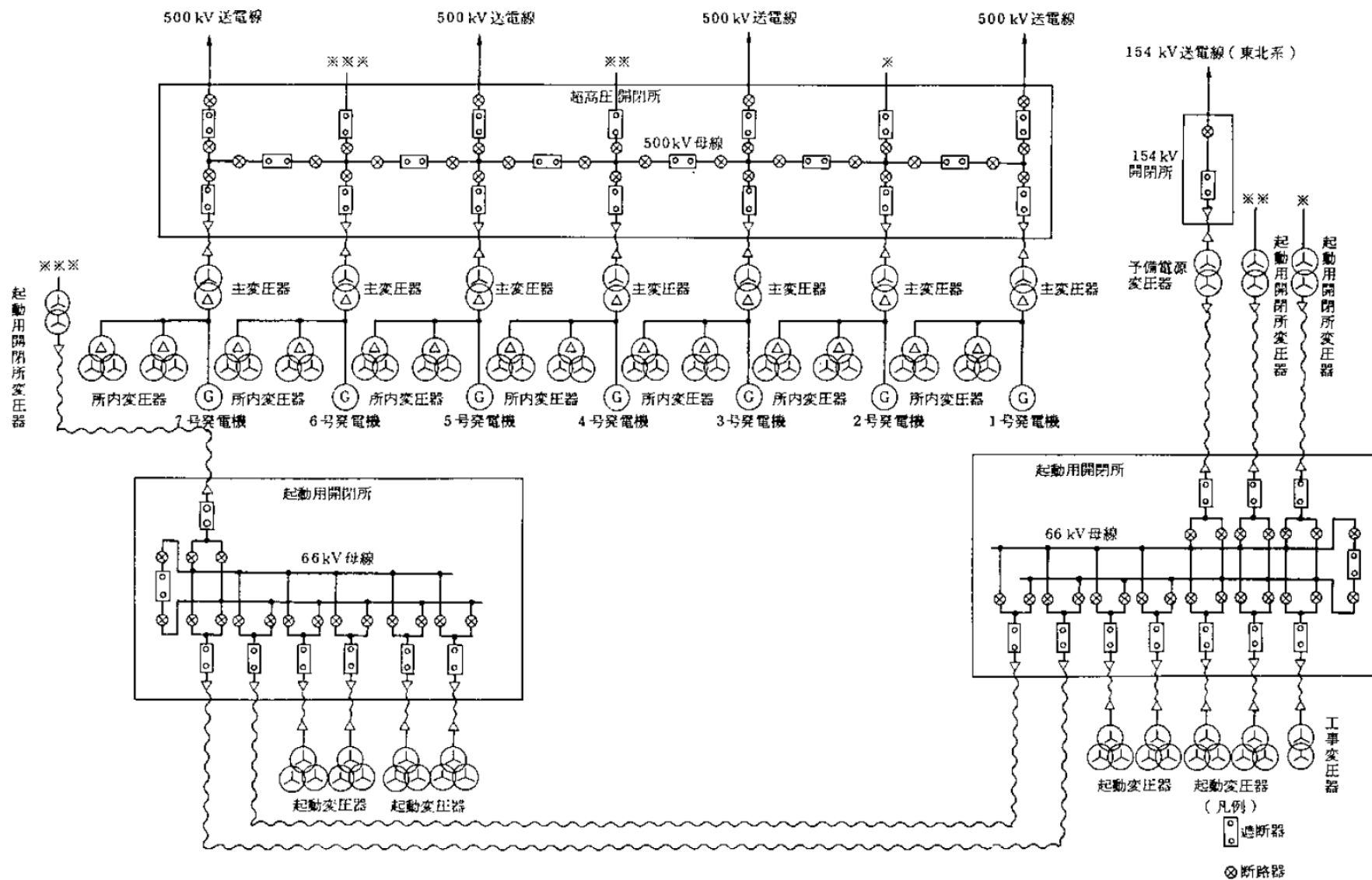
第 1.1.1. a-17 圖 開閉所單線結線圖
