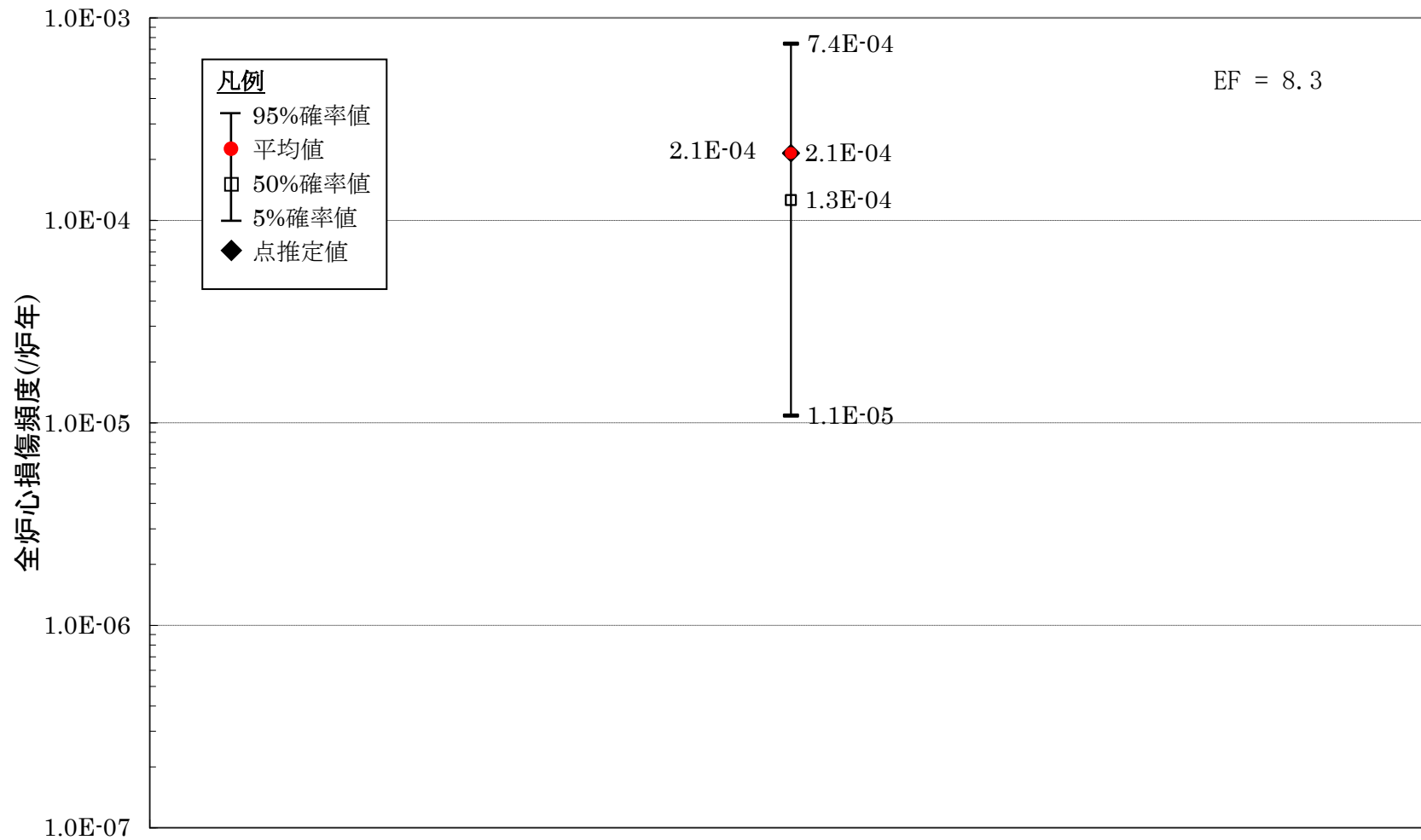
第 1. 2. 2. d-6(a) 図 不確実さ解析の結果 (7 号炉)
