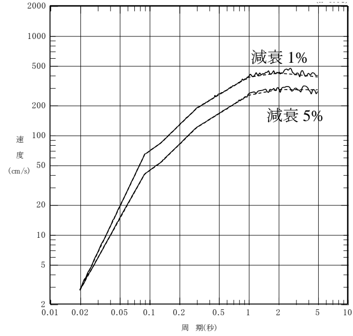
第 1. 2. 1. b-20 図 フラジリティ評価に用いる模擬地震波と目標応答スペクトルに対するフィッティング (大湊側)
