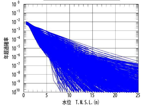
2000本のハザード曲線 (大湊側遡上域)
