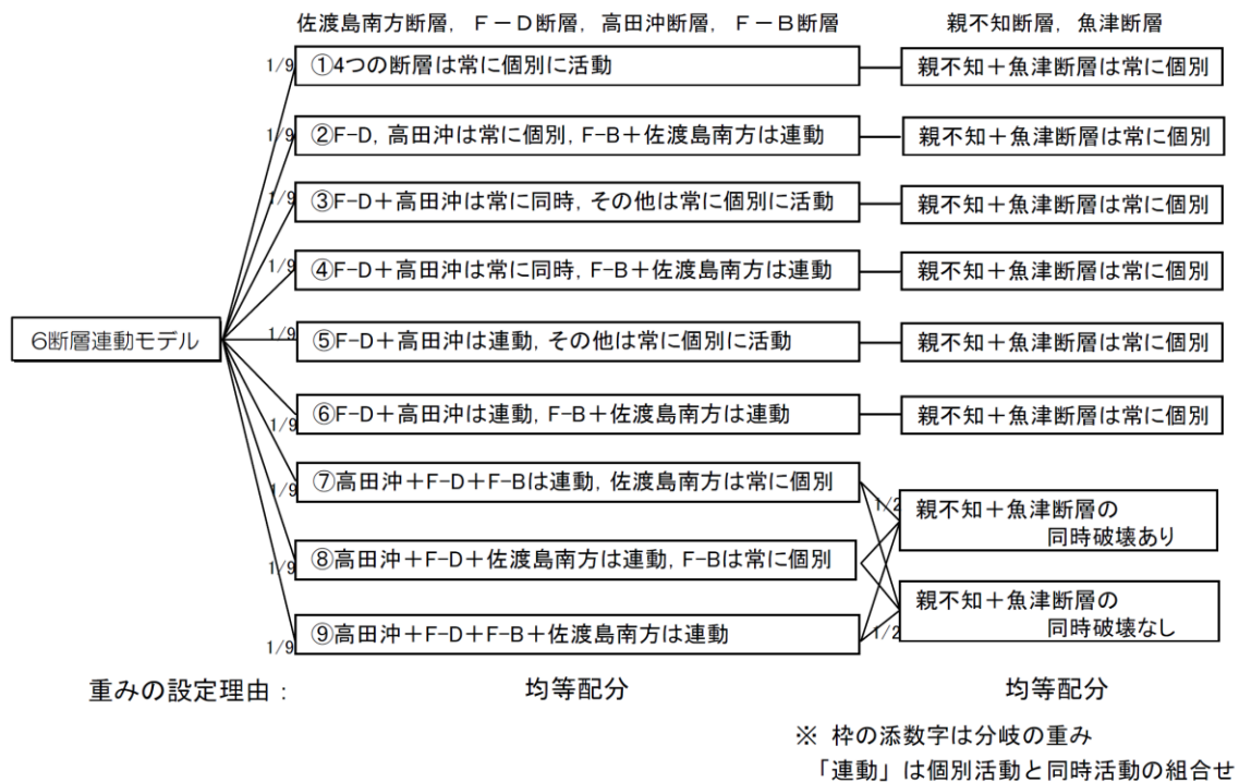
第 1. 2. 2. b-2 図 断層連動に関するロジックツリー (6断層連動モデル)
