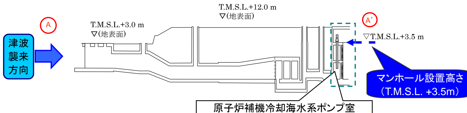
7号炉取水設備断面図
