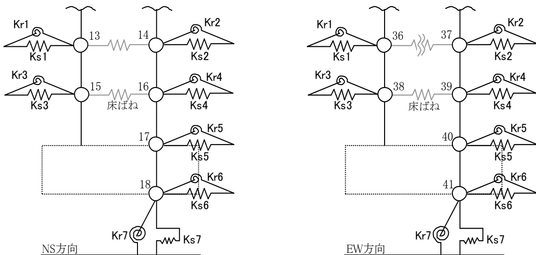
第 1.2.1. c-1-11(3) 図 地盤ばねの記号
