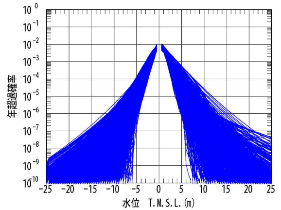
2000本のハザード曲線 (1号炉取水口前面)
