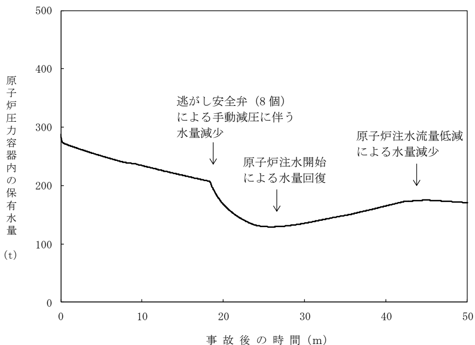
第 2.6.11 図 原子炉压力容器内の保有水量の推移
