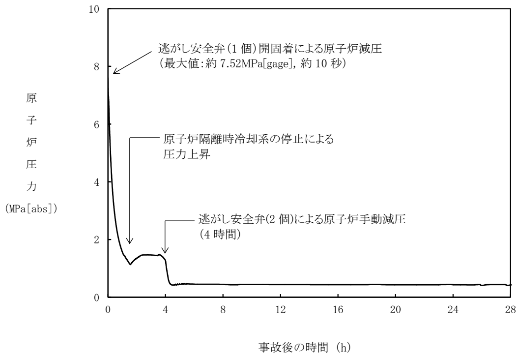
第 2.3.4.7 図 原子炉圧力の推移
