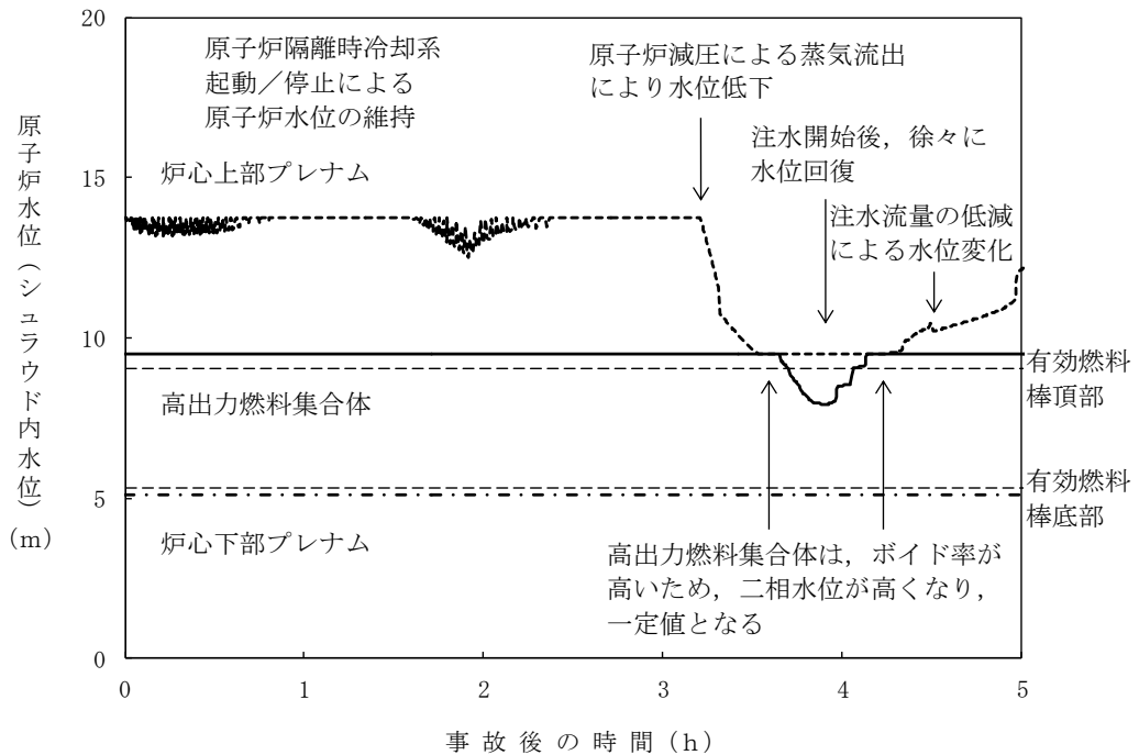
第 2.4.1.8 図 原子炉水位 (シユラウド内水位) の推移
