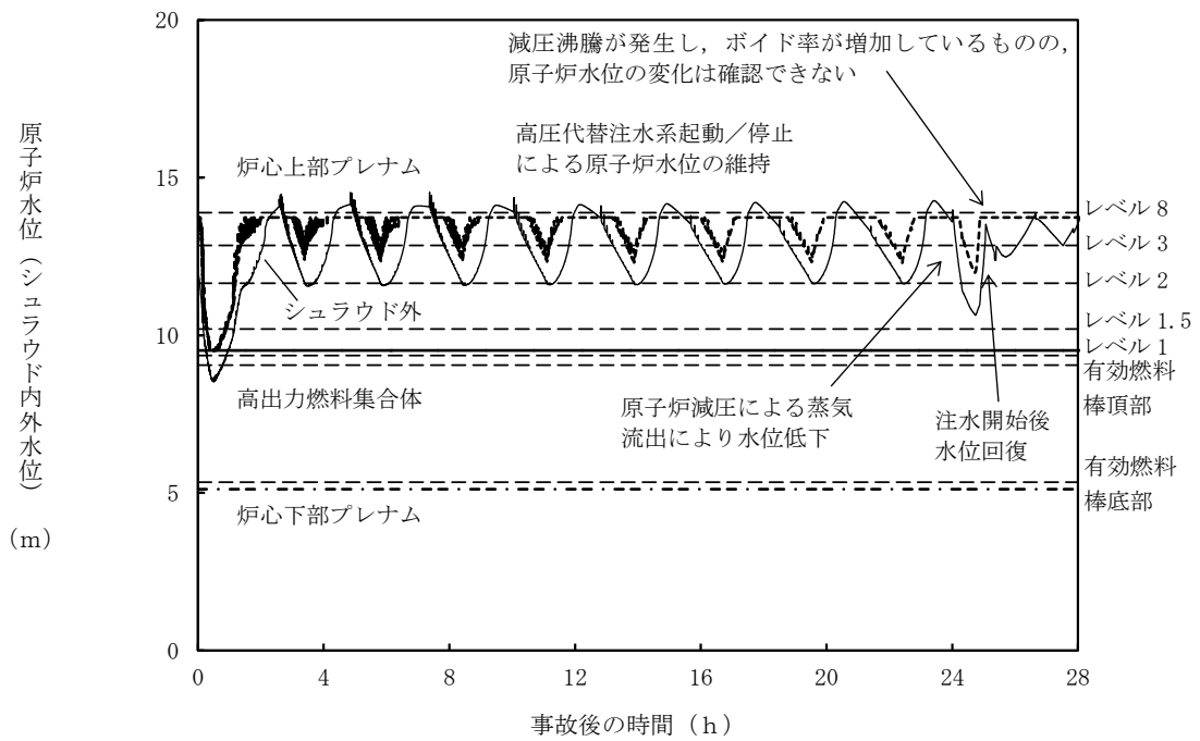
第 2.3.2.9 図 原子炉水位（シユラウド内外水位）の推移
