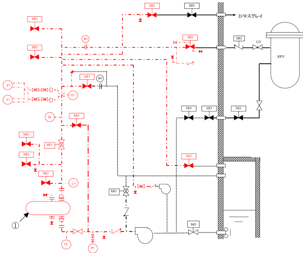
図-補5：評価対象の熱交換器
