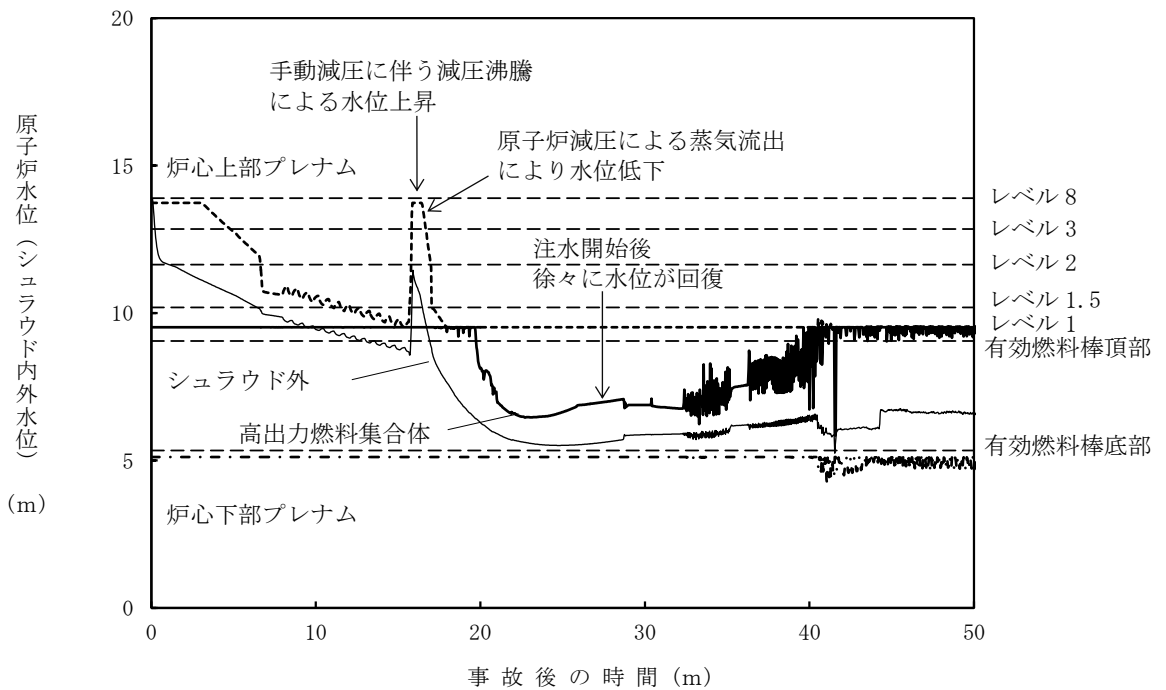
第 2.6.24 図 原子炉水位 (シュラウド内外水位) の推移
