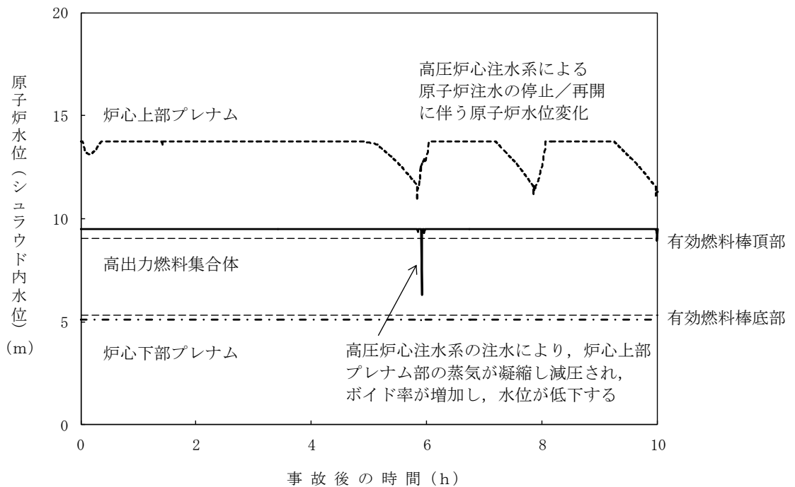
第 2.4.2.7 図 原子炉水位 (シミュラウド内水位) の推移
