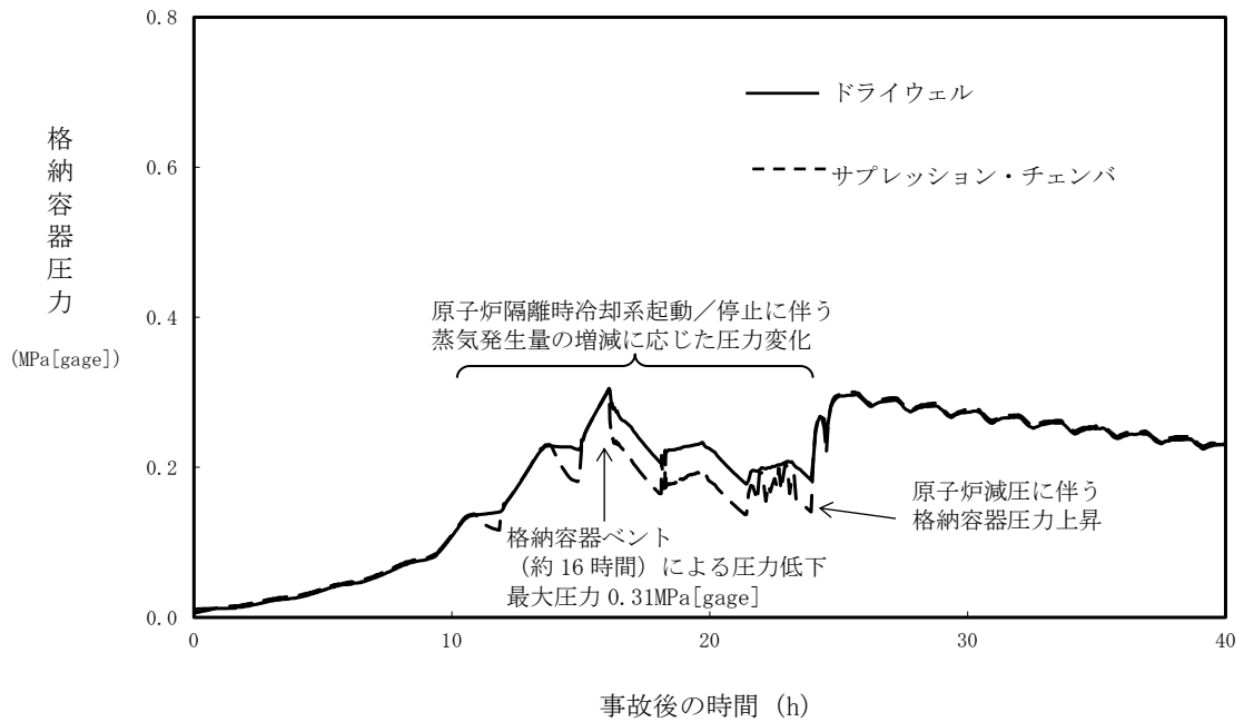
第 2. 3. 1. 16 図 格納容器圧力の推移
