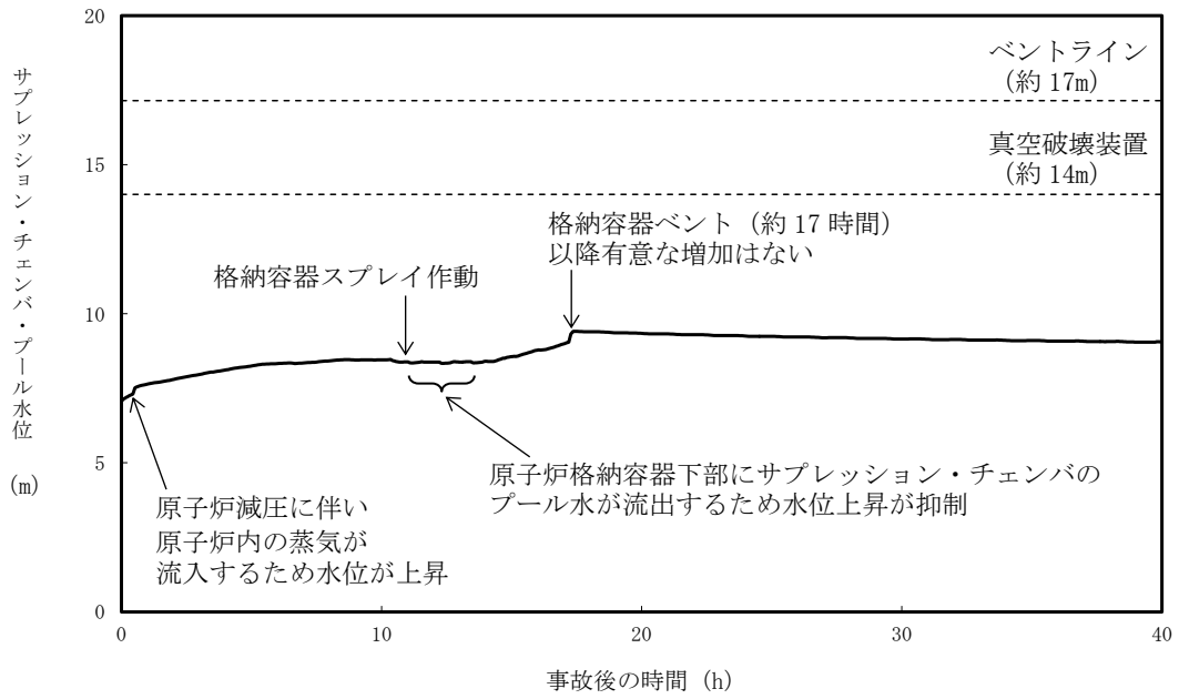
第 2.1.20 図 サプレッション・チェンバ・プール水位の推移
