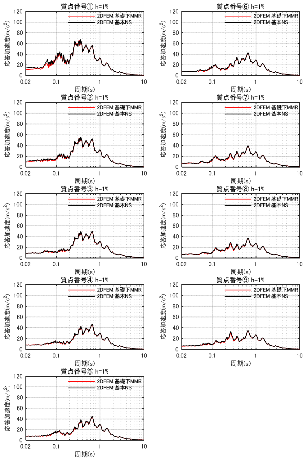
第 5.4 図 床応答スペクトルの比較 (基本モデルと 6 号炉基礎下マンメイドロックモデル) (NS 方向) h=1\%
