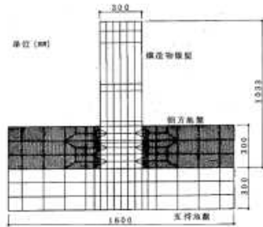
図-2 解析モデル (埋め込み深さ 30cm)
