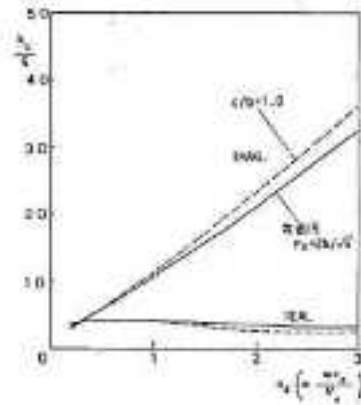
図 7.2 正方形平面と等価円の K_H
