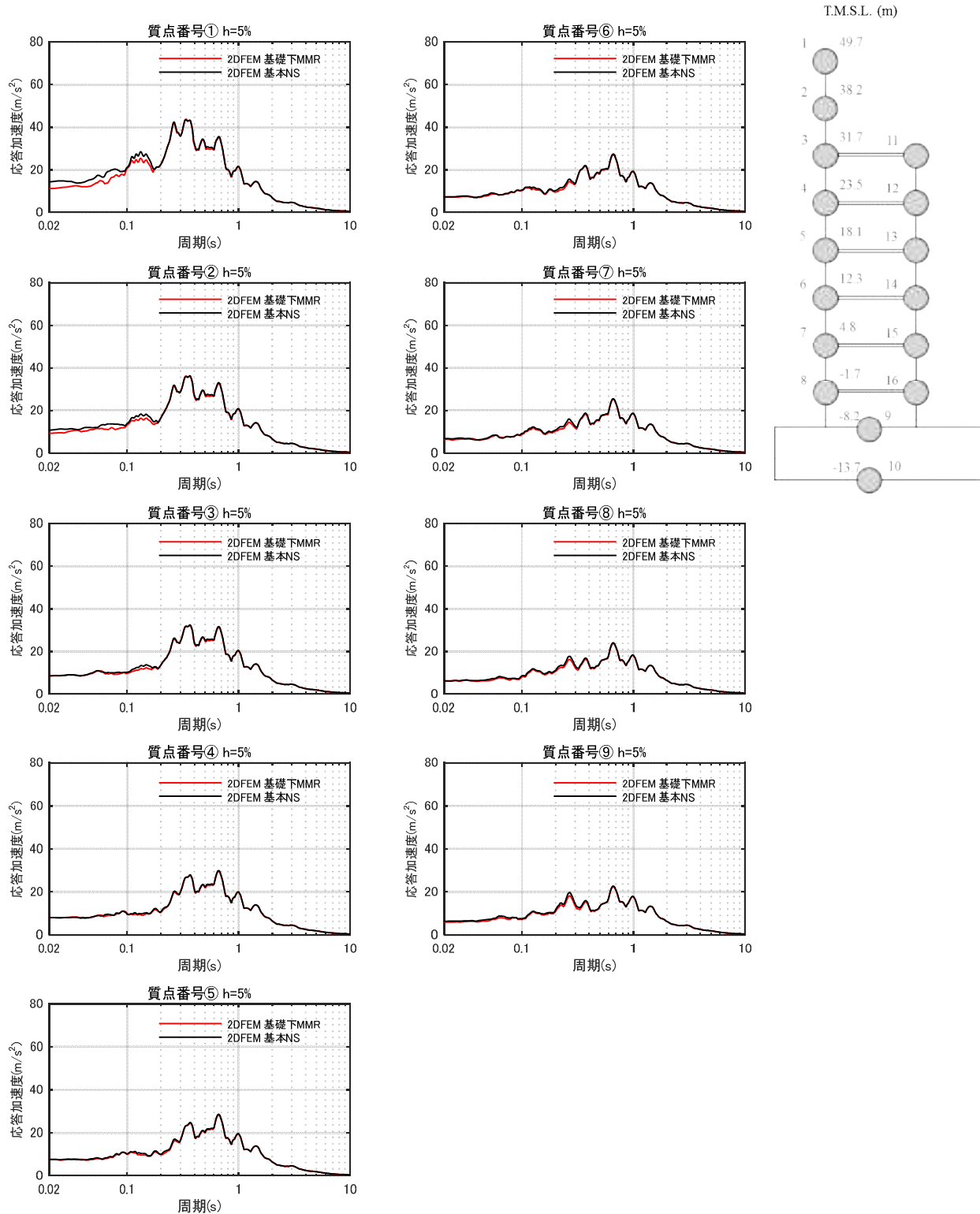
第 5.3 図 床応答スペクトルの比較 (基本モデルと 6 号炉基礎下マンメイドロックモデル) (NS 方向) h=5\%
