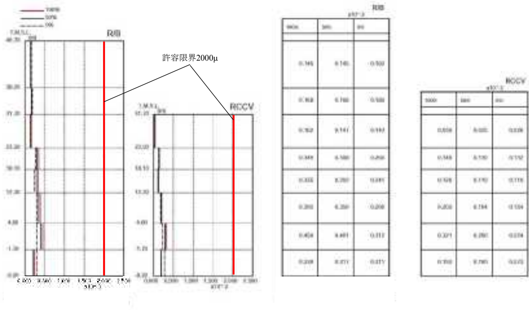
第7図 最大応答せん断ひずみ(6号炉原子炉建屋、NS方向、Ss-1)
