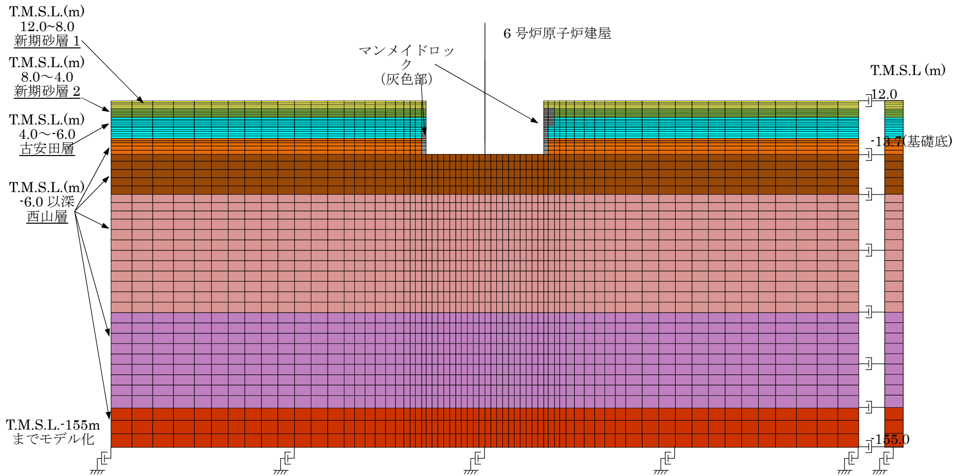
第 4.1.2.1 図 地盤メッシュ図 (NS 方向)
