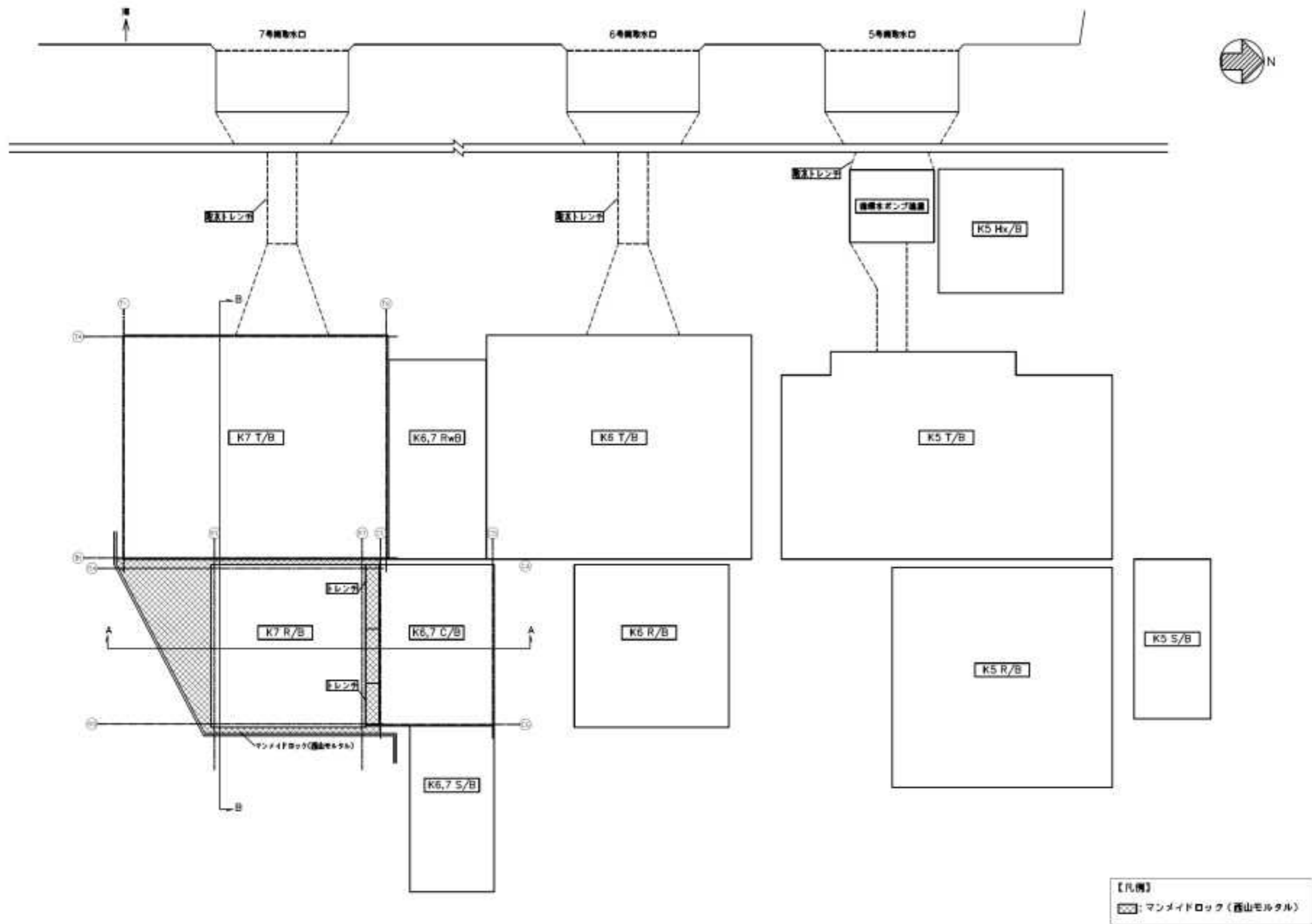
第 2.3.4 図 7号炉原子炉建屋の設置状況（平面図）
