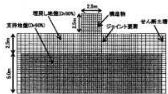
図5 2次元FEM解析モデル (1g場換算表示)
