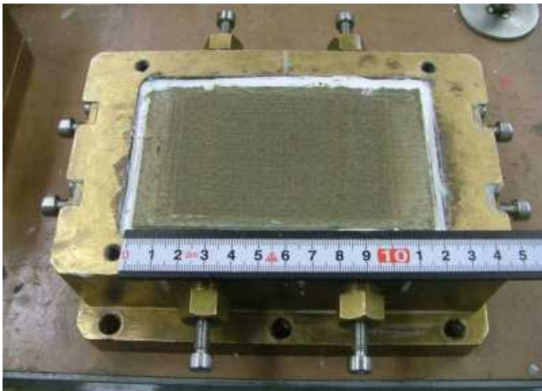
第 3.3.20 図 繰返し載荷試験後の供試体状況 ケース 1-8 (西山モルタル表面)
