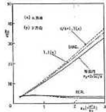
図 7.4 c/d=1.1 と等価円の K_H
