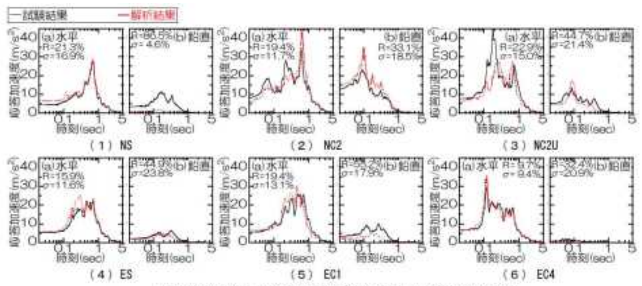
図3 構造物頂部における加速度応答スペクトル (減衰5%) の比較
