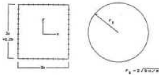
図 7.3 c/d=1.1 の長方形平面のBEM解析モデルと等価円半径 r_0
