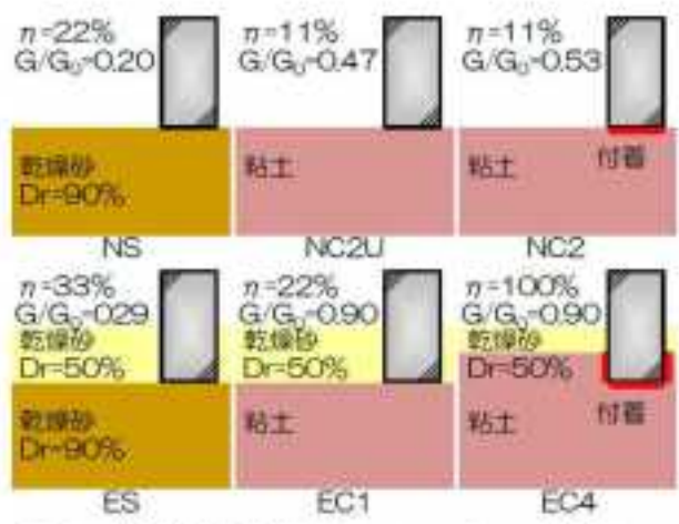
図1 遠心振動台実験のシミュレーション解析ケース
