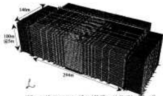
図1 3次元FEMモデル(基礎-地盤系)
