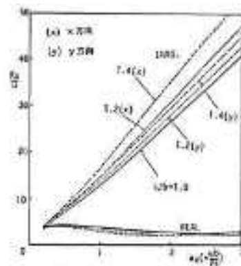
図 7.6 辺長比の違いによる K_H の比較
