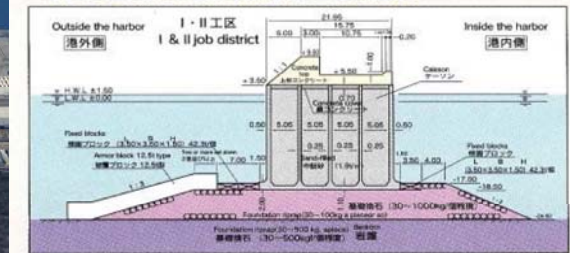
東防波堤標準構造
