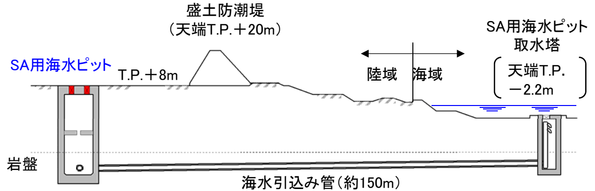
【取水塔～SA用海水ピット断面図】
