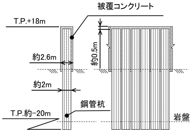
<断面図>
