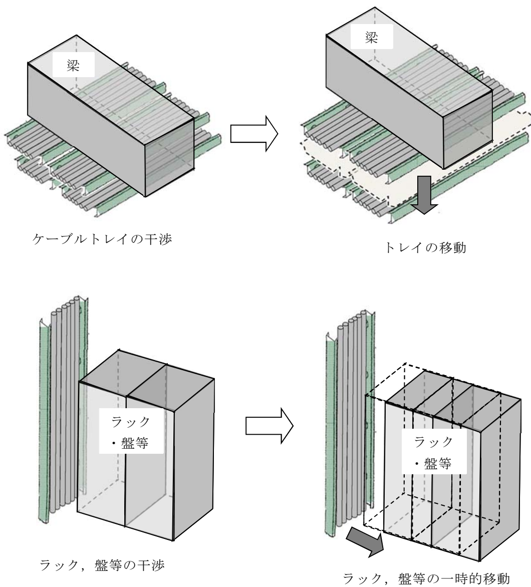
第 5.1-5 図 干渉物移動による作業
