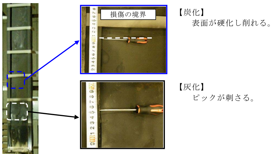
第 3-4-1 図 ケーブル及び防火シートの損傷長の判定方法
