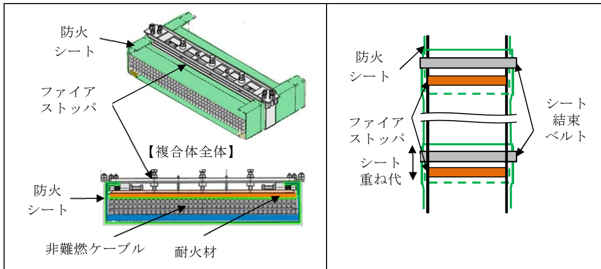
第 1.3-3 図 ファイアストップの施工例
