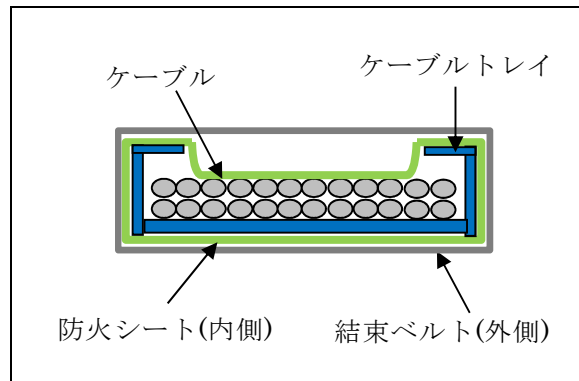
第 1.3-2 図 複合体形成の施工例
