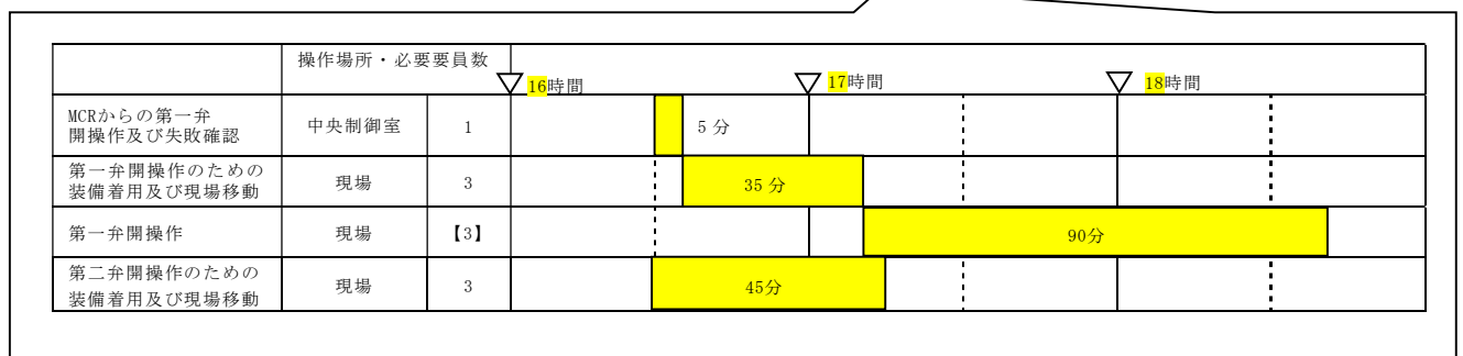
図 4.1.3-5 ベント準備操作のタイムチャート
