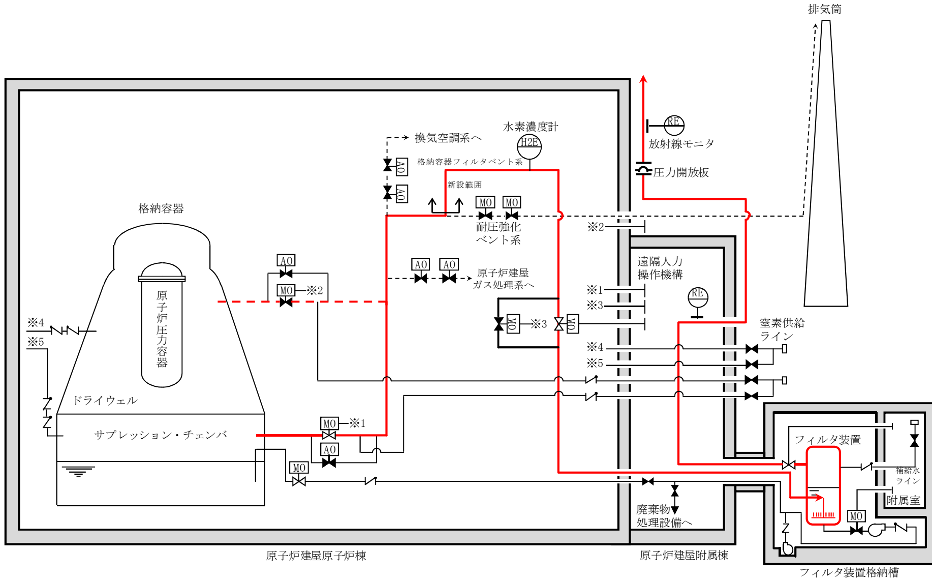
第 1.3-1 図 格納容器フィルタベント系 系統概要図
