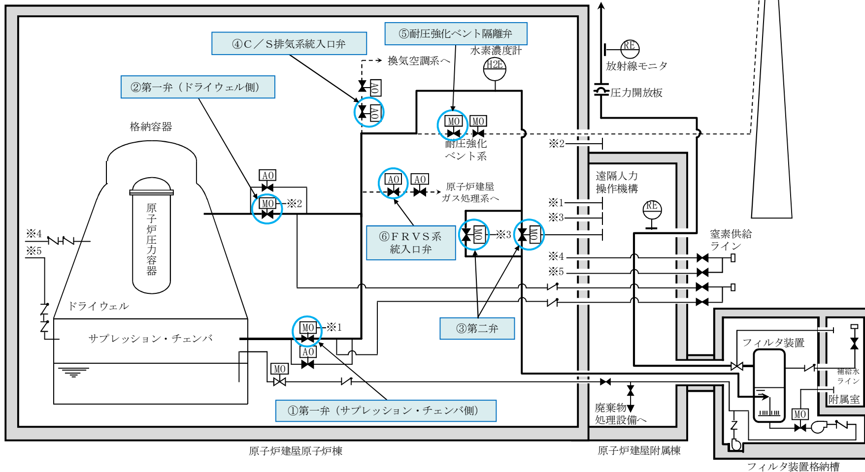
図 4.1.3-1 格納容器フィルタベント系の系統概要図(操作対象箇所)
