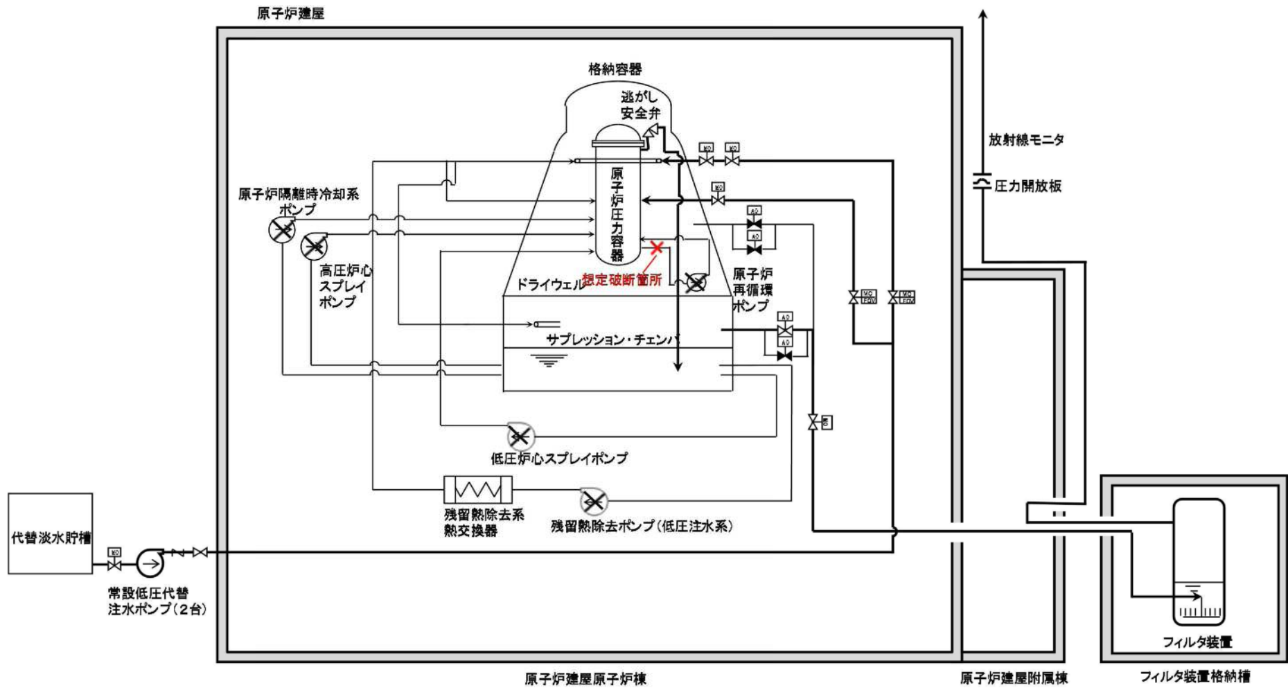
図 4. 1. 2-2 「雰囲気圧力・温度による静的負荷（格納容器過圧・過温破損）（循環冷却を使用しない場合）」 における系統概要図
