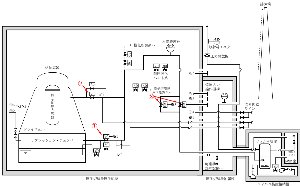
第 4.4-1 図 格納容器フィルタベント系機能検査対象弁
