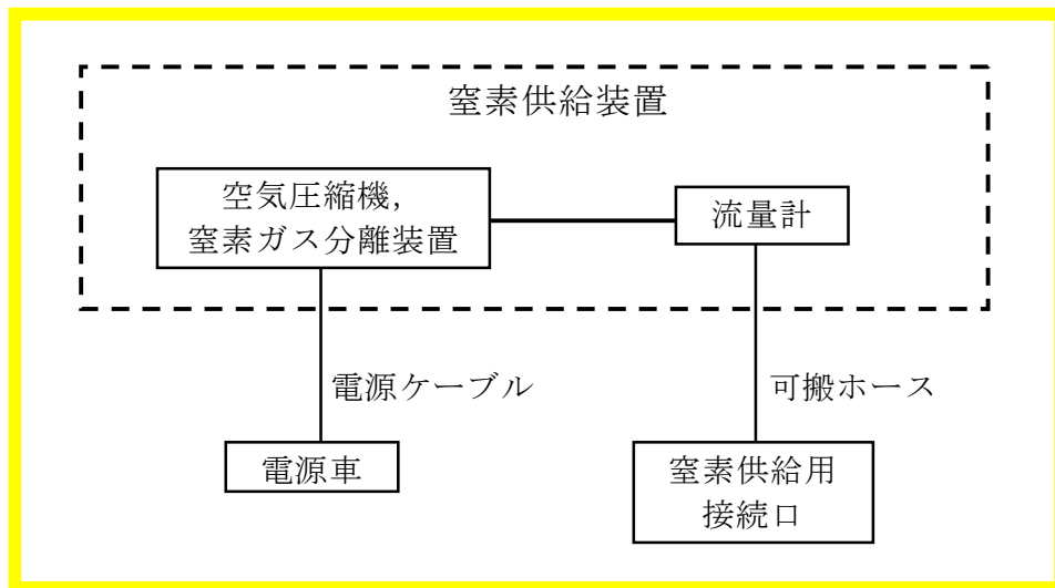
第 2.4.4-2 図 窒素供給装置構成概略
