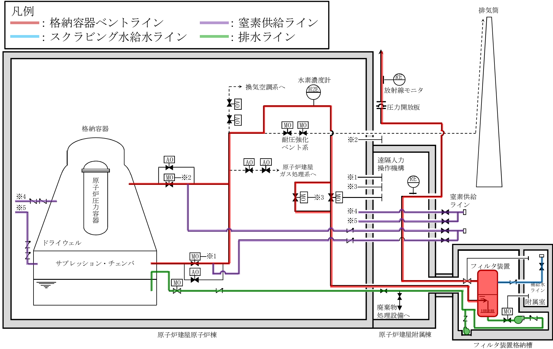
第 2.3.1-1 図 格納容器フィルタベント系 系統概要図
