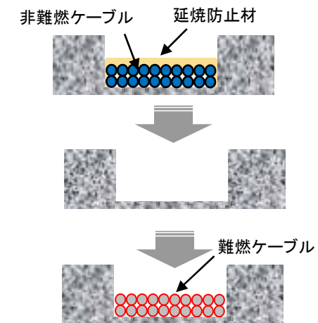
【ピットのケーブル取替イメージ】
