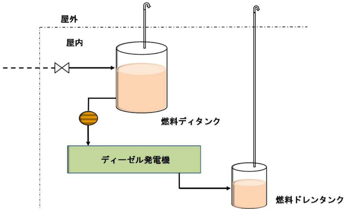
第1-32図 油タンクのベント管設置の例
