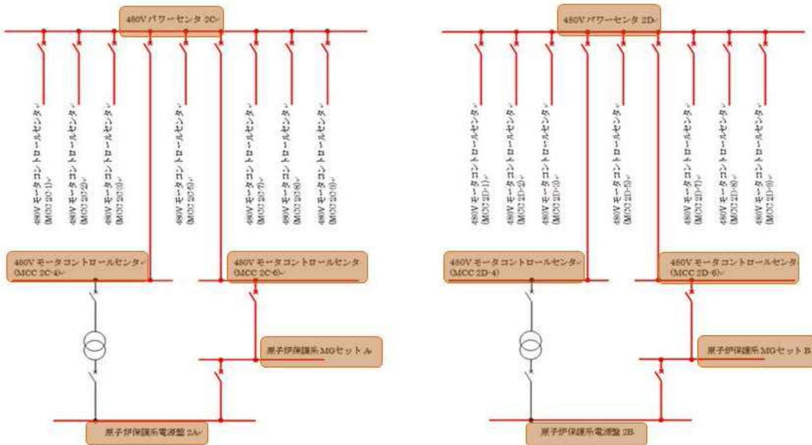
第 12 図 非常用電源系 (MCC (2C, 2D))
