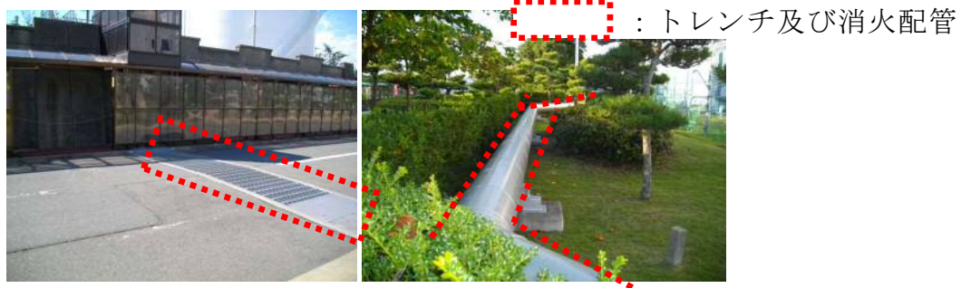
第1-30図 消火配管地下トレンチ,地上化状況
