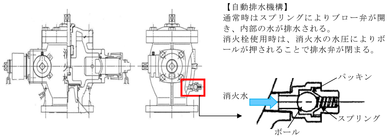
第1-25図 屋外消火栓の構造概要
