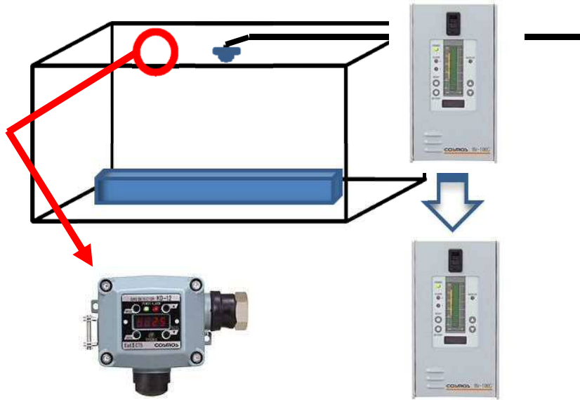
第 1-5 図 水素濃度検知設備の例
