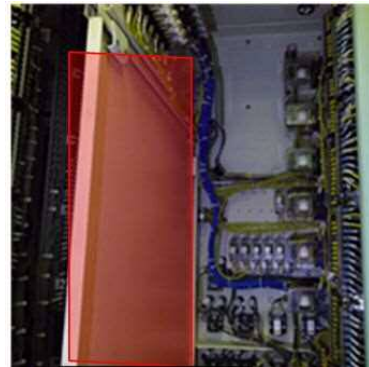
金属製バリア：厚さ 3.2mm 以上 (約 4mm)
