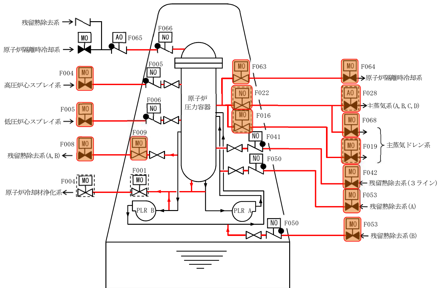
第 1 図 原子炉冷却材圧力バウンダリ
