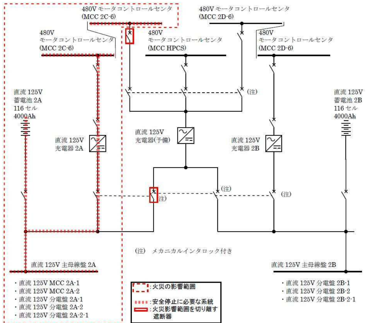
第 6 図 直流電源設備の分離（区分 I の例）
