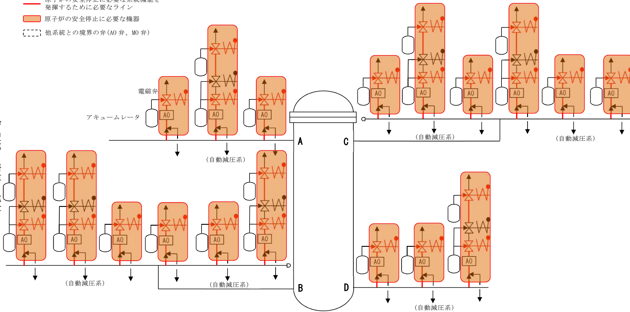
3 図 自動減圧系
