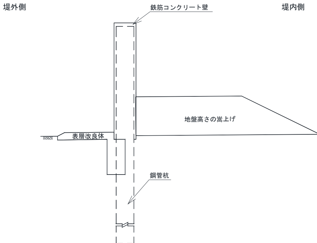
図25 洗掘に係る防止対策
