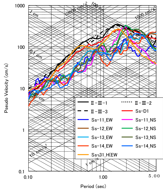
図 3 6 基準地震動 S s と Type II 地震動との比較
