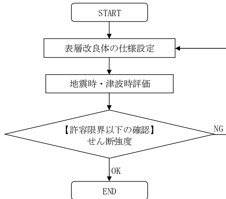
図 2 6 表層改良体の検討フロー
