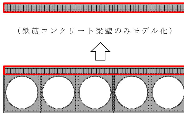
図15 解析モデル概念図
