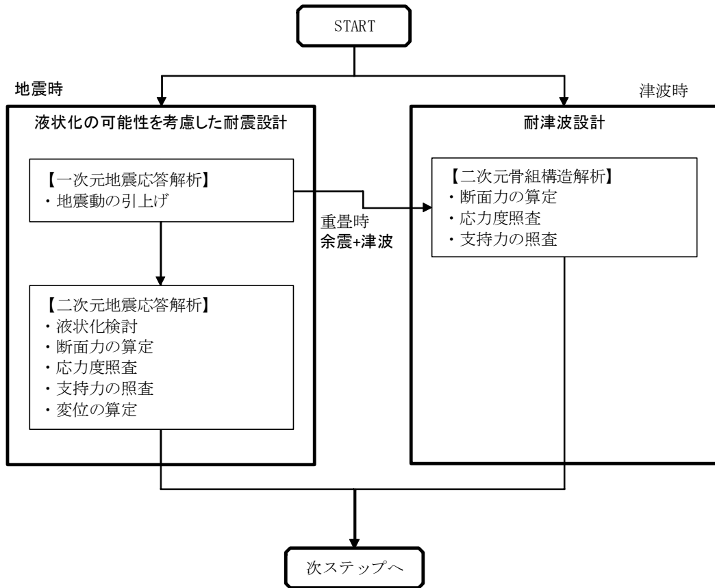
図10 鋼管杭の設計フロー
