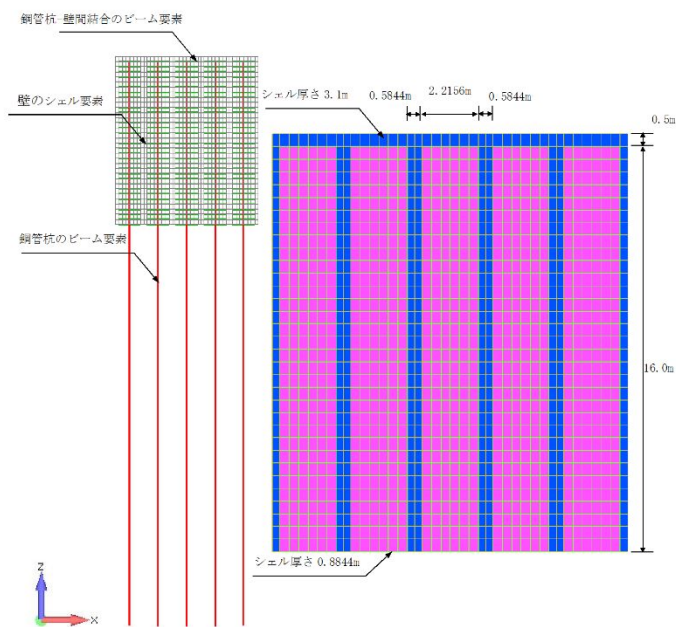
図 1 9 三次元シェルによるモデル化
