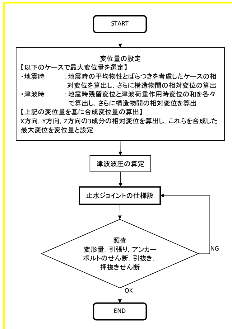
図 2 3 止水ジョイント部の設計フロー
