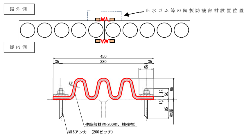
図22 止水ジョイント部の概念図
