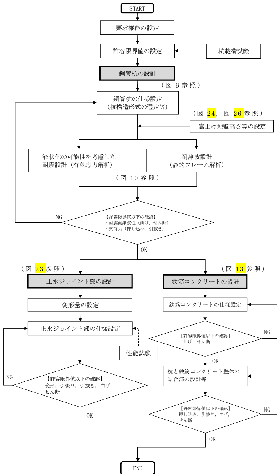
図 4 鋼管杭鉄筋コンクリート防潮壁の構造健全性評価の検討フロー
