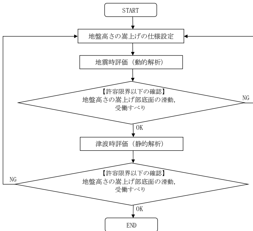
図24 地盤高さの嵩上げの検討フロー
