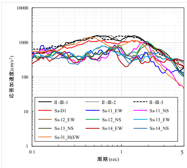
図 3 6 基準地震動 S s と Type II 地震動との比較
