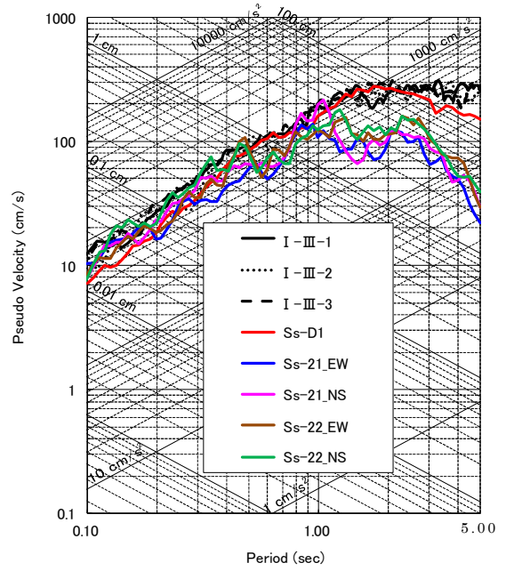
図 3 5 基準地震動 S s と Type I 地震動との比較
