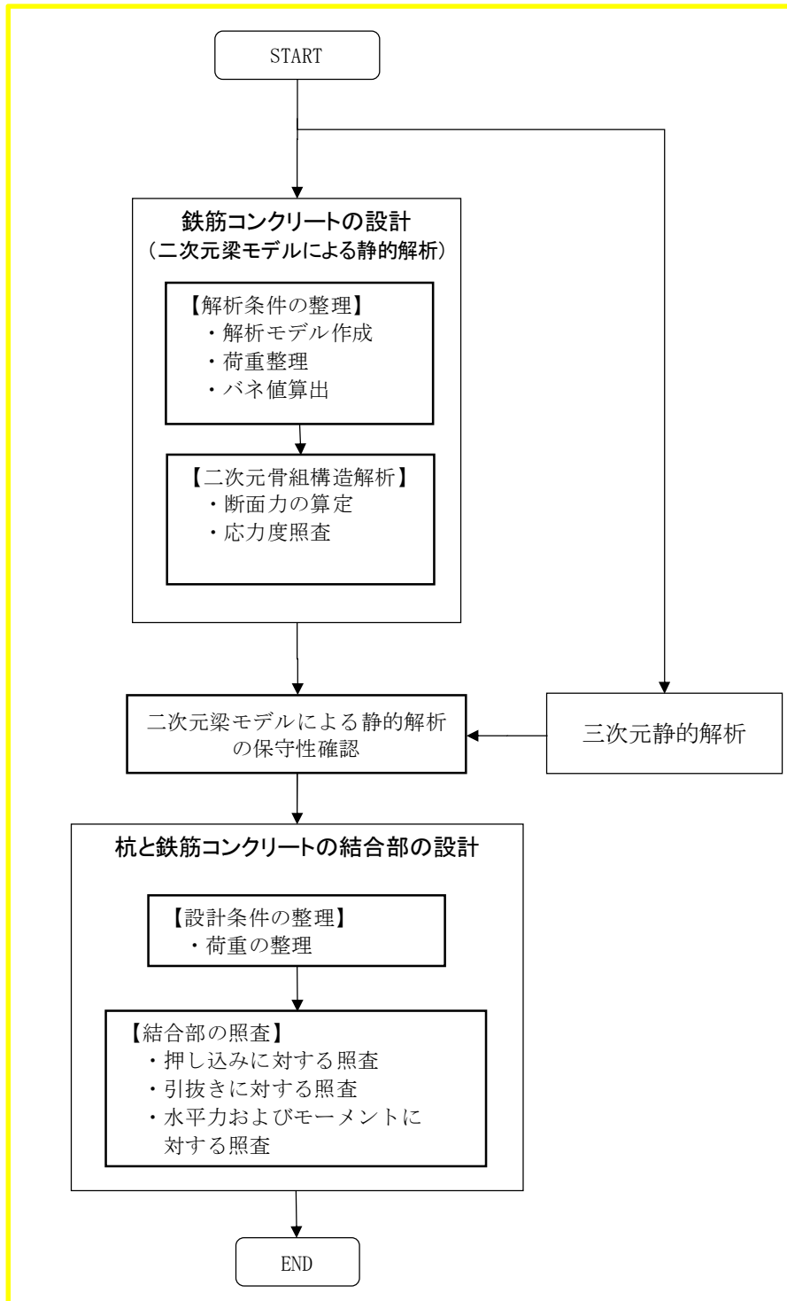
図 1 3 上部工の設計フロー
