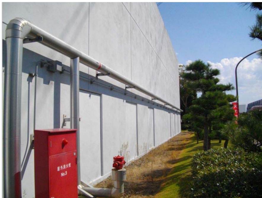
第1-36図 屋外消火配管への保温材設置状況
