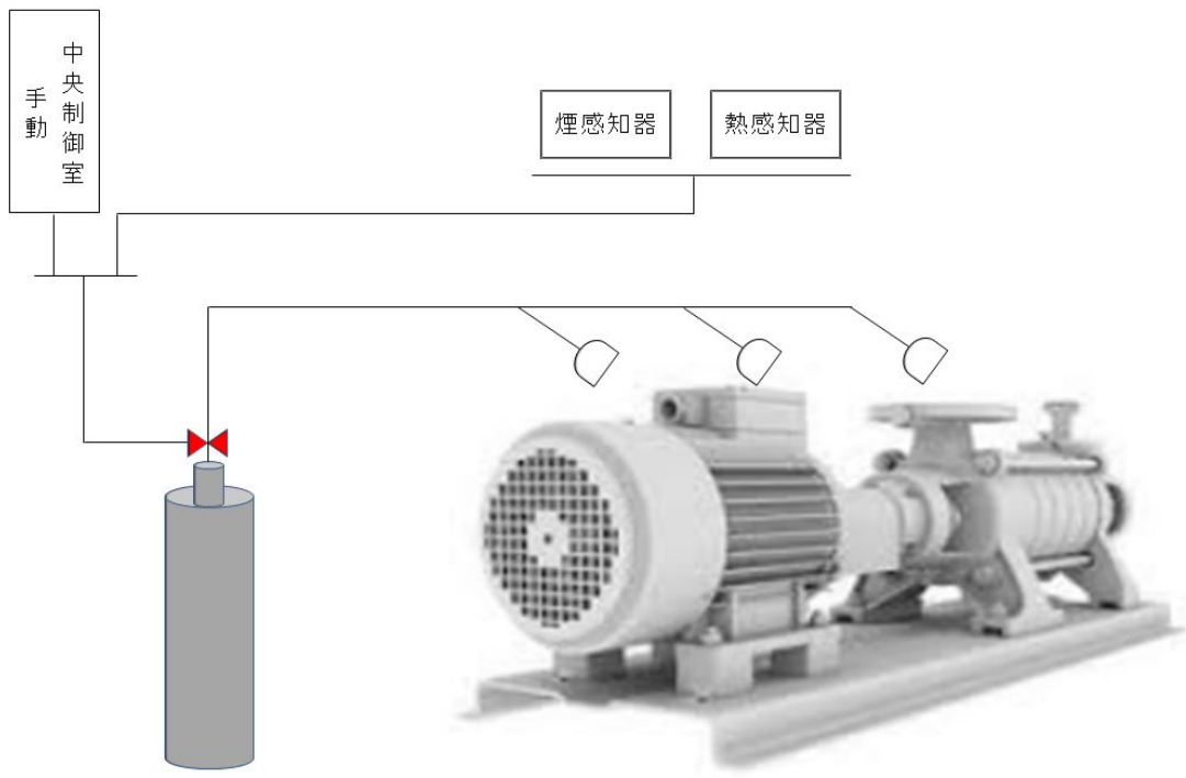
油内包機器に対する消火設備の例
