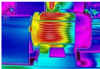
第2図 熱感知カメラ画像イメージ
