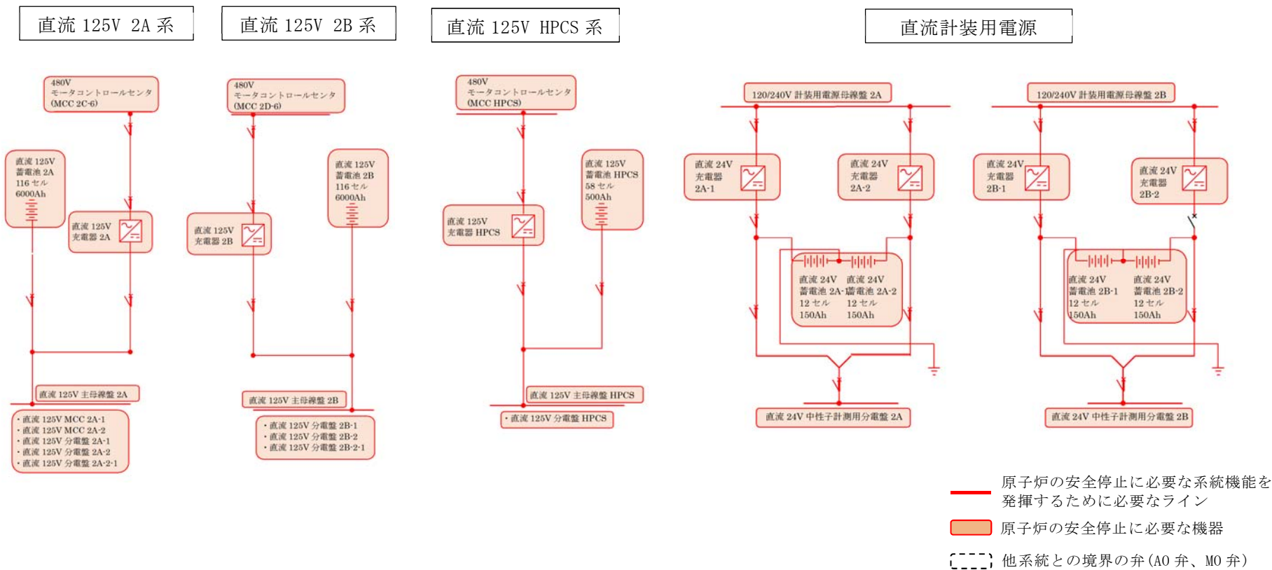
第 13 図 非常用電源系(直流電源系)
