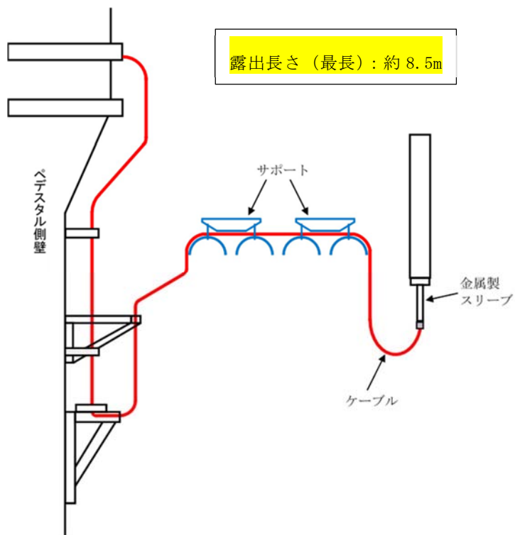
第 8-10 図 原子炉压力容器下部の核計装ケーブルの敷設概要
