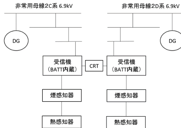
第 1-19 図 火災感知設備の電源確保の概要
