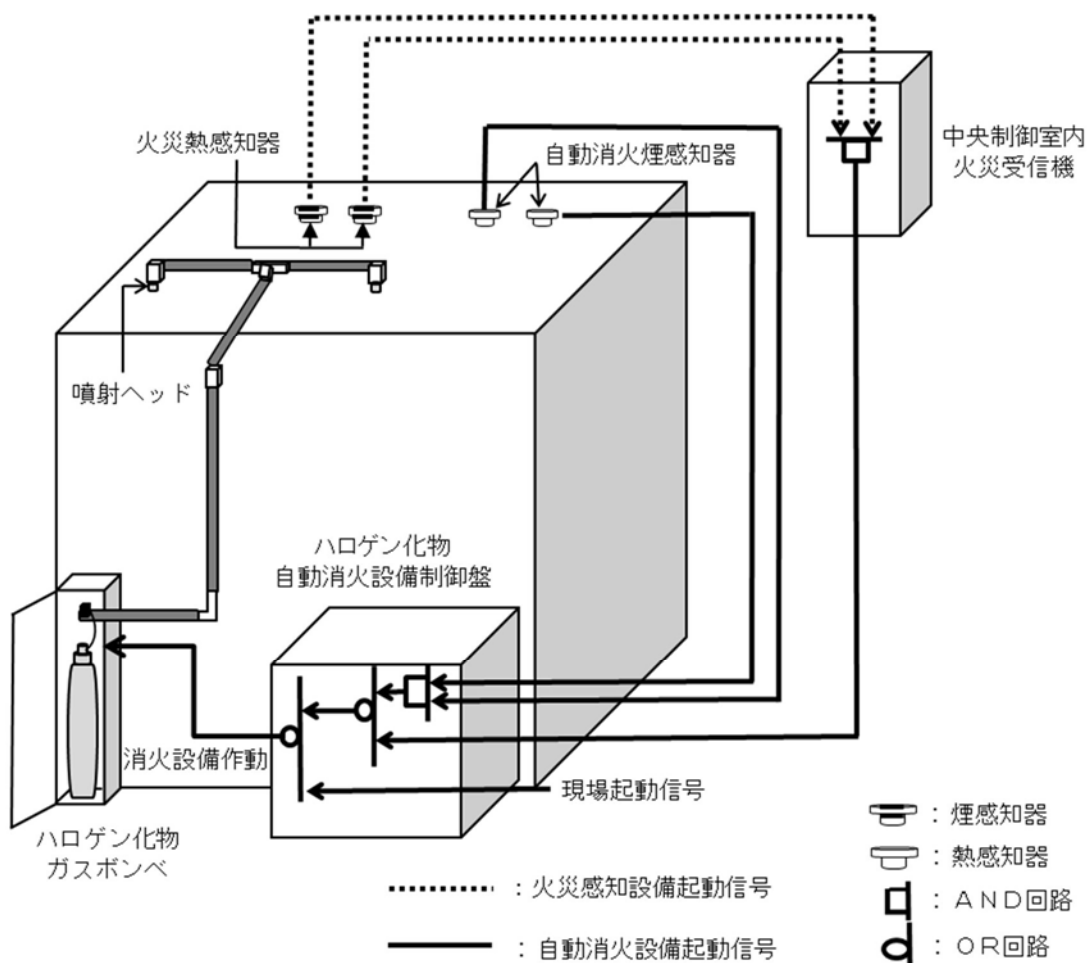
第1-20図 ハロゲン化物消火設備概要図
