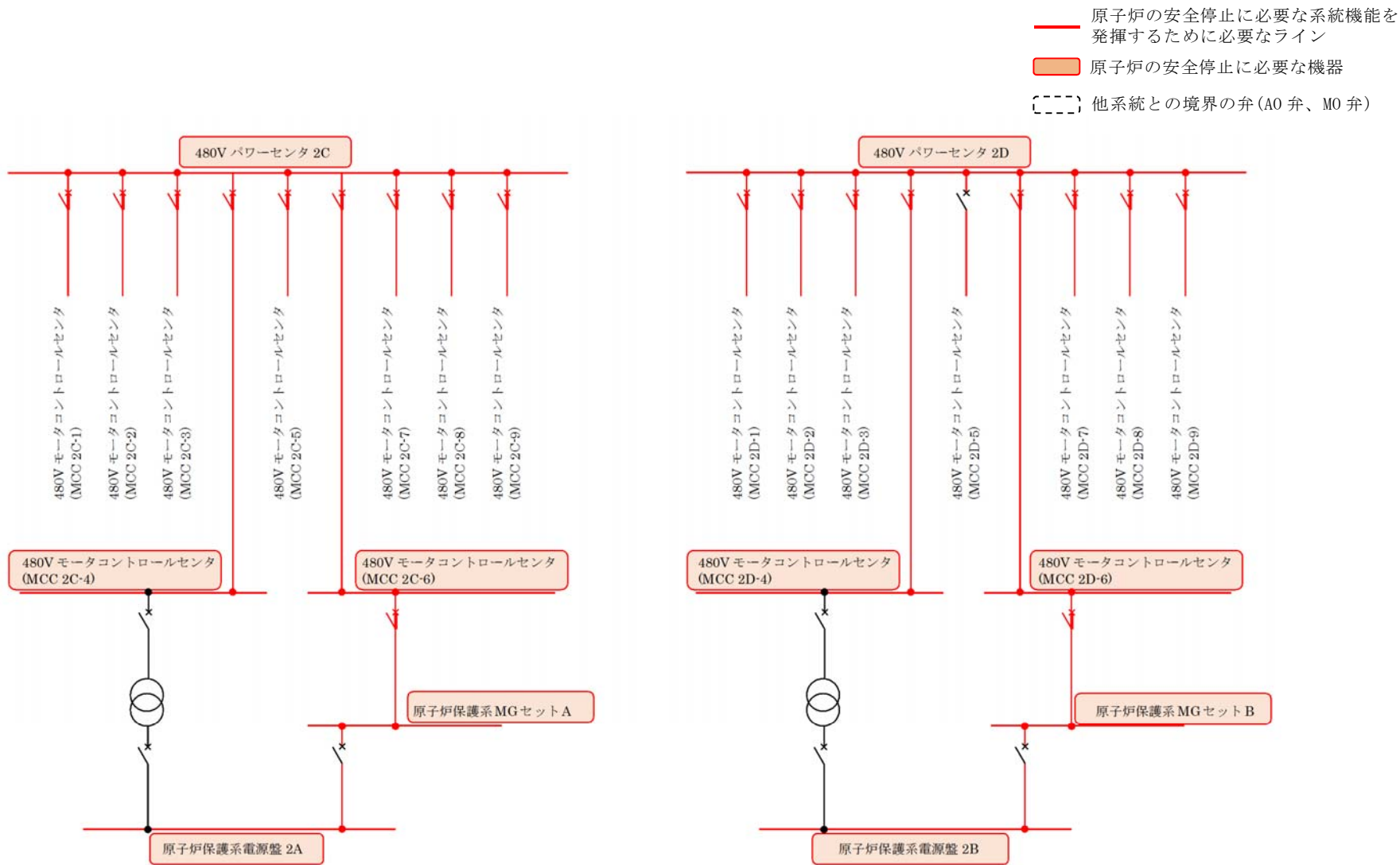
第 12 図 非常用電源系 (MCC (2C, 2D))
