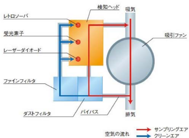
第1図 煙検知のセンサの構成
