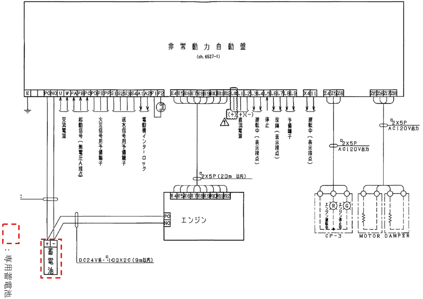
第 1-30 図 デイゼル駆動消火ポンプ結線図
