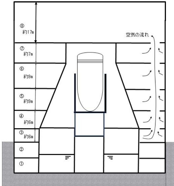
第1図 原子炉建屋断面図
