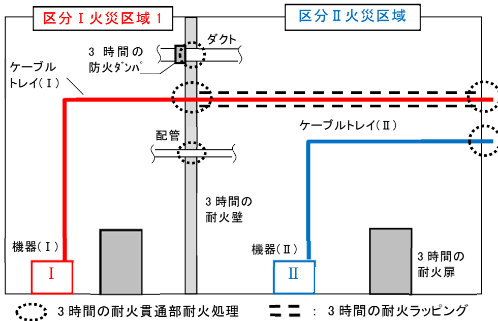
第7-2図 ケーブルラッピングによる系統分離概要
