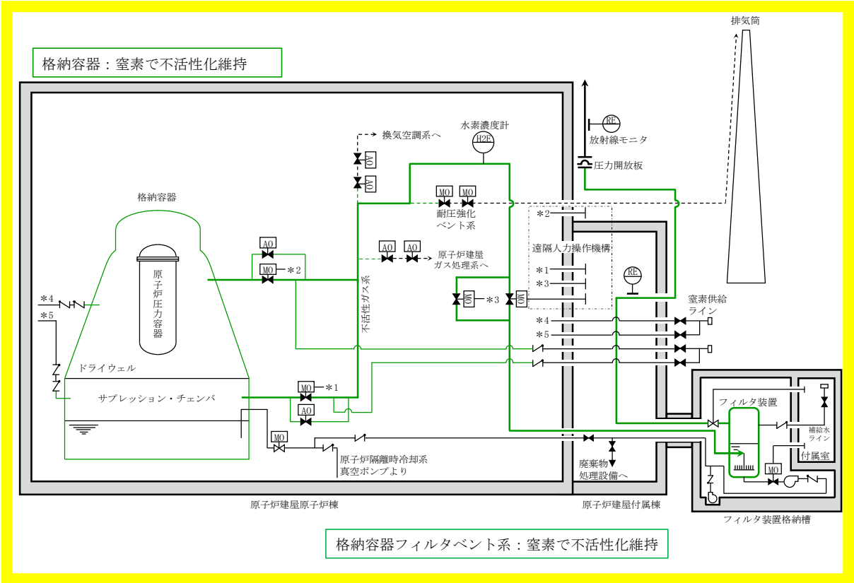
第 1 図 系統待機時の状態概要図
