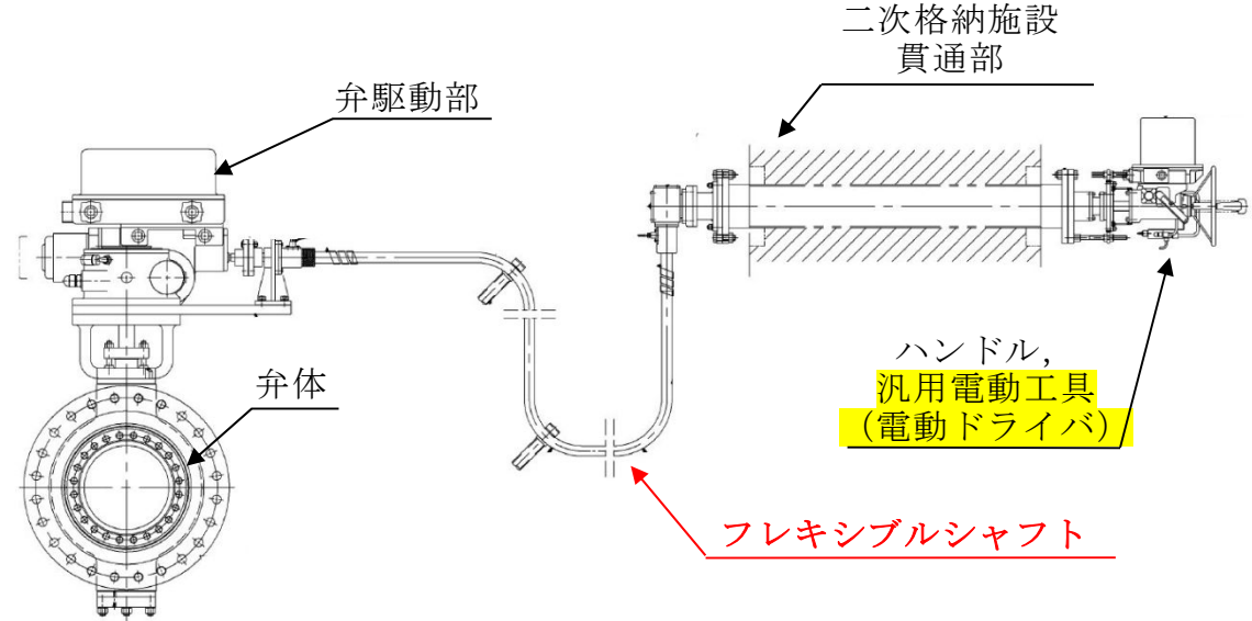
第 4 図 遠隔人力操作機構の模式図
