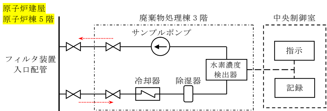
第 6 図 フィルタ装置入口水素濃度 システム概要図
