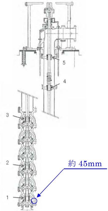
図4 残留熱除去系海水系ポンプ断面図
