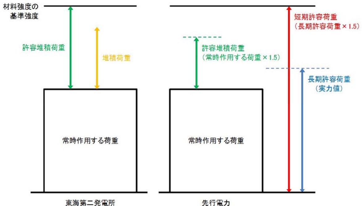
図 1 許容堆積荷重の考え方 イメージ図
