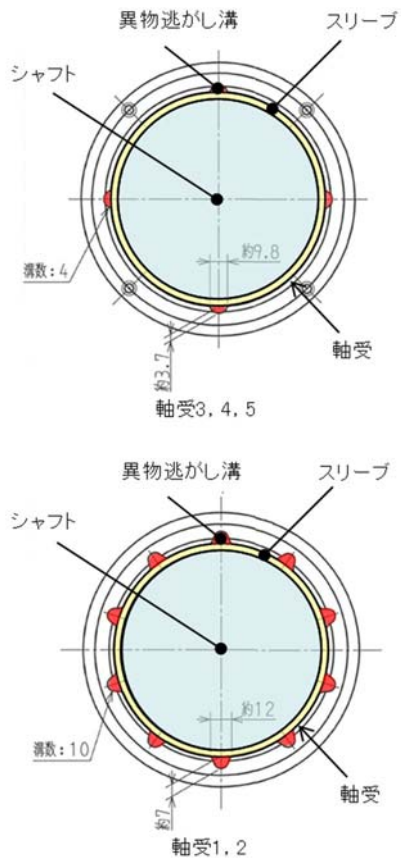
図3 残留熱除去系海水系ポンプ軸受部
