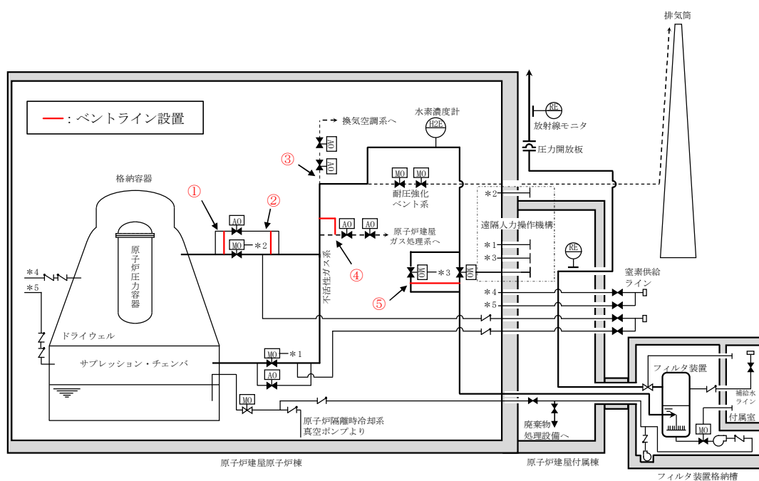
第 4 図 ベントライン設置概要図
