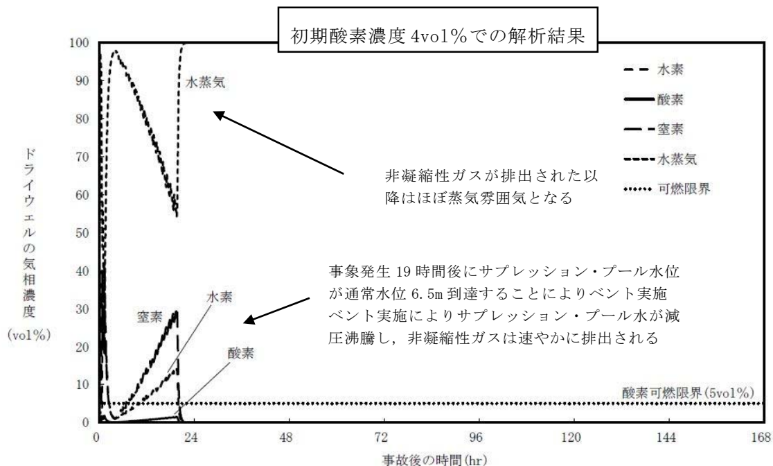
第 7 図 「雰囲気圧力・温度による静的負荷（格納容器過圧・過温破損） （代替循環冷却系を使用しない場合）」における ドライウエルの気相濃度の推移（ウェット条件）
