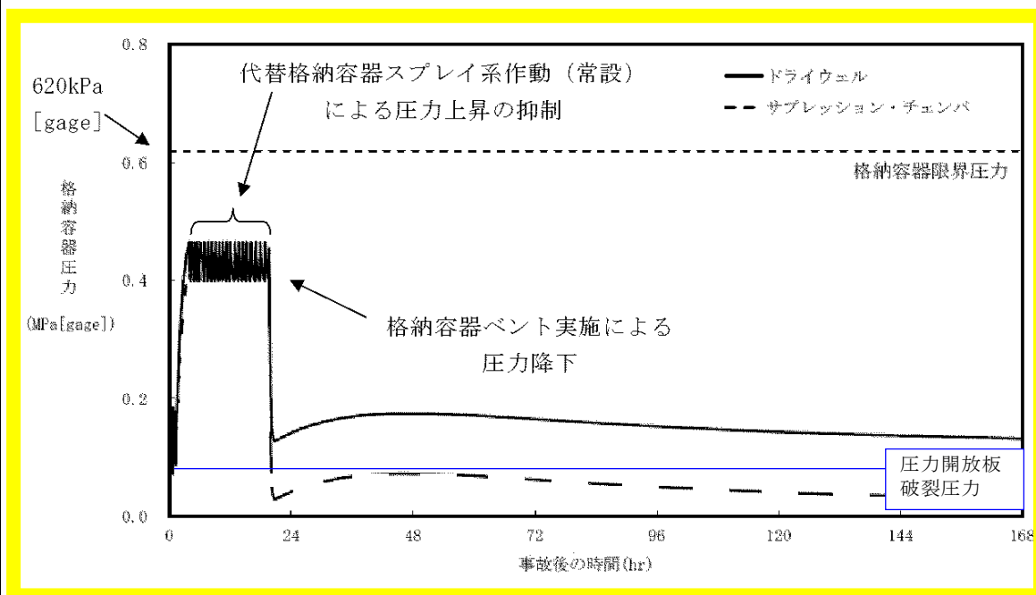
第 50-6-3 図 「雰囲気圧力・温度による静的負荷（格納容器過圧・過温破損）（代替循環冷却を使用しない場合）」における格納容器圧力の推移と圧力開放板の関係
