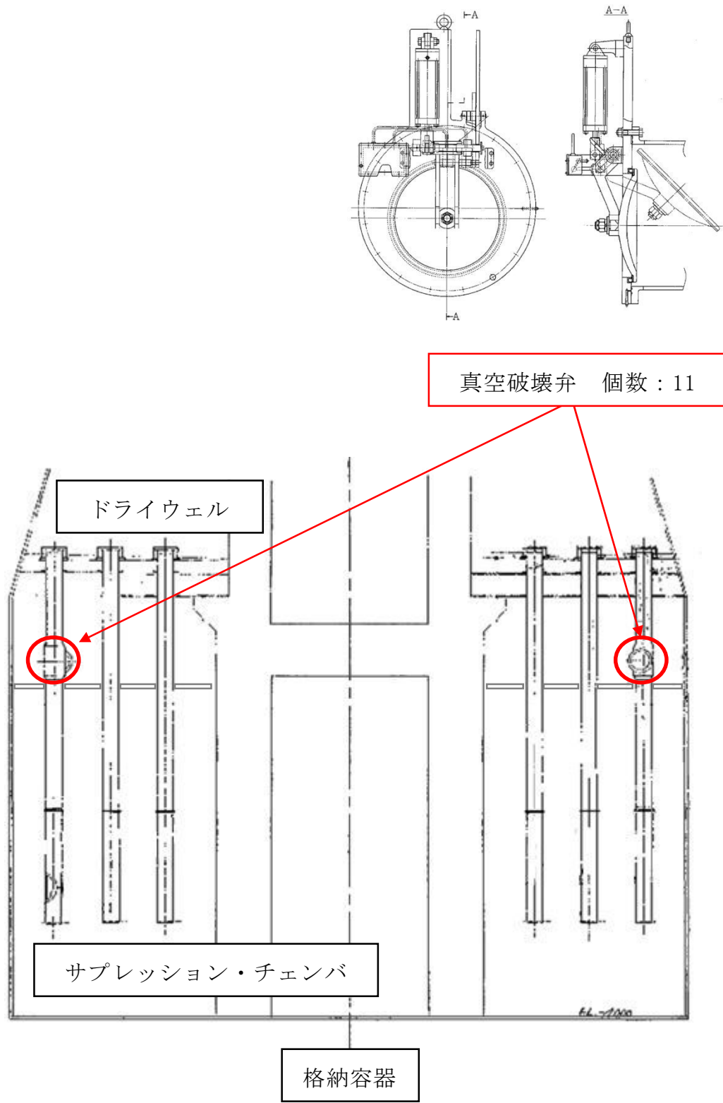
第 50-3-5 図 真空破壊弁設置場所
