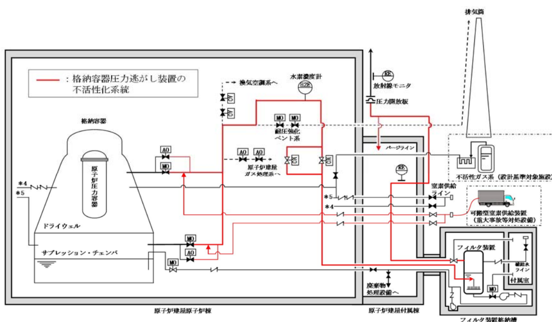
第 1 図 格納容器圧力逃がし装置の不活性化系統
