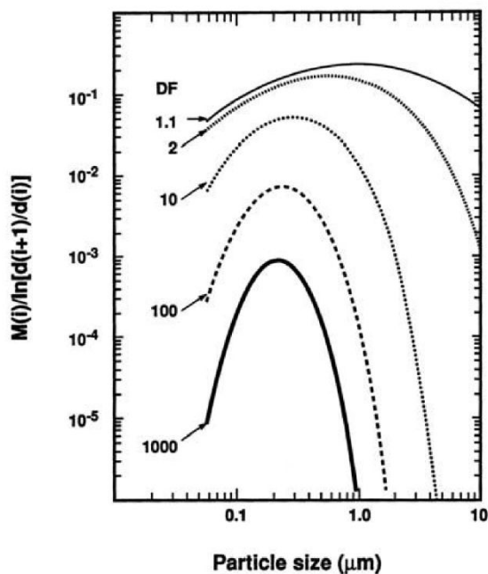
第 6 図 格納容器スプレイを継続することによる格納容器内のエアロゾル粒径分布の変化（参考図書 1）
