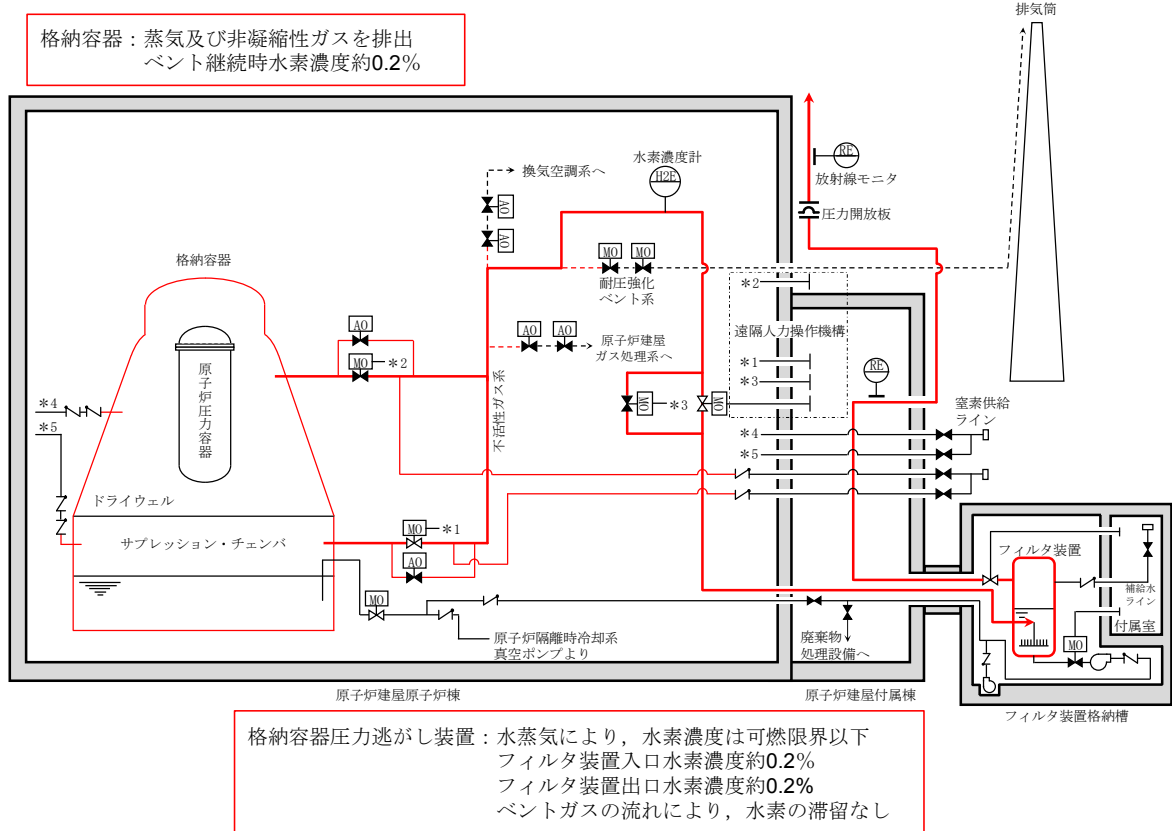
第2図 ベント実施時状態概要図
