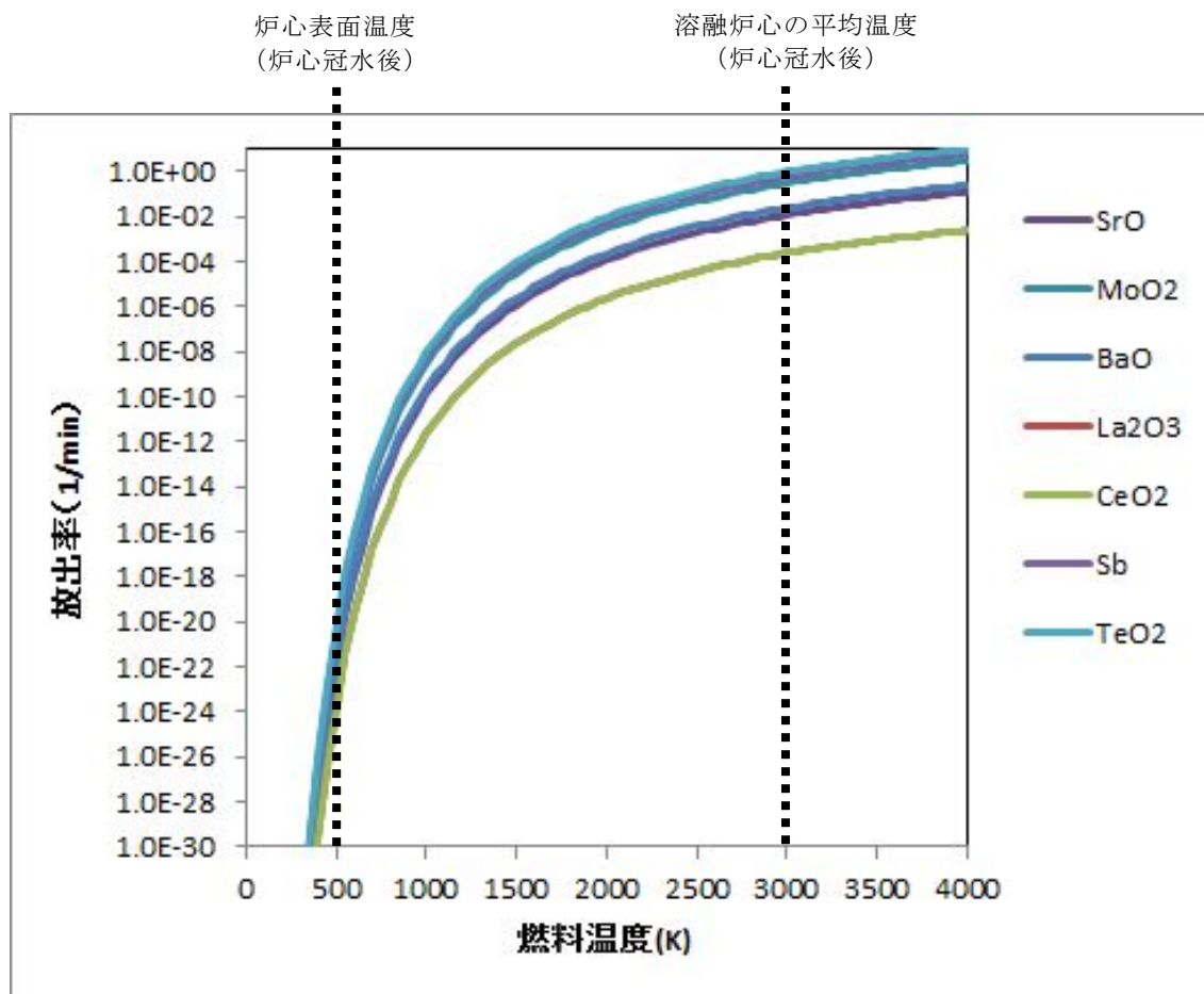
第2図 炉心の温度及び放射性物質の放出率（中・低揮発性核種）
