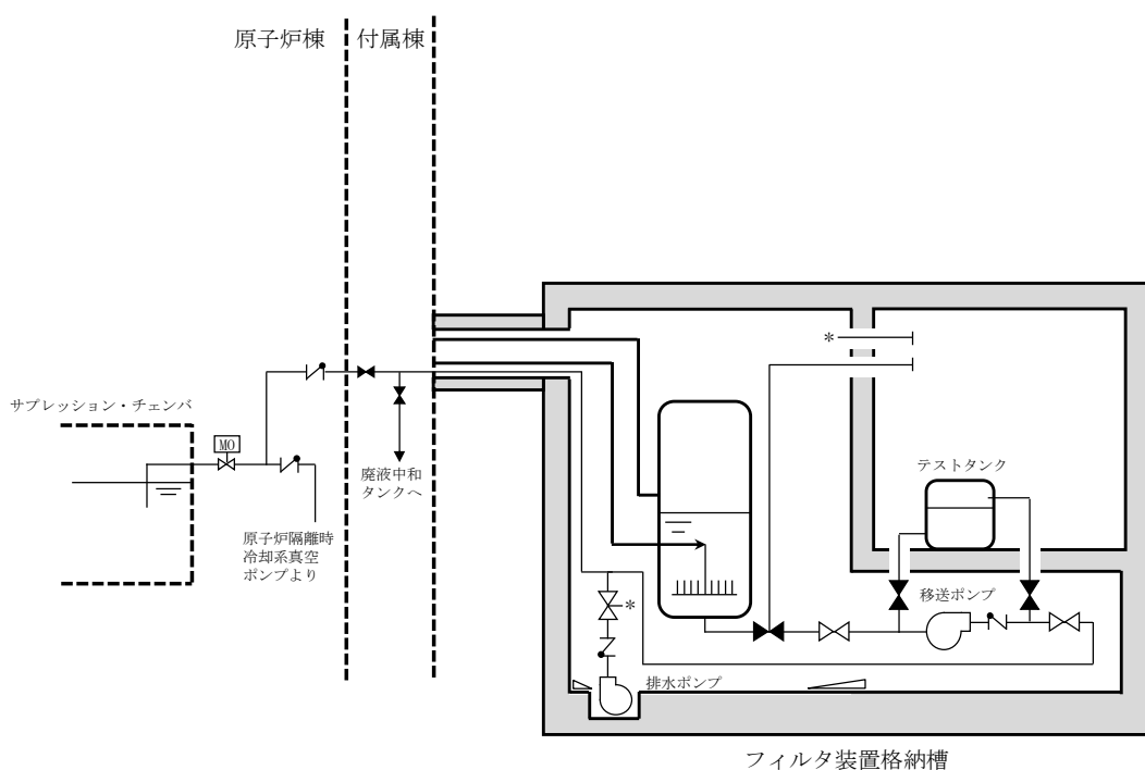
第 1 図 排水設備の構成
