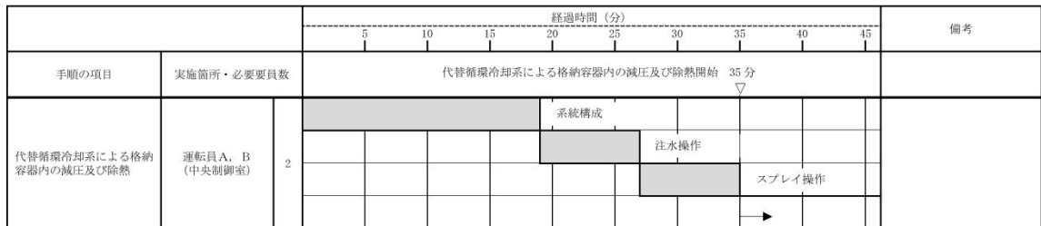
第 3.7-3 図 代替循環冷却系 タイムチャート*
