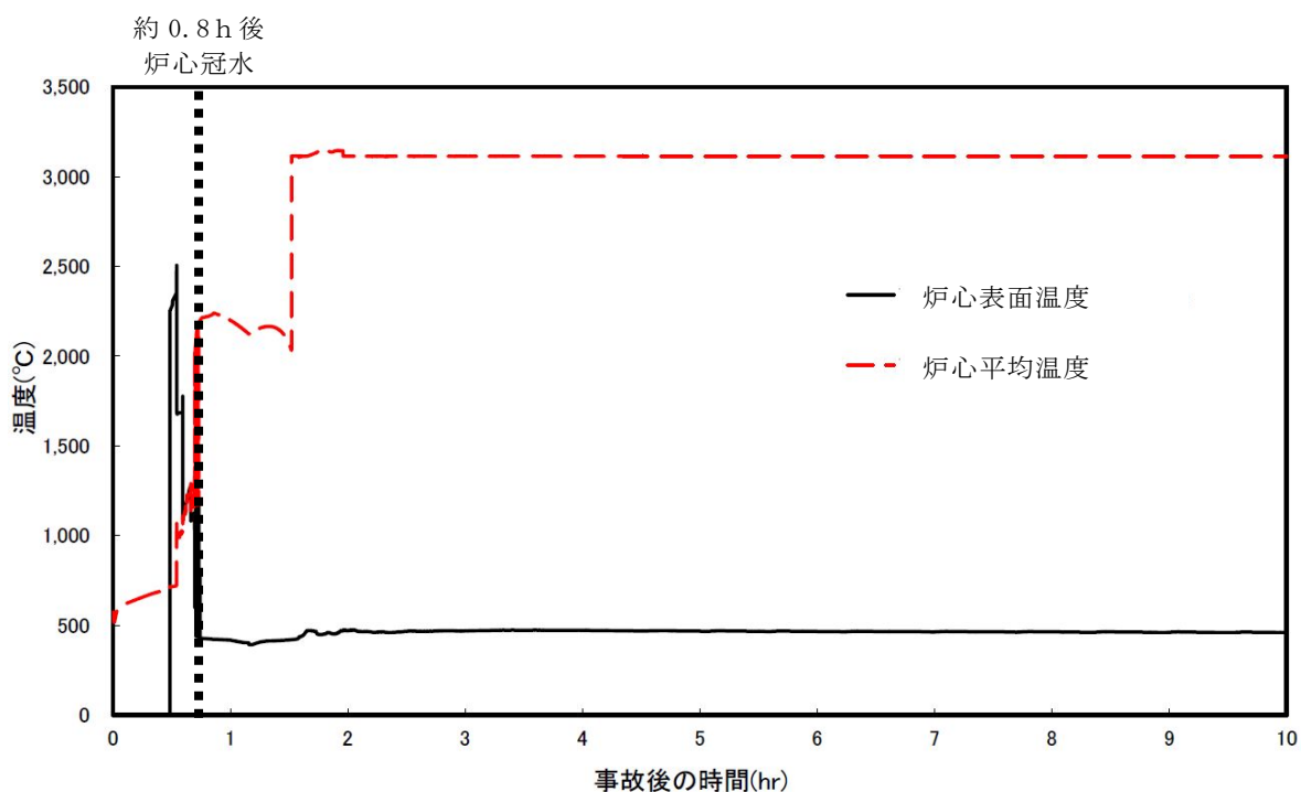
第1図 事故初期における溶融炉心の平均温度及び炉心表面温度
