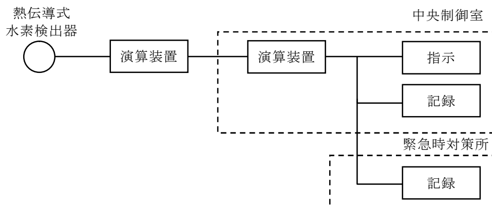
第4図 フィルタ装置入口水素濃度の概略構成図
