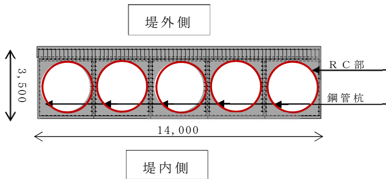
第 1 図 鋼管杭鉄筋コンクリート防潮壁の概要図
