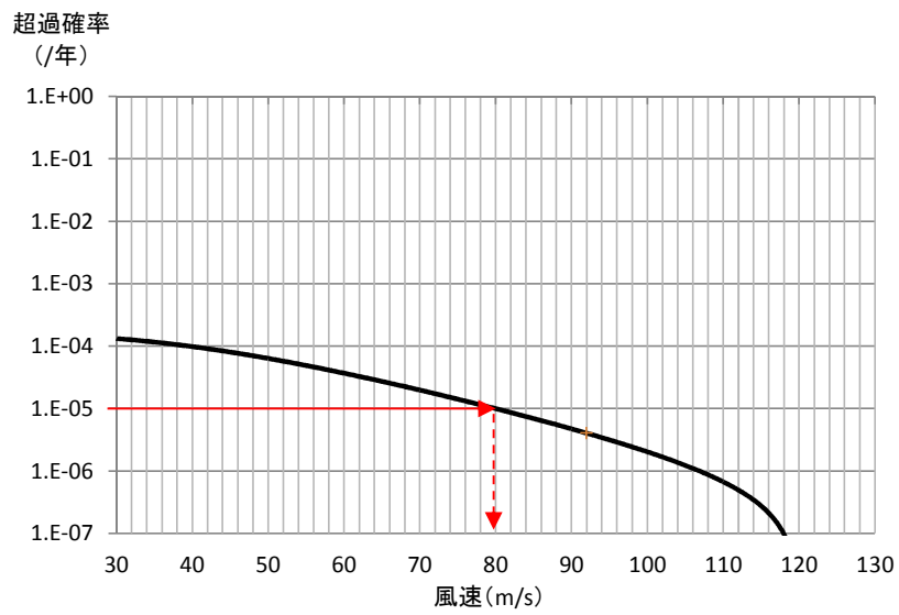
第 8.1-12 図 竜巻最大風速のハザード曲線
