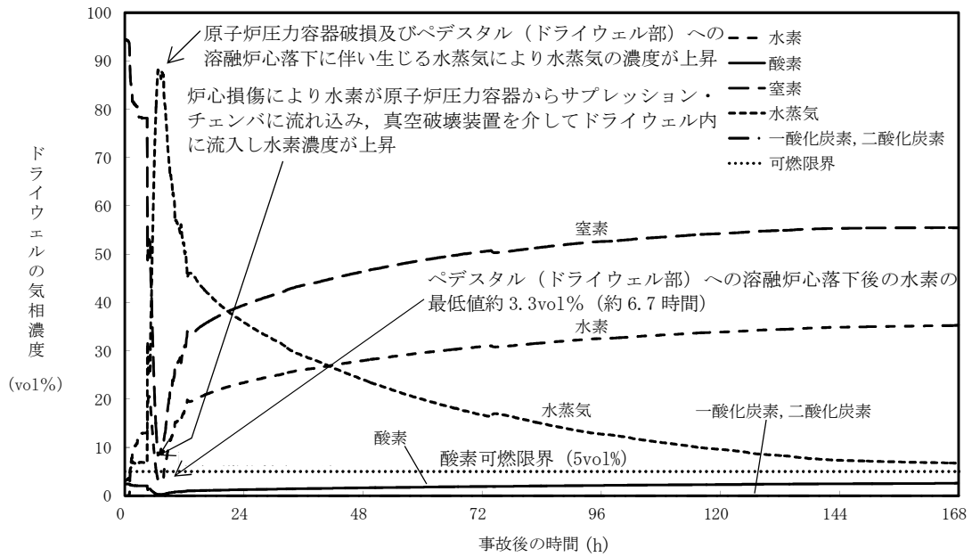
第 3.5-5 図 ドライウエルの気相濃度の推移 (ウェット条件)
