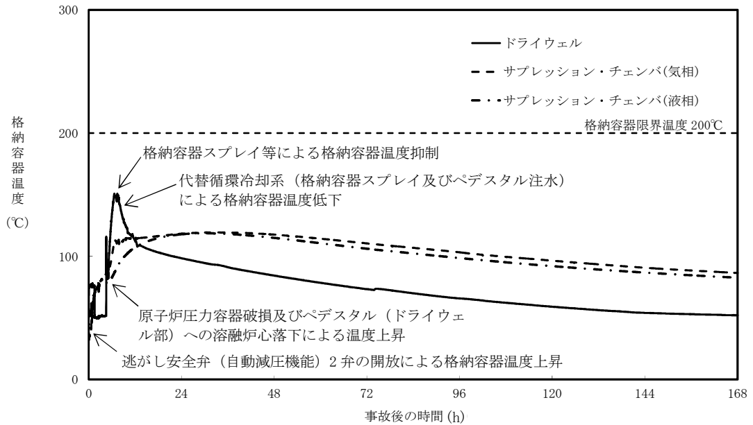
第 3.5-4 図 格納容器雰囲気温度の推移
