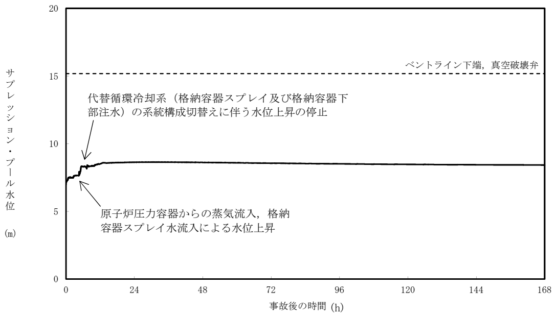
第 3.5-9 図 サプレッション・プール水位の推移
