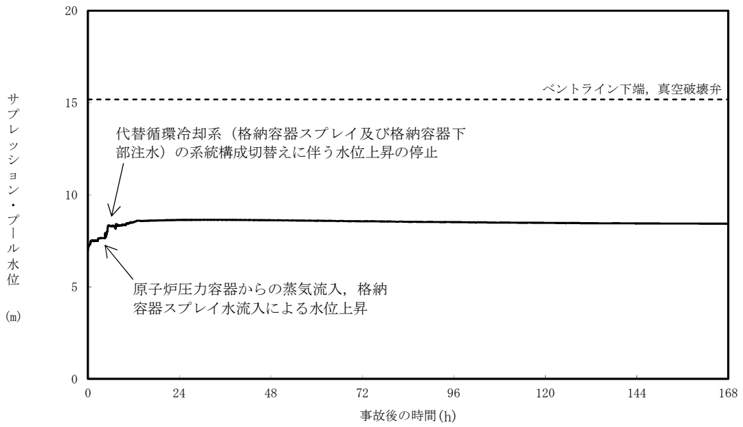
第 3.2-8 図 サプレッション・プール水位の推移
