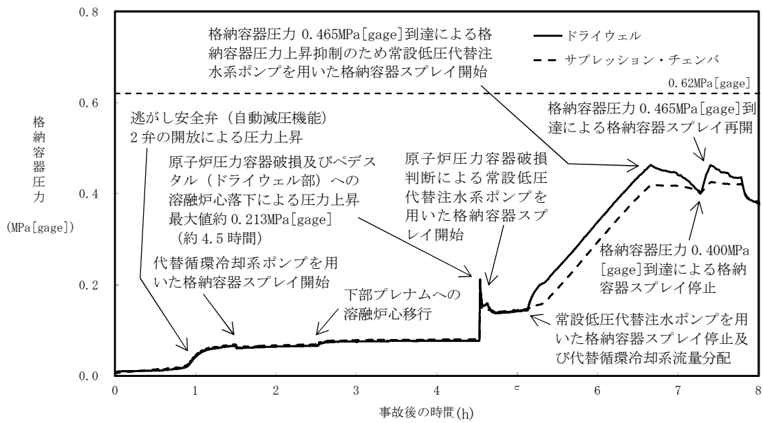
第 3.3-3 図 格納容器圧力の推移
