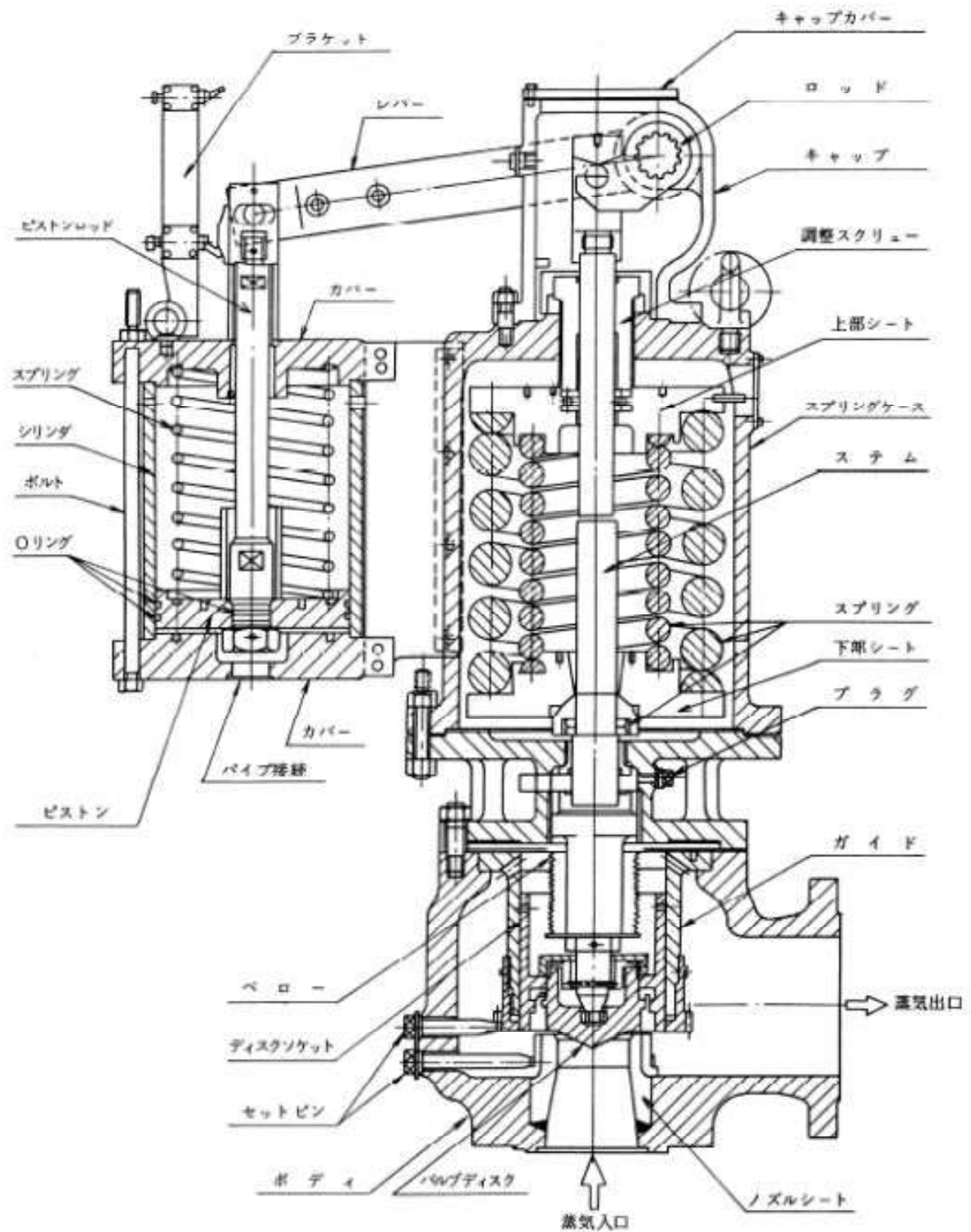
第 1a 図 SRV 構造図 (断面図)
