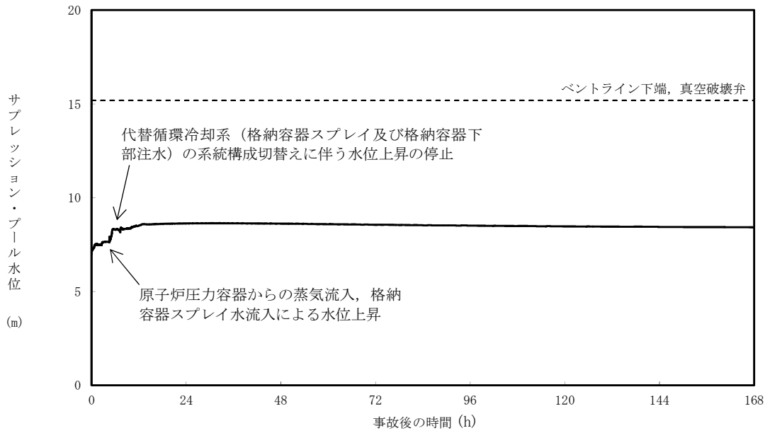
図 3.2-8 サプレッション・プール水位の推移
