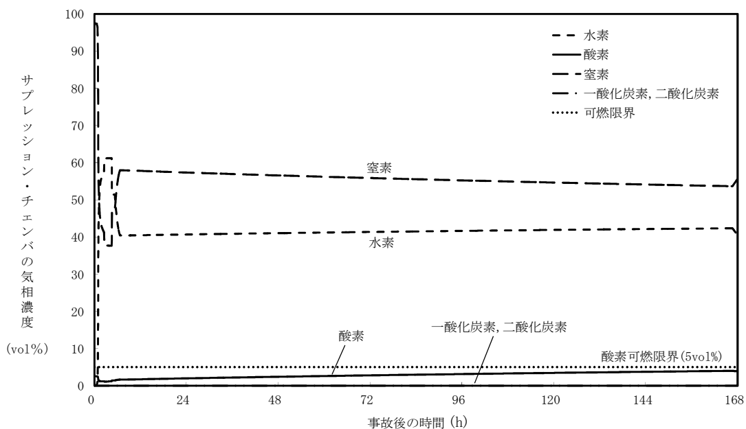
第 3.5-8 図 サプレッション・チェンバの気相濃度の推移 (ドライ条件)
