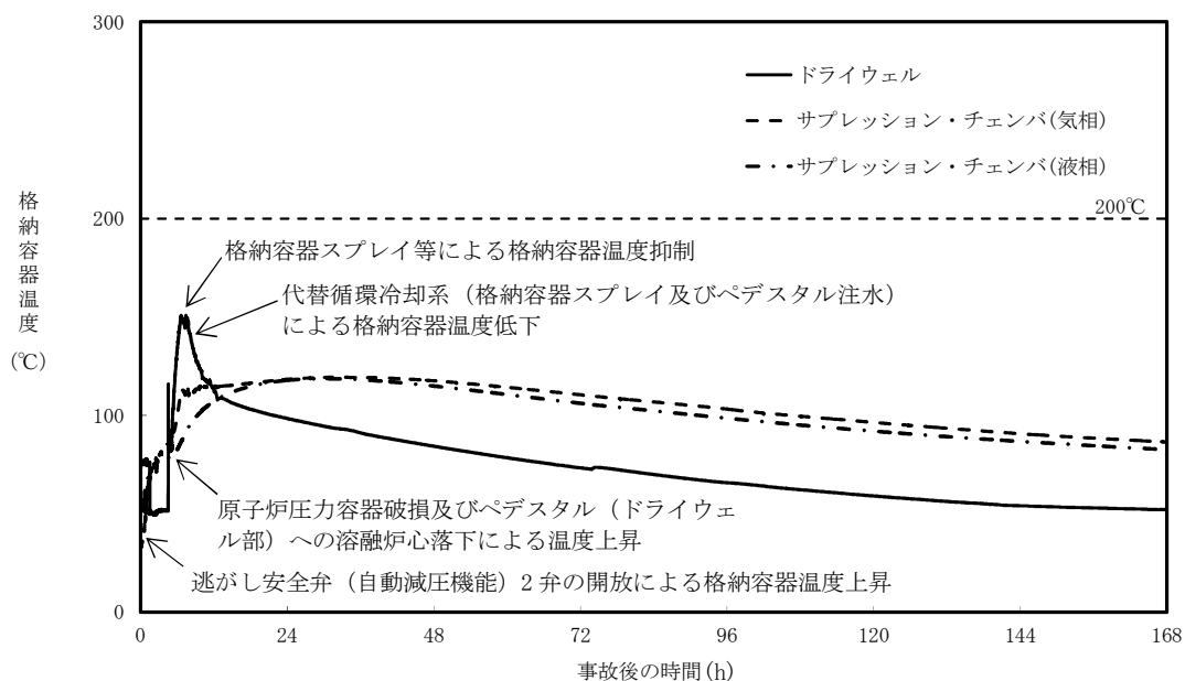
第 3.2-7 図 格納容器雰囲気温度の推移
