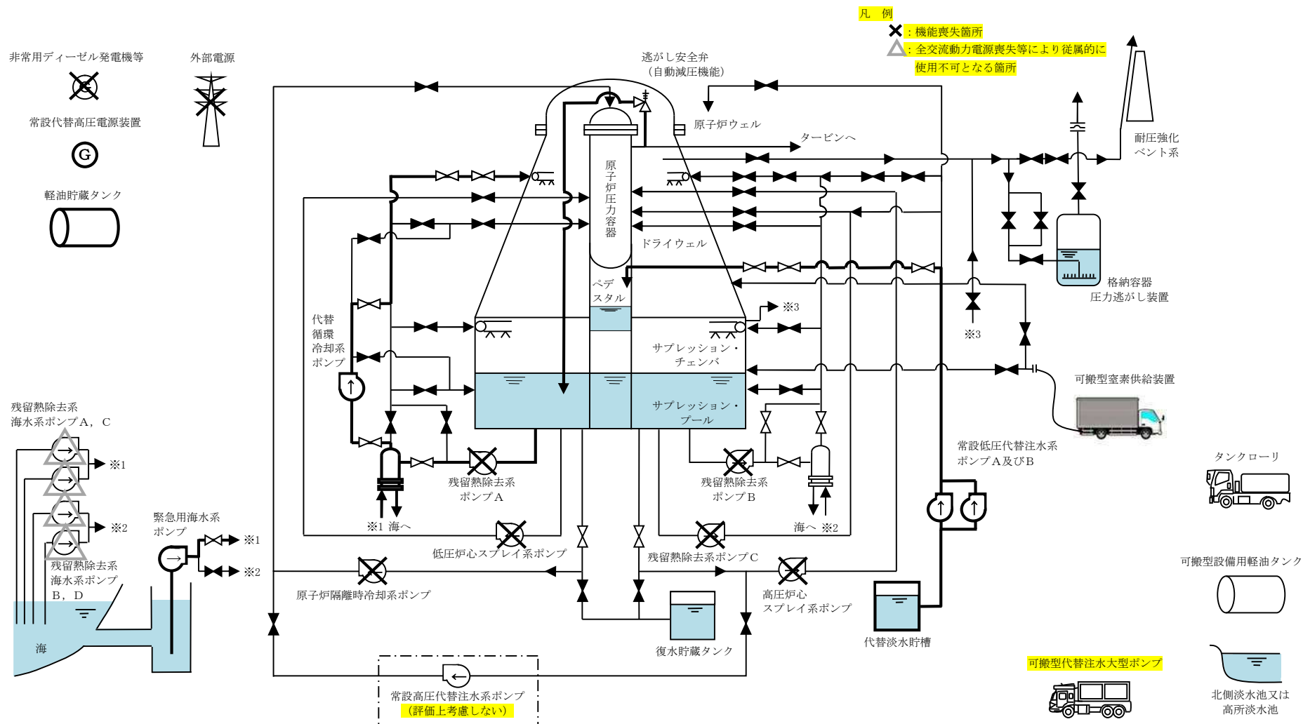
第 3.2-1 図 高压熔融物放出／格納容器雰囲気直接加熱時の重大事故対処設備の概略系統図 (2/4) (原子炉压力容器破損前の代替循環冷却系による格納容器除熱，及び 格納容器下部注水系 (常設) による格納容器下部水位確保段階)
