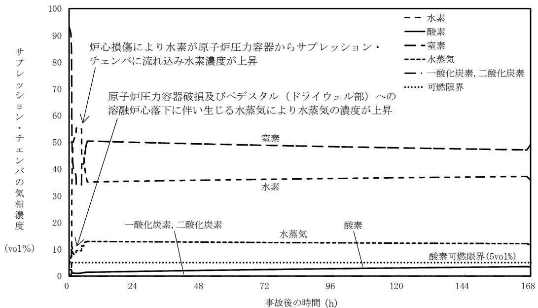
第 3.5-6 図 サプレッション・チェンバの気相濃度の推移 (ウェット条件)
