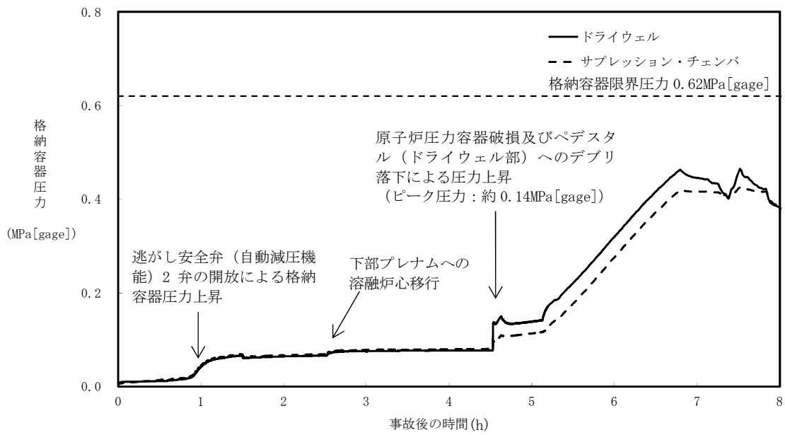
第 3.3-7 図 格納容器圧力の推移 (感度解析ケース (エントレインメント係数最小値) )
