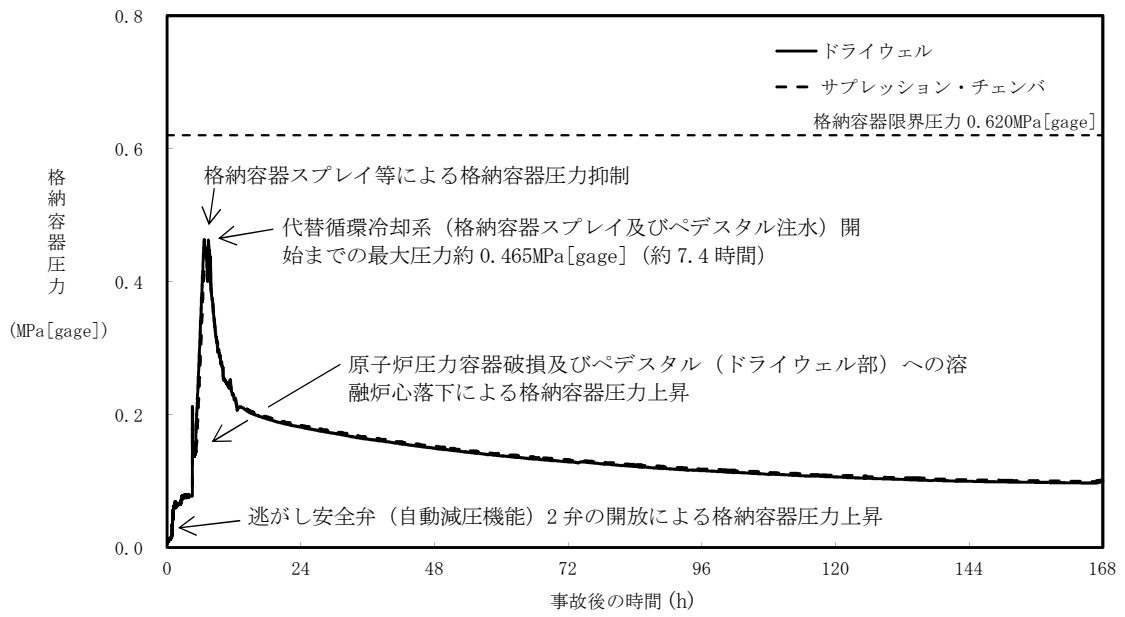
第 3.5-3 図 格納容器圧力の推移
