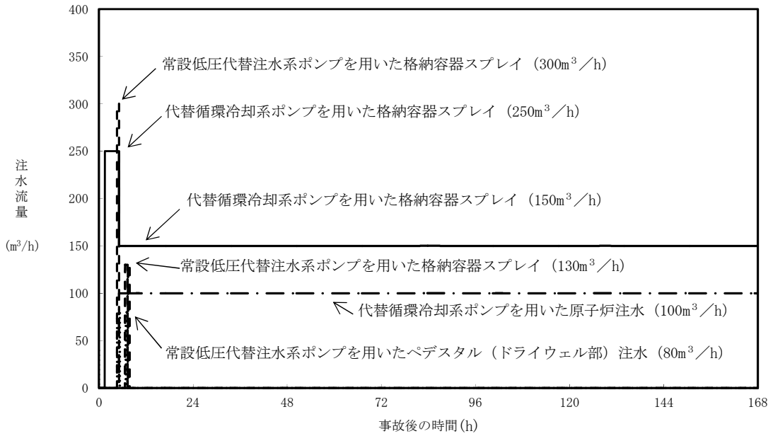
第 3.2-9 図 注水流量の推移
