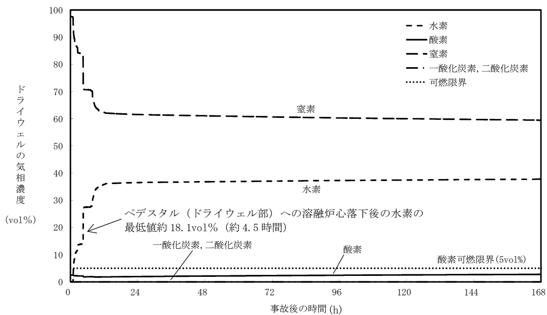
第 3.5-7 図 ドライウエルの気相濃度の推移 (ドライ条件)
