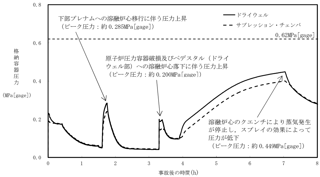
第3.3-9図 格納容器圧力の推移 (感度解析ケース (起因事象をLOCAとした場合) )
