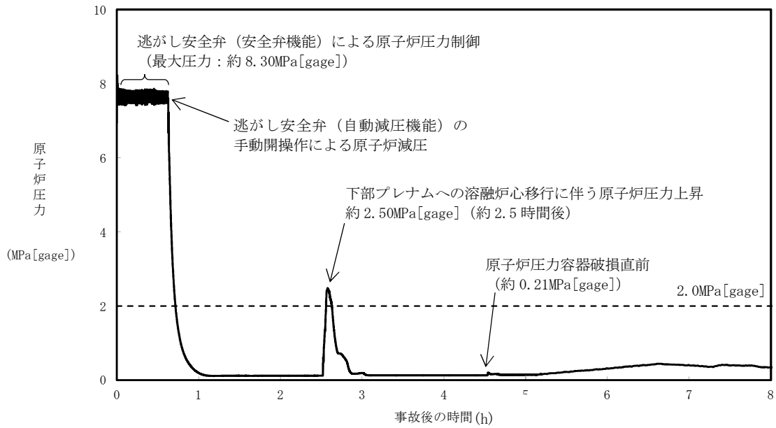
第 3.3-1 図 原子炉圧力の推移
