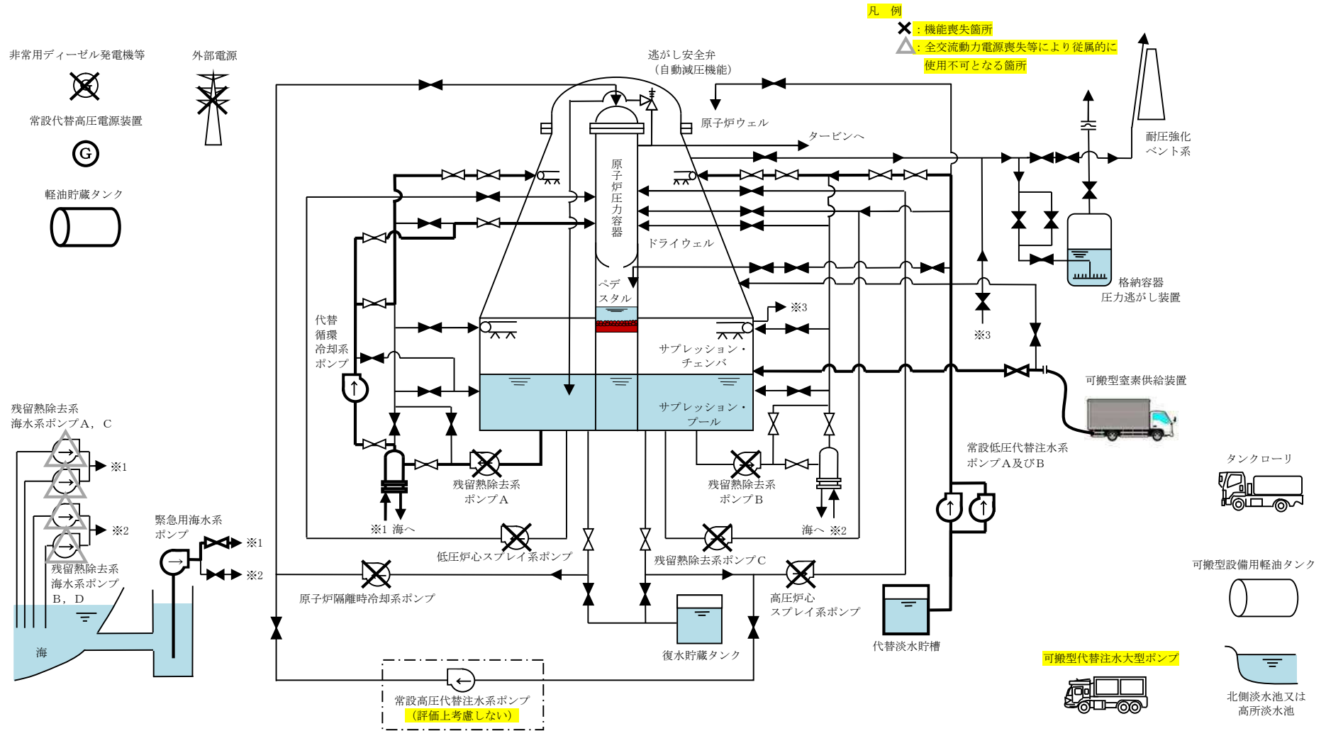
第3.2-1 図 高压熔融物放出／格納容器雰囲気直接加熱時の重大事故事故対処設備の概略系統図(4/4) (原子炉压力容器破損後の代替循環冷却系による原子炉注水及び格納容器除熱， 代替格納容器スプレー冷却系 (常設)による格納容器圧力制御及び可搬型窒素供給装置を用いた格納容器内窒素供給操作段階)
