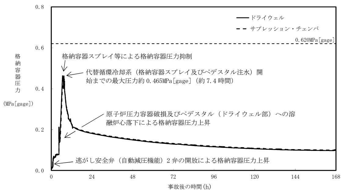
第 3.2-6 図 格納容器圧力の推移
