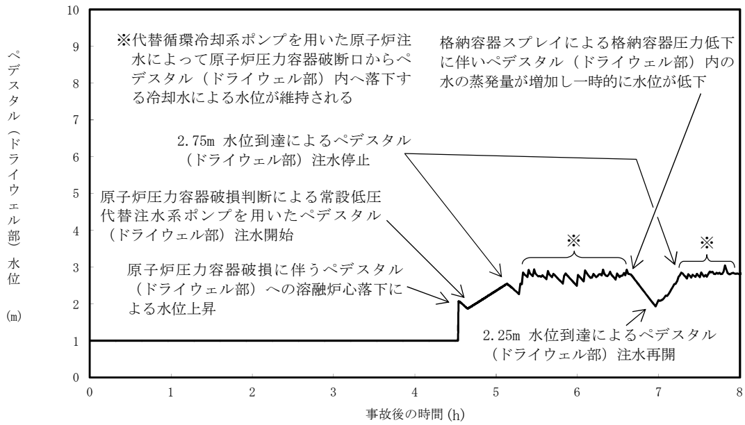
第 3.3-5 図 ペDESTAL (ドライウエル部) の水位の推移
