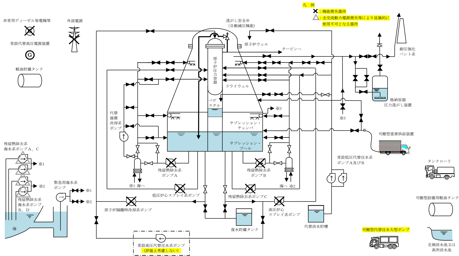
第 3.2-1 図 高圧溶融物放出／格納容器雰囲気直接加熱時の重大事故対処設備の概略系統図 (1/4) (原子炉圧力容器破損前の逃がし安全弁による原子炉減圧段階)
