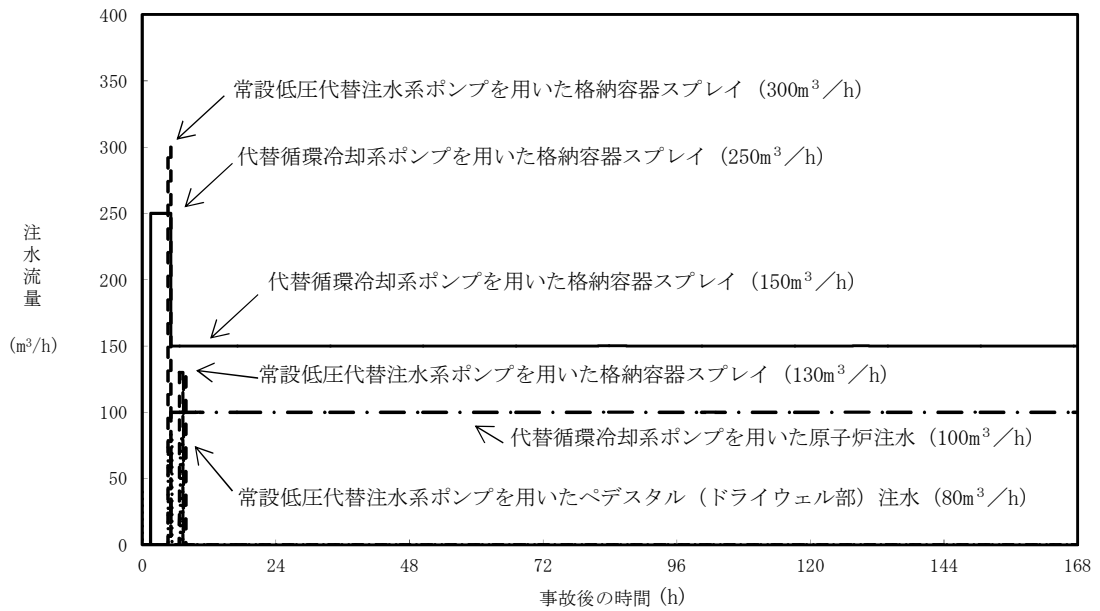
図 3.2-9 注水流量の推移
