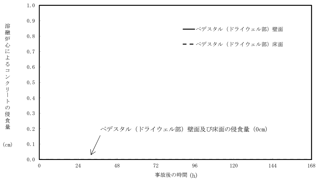
第 3.5-11 図 ペDESTAL (ドライウエル部) の 壁面及び床面のコンクリート侵食量の推移
