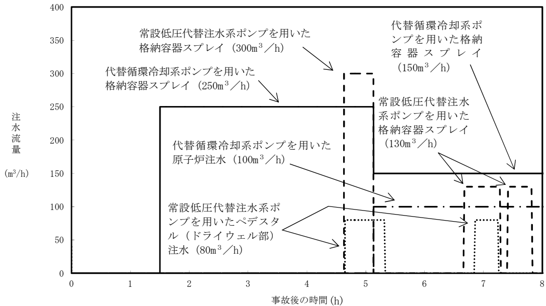
第 3.3-6 図 注水流量の推移
