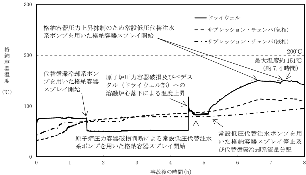
第 3.3-4 図 格納容器雰囲気温度の推移
