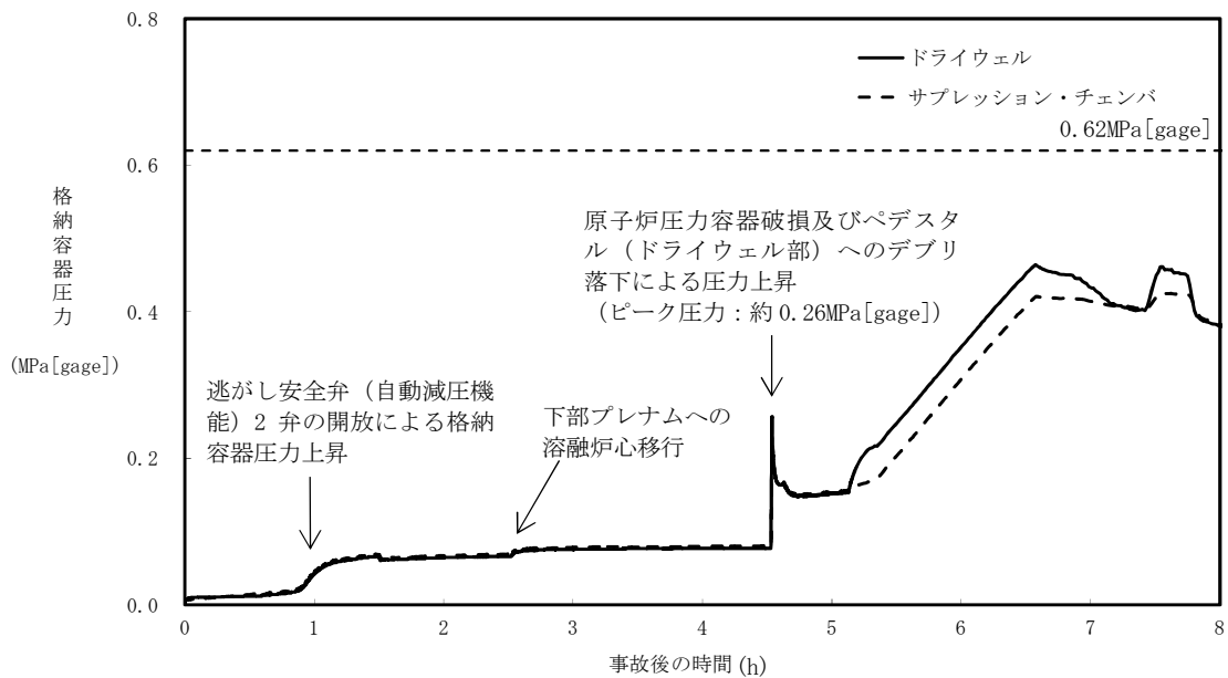
第3.3-8図 格納容器圧力の推移 (感度解析ケース (エントレインメント係数最大値) )
