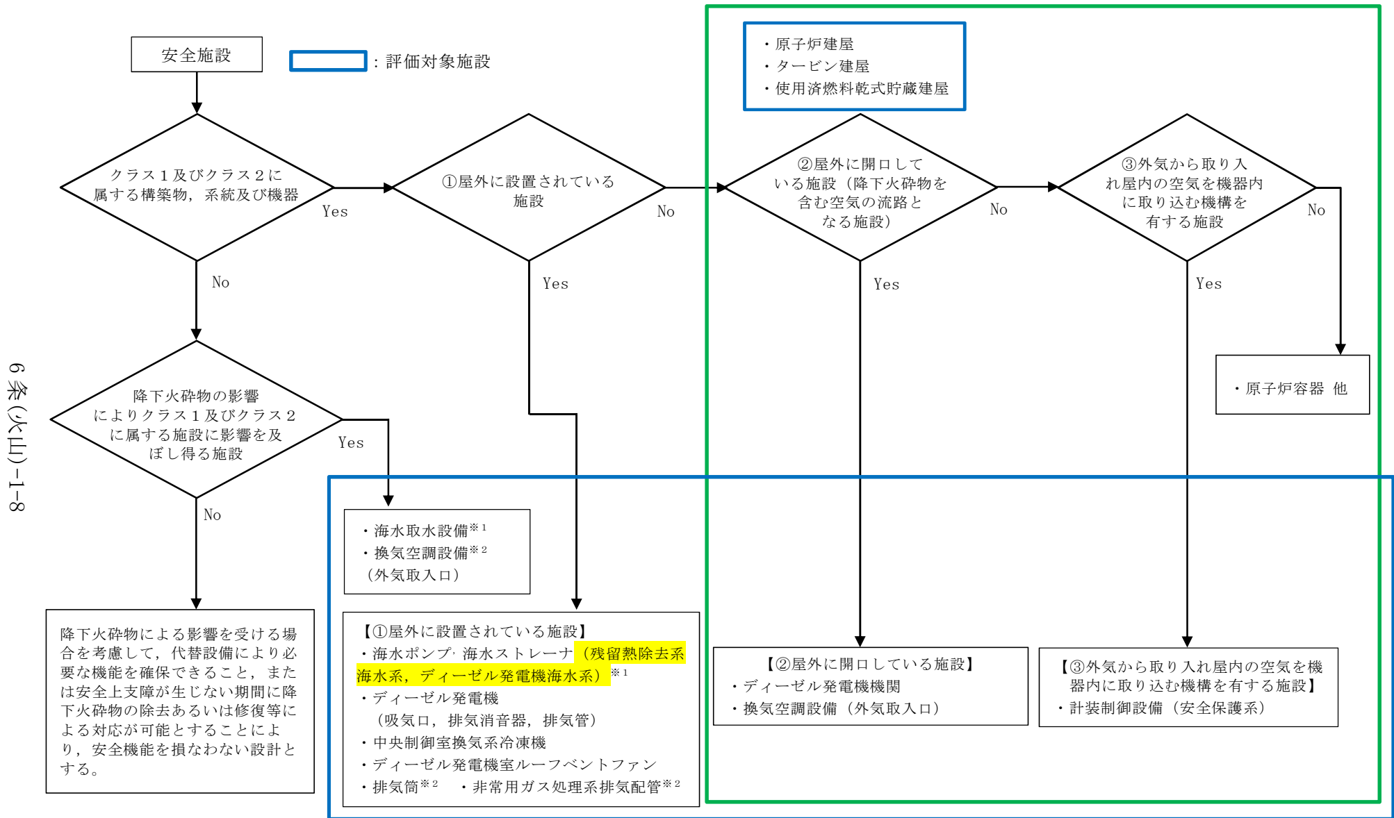
第3.3-1図 評価対象施設の抽出フロー
