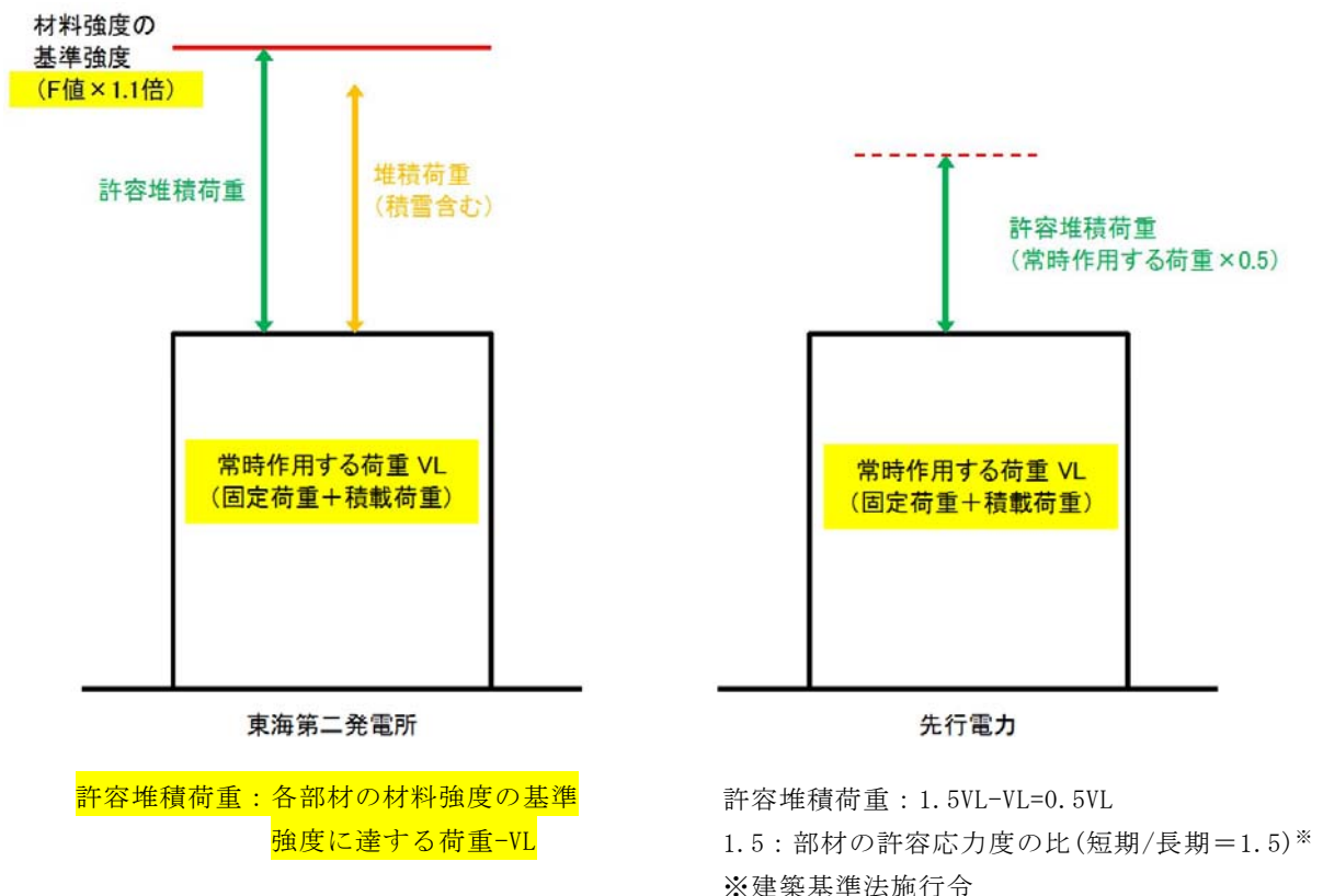
図 1 許容堆積荷重の考え方 イメージ図
