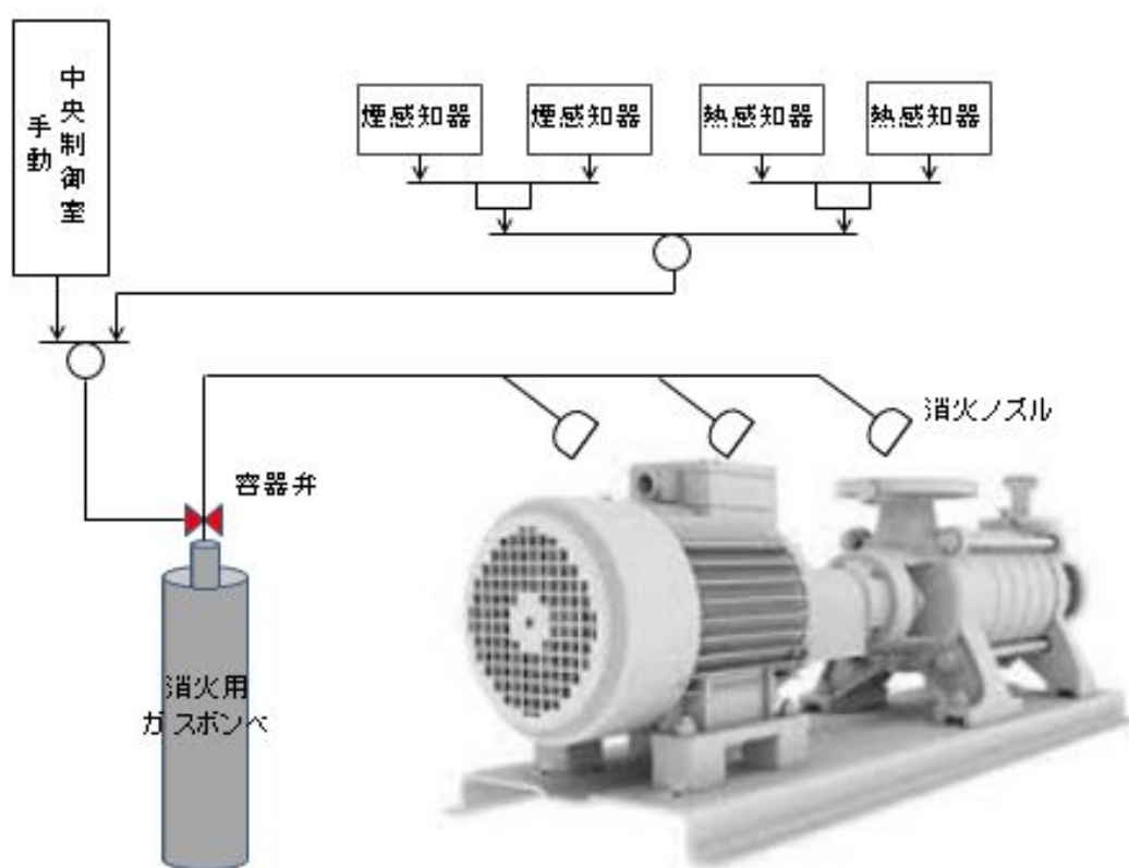
第3図 固定式のハロゲン化物自動消火設備 (局所) の概要
