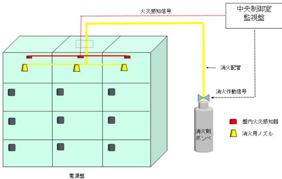
第4図 電源盤に対する固定式のハロゲン化物自動消火設備（局所）の概要
