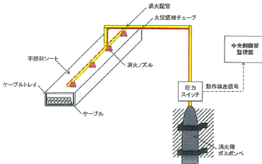
電気品消火設備の例（ケーブルトレイを例示）
