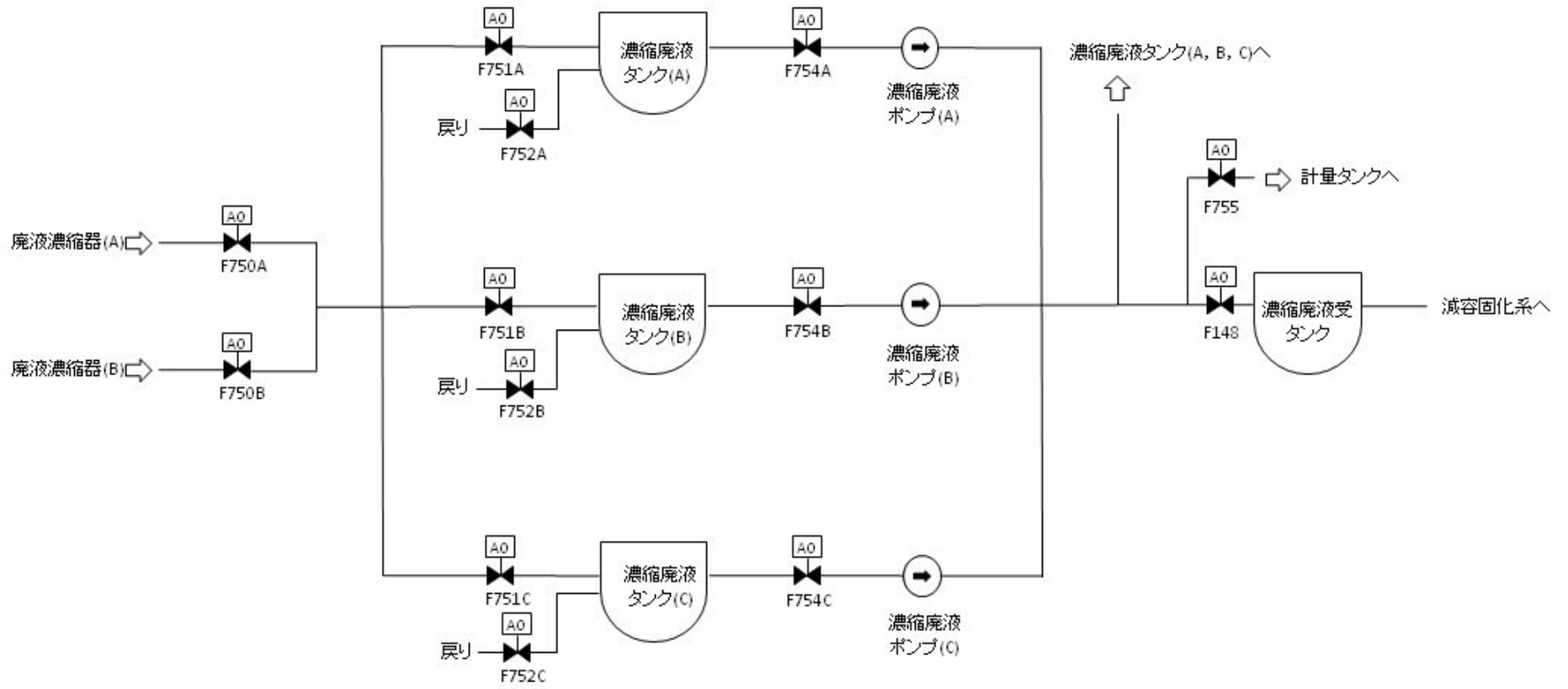
第9-10図 濃縮廃液系 系統概略図
