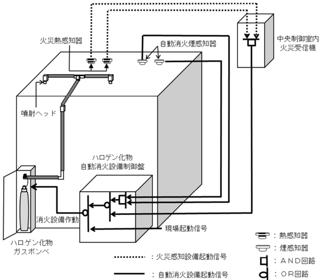
第1図 ハロゲン化物自動消火設備（全域）動作概要
