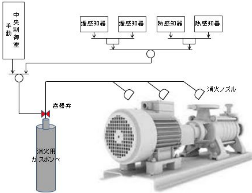
油内包機器に対する消火設備の例
