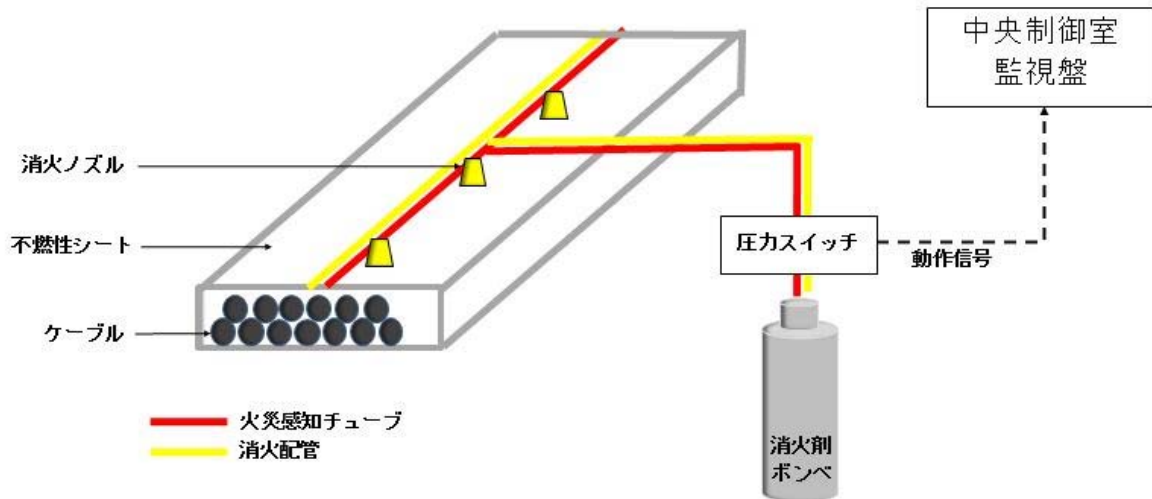
第5図 ケーブルトレイに対するハロゲン化物自動消火設備（局所）の概要
