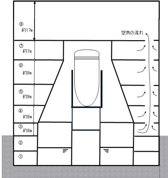
第1図 原子炉建屋断面図
