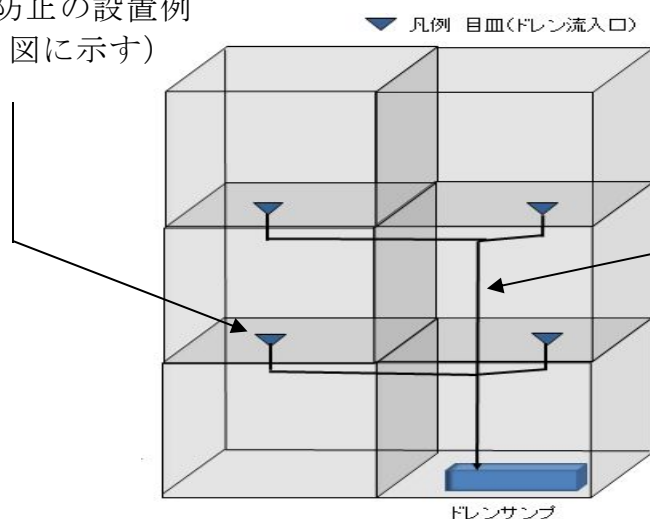
第1図 建屋内排水系統概要
