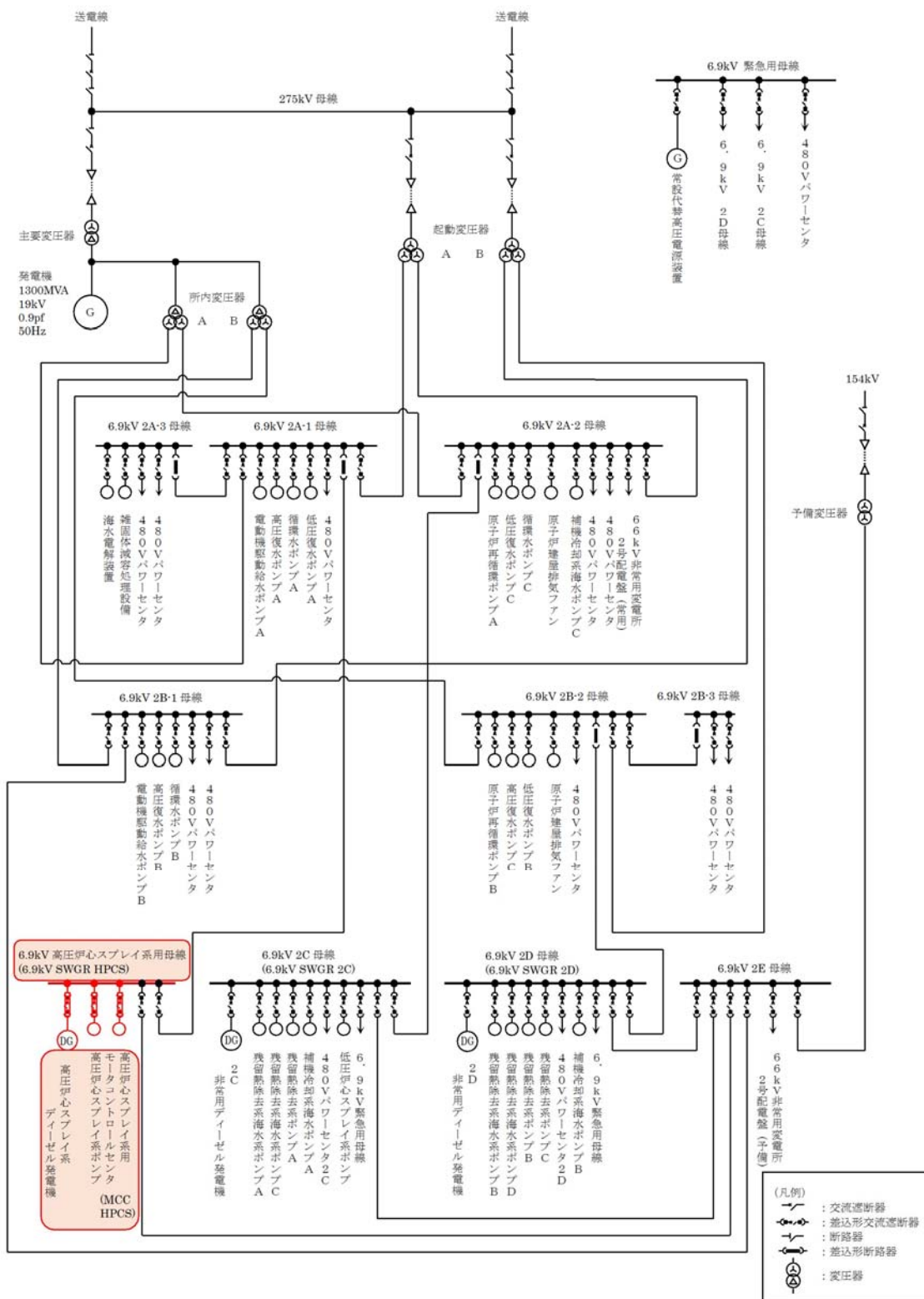
第 12 図 非常用電源系 (SWGR, P/C(HPCS))
