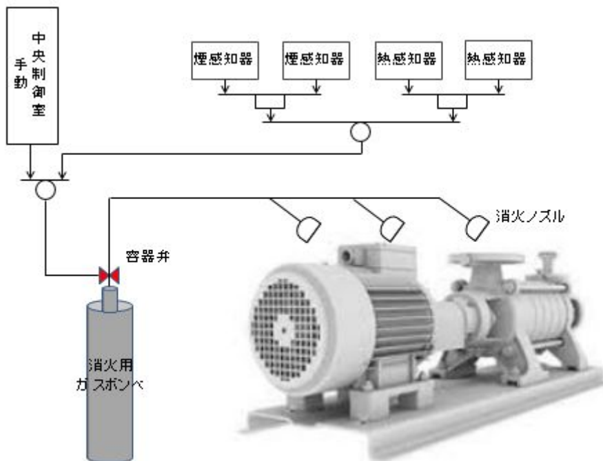
第1図 ハロゲン化物自動消火設備（全域）動作概要
