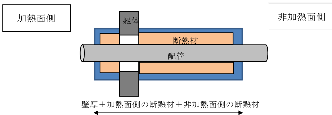
第5図 耐火対策イメージ
