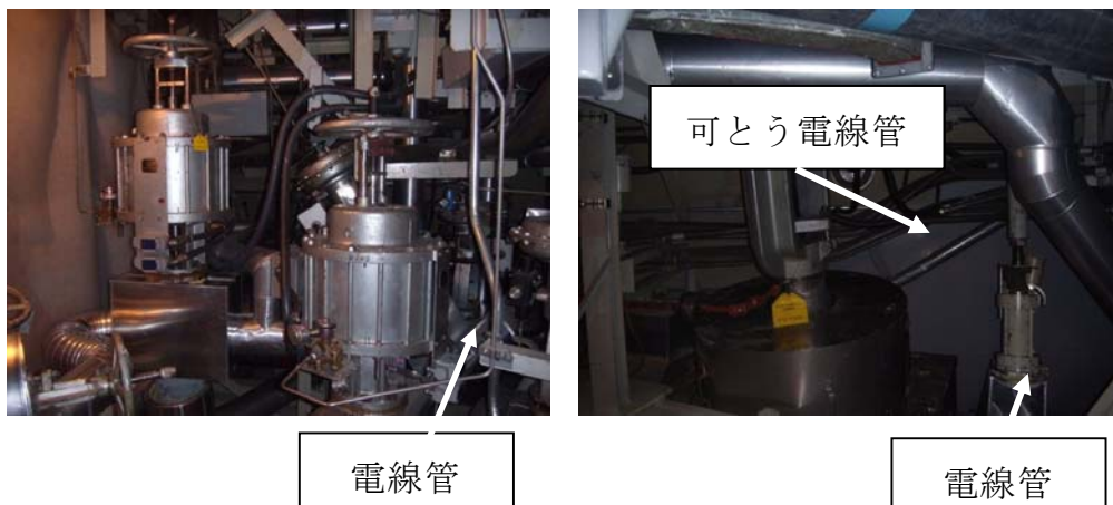
第 8-12 格納容器内の機器等の設置状況
