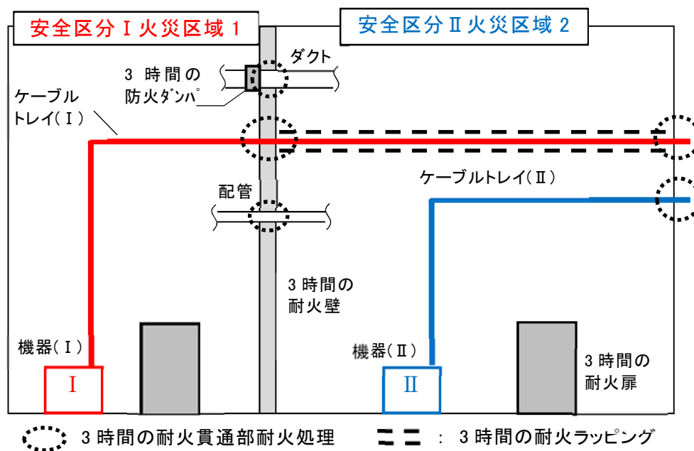
第 7-2 図 火災の影響軽減対策のイメージ
