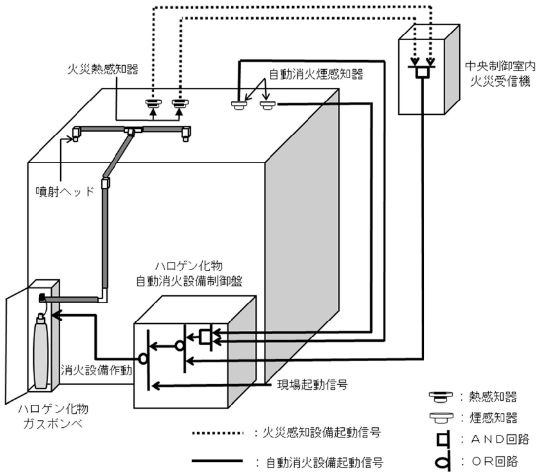
第10.5.1図 ハロゲン化物自動消火設備 (全域) (ハロン1301) 概要図
