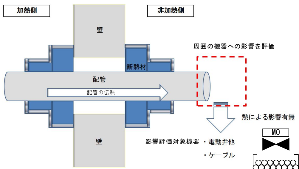
第1図 非加熱面側の貫通配管周囲の機器への伝熱影響
