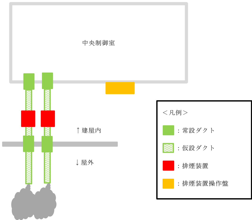
図1 中央制御室排煙設備概要
