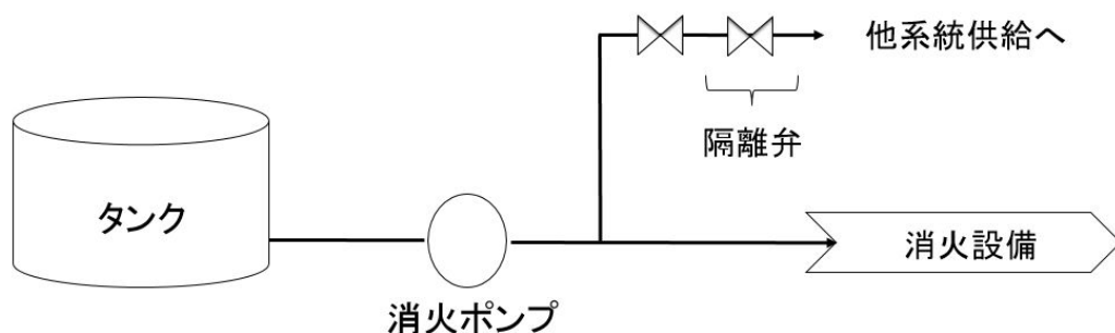
第1-29 消火水系の優先供給の概略図
