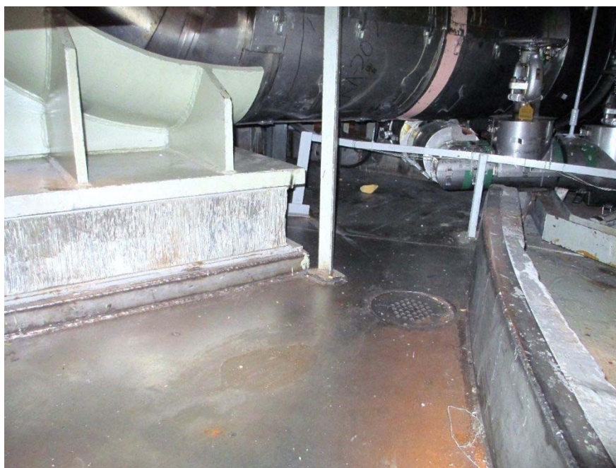
第 8-2 図 原子炉再循環系流量制御弁用の油受堰
