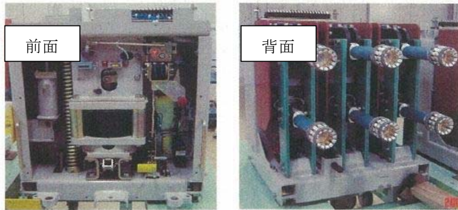
第1-13図 真空遮断器外観
