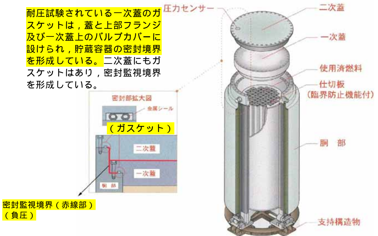
第 3-1 図 貯蔵容器の蓋部詳細
