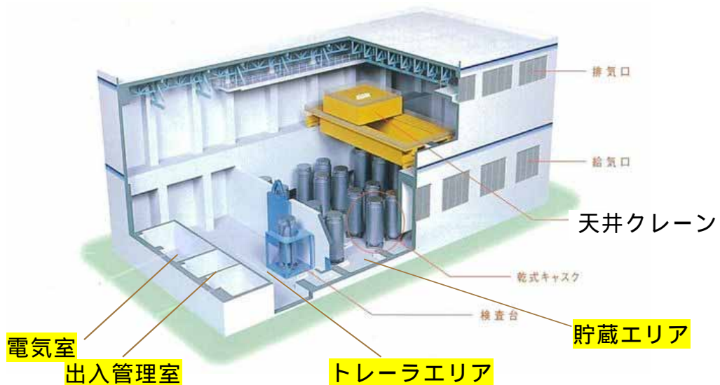
第 4 図 貯蔵建屋概念図
