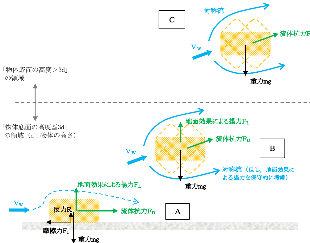
第 5.1-3 図 物体の運動モデルの模式図
