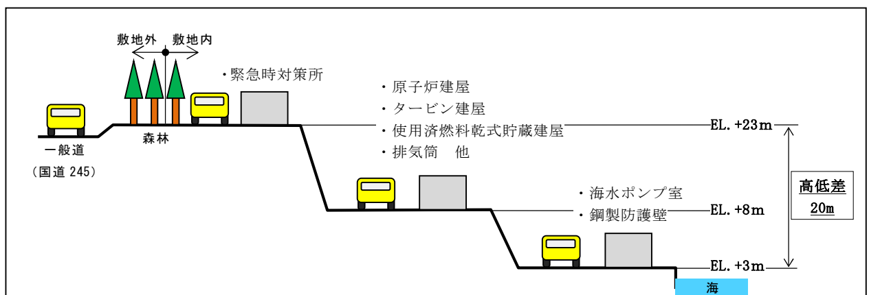
別図3-1 竜巻防護施設等と車両の存在場所との高さ関係
