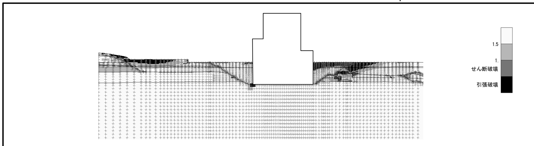
地盤の局所安全係数及びモビライズド面
