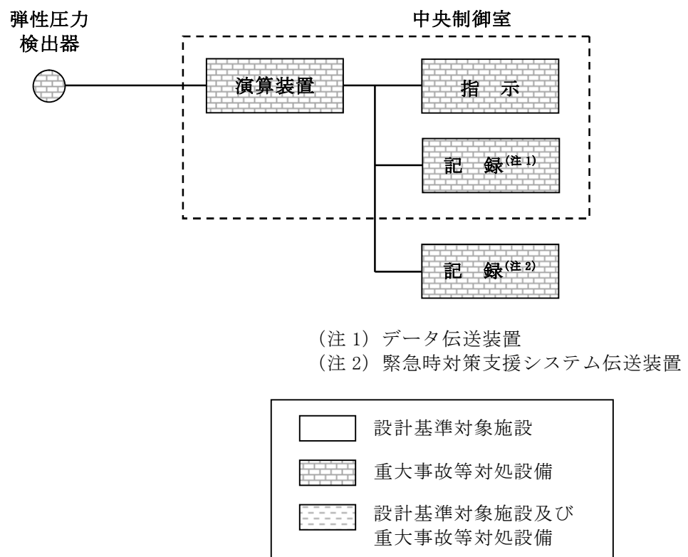
第 58-6-5 図 代替循環冷却系ポンプ吐出圧力の概略構成図
