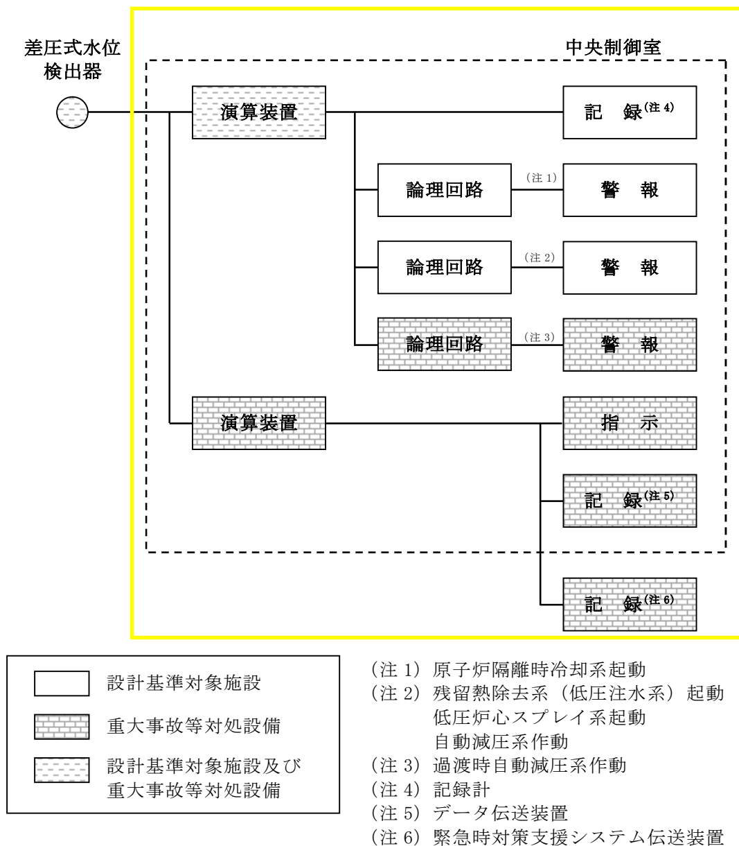
第 58-6-22 図 原子炉水位（広帯域）の概略構成図
