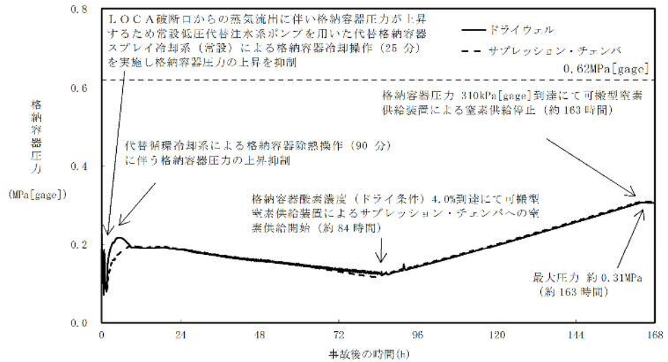
第 58-7-14 図 「雰囲気圧力・温度による静的負荷（格納容器過圧・過温破損）」 において代替循環冷却を使用する場合の格納容器内圧力変化
