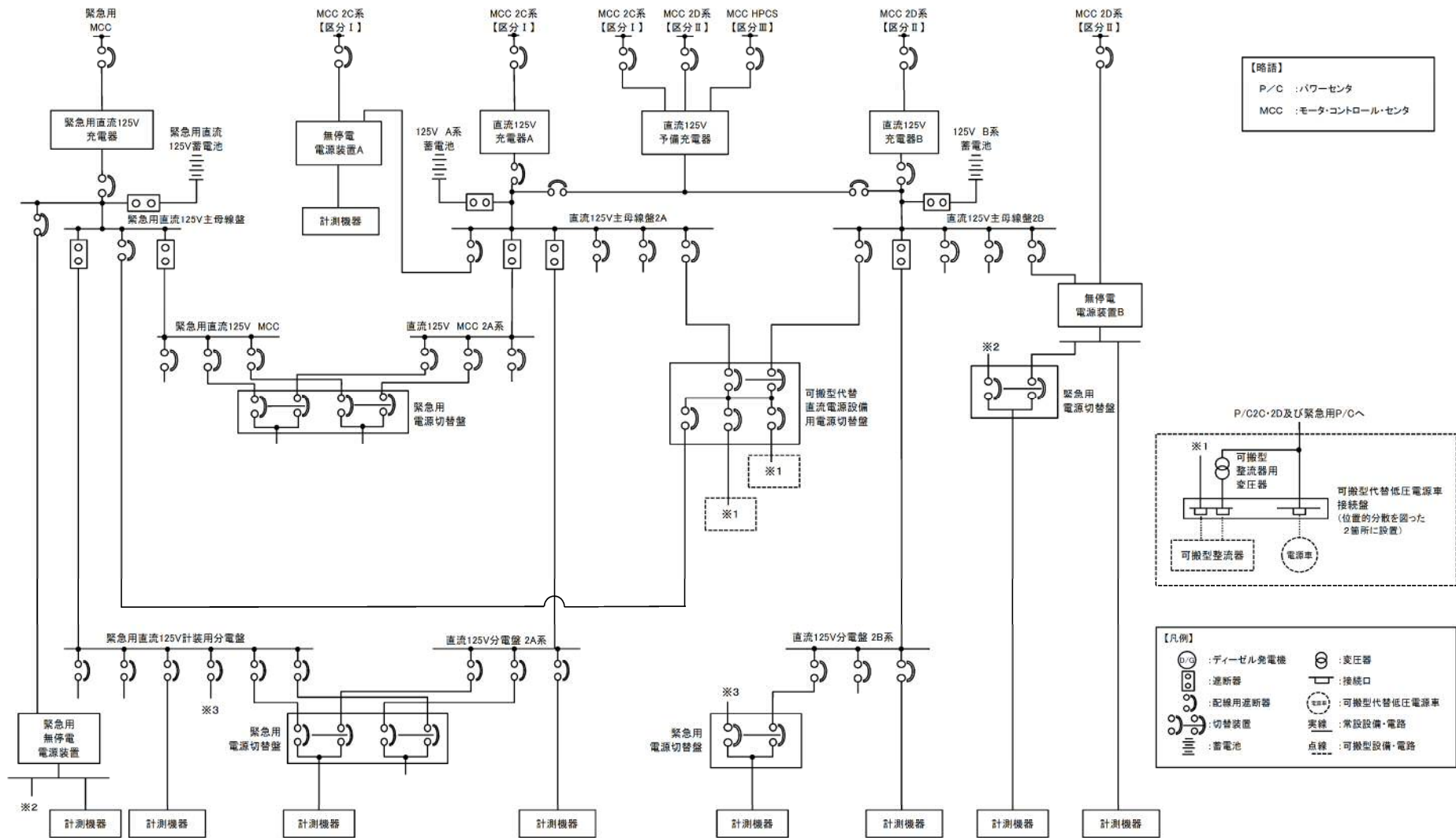
第 58-2-1 図 単線結線図 (直流) (1/3)
