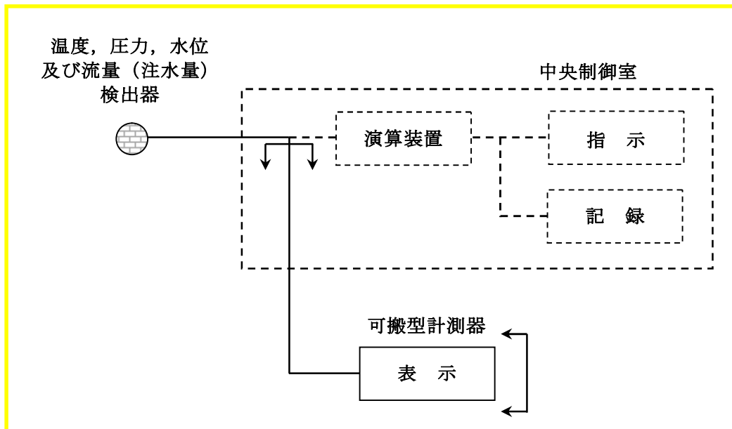
第 58-6-57 図 可搬型計測器の概略構成図
