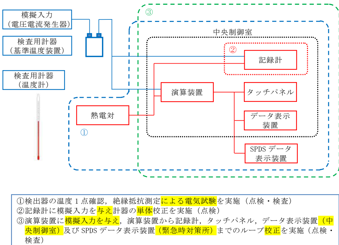
第 58-5-6 図 温度計の試験及び検査
