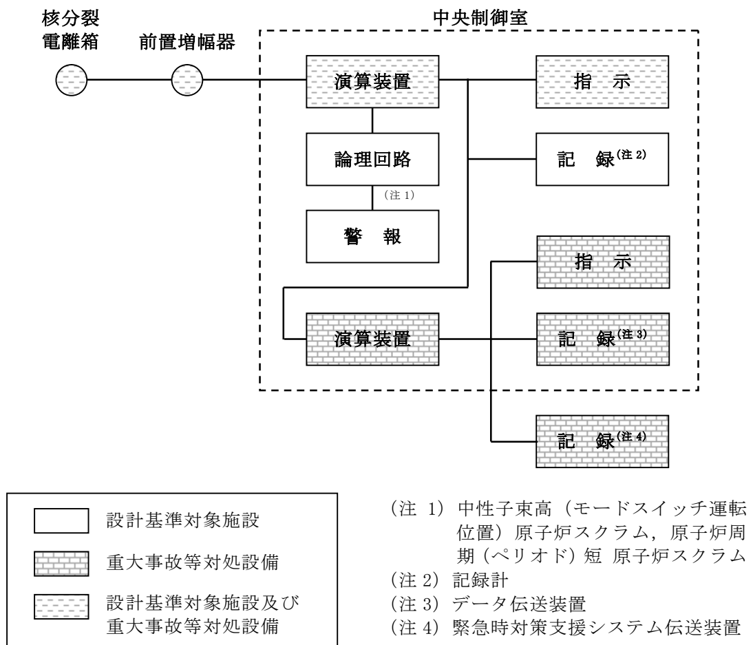
第 58-6-1 図 起動領域計装の概略構成図
