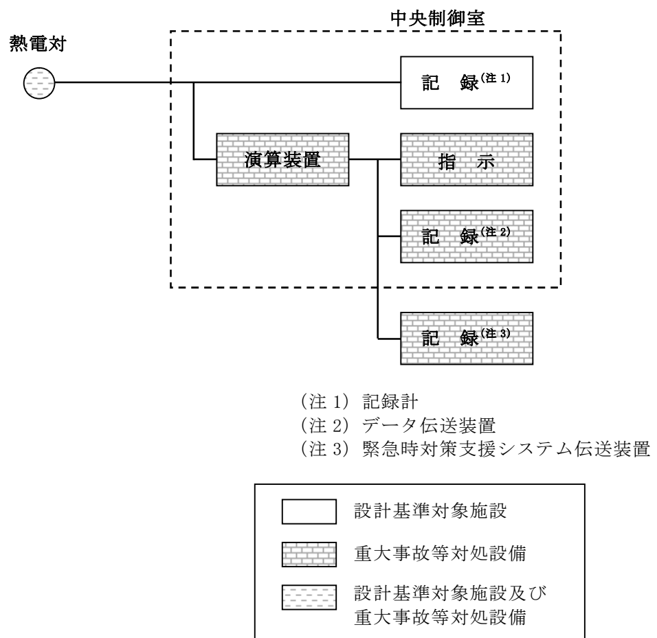
第 58-6-11 図 残留熱除去系熱交換器入口温度の概略構成図
