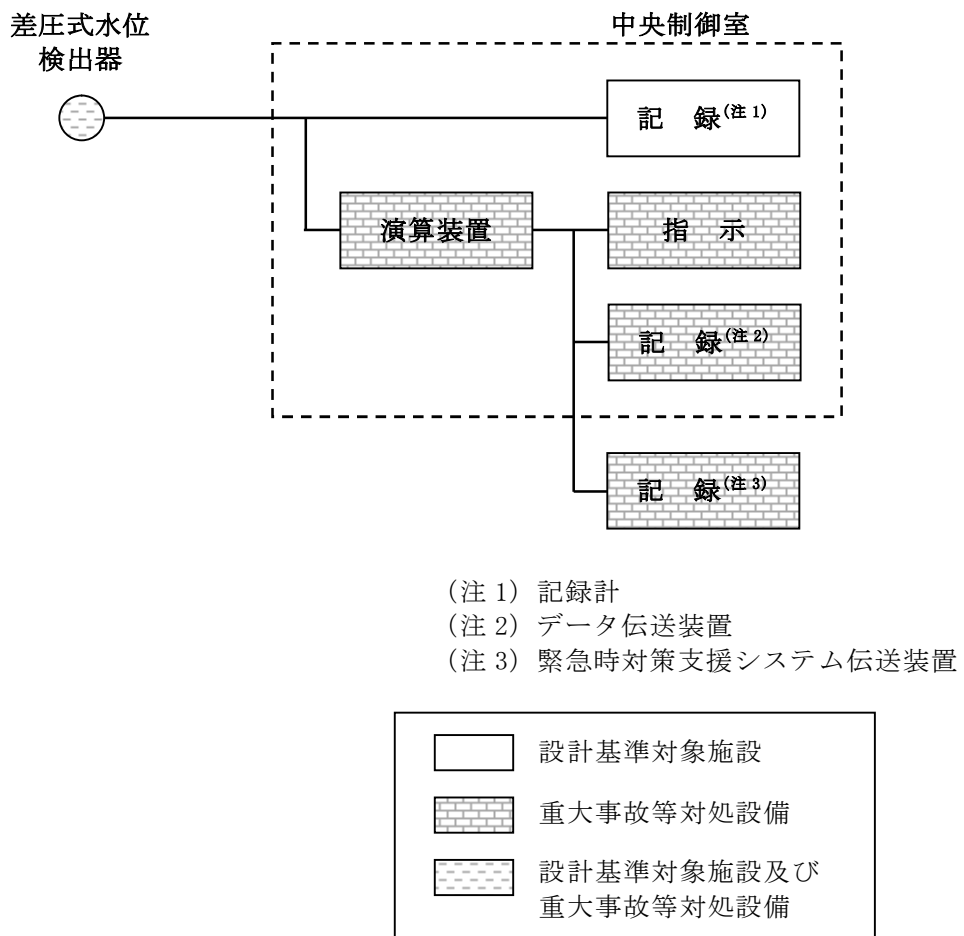
第 58-6-23 図 原子炉水位（燃料域）の概略構成図
