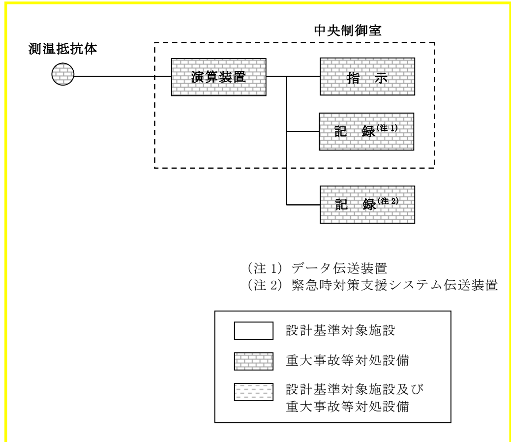
第 58-6-30 図 格納容器下部水温の概略構成図
