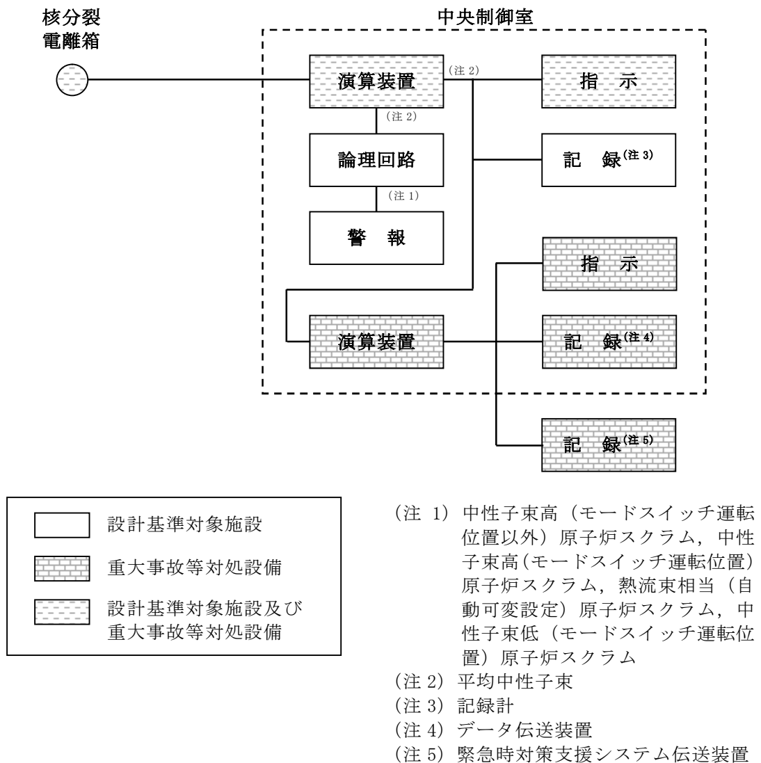
第 58-6-2 図 平均出力領域計装の概略構成図
