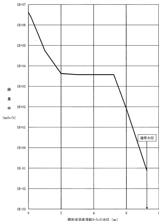
第 58-7-18 図 水位と放射線量率の関係
