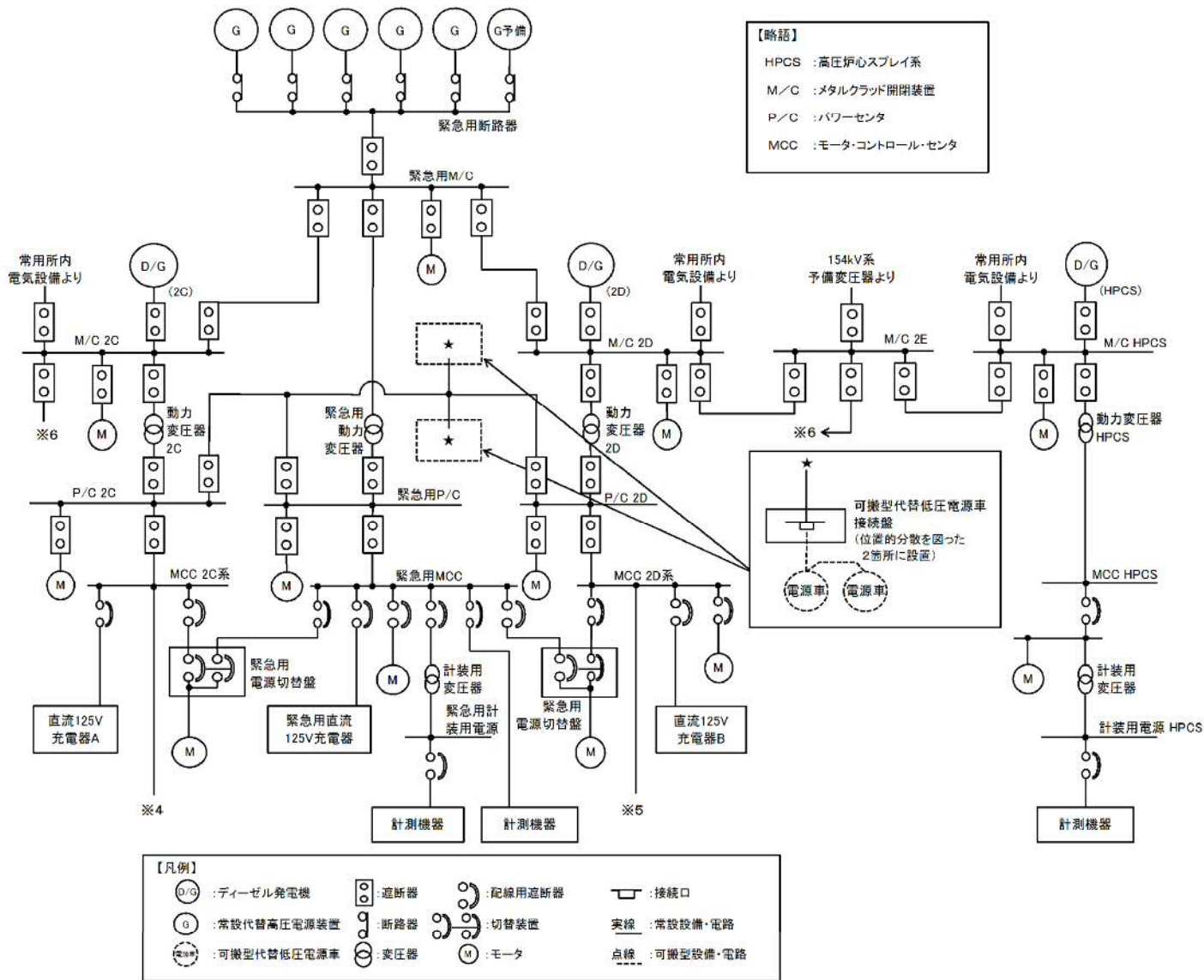
第 58-2-3 図 単線結線図 (交流) (3/3)
