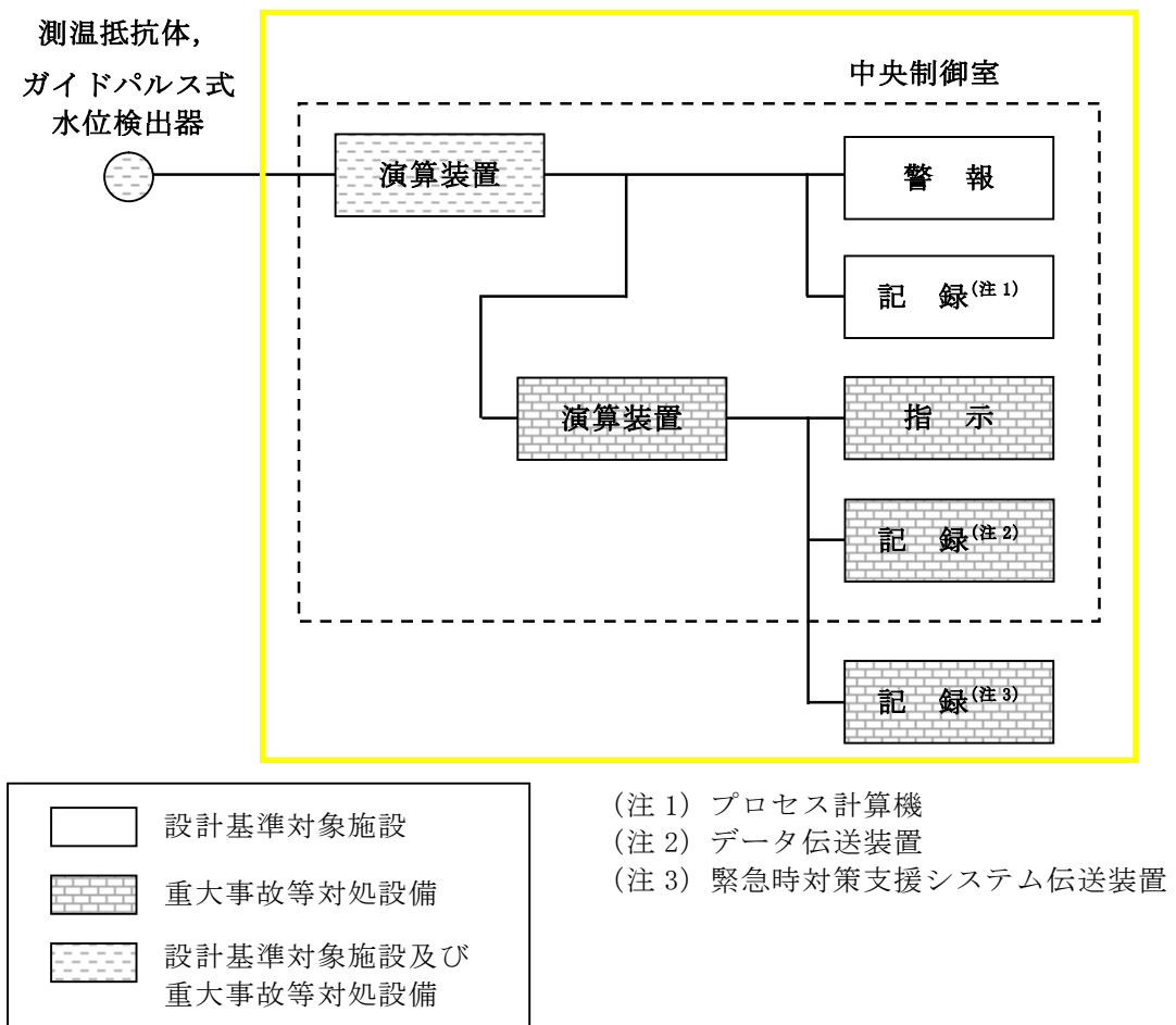
第 58-6-54 図 使用済燃料プール水位・温度 (SA 広域) 概略構成図
