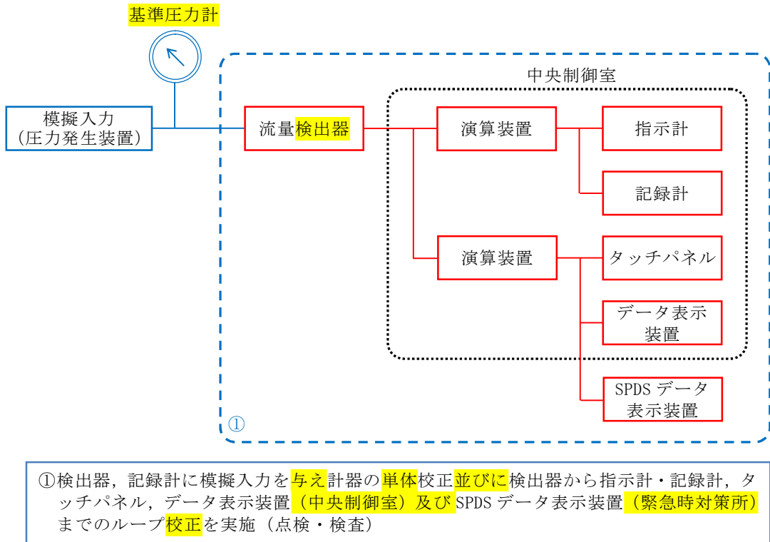
第 58-5-5 図 流量計の試験及び検査
