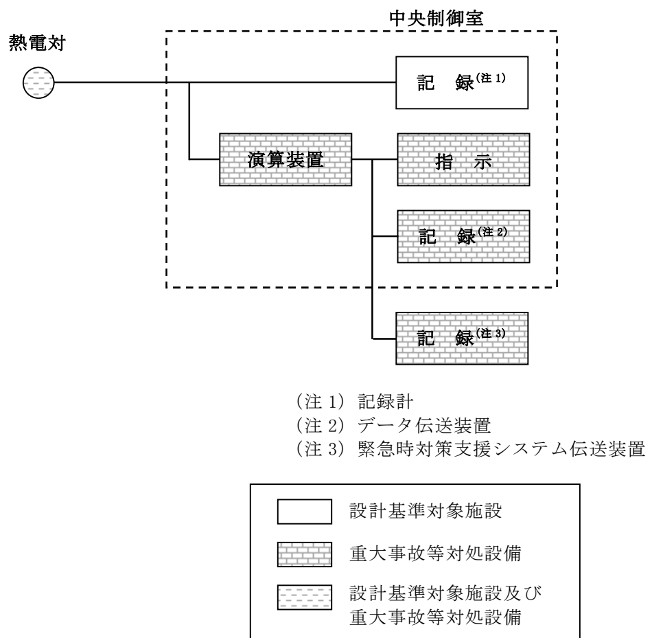
第 58-6-12 図 残留熱除去系熱交換器出口温度の概略構成図
