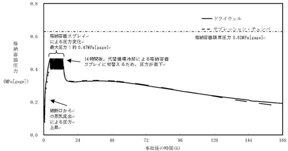
第 58-7-17 図 「雰囲気圧力・温度による静的負荷（格納容器過圧・過温破損）」 において代替循環冷却を使用する場合の格納容器内圧力変化
