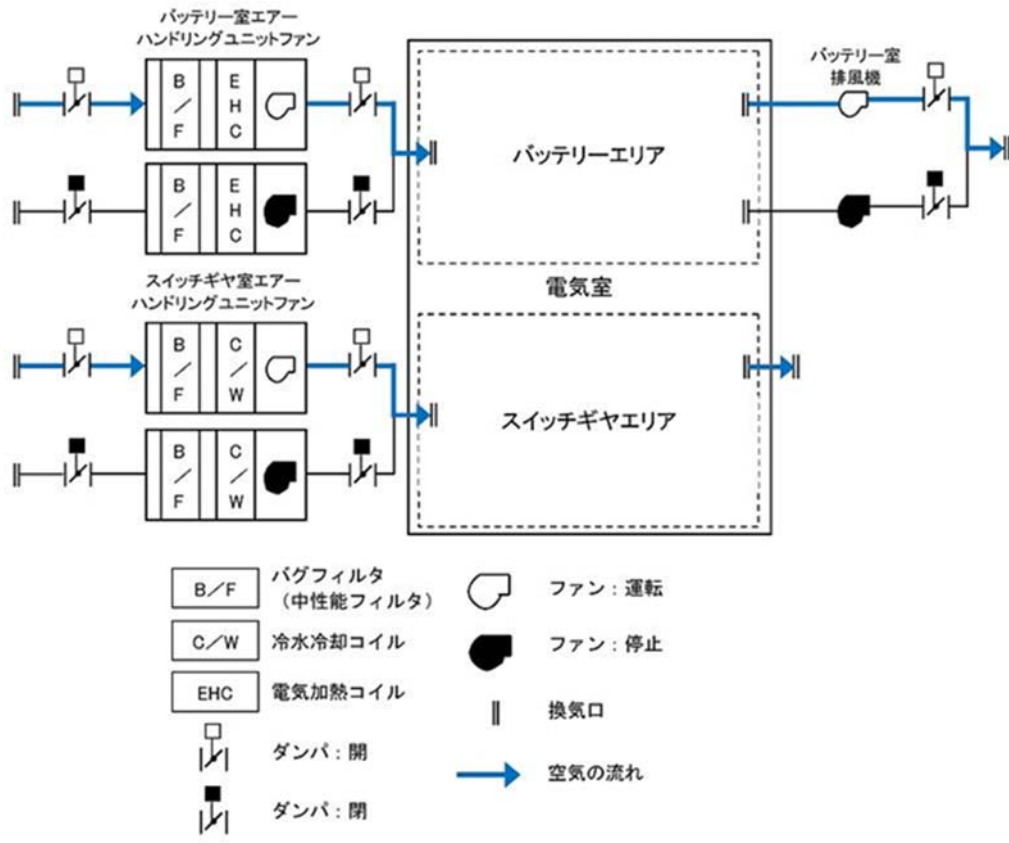
第 2.4.2-4 図 電気室換気系の系統概略図
