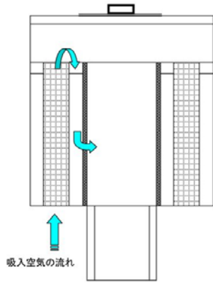
フィルタ構造 フィルタ
