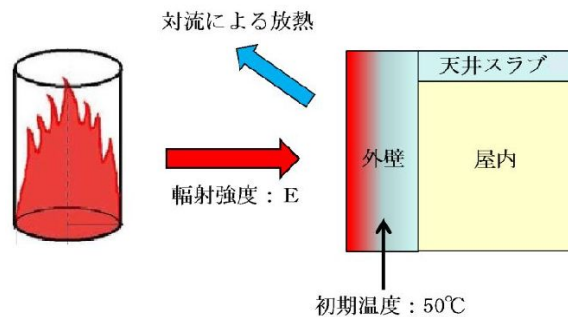
第 4.3.2.1-1 図 建屋外壁の評価概念図
