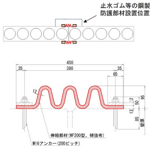
図3 止水ジョイント部の概要図
