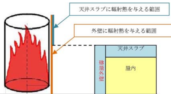
第 4.3.2.1-3 図 天井スラブへの輻射熱の影響
