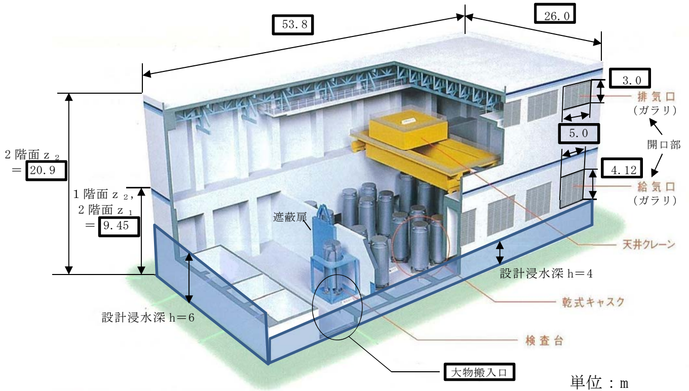
第 1-1 図 貯蔵建屋寸法等
