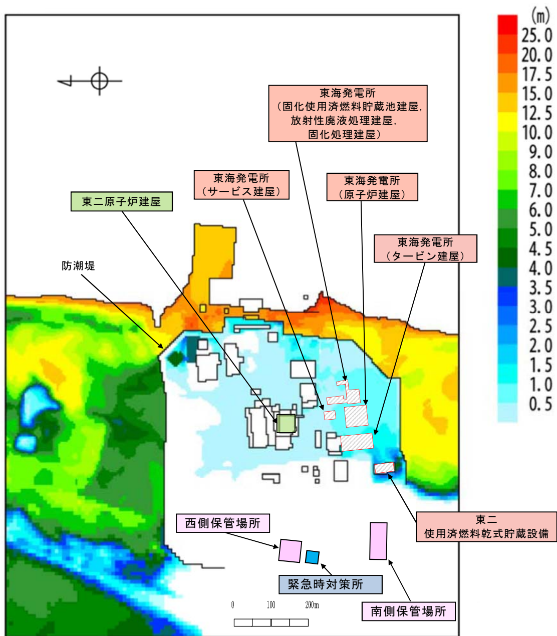
第 1.0.16-1 図 敷地遶上津波のシミュレーション結果（最大浸水深分布）
