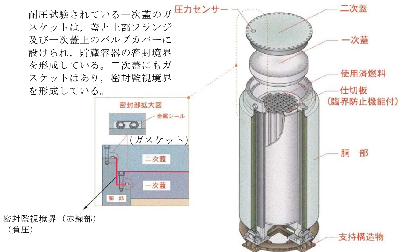
第 3-1 図 貯蔵容器の蓋部詳細
