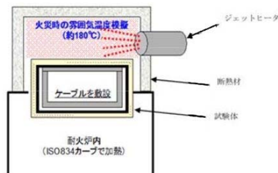
第3図 試験概要
