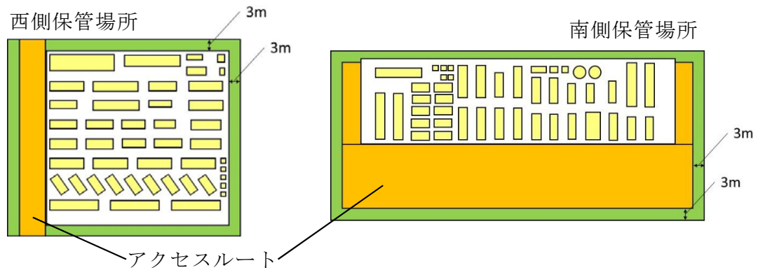
第 1-44 図 可搬型重大事故等対処設備の火災区域設定
