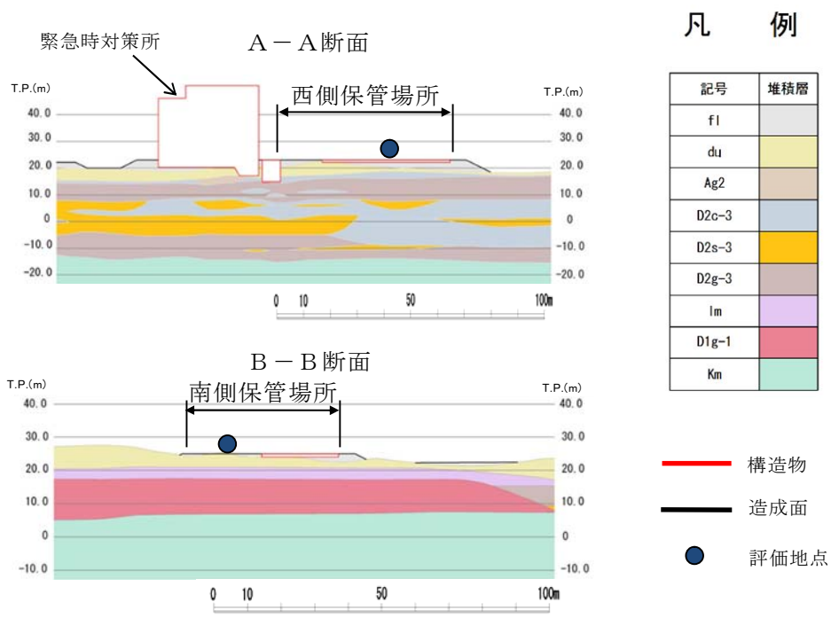
第 4.3.3-2 図 保管場所の液状化及び揺すり込みによる不等沈下に対する影響評価断面の位置図及び断面図
