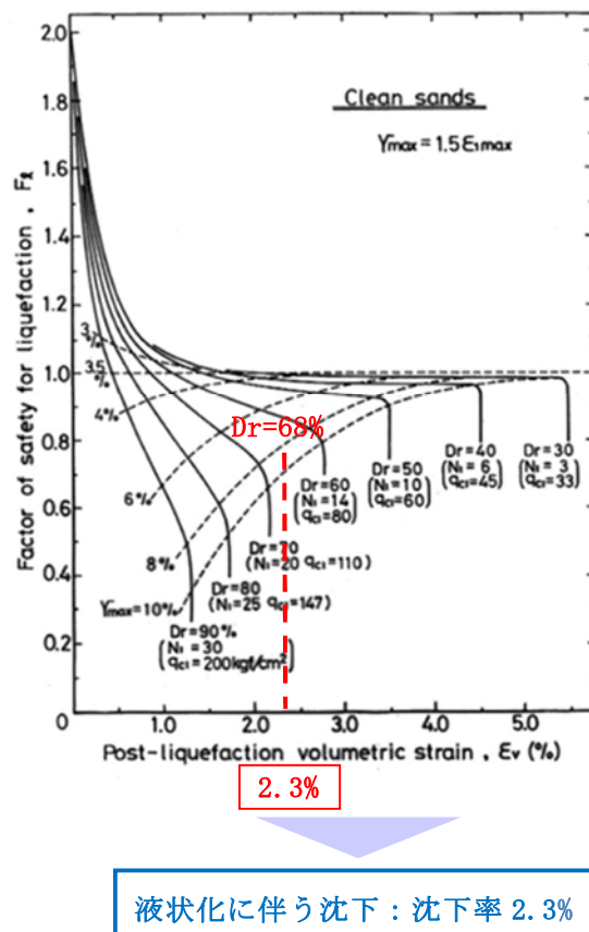
第5.4.3-3図 体積ひずみと液状化抵抗の関係及び想定する沈下率
