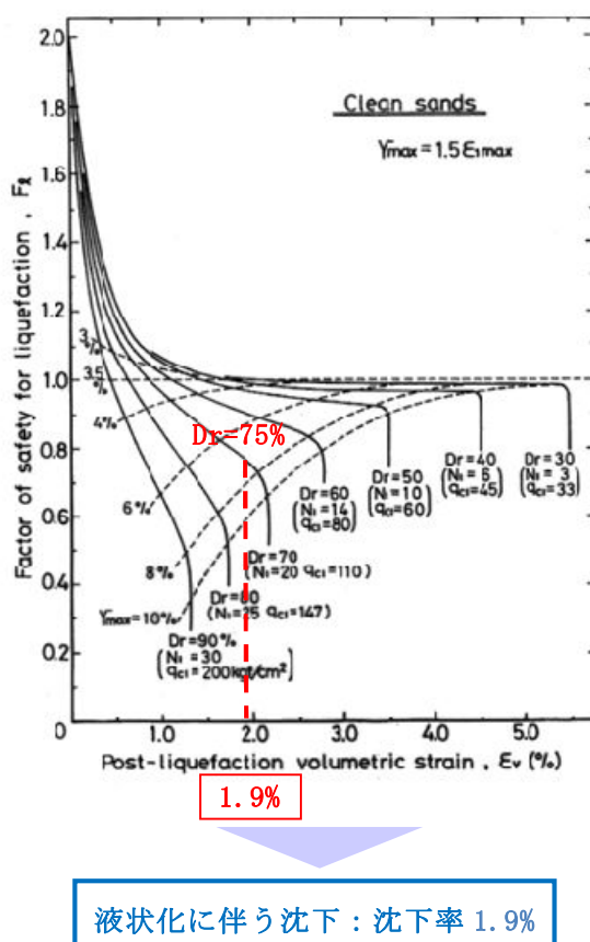
第 4. 3. 3-5 図 体積ひずみと液状化抵抗のj関係及び想定する沈下率
