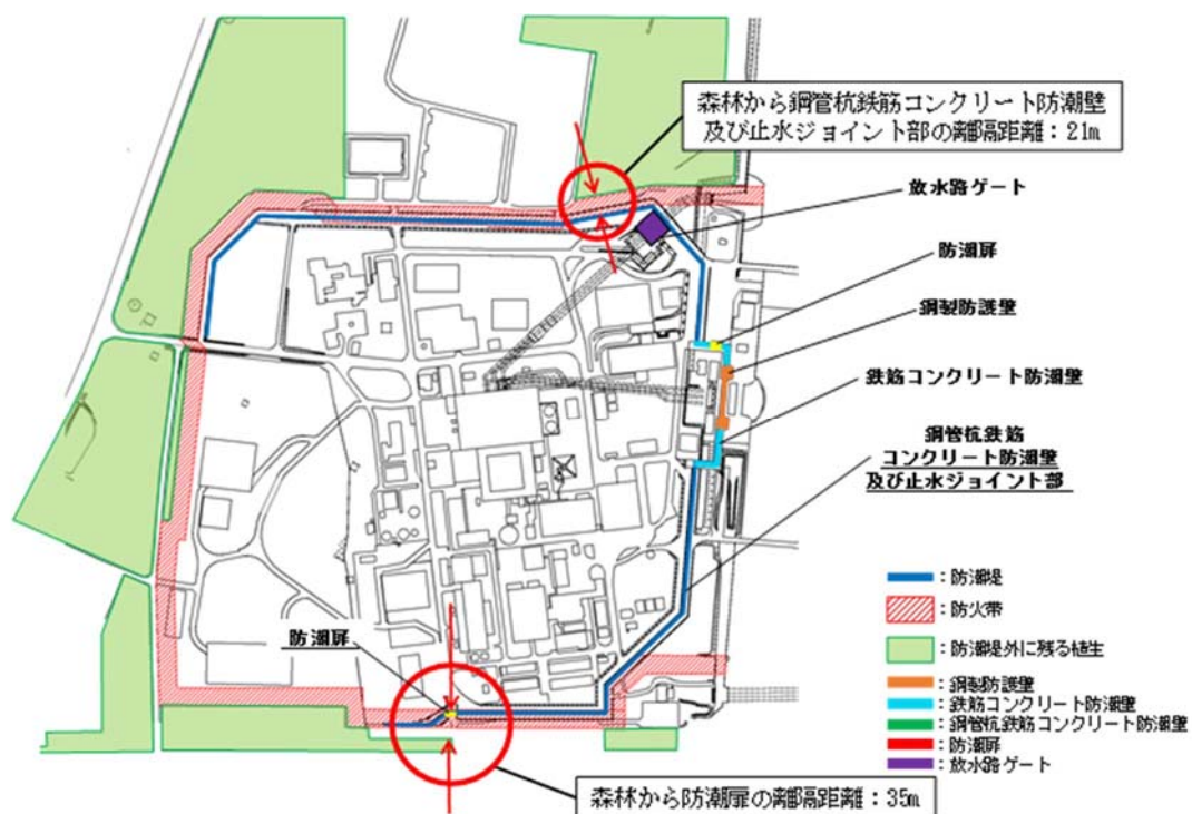
第 4. 2-3 図 防潮堤及び防火帯と近接する森林との位置関係
