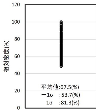
第 3 図 As 層（砂層）の相対密度
