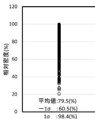
第 2 図 Ag2 層（砂礫層）の相対密度
