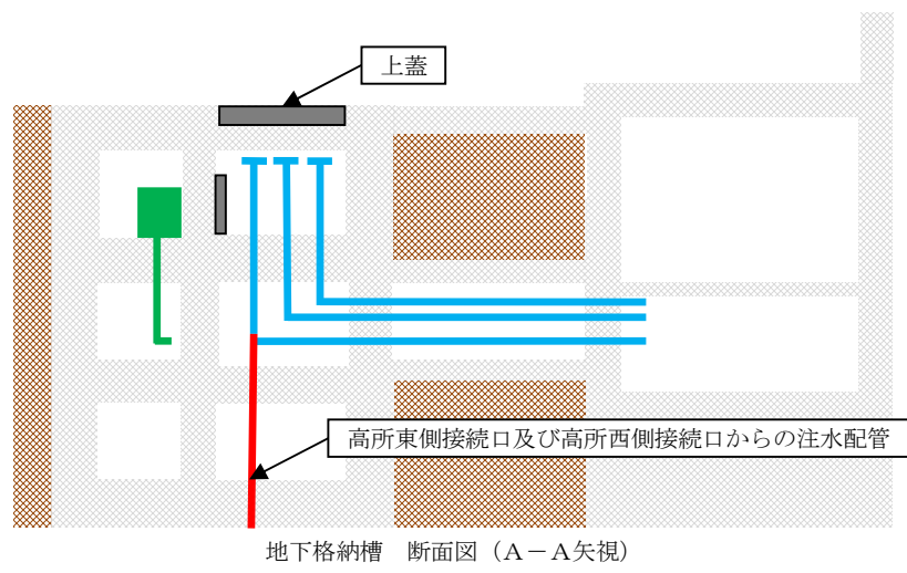
第5図 西側接続口の構造
