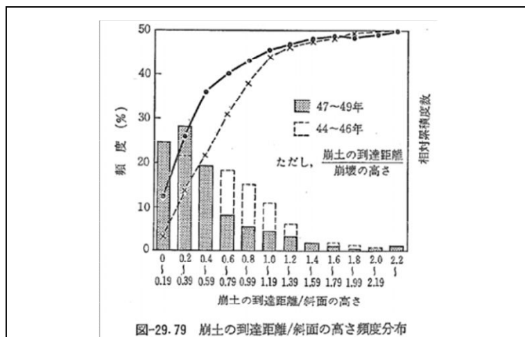
図-29.79 崩土の到達距離/斜面の高さ頻度分布
