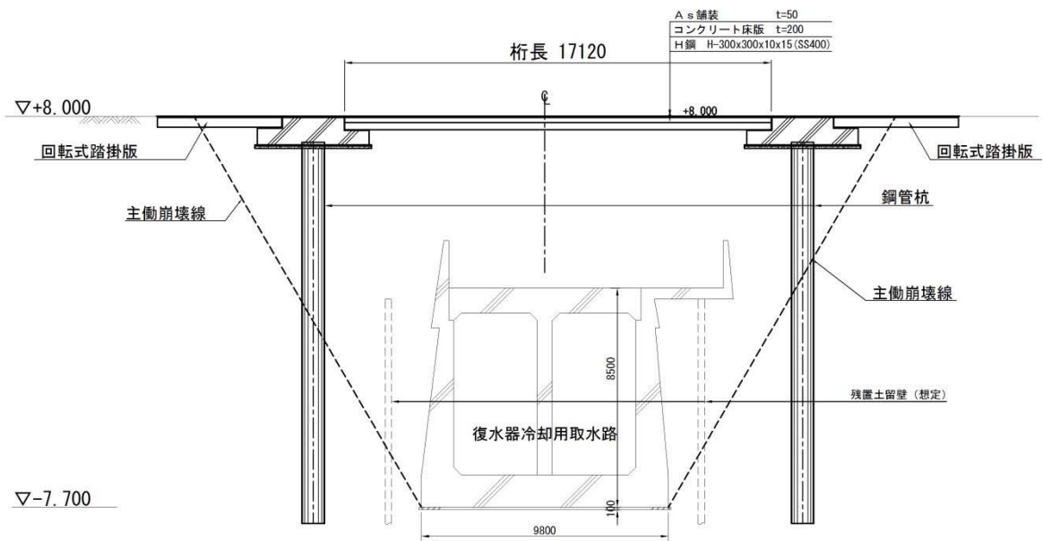
第1図 評価箇所断面図
