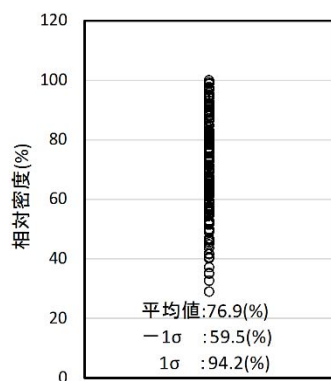
第 1 図 du 層（砂層）の相対密度
