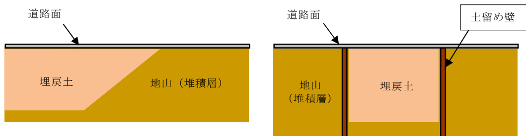
第 5.4.3-3 図 地山と埋戻部との境界の状況
