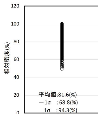
第 4 図 Ag1 層（砂礫層）の相対密度
