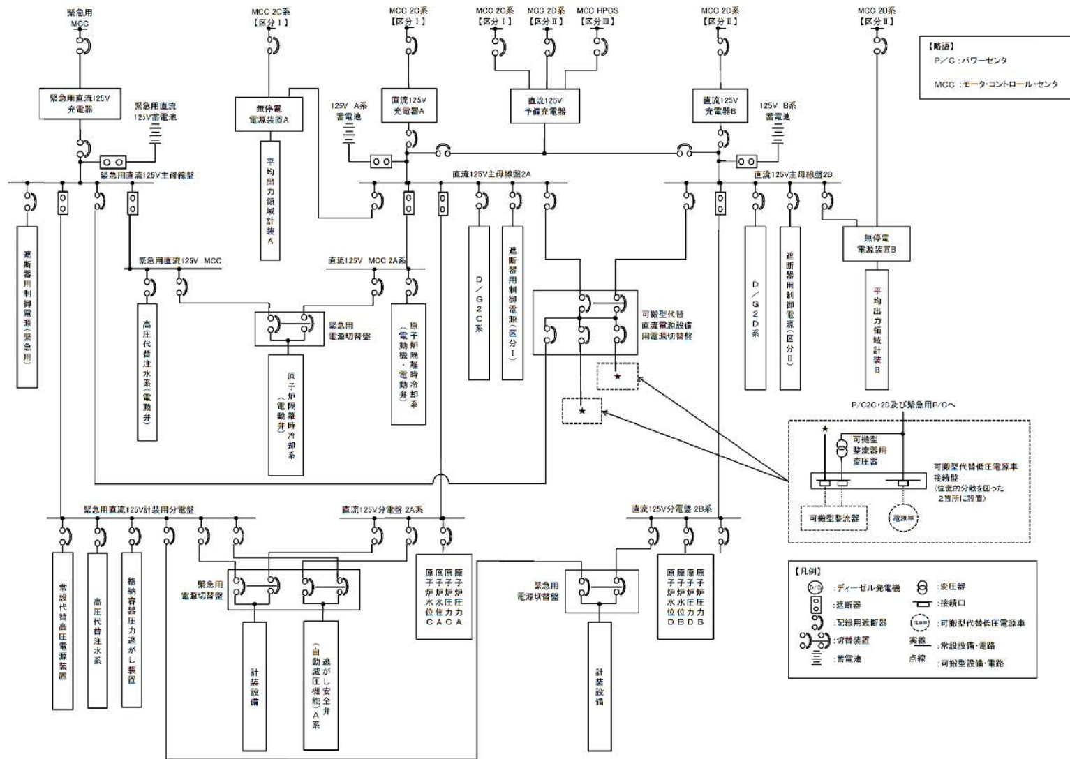
第 44-2-1 図 直流電源単線結線図
