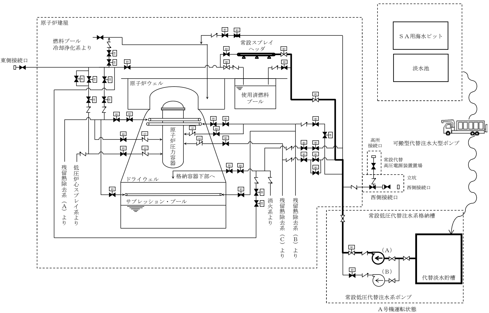
第 4.3-3 図 使用済燃料燃料プールの冷却等のための設備の系統概要図(3)
