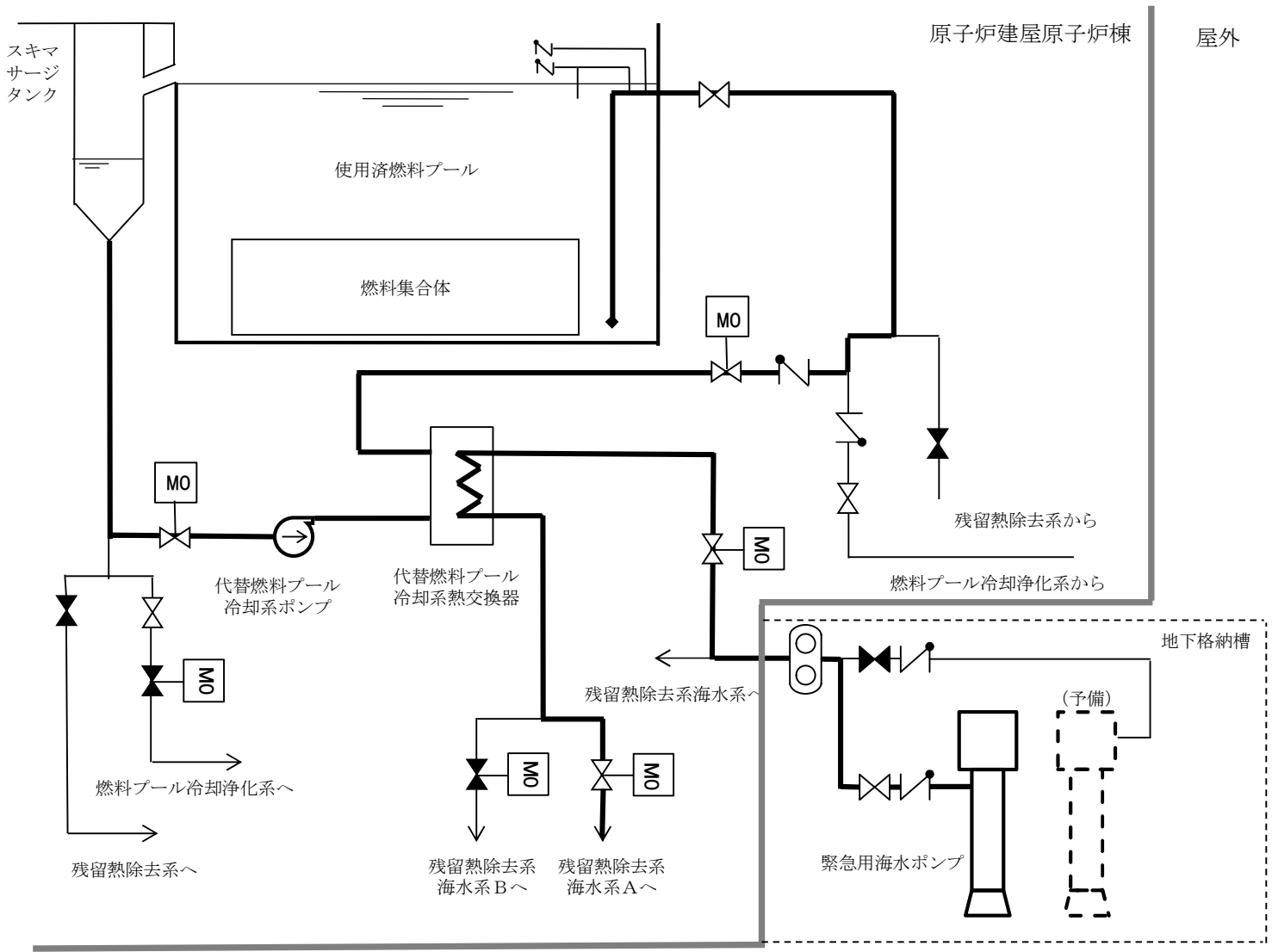
第 4.3-6 図 使用済燃料燃料プールの冷却等のための設備の系統概要図(6)
