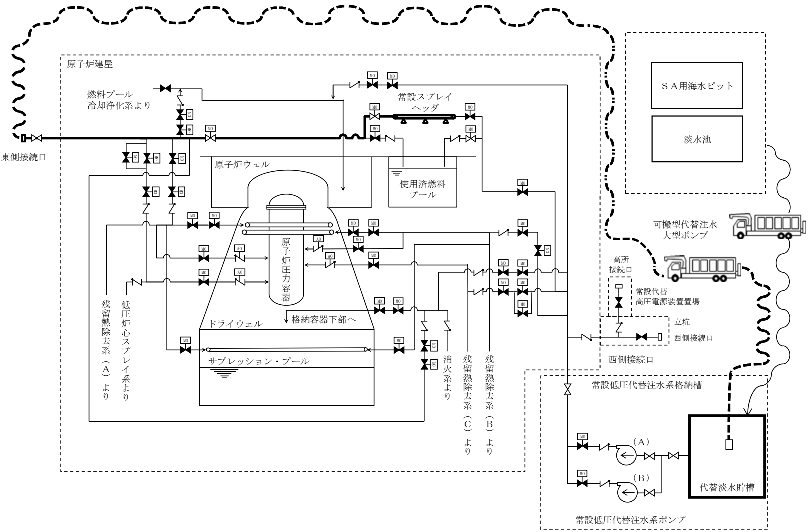
第 4.3-4 図 使用済燃料燃料プールの冷却等のための設備の系統概要図(4)
