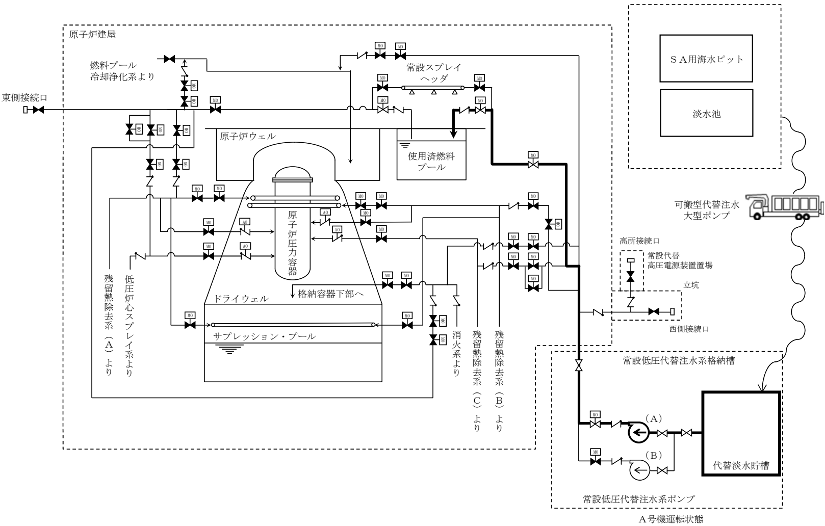
第 4.3-1 図 使用済燃料燃料プールの冷却等のための設備の系統概要図 (1)
