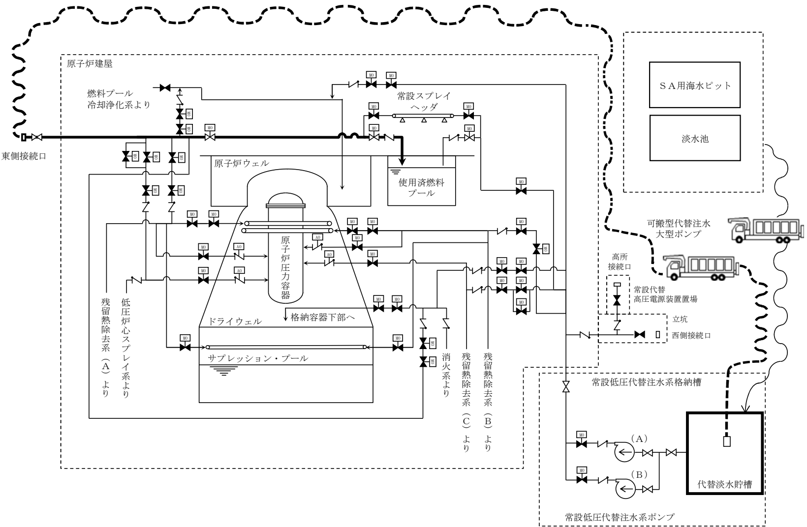
第 4.3-2 図 使用済燃料燃料プールの冷却等のための設備の系統概要図 (2)
