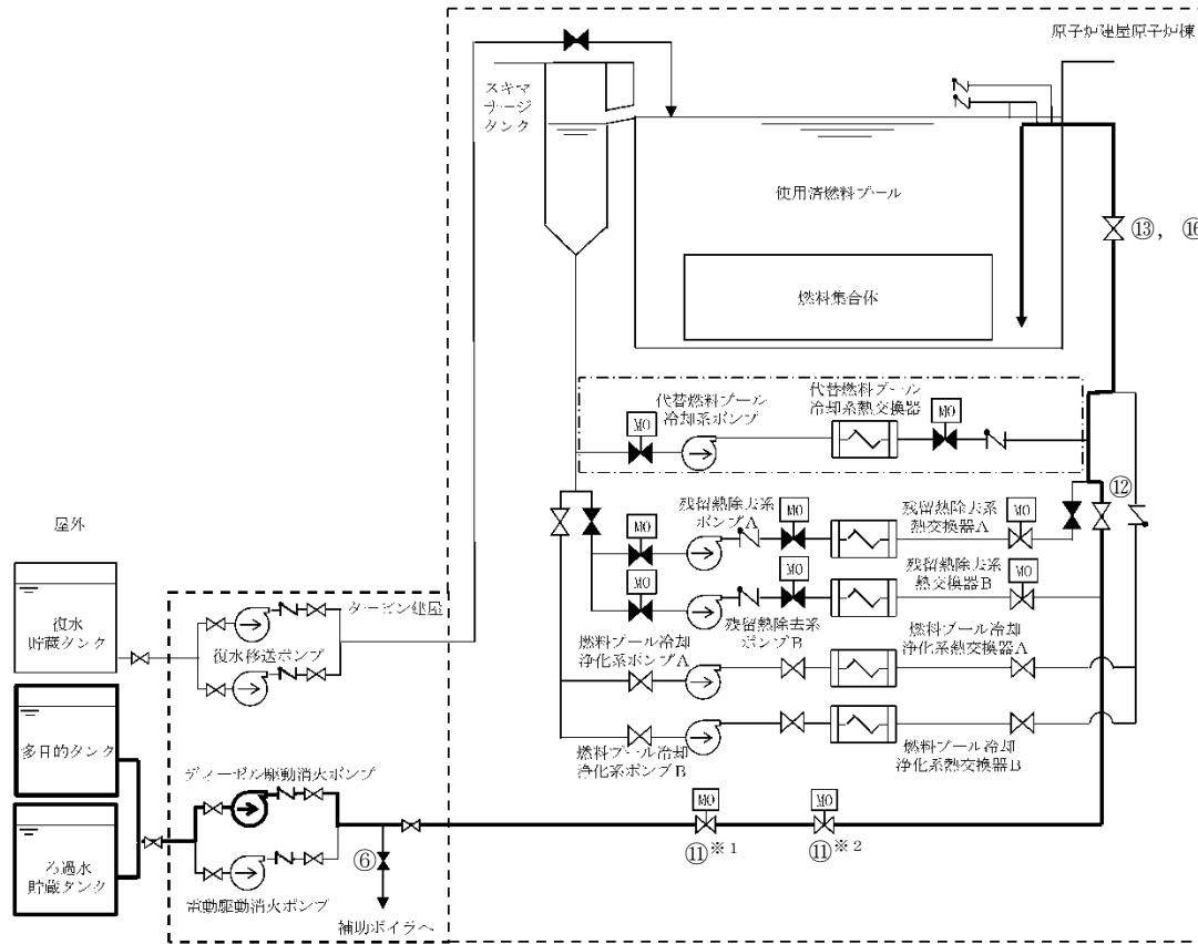
【残留熱除去系ラインを使用した使用済燃料プール注水の場合】
