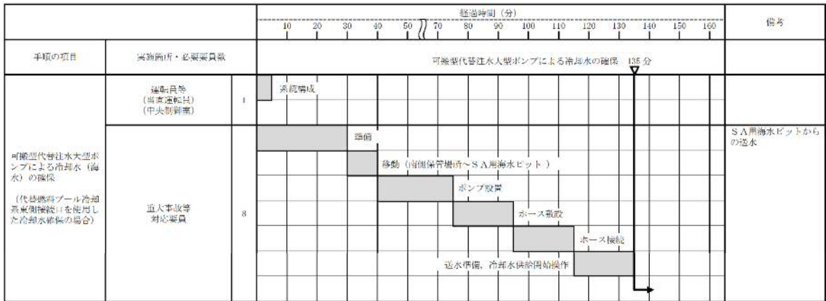
第1.11-24図 可搬型代替注水大型ポンプによる冷却水（海水）の確保 タイムチャート
